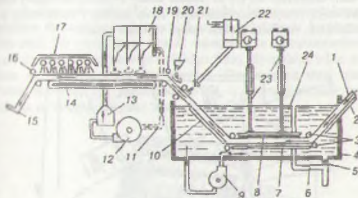
6.13-rasm. Tasmasli tashish qurilmasi bo'lgan FBQga ishlov beruvchi oqim tizimi.
