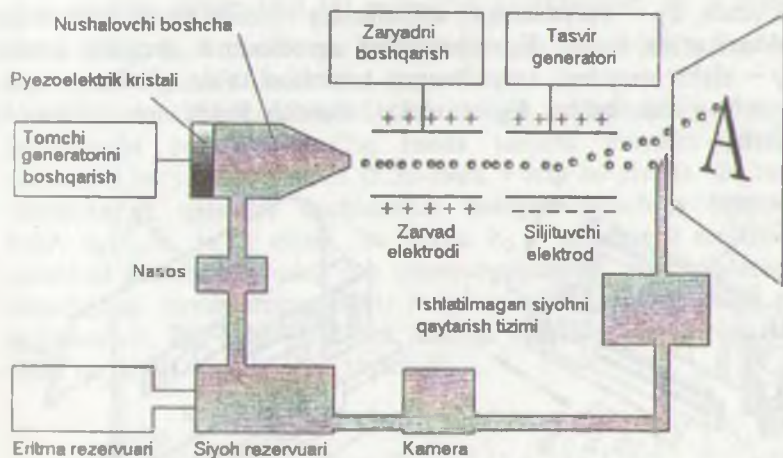
8.24-rasm. Uzlüksiz oqimli bosma printerining sxemasi.
