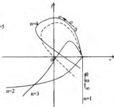
5.4-rasm. Nobarqaror sistemalar godograflari
