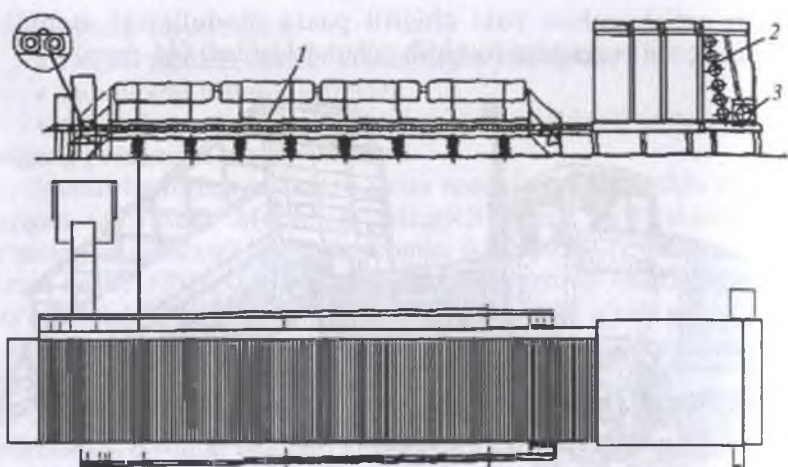
45-rasm. Qo'zg'almas modul buzgich: 1-valikli platforma loki; 2-qoziqli baraban; 3-olib ketuvchi shnek.
