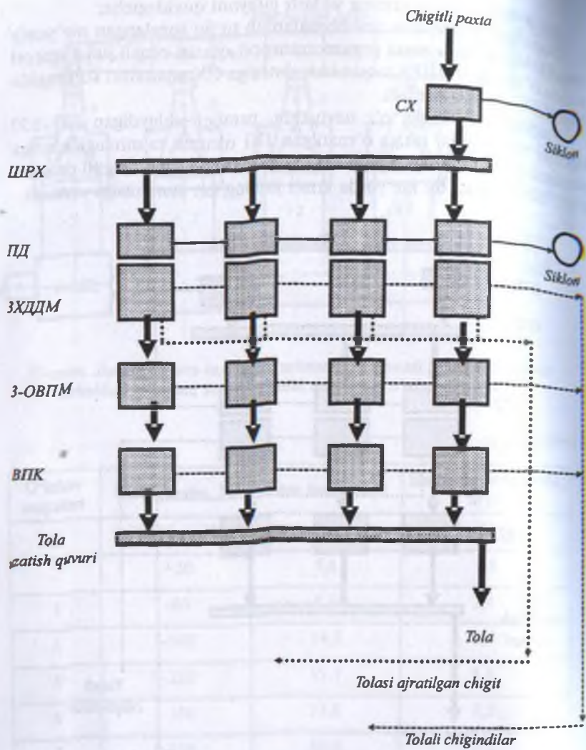
29-rasm. Arrali jinli sexda tola tozalashning kuchaytirilgan texnologik jarayon sxemasi.
