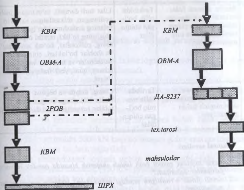
37-rasm. Tolali chiqindilarni qayta ishlash texnologik jarayon sxemasi.
