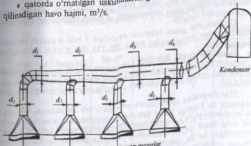
31-rasm. Tola uzatish quvurining moslamasi.
