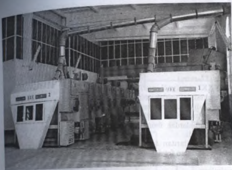
16-rasm. 6KXO.02 rusumli oqim yo'lli uskunalar majmuasining umumiy ko'rinishi.
