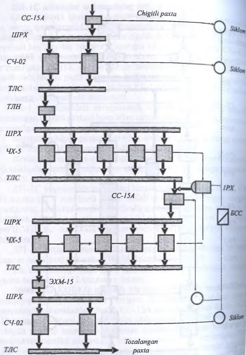
20-rasm. КОБКО uskunalarining texnologik jarayon sxemasi.
