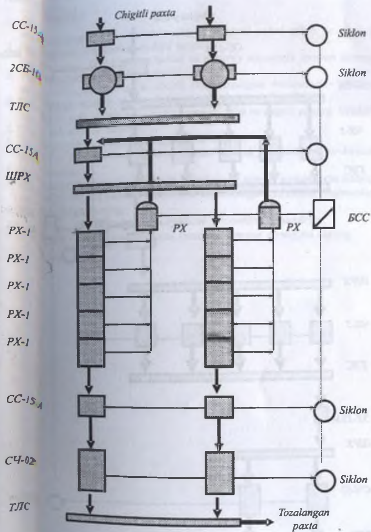
23-rasm. JIP-1CT uskunalar majmuasining texnologik jarayon sxemasi.
