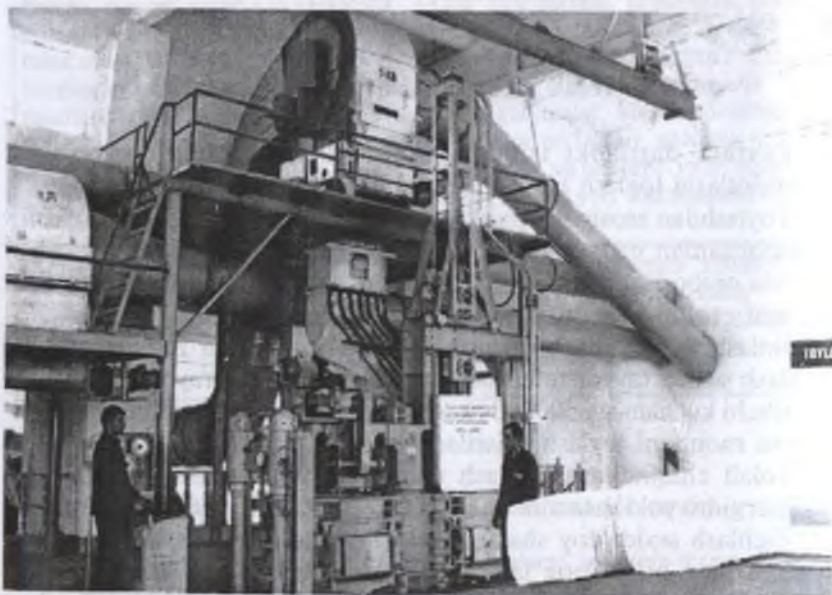
38-rasm. Paxta tolasini toylashda ishlatiladigan AK DB-8238.31 rusumli gidravlik press (zichlash) qurilmasi.
