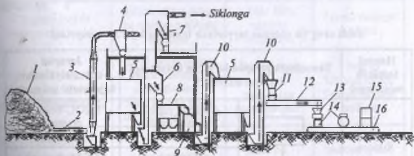
40-rasm. Urug'lik chigitni tayyorlash sexi uskunalarining texnologik jarayon sxemasi:
