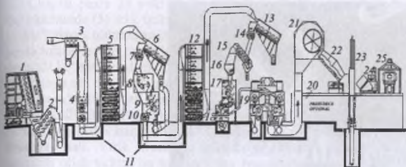
46-rasm. «Kontinental Igl» korporatsiyasining o'rta tolali chigitli paxtani qayta ishlab chiqarish texnologik jarayoni.
