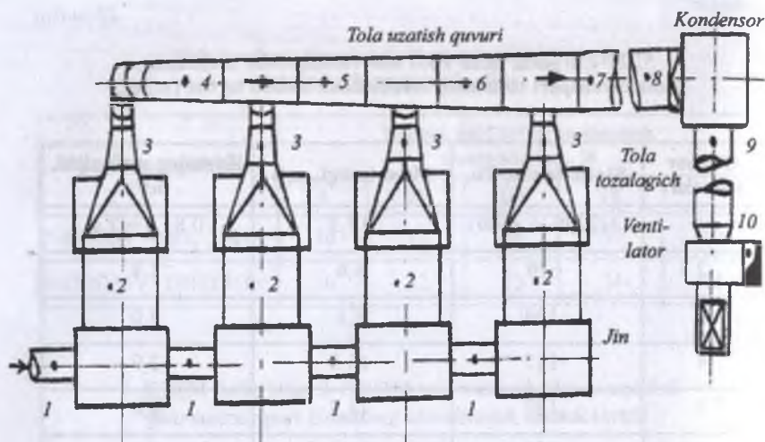
27-rasm. Jinlash va tola tozalagich uskunalar majmuasi pnevmotransport tizimidagi havoning statik bosimini aniqlashda o'lchov nuqtalari.
