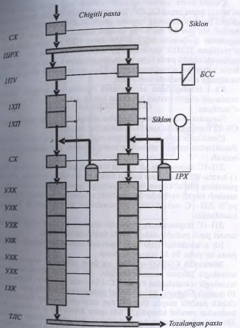
18-rasm. KOTT-uskunolari majmuasining texnologik jarayon sxemasi.
