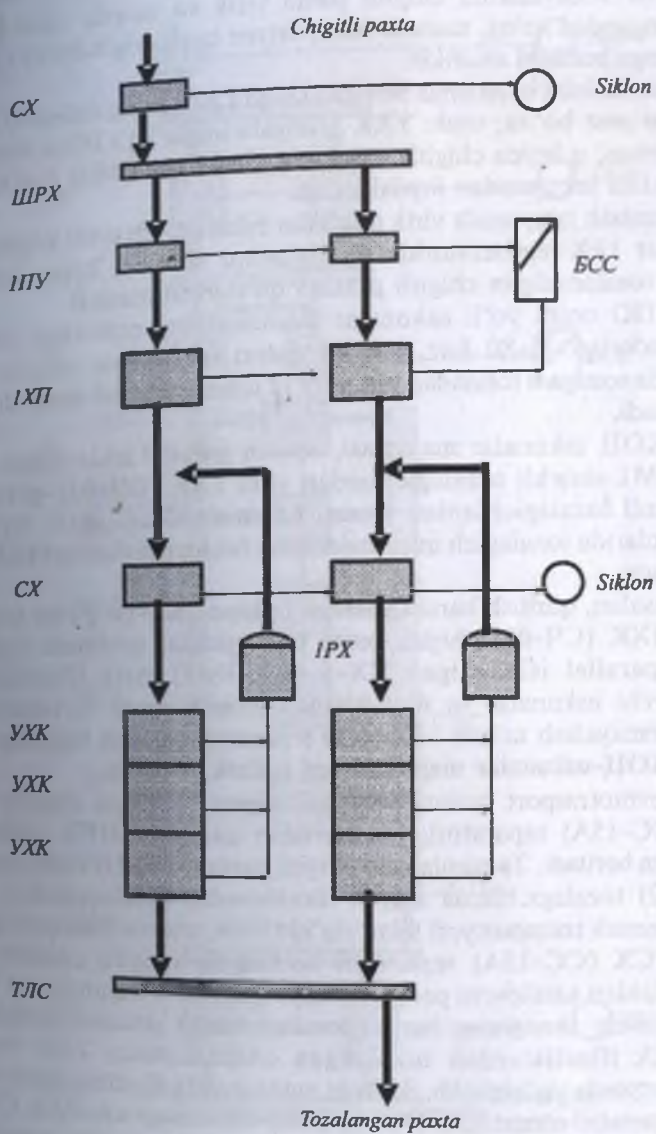
12-rasm. 2LPO-ushkunar majmuasining texnologik jarayon sxemasi.
