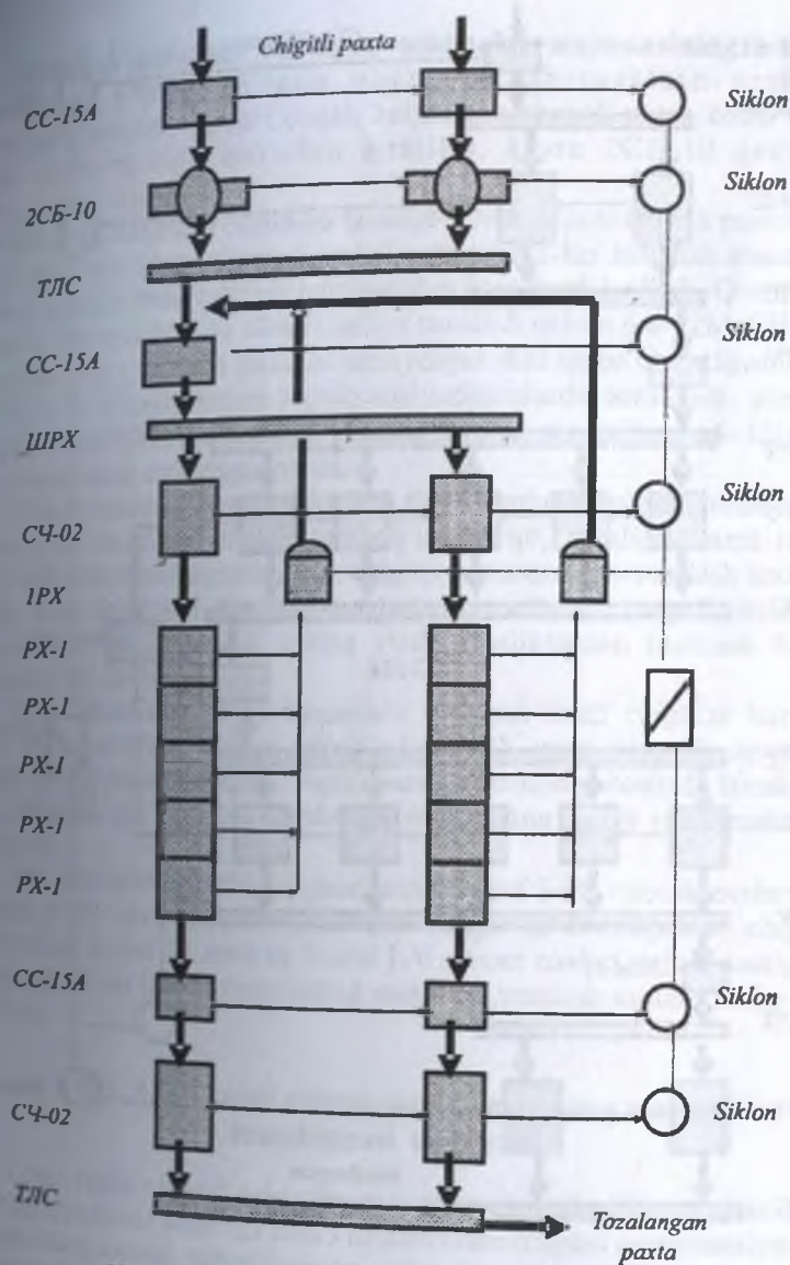
19-rasm. ЛП-1С-uskunalar majmuasining texnologik jarayon sxemasi.
