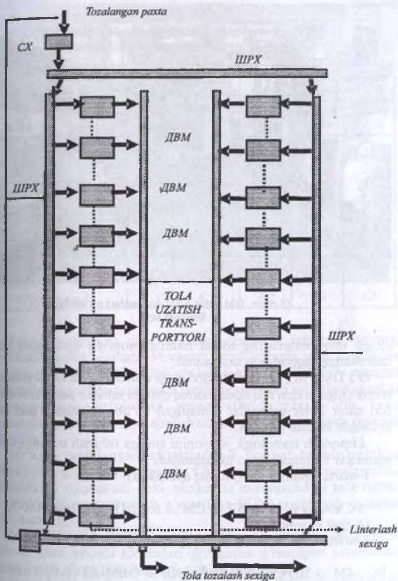
32-rasm. Ikki qator g'o'lali jinlar o'rnatilgan sexining texnologik jarayon sxemasi.
