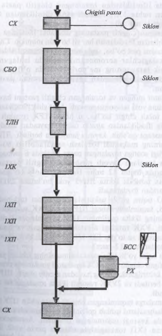
11-rasm. JP-3 uskunalar majmuasining texnologik jarayon sxemasi.
