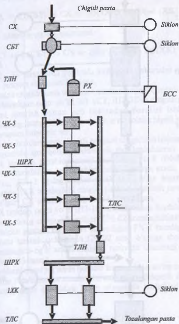
22-rasm. 2KOC-T uskunalar majmuasining texnologik jarayon sxemasi.
