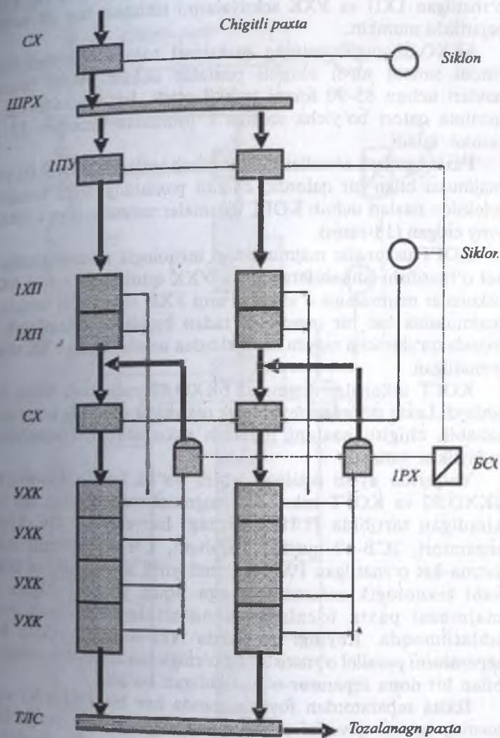
17-rasm. 6KXO.02- uskunalar majmuasining texnologik jarayon sxemasi.
