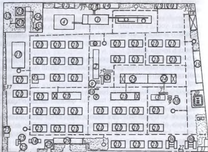
52-rasm. Paxta tozalash zavodi bosh planining gorizontol joylashishidagi ko'rinishi.
