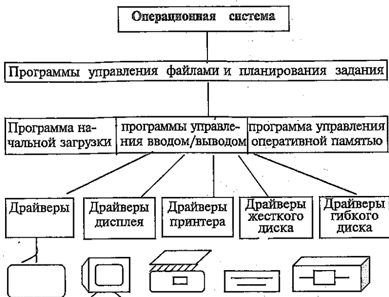
Рис. 4. Организация операционной системы.
