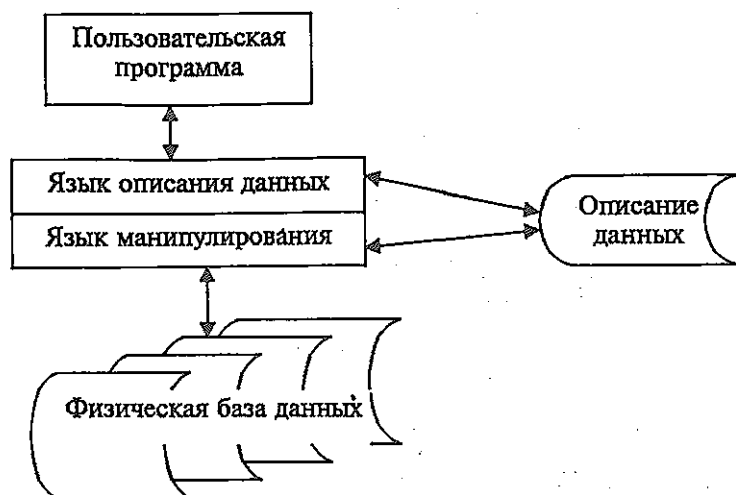
Рис. 3. Архитектура системы управления базами данных.
