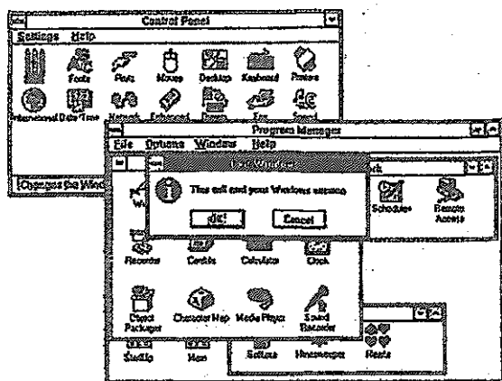
Windows 3.1.
