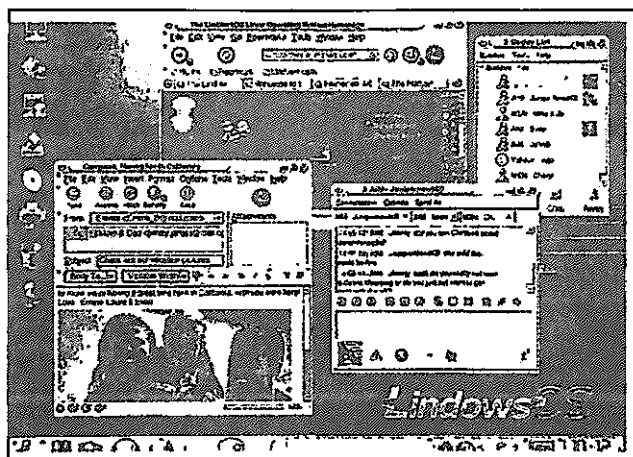
Lindows
