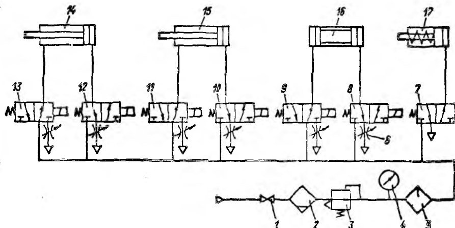
Рис. 4.7. Пневматическая схема промышленного робота МП-9С
