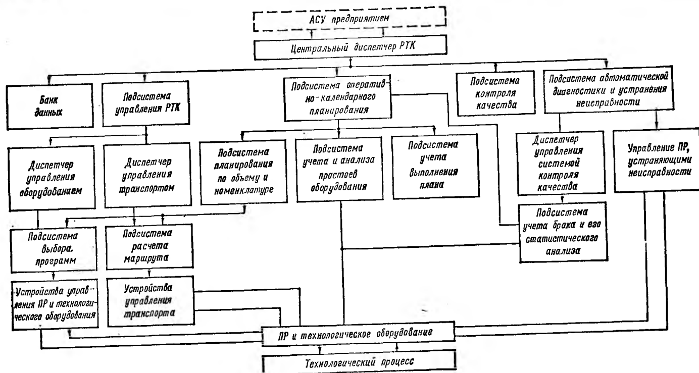
Рис. 8.11. Схема организации управления РТК
