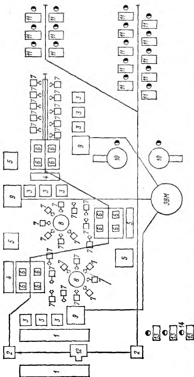
Рис. 9.3. Роботизированный участок намотки и сборки контурных катушек радиоприсоединений:
