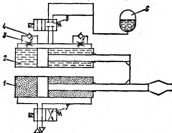
Рис. 4.24. Схема пневмогидравлического привода
