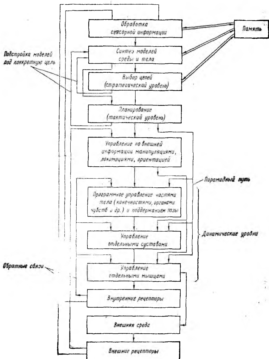
Рис. 2.3. Общая функциональная схема нерархической системы управления движениями человека
