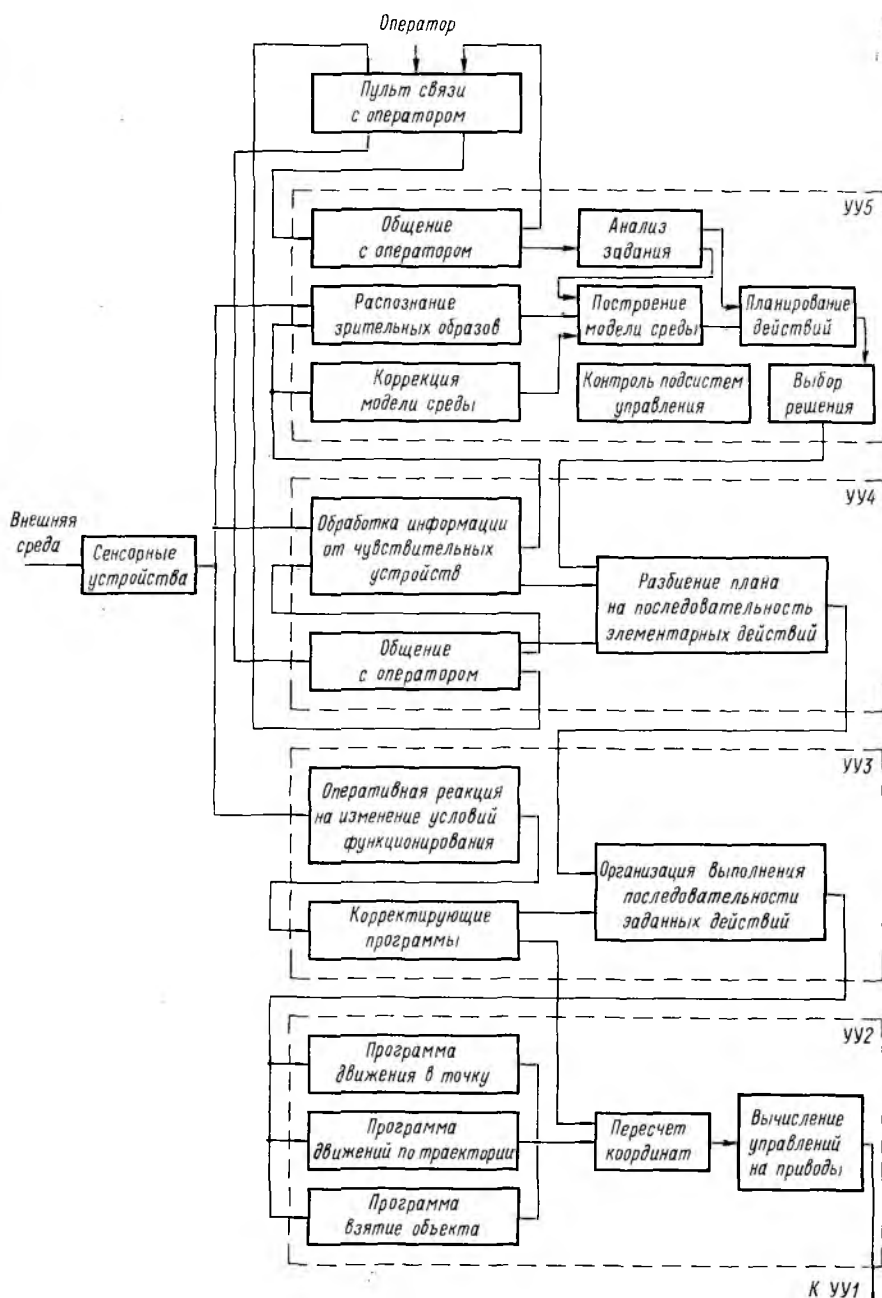
Рис. 5.8. Структура задач, решаемых на различных уровнях управления роботом
