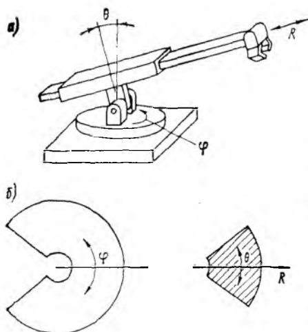
Рис. 3.3. Манипулятор со сферической системой координат (а) и его рабочая зона (б)
