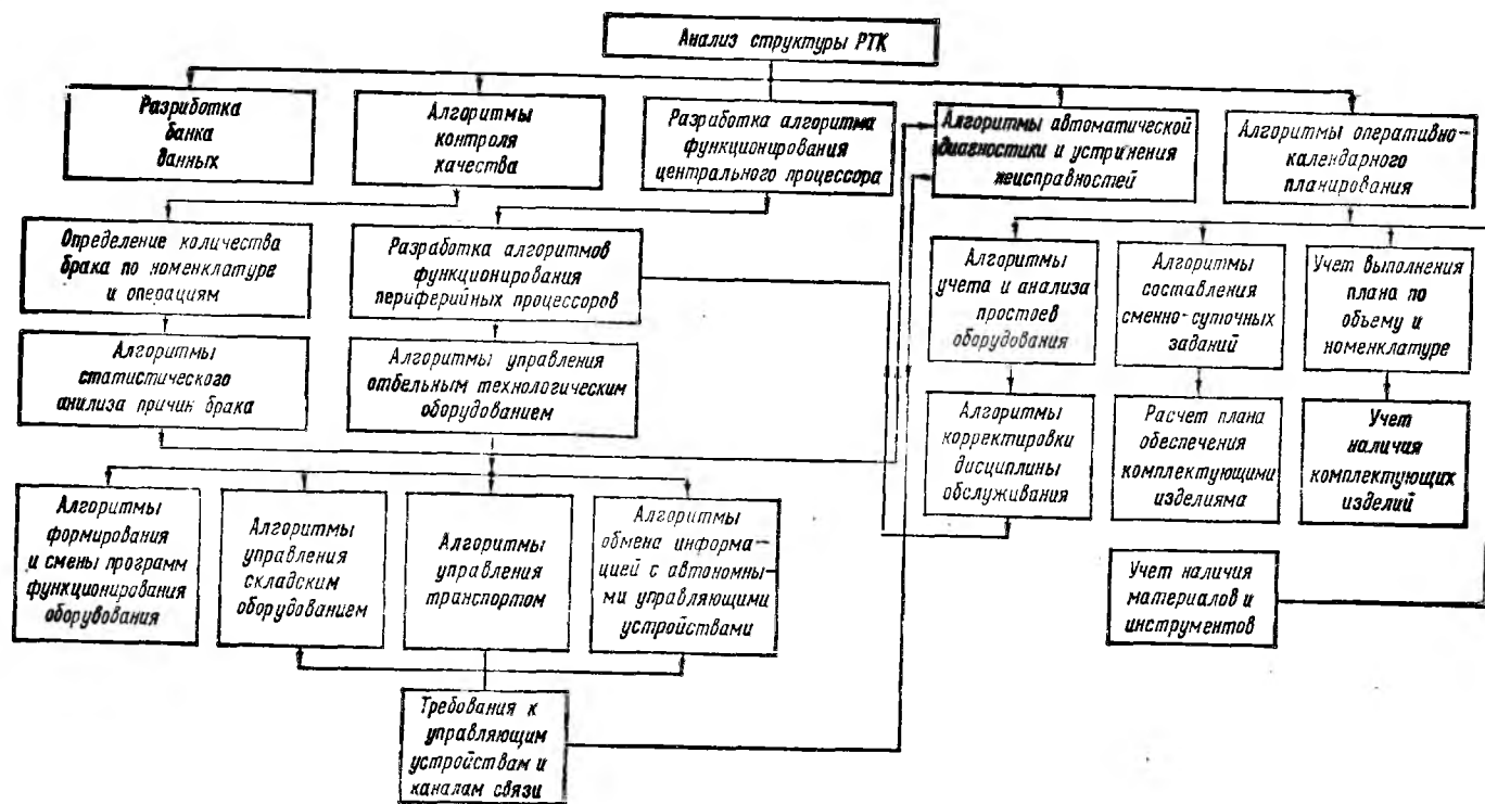
Рис. 8.10. Состав алгоритмического этапа проектирования РТК
