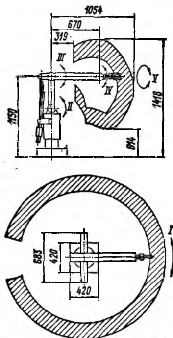
Рис. 4.22. Схема робота ИР6-6
