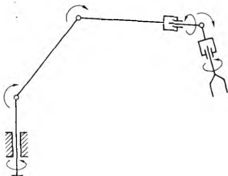
Рис. 6.1. Кинематическая цепь шестизвеного манипулятора
