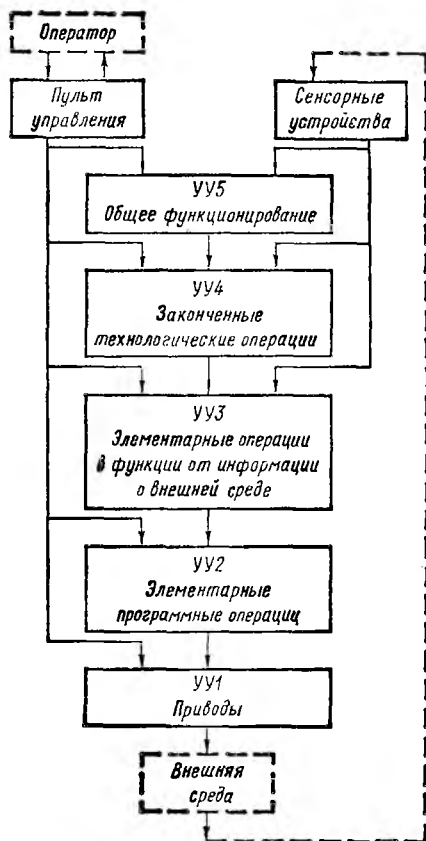
Рис. 5.8. Обобщенная структура системы управления оучувствленным роботом
