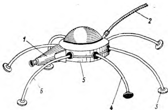
Рис. 11.18. Шестиногая шагающая транспортная машина с приклеиваемыми стопами ног:
