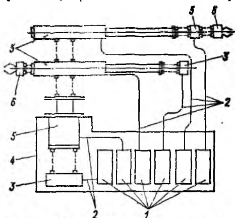
Рис. 7.5. Модульный пневматический промышленный робот МП-11 с двумя манипуляторами грузоподъемностью 0,5 кг:
