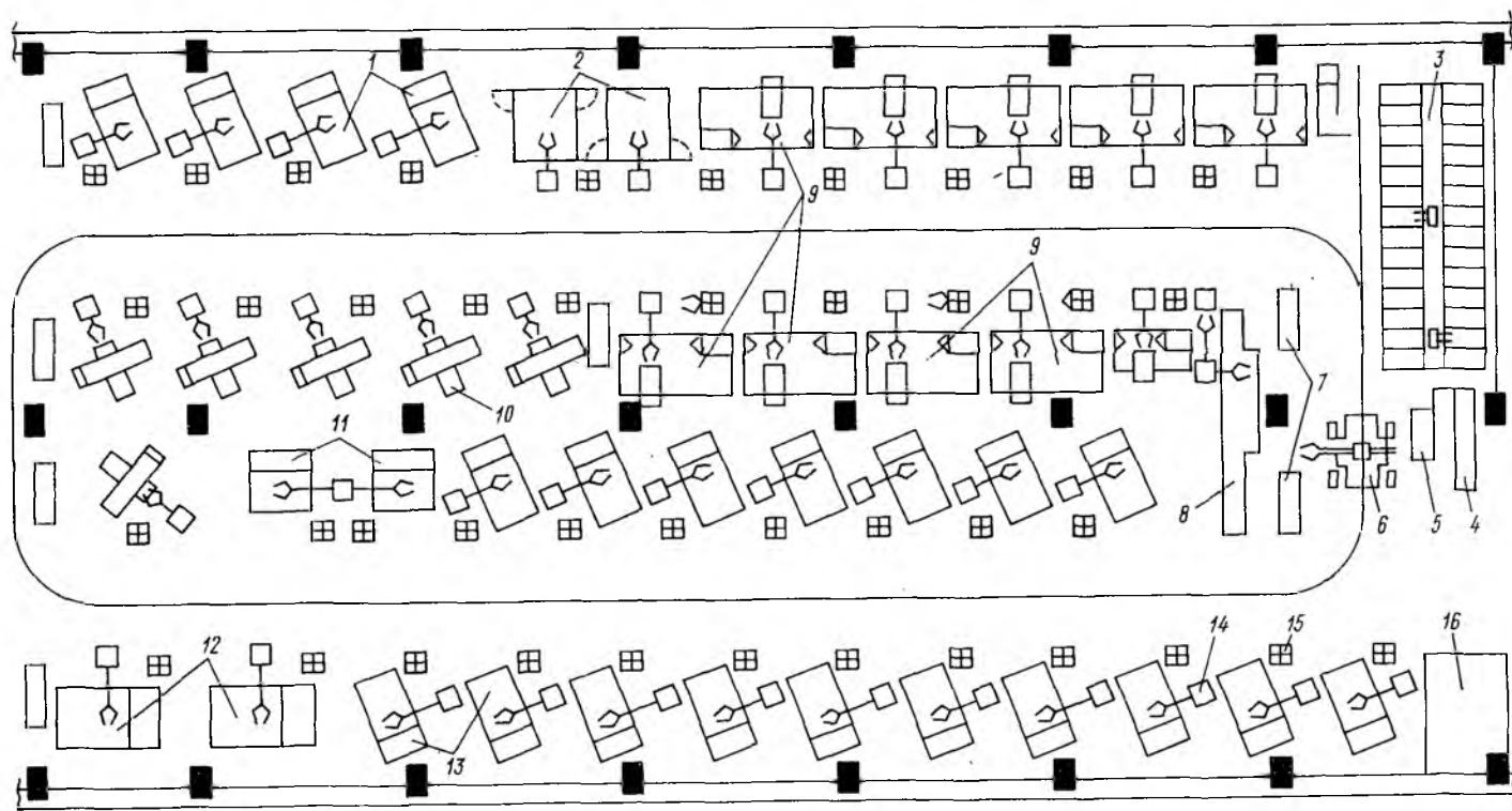
Рис. 10.3. Роботизированный цех механообработки:
