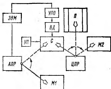
Рис. 10.5. Роботизированный комплекс холодной штамповки с адаптивным ПР на входе
