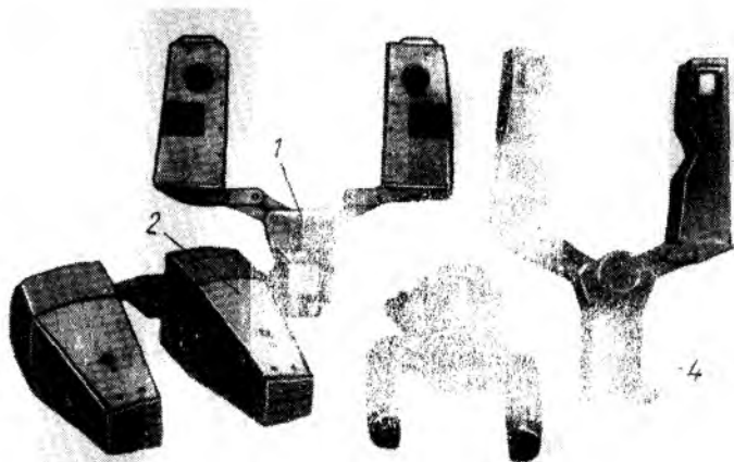
Рис. 3.21. Очувствленные схваты ЦНИИ РТК:
