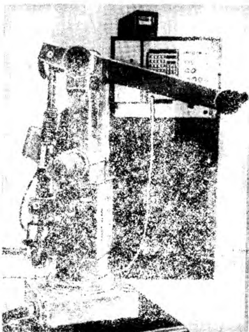
Рис. 4.21. Электромеханический промышленный робот с позиционно-контурным управлением фирмы АСЕА (Швеция)
