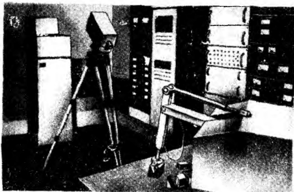
Рис. 1.10. Экспериментальный робот «Хивип» Центральной научно-исследовательской лаборатории фирмы «Хита-чи» (Япония) для механической сборки простых объектов по чертежу
