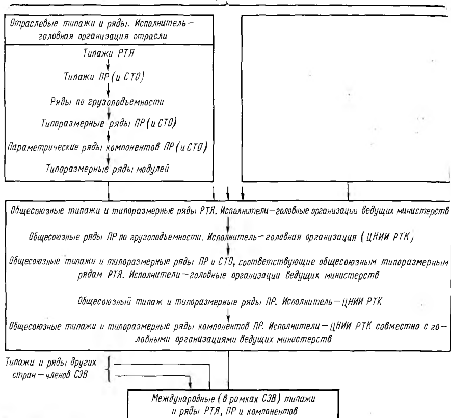
Рис. 7.10. Схема осуществления унификации в промышленной робототехнике: РТЯ — унифицированная технологическая ячейка; СТО — специальное технологическое оборудование.
