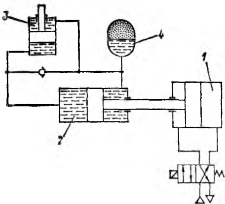
Рис. 4.25. Схема гидропневматического привода
