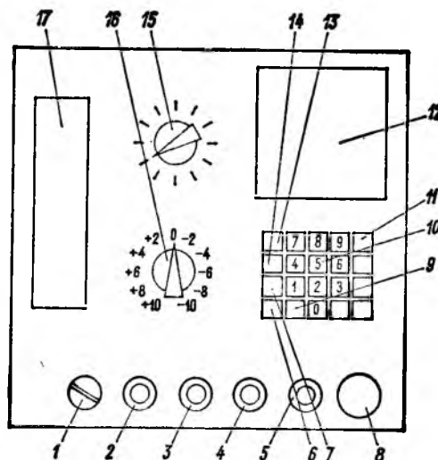
Рис. 4.15. Лицевая панель устройства управления робота «Коат-а-Матик»
