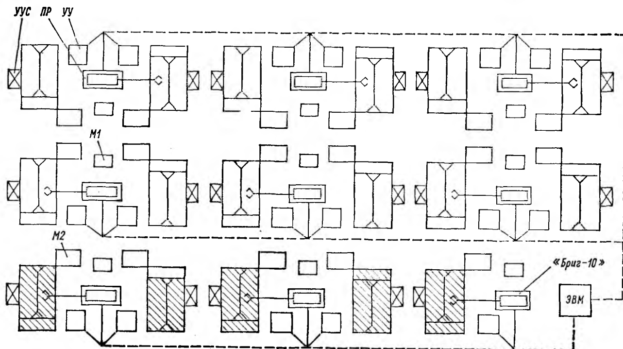
Рис. 10.2. Роботизированный участок механообработки шлицерно-торцевых соединений НПО «Буревестник» (Ленинград): М1 и М2 — магазин соответственно обрабатываемых и обработанных деталей; УУС — устройство удаления стружки; УУ — устройство управления
