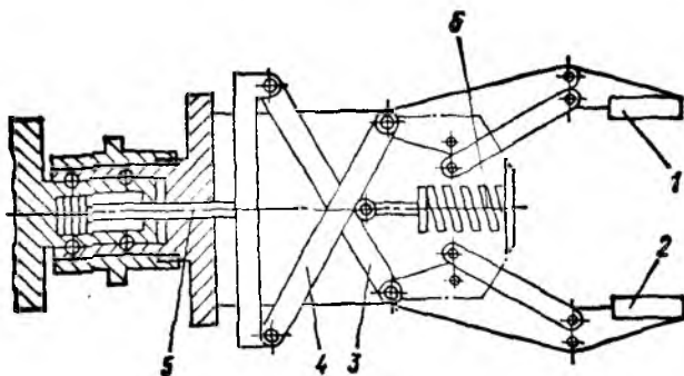
Рис. 3.9. Двухпальцевый схват:
