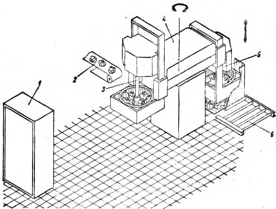
Рис. 11.5. Роботизированный комплекс для погрузки капусты
