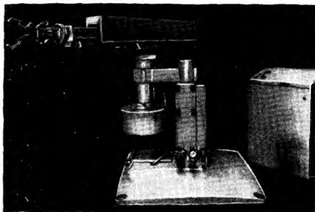
Рис. 4.9. Пневматический промышленный робот «МХУ Юниор» грузоподъемностью 5 кг фирмы «Электрорюкс» (Швеция)
