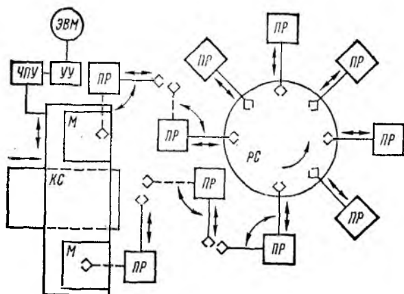
Рис. 8.8. Схема типового роботизированного сборочного участка с круговой компоновкой:
