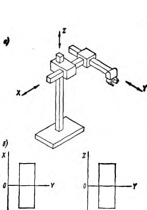
Рис. 3.1. Манипулятор с прямоугольной системой координат (а) и его рабочая зона (б)
