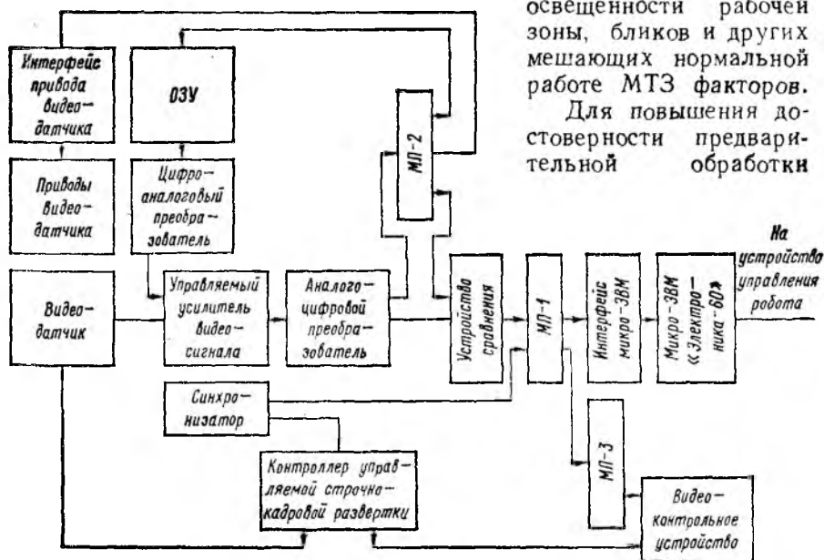
Рис. 3.20. Структурная схема МТЗ промышленного робота МП-8
