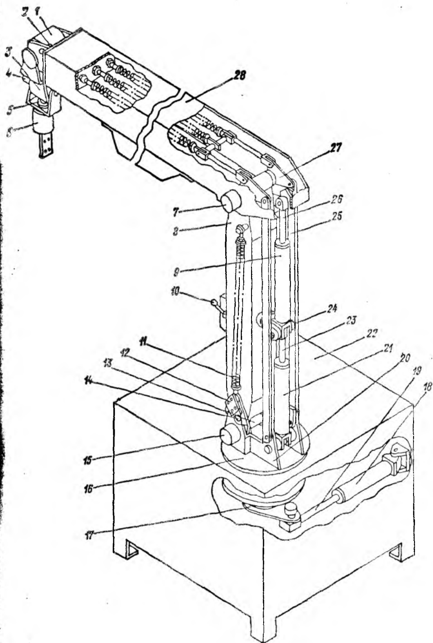
Рис. 4.13. Кинематическая схема робота «Коат-а-Матик»
