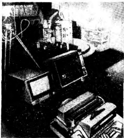
Рис. 1.11. Экспериментальный электромеханический робот ЭТЛ-1 электротехнической лаборатории ЭТЛ (Япония)
