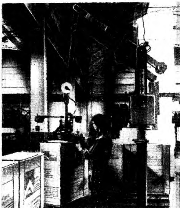
Рис. 3.6. Пневматический сбалансированный манипулятор
