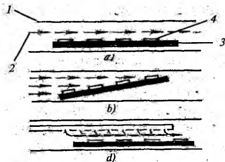
III.20-rasm. Gorizontalar reaktorlar turlari:
