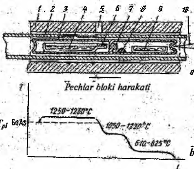
II.18—rasm. Galliy arsenidi mono-kristalini sintezlash va brijmen usulida o'stirish chizmasi: a —kovsharlangan ampulada; b —pechlar bloki uzunligi bo'yicha temperatura taqsimoti:
