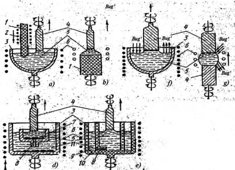
II.51-rasm. Uzunligi bo'yicha birday legirlangan kristallarni o'stirishda kristallanuvchi suylamani qattiq (a, b), suyuq (d, e) va bug' (gaz) (f, g) fazalardan oziqlantirishdan foydalanadigan asosiy usullar:
