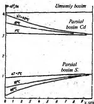
II.47-rasm. Nostexiometrik \text{CdS} tarkiblovchilarning parsial bosimlari hisoblangan qiymatlarining (turli \Delta T lar uchun) manbagacha masofaga bog'liqligi.
