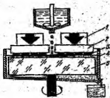
III.9-rasm. Tekislashda yarimo'kazgich plastinkalar joylashishi:
