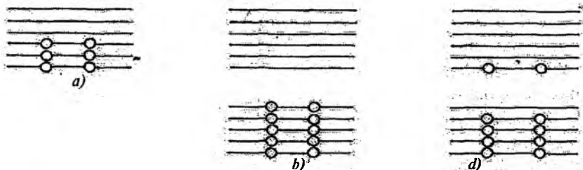
1.6— rasm. Energiya zonalarining elektronlar bilan to'ldiriliqlari hollari.
