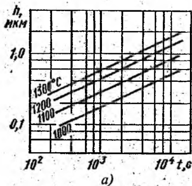
5- rasm . Turli temperaturalarda kremniyni niqoblash uchun kerakli bo'lgan \text{SiO}_2 oksidi qalinligining diffuziya vaqtiga bog'liqligi: a) fosfor diffuziyasida; b) bor diffuziyasida.
