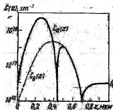
III.35-rasm. Ion legirlash usulida olingan n - p - n tuzilmali tranzistorda bor va fosfor taqsimoti.
