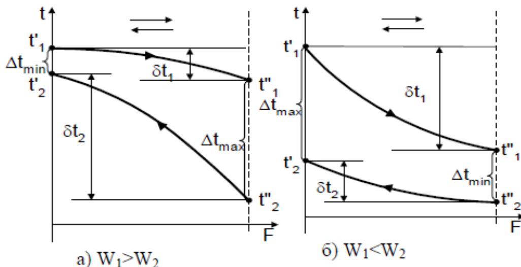
2.2 b-rasm. Issiqlik tashuvchilarning oqimga qarshi harakatlanish sxemasida ularning suv ekvivalentlari nisbatiga bog'liq ravishda qaynoq va sovuq issiqlik tashuvchilar haroratining issiqlik almashinish yuzasi bo'ylab o'zgarishi
