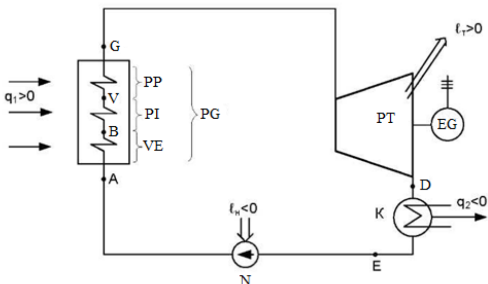
1.12-rasm. Bug' - kuch uskunasiining prinsipial sxemasi:
