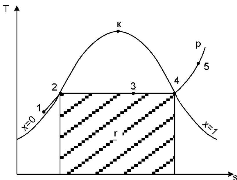
2.1-rasm. Suv bug'ining fazaviy T, s - diagrammasi
