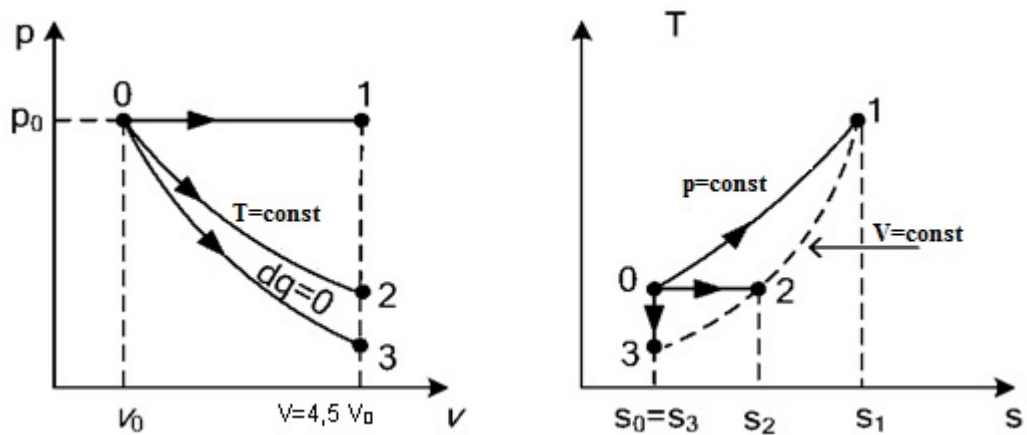
1.5-rasm. Gazning kengayish jarayoni:
