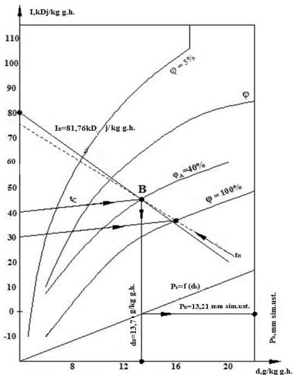
1.11-rasm. Nam havo parametrlarini I, d - diagramma bo'yicha aniqlash
