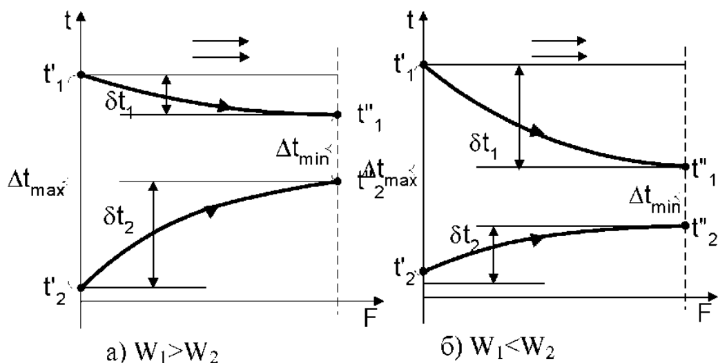
2.2 a-rasm. Issiqlik tashuvchilarning oqim bo'ylab harakatlanish sxemasida ularning suv ekvivalentlari nisbatiga bog'liq ravishda qaynoq va sovuq issiqlik tashuvchilar haroratining issiqlik almashinish yuzasi bo'ylab o'zgarishi
