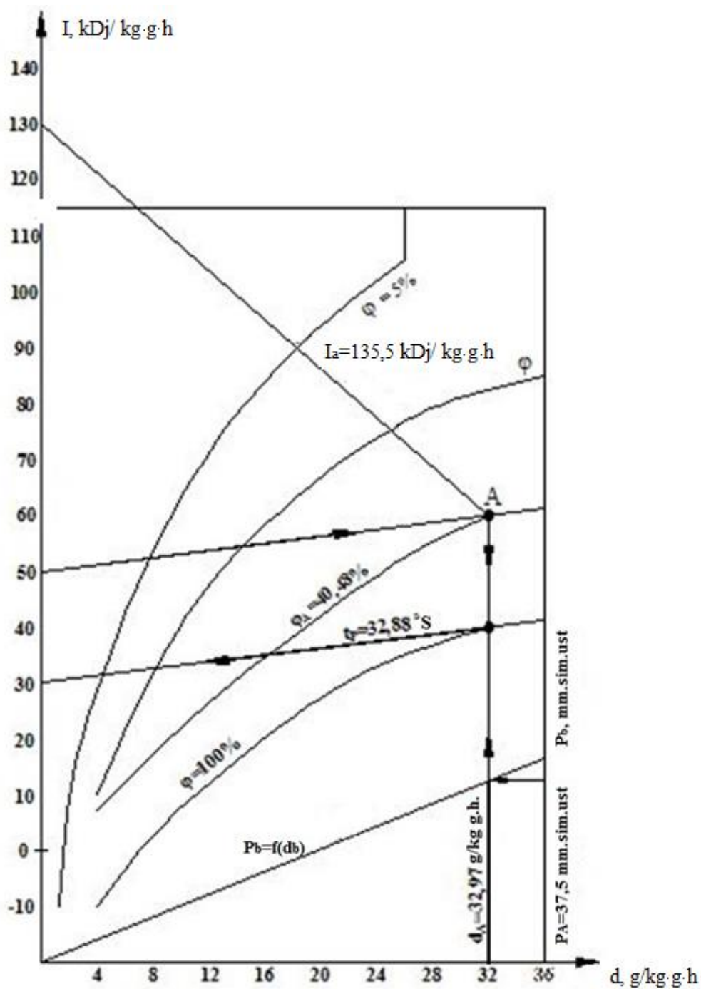
1.10-rasm. Nam havo parametrlarini I,d - diagramma bo'yicha aniqlash
