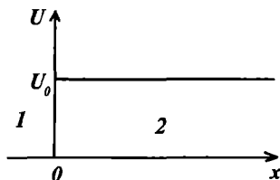
7-rasm. To'g'ri burchakli cheksiz uzunlikdagi bir o'lchamli potentsial to'siq.
