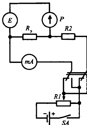
2.10-rasm. EYuK ni o'lchashning kompensatsion sxemasi.
