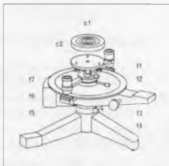
5 - rasm. Spektrometrning asosiy qurilmasi va prizma stoli
