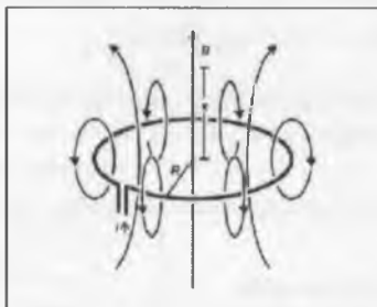
3-rasm. Aylanma halqa shaklidagi o'tkazgichning magnit maydoni.
