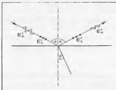
1 - rasm. Qutblanish yo'nalishlarini va amplitudalar belgilanishlarini tushuntirish.
