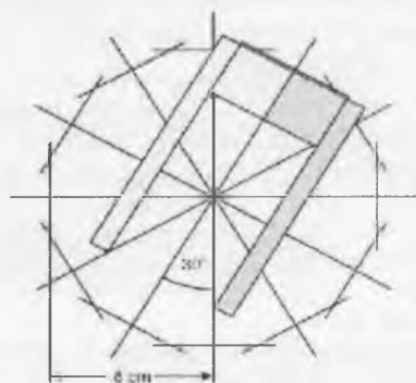
2 – rasm. Taqasimon magnitni kerkli holda joylashtirish uchun moslamadan foydalanish
