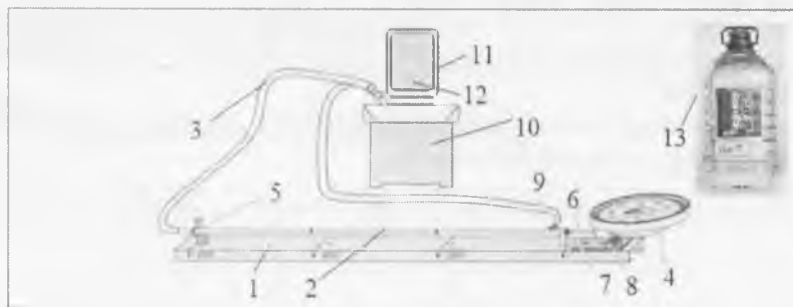
1-rasm. Quvurlarning chiziqli kengayishini temperatura funksiyasi sifatida o'lchash bo'yicha tajriba qurilmasining ko'rinishi.
