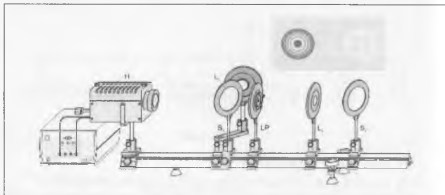
3- rasm. Nyuton xalqalarini kuzatish uchun tajriba qurilmasi.
