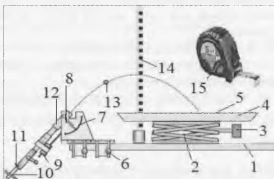
2-rasm. Uchish uzoqligi va balandligining otilish burchagiga bog'liqligini aniqlovchi tajriba qurilmasi tuzilish chizmasi
