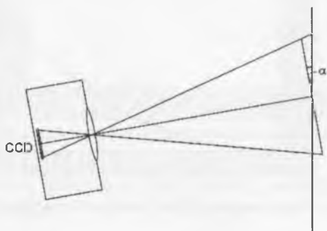
2-rasm. VideoCom va erkin tushish trayektoriyasi orasidagi \alpha burchakni aniqlash chizmasi.
