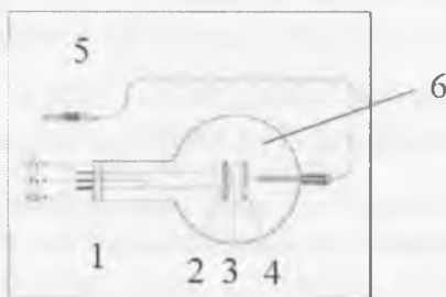
1-rasm. 1 - qizdiruvehi vilka, 2 - katod plastinkasi, 3 - katod qizdirgich simi, 4 - Anod, 5 - anodni ulash simi, 6 - havosi so'rib olingan shisha bolon.
