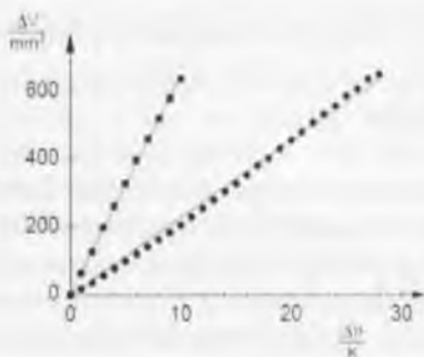
3-rasm. Suv hajmining \Delta V (doiralalar) va etanol hajmining (to'rtburchaklar) temperaturalar farqi \Delta t funksiyasi sifatida issiqlikdan kengayishi
