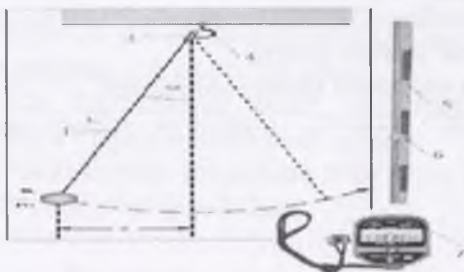
1-rasm. L uzunlkdagi \varphi burchakka og'dirilgan matematik mayatnik tebranish davrini aniqlash qurilmasi.
