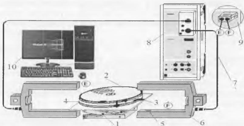
1- rasm. Burchak momenti va energiyaning saqlanishi (aylanma to'qnashuv) namoyish qilish
