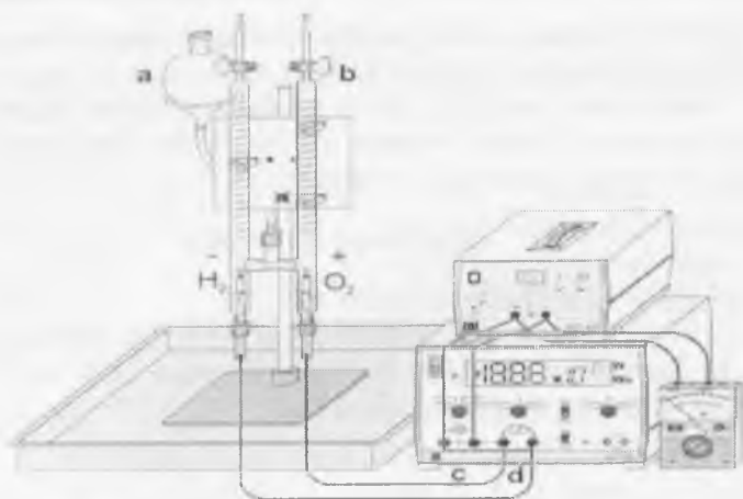
1-rasm. Faradey doimiysini suvni elektroliz qilish qismi yordamida aniqlash qurilmasi.
