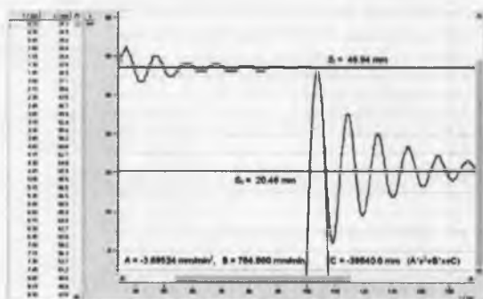
10-rasm. Qo'rg'oshin sarchalar // holatdan / holatga aylanib qaytganida tebranishlarning birinchi fazasi uchun tezlanishni aniqlash (kattaroq tasvirini 7-rasmga ko'ring).
