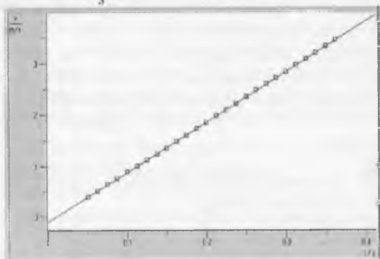
4-rasm. Erkin tushuvchi jism uchun tezlik-vaqt diagrammasi.
