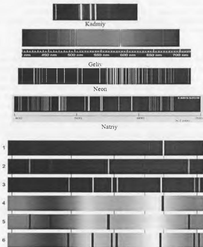
Спектры испускания: 1 - натрия; 2 - водорода; 3 - гелия. Спектры поглощения: 4 - натрия; 5 - водорода; 6 - гелия.
