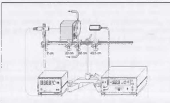
1 - rasm. Stefan-Bolsmannning issiqlikdan nurlanish qonunini tasdiqlash uchun tajriba qurilmasi
