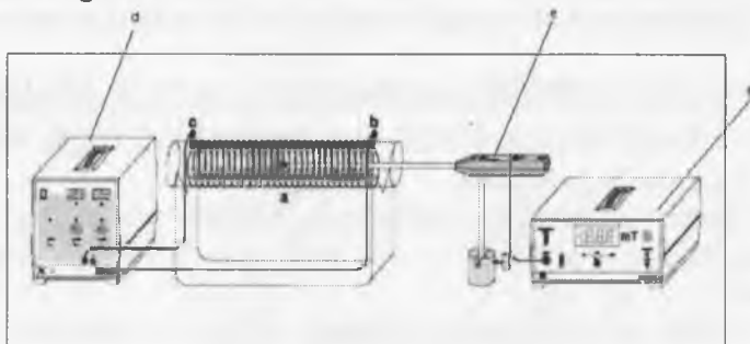
2 - rasm: o'zaksiz g'altakning induktivligini aniqlash
