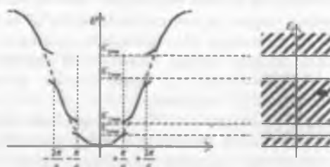
27.2-rasm. Kristallda erkin elektronlar energiyasi E ni to'liq son k ga bog'liqlik grafiqi.
