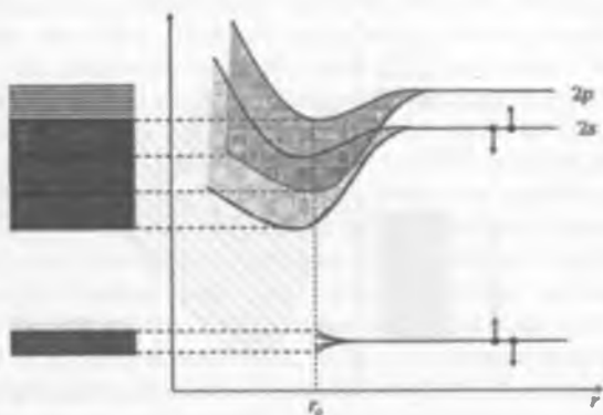
27.8-rasm. Beriliiy kristalida 2s- va 2p-zo'nalarining o'zaro qoplanishi.
