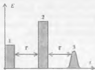
32.6-rasm. Foton sadosi
