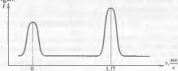
23.12-rasm. Yutkichdan (yutuvchi modda) o'tgan gamma kvantlarni osillogrammasi.
