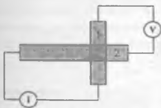
29.22-rasm. Tunnel eksperimentining chizmasi.
