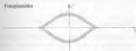
18.7-rasm. Shtern-Gerlax tajribasida kumush atomlarini fotoplastinkada joylanishi.
