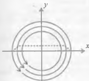
18.11-rasmi. Doiraviy elektromag-nit to'liqin paketida vaqt bo'yicha energiya oqimining o'rtacha sirkulatsiyasi.
