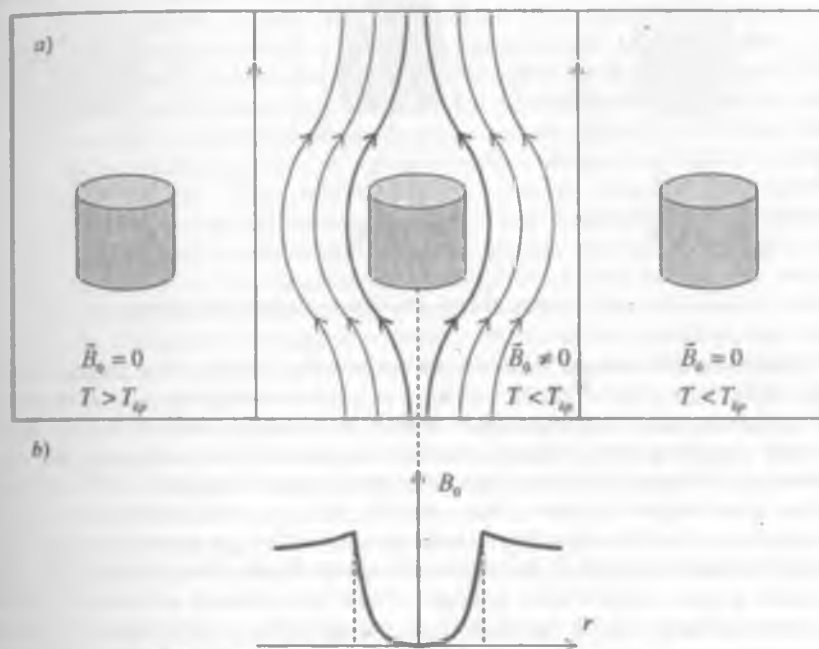
29.4- rasm a) Magnit maydonda o'ta o'tkazuvchan tsilindr
