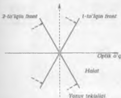
22.16-rasm. Optik o'qqa nisbatan simmetrik joylashgan ikkita yassi to'lqinlarni qo'shish.
