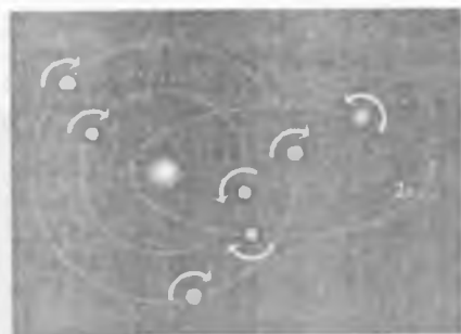
Azot atomining elektron konfiguratsiyasi
