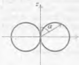
20.5-рисунок. Energiyaning burchak taqsimoti.
