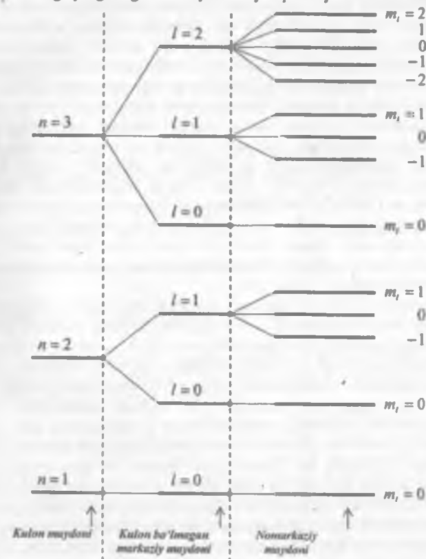
19.1-rasm. Vodorod atomining energetik sathlarni aynishi va yo'qotishi yo'llari.
