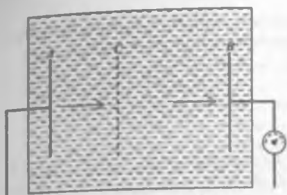
28.6-rasm. Suyuq geliy ichidan o'tayotgan geliy ionlari harakatini o'rganadigan asbob chizmasi.
