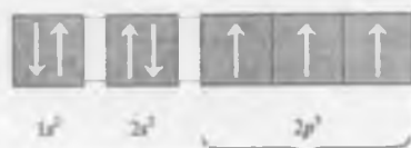
Xund qoidasiga binoan uchchala elektronning spini yuqoriga qarang
