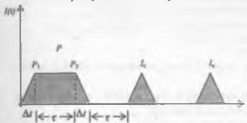
32.12-rasm Chekkaviy va ko'p karrali sado. R — uyg'otuvchi impuls, \Delta t va \tau chekkani davomligi va davomlilik, I_k — chekkaviy sado, I_k — ko'p karrali sado.
