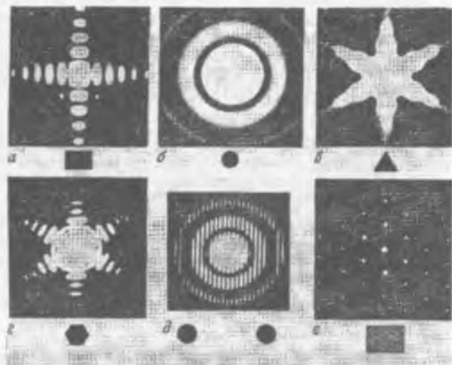
22.20-rasm. Ba'zi tirqishlarda Fraunhofer difraksiyasi.
