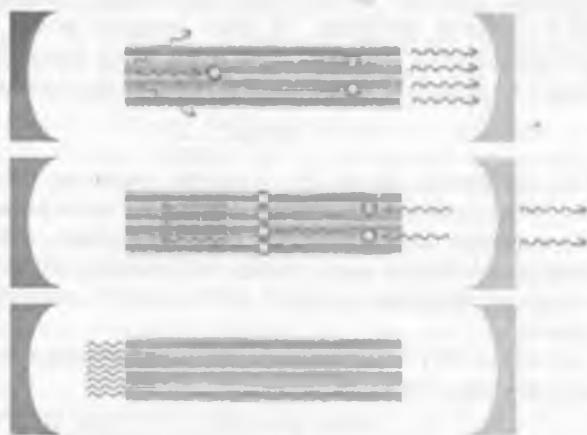
22.7-rasm. Optikaviy kvant generatorida foton lavinasini (uyumi) hosil bo'lishi.
