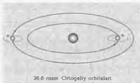
26.6-rasm. Ortogeliy orbitalari.
