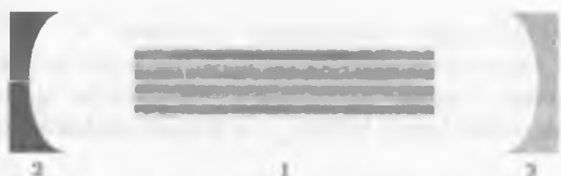
22.6-rasm Optikaviy kvant generatorning prinsipial chizmasi 1-aktiv muhit; 2-yaxlit ko'zgu; 3-yarim tiniq ko'zgu.
