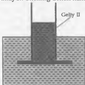
28.1-rasm. He-II ni o'ta oquvchanligi Ikki ta silliqlangan shisha plastinka orasidagi tor kanaldan Geliy-II bemolol oqib o'tadi. Suv esa bu kanaldan o'ta olmaydi.
