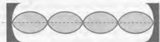
22.7-rasm. Rezonator turg'un to'lqin.
