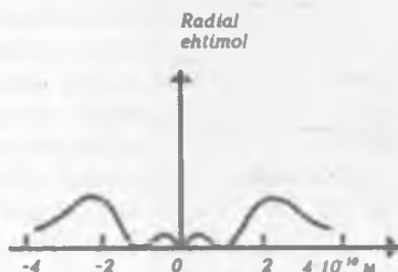
2s uyg'ongan holatda elektronning radial ehtimol zichligi
