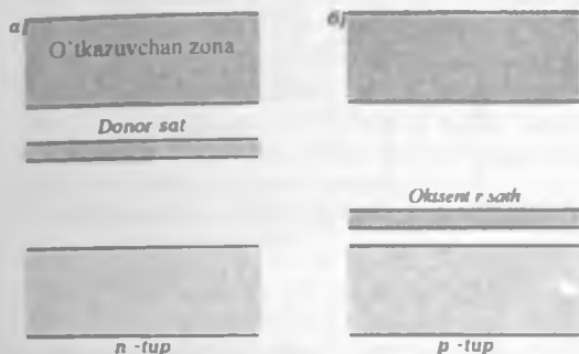
27.16-rasm. Aralashmagi yarimo'tkazgichlarda donor va akseptop energetik sathlar.
