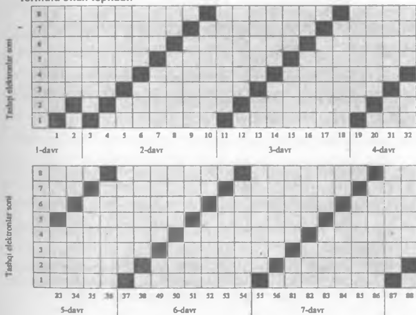
26.3-rasm. Elementar atomlari tuzilishining davriy o'zgarishi.
