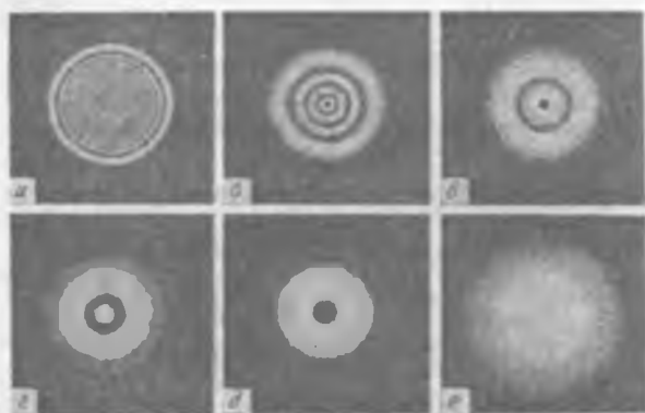
22.19-rasm. Doiraviy tirqishda Frenel difraksiyasi. z kattalik o'zgarmas, z esa a dan e gacha o'lib boradi.
