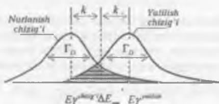
23.6-rasm. Chiziqlarning dopler kengayishu hisobiga yadroviy gamma rezonansining ro'y berishi.
