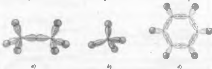
24.6-rasm. Molekula strukturasi
