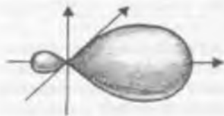
24.4-rasm sp^3 -gibrid orbitali.
