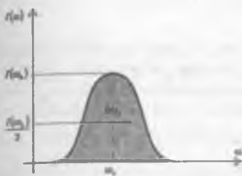
21.5-rasm. Spektral chiziqlarning Dopler kengligi.
