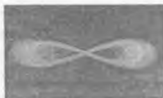
2p z uyg'ongan holatda elektronning bo'lishi ehtimoli katta bo'lgan soha
