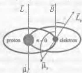
18.2-rasm. Vodorod atomida elektron va proton harakati.
