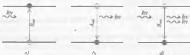
20.7-рasm. Atomda pastdan yuqoriga ( n \rightarrow m ) va yuqoridan pastga ( m \rightarrow n ) o'tishlar. a) yutilish; b) spontan nurlanish; d) induksirlangan (majburlangan) nurlanish.
