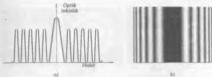
22.18-rasm. Yassi va silindrik to'liqlarni interferensiyasi tufayli intensivlikning taqsimlanishi.
