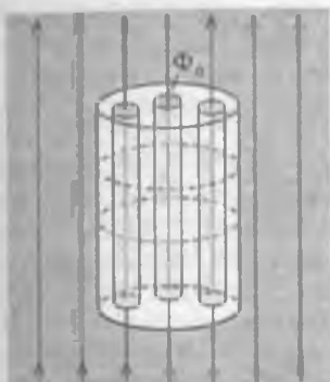
29.12-rasm. O'ta o'tkazuvchan metal perdasida kvant uyurmalarining paydo bo'lishi.
