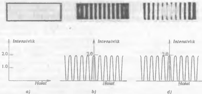
22.17-rasm. Ikkita to'ldinni qo'shilishi natijasida hosil bo'lgan normalangan intensivlik: a) nogogerent; b) kogerent; d) qisman kogerent.
