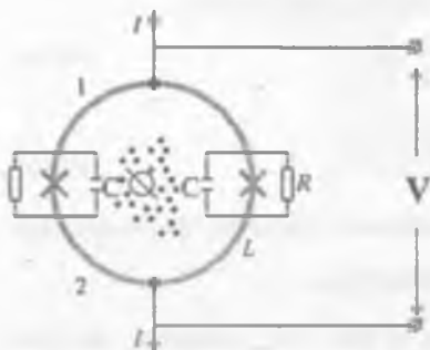
29.26-rasm. Magnit oqimi \Phi va o'rtacha tok I bo'lgan o'zgarimas tok SKVID sxemasi.
