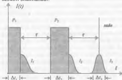
32.8-rasm. Vaqt bo'yicha foton sadosi. I(t) – javoblar (sado)lar) intensivligi: I_1 , I_2 va I_3 mos ravishda, 1– 2–, 3– induksiya va sado intensivliklari: t –vaqt, R_1 va R_2 uyg'otuvchi impuls: \Delta t_1 va \Delta t_2 , ularning davomiyligi.
