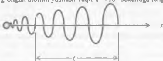
20.2-rasm. Yorug'lik impuls yoki to'lqinlar sistemasini sug.
