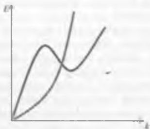
28.4-rasm. Real zarra va kvazizarralar uchun energiya va impuls bog'liqligi grafigi.
