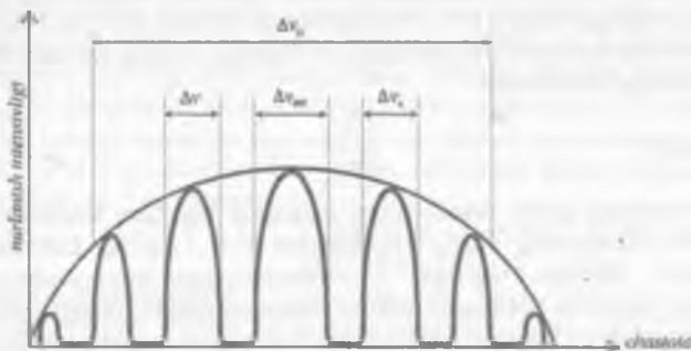
22.8-rasm. Optikaviy kvant generatorida nurlanish chizig'ini xarakterlovchi kattaliklar: \Delta\nu – chiziqning tabiiy kengligi;
