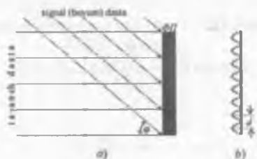
22.11-rasm. Qo'shni interferensiyon tasmlar orasidagi masofa.
