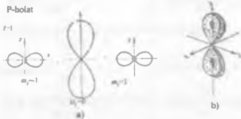
17.8-rasm. a) \theta - burchakka bog'liq bo'lgan p_\theta = |\psi|^2 va p_r = |\psi|^2 r holat uchun ehtimol zichligi; b) To'la ehtimol zichlik, burchak ehtimol zichligi p_\theta bilan radial ehtimol zichligi p_r ga ko'paytmasi.
