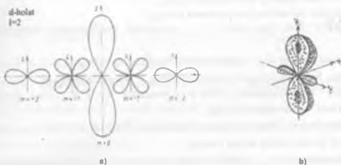
17.9-rasm. a) \theta - burchakka bog'liq bo'lgan \rho_\theta = |\psi_{2,1,1}, \psi_{2,1,1}| va \rho_\theta = |\psi_{2,1,2}, \psi_{2,1,2}| holat uchun ehtimol zichligi; b) To'la ehtimol zichlik, burchak ehtimol zichligi \rho_\theta bilan radial ehtimol zichligi \rho_r ga ko'paytmasi.
