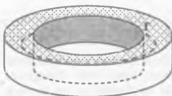
29.10-rasm. O'ta o'tkazuvchan halqa. G-ekontur.
