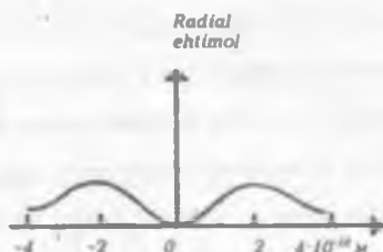
2p z uyg'ongan holatda elektronning radial ehtimol zichligi
