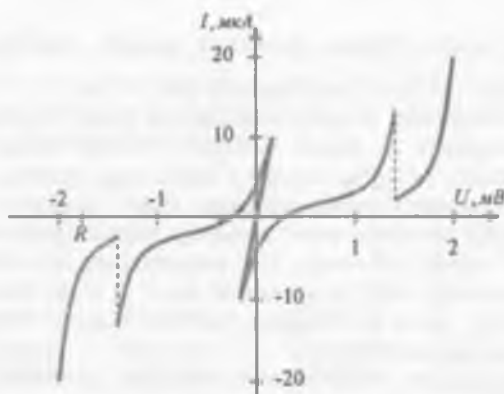
29.18-rasm Djozefson tunnel kontaktining volt-ampér xarakteristikasi.
