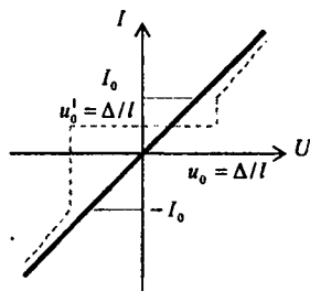
29.15-rasm. Tunnel kontaktning volt-ampere xarakteristikasi.
