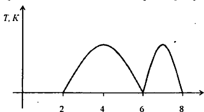
29.2-rasm. O'ta o'tkazuvchanlik holatiga o'tish temperaturasi valentli elektronlar soniga bog'liqligi grafiqi.
