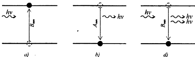
20.7- pacm. Atomda pastdan yuqoriga ( n \rightarrow m ) va yuqoridan pastga ( m \rightarrow n ) o'tishlar. a) yutilish; b) spontan nurlanish; d) induksirlangan (majburlangan) nurlanish.
