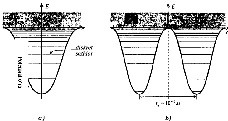
27.1-rasm. Potensial o'ra.
