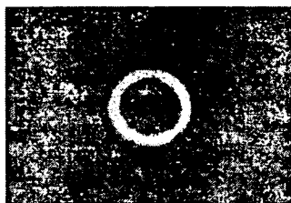
1s asosiy holatda elektronning bo'lishi ehtimoli katta bo'lgan
