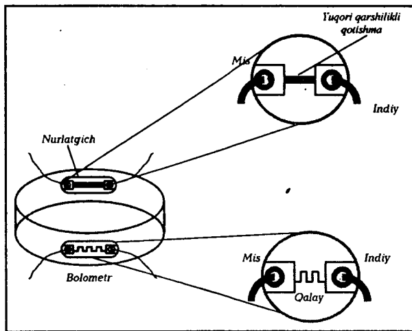
31.2-rasm. Fononoatom effekti tajriba.
