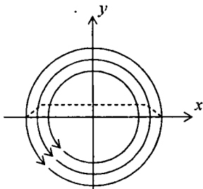
18.11-rasm. Doiraviy elektromag-nit to'liqin paketida vaqt bo'yicha energiya oqimining sirkulatsiyasi.
