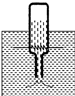
28.3-rasm. Geliy II ning fontan effekti.
