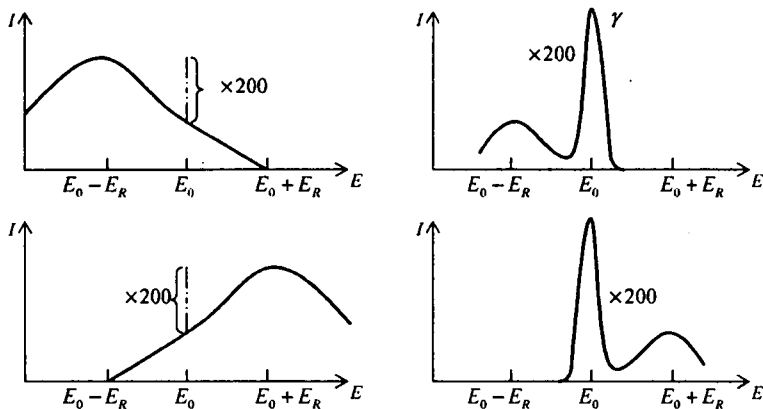
23.7-rasm. 88 K temperaturada ^{191}_{77}\text{Ir} -iridiy izotopi uchun gamma kvantlarni chiqarilishi va yutilishi.
