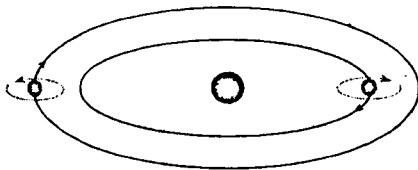
26.6-rasm. Ortogeliy orbitalari.
