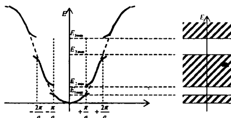
27.2-rasm. Kristallda erkin elektronlar energiyasi E ni to'liq son k ga bog'liqlik grafigi.
