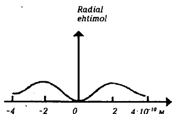
2p_x uyg'ongan holatda elektronning radial ehtimol zichligi
