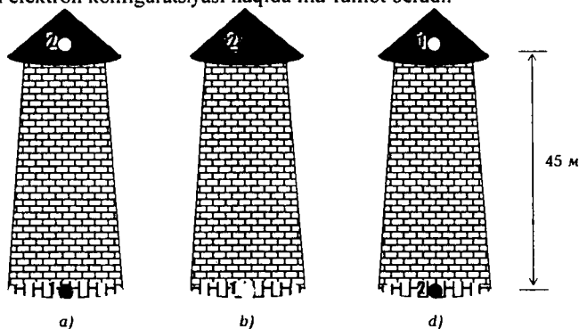
23.16-rasm. Gravitatsion maydonda gamma kvantni qizil siljishi. R.V.Paund va G.A.Rebke tajribasi.
