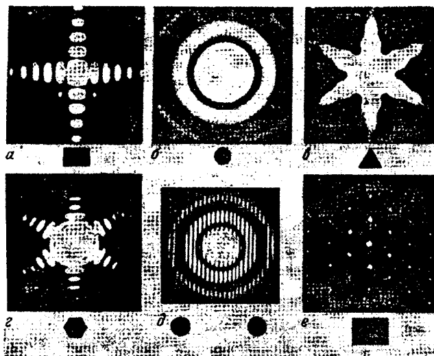
22.20-rasm. Ba'zi tirqishlarda Fraungofer difraktsiyasi.
