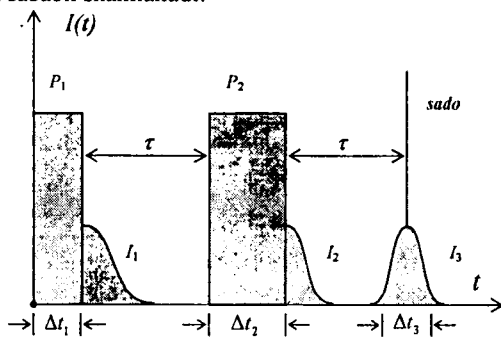
32.8-rasm. Vaqt bo'yicha foton sadosi.
