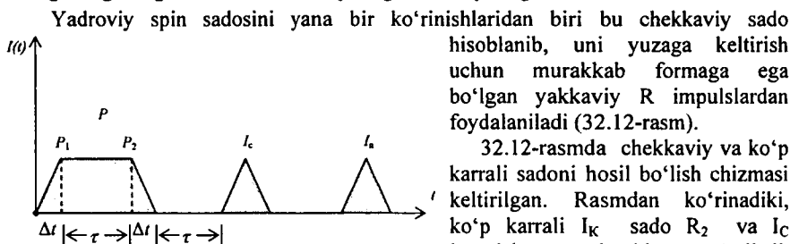
32.12-rasm. Chekkaviy va ko'p karrali sado. R uyg'otuvchi impuls, \Delta t va \tau chekkani davomligi va davomlilik. I_s - chekkaviy sado, I_k - ko'p karrali sado.
