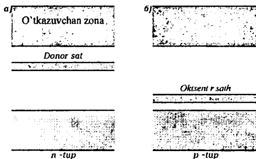
27.16-rasm. Aralashmagi yarimo'tkazgichlarda donor va akseptop energetit sathlar.
