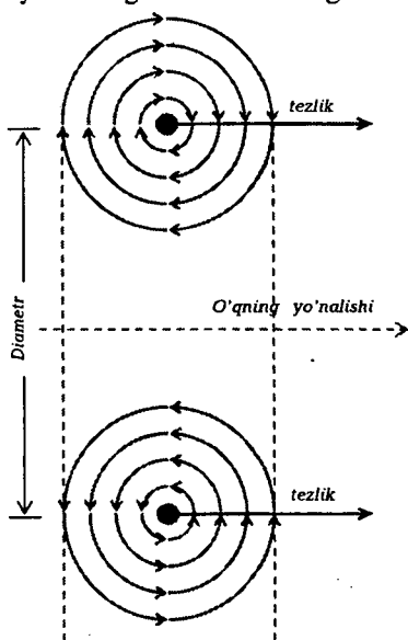
28.8-rasm. Suyda uyurma halqalari.
