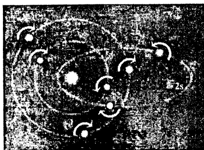
25.2-rasm. Azot atomi uchun Pauli printsipi va Xund qoidasini tatbiqi.
