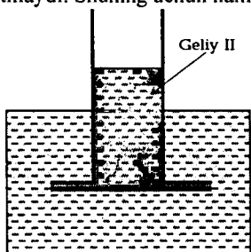
28.1-rasm. He-II ni o'ta oquvchanligi Ikkita silliq shisha plastinka orasidagi tor kanaldan Geliy-II bemolol oqib o'tadi. Suv esa bu kanaldan o'ta olmaydi.
