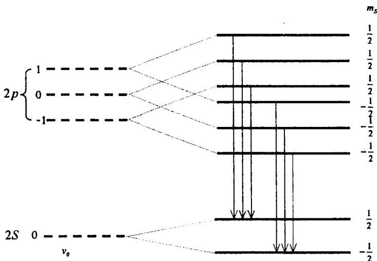
19.6-rasm. Pashen-Bak effekti (kuchli magnit maydonida) mavjudligiga doir natriy atomining nurlanishi bosh seriyadagi mumkin bo'lgan o'tishlar chizmasi.
