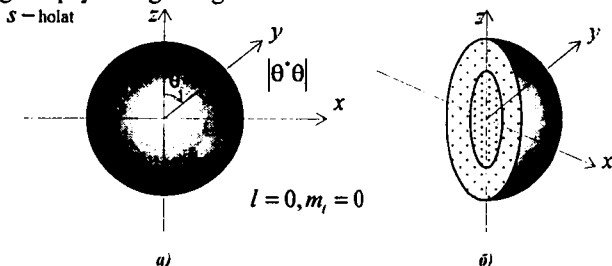
17.7-rasm. a) \theta - burchakka bog'liq bo'lgan p_\theta = |\theta'| holat uchun ehtimol zichligi; b) To'la ehtimol zichlik, burchak ehtimol zichligi p_\theta bilan radial ehtimol zichligi p_r ga ko'paytmasi
