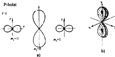
17.8-rasm. a) \theta - burchakka bog'liq bo'lgan p_\theta = |\theta'| va p_r = |\theta'_{1,1} \theta_{1,1}| holat uchun ehtimol zichligi; b) To'la ehtimol zichlik, burchak ehtimol zichligi p_\theta bilan radial ehtimol zichligi p_r ga ko'paytmasi.
