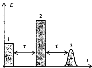
32.6-rasm. Foton sdosi
