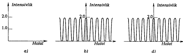
22.17-rasm. Ikkita to'liqinni qo'shilishi natijasida hosil bo'lgan normalangan intensivlik:
