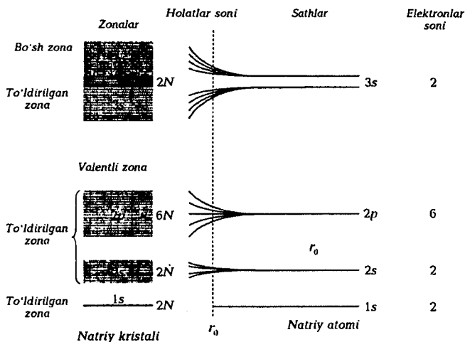
27.7-rasm. Natriy atomlarini bir-biriga yaqinlashganda atom satrlarining zonalarga ajralishi.
