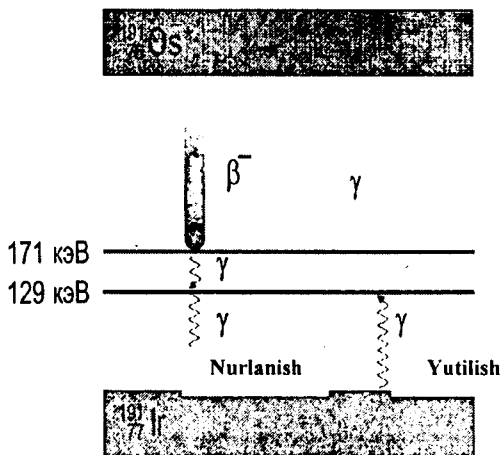
23.9-rasm. Osmiy 191 ning yemirilish chizmasi.
