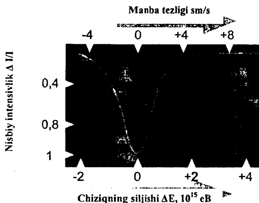
23.10-rasm. Yutgich nurlanish intensivligining manba tezligini o'zgarishiga bog'liqlik grafiki.
