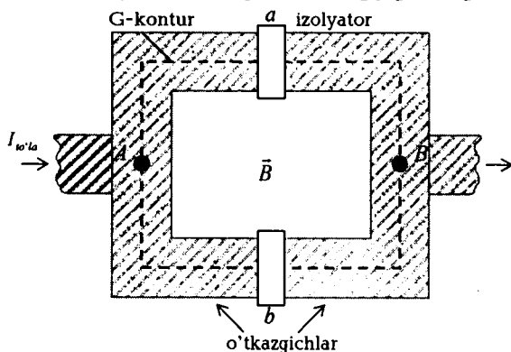
29.24-rasm. Bir-biriga parallel ulangan ikkita tunnel kontakt.
