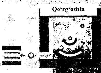
23.8-rasm. Myossbauerning eksperimental qurilmasining chizmasi.
