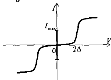
29.23-rasm. Namunaga past chastotadagi o'zgaruvchan tok berilganda I - V volt-ampere xarakteristikasi.
