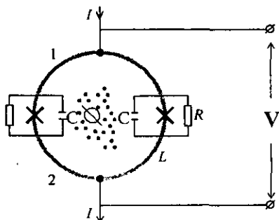
29.26-rasm. Magnit oqimi \Phi va o'rtacha tok I bo'lgan o'zgarmas tok SKVID sxemasi.
