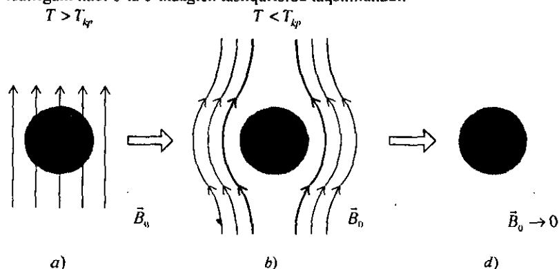
29.6-rasm. O'ta o'tkazgichda Meysner effekti.
