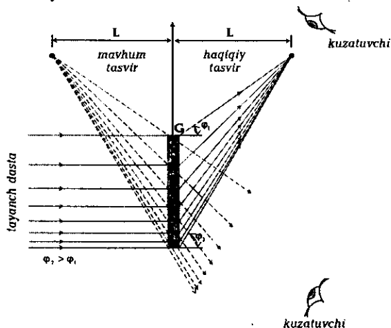
22.15-rasm. Gologrammadan tayanch dastaning o'ushi va obyektning haqiqiy va mayhum tasviri.
