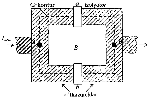
29.24-rasm. Bir-biriga parallel ulangan ikkita tunnel kontakt.
