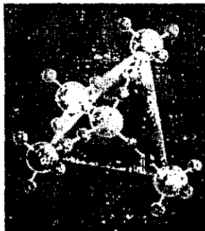
27.14-rasm. Germaniy strukturalari.
