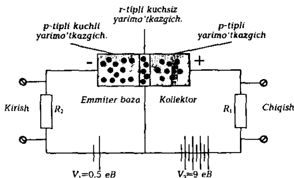
27.20-rasm. p-r-p tipidagi tranzistor chizmasi
