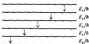
20.8- pacm . Garmonik ossillator uchun ruxsat etilgan o'tishlar
