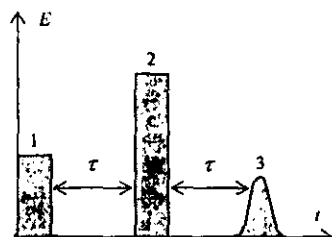
32.6-rasm. Foton sadosi
