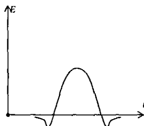
32.5-rasm. 0\pi impulsning shakli.
