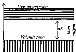
27.4-rasm. Kristallda energetik zonalarni soddalashtirilgan chizmasi.
