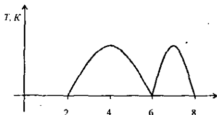
29.2-rasm. O'ta o'tkazuvchanlik holatiga o'tish temperaturasi valentli elektronlar soniga bog'liqligi grafiqi.
