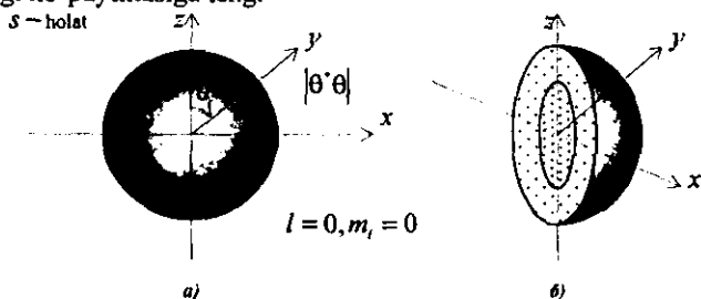
17.7-rasm. a) \theta - burchakka bog'liq bo'lgan p_\theta = |\theta|^2 holat uchun ehtimol zichligi; b) To'la ehtimol zichlik, burchak ehtimol zichligi p_\theta bilan radial ehtimol zichligi p_r ga ko'paytmasi
