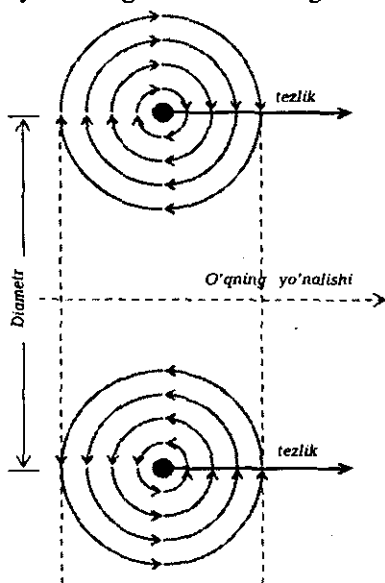
28.8-rasm. Suyda uyurma halqalari.
