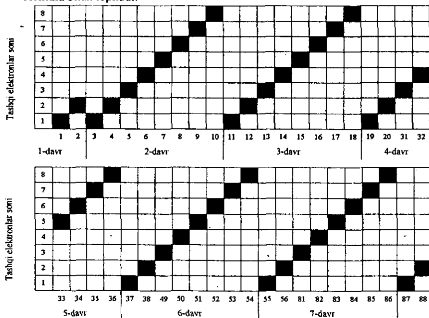
26.3-rasm. Elementlar atomlari tuzilishining davriy o'zgarishi.
