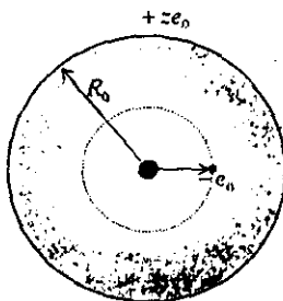
20.1-rasm. Vodorod atomi ( Z=1 ) uchun Tomson modeli. Ze_0 musbat zaryad radiusi R_0 bo'lgan sfera ichida bir tekis taqsimlangan. -e_0 zaryadga ega elektron atom markazidan x_0 masofa uzoqda turibdi.
