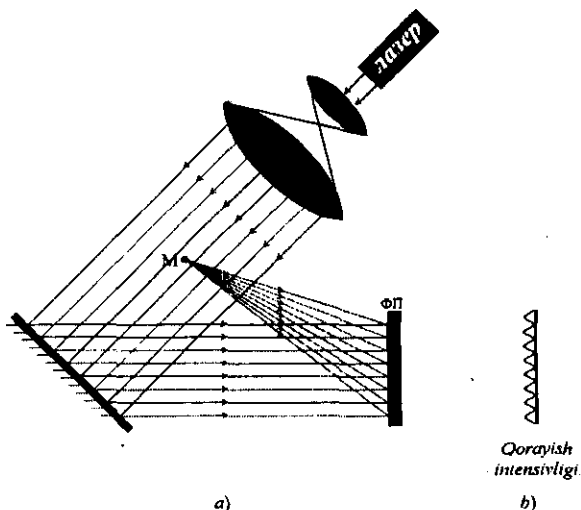
22.13-rasm. Nuqtaviy obyektning gologrammasi.
