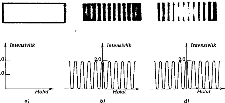
22.17-rasm. Ikkita to'liqni qo'shilishi natijasida hosil bo'lgan normalangan intensivlik:
