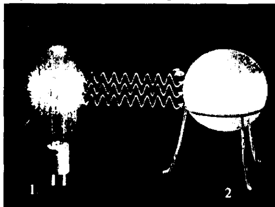
23.3.-rasm. Natriy bug'ini rezonansli yorug'lanishi. 1) Natriy bug'i joylashtirilgan lampochka; 2) rezonansli kovak.
