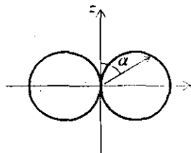
20.5-рису. Energiyaning burchak taqsimoti.
