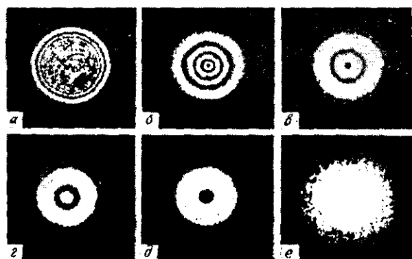
22.19-rasm. Doiravly tirqishda Frenel difraksiyasi. z_0 kattalik o'zgarmas, z esa a dan e gacha o'sib boradi.
