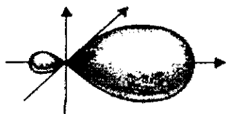
24.4-rasm. sp^3 -gibrid orbitali.
