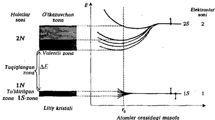
27.6-расм. Litiy kristalli uchun energetik zonalar. r_0 - kristall doimiysi
