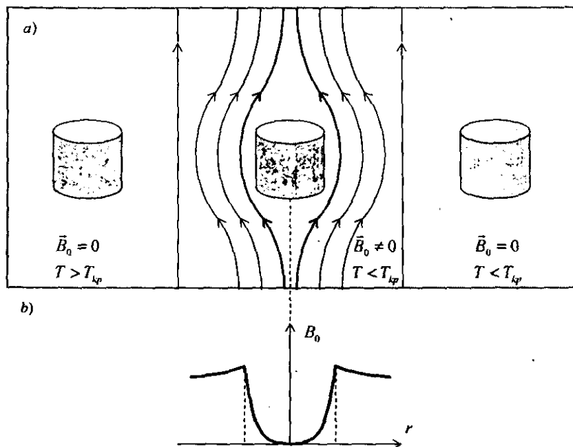
29.4- rasm a) Magnit maydonda o'ta o'tkazuvchan tsilindr b) \vec{B} magnit induksiyaning r ga bog'liqlik grafigi.
