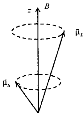
19.5-rasm. Kuchli magnit maydonda spin-orbital bog'lanishning uzilishi.
