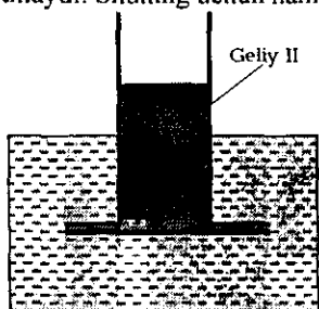
28.1-rasm. He-II ni o'ta oquvchanligi Ikkita silliq shisha plastinka orasidagi tor kanaldan Geliy-II bemolol oqib o'tadi. Suv esa bu kanaldan o'ta olmaydi.
