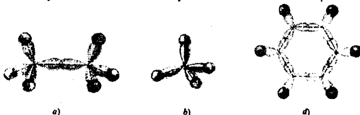
24.6-rasm. Molekula strukturalari.
