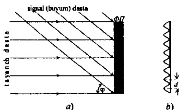
22.11-rasm. Qo'shni interferension tasmlar orasidagi masofa.
