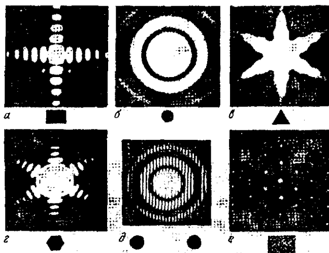
22.20-rasm. Ba'zi tirqishlarda Fraungofer difraksiyasi.
