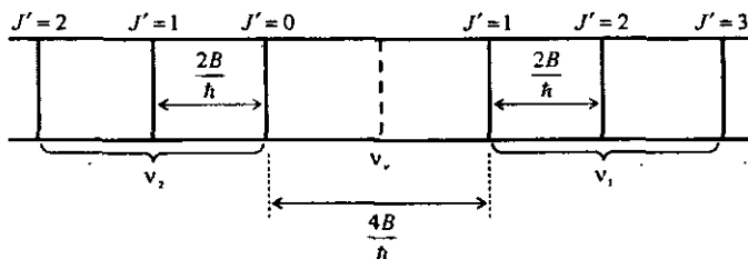
24.10-rasm. Ikki atomli molekulada tebranma-aylanma spektr chizmasi.
