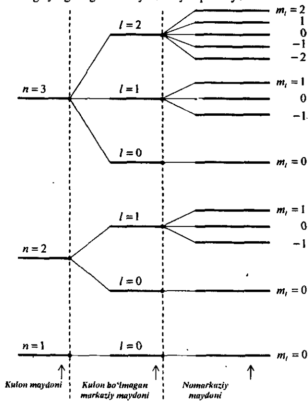
19.1-pacm. Vodorod atomining energetik sathlarni aynishi va yo'qolishi yo'llari.
