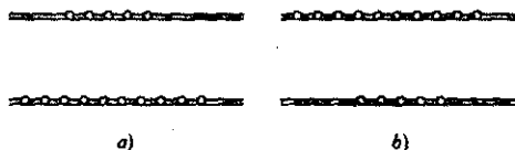
22.4-rasm. a) termodinamik muvozanat; b) inversiya holati.
