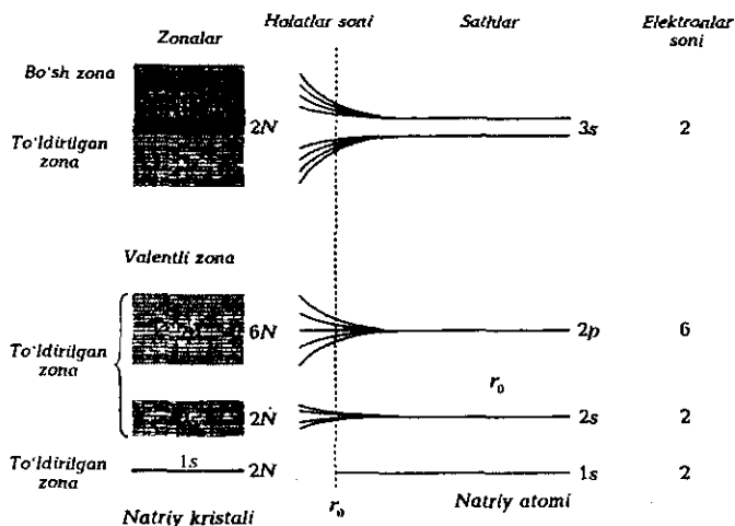
27.7-rasm. Natriy atomlarini bir-biriga yaqinlashganda atom sathlarining zonalarga ajralishi.
