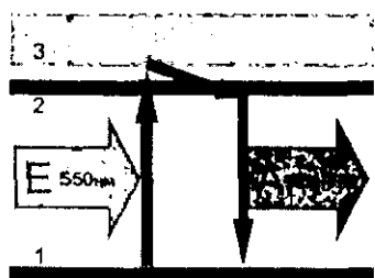
22.9-rasm. Yoqut lazerida xrom ionlari termlaridan ayrimlarining chizmasi. A – tushayotgan yasxil yorug'lik nuri. V – lazer nurlayotgan qizil nuri.
