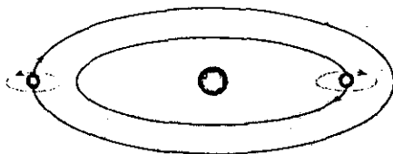
26.6-rasm. Ortogeliy orbitalari.
