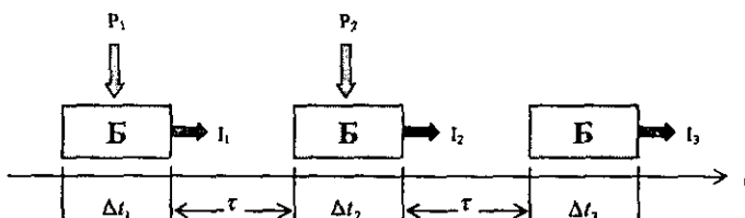
32.7-rasm. Sado jarayoni.
