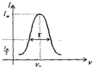
23.2-rasm. Rezonans egriligi va uning kengligi.
