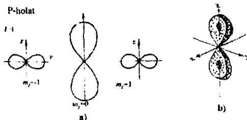
17.8-rasm. a) \theta - burchakka bog'liq bo'lgan p_\theta = |\theta_{1,-1}|^2 va p_\theta = |\theta_{1,0}|^2 holat uchun ehtimol zichligi; b) To'la ehtimol zichlik, burchak ehtimol zichligi p_\theta bilan radial ehtimol zichligi p_r ga ko'paytmasi.
