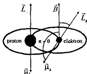
18.2-rasm. Vodorod atomida elektron va proton harakati.
