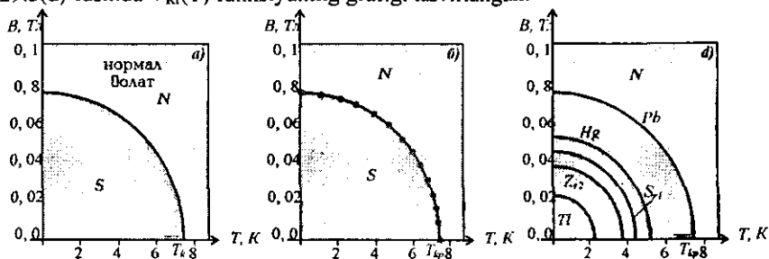
29.3-rasm. Kritik magnit induksiya V_{kr} ni temperatura T ga bog'liqlik grafigi.
