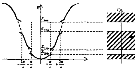
27.2-rasm. Kristallda erkin elektronlar energiyasi E ni to'liqin son k ga bog'liqlik grafigi.
