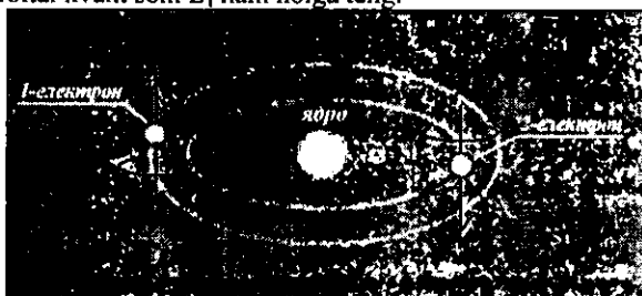
25.4-rasm. Geliy atomining orbitali.
