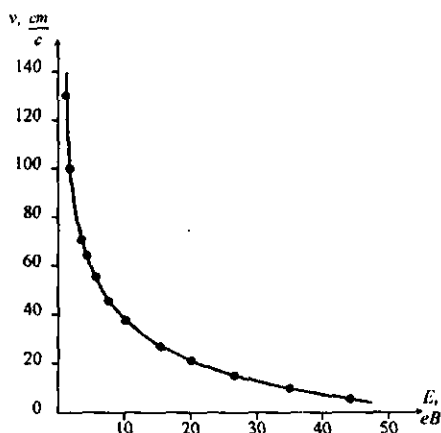
28.10-rasm. Zaryad tashuvchilar tezligini energiyasiga bog'liqlik grafigi.
