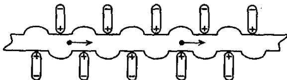
29.28-rasm. O'ta o'tkazuvchan organik o'ta o'tkazgich (Littl modeli).
