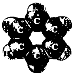
e) Benzol molekulasining modeli (siklik formasi)
