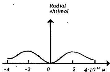
2p n uyg'ongan holatda elektronning radial ehtimol zichligi
