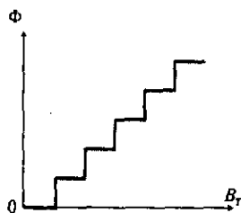
29.11-rasm. Halqa teshigida ushlanib qolgan magnit oqimi tashqi magnit maydon induktsiyasiga bog'liqlik grafigi.
