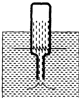
28.3-rasm. Geliy II ning fontan effekti.
