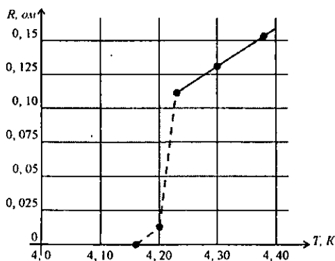
29.1-rasm. Simob metalini elektr qarshiligini temperaturaga bog'liqligi grafiki.
