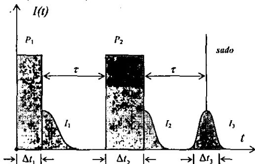
32.8-rasm. Vaqt bo'yicha foton sadosi. I(t) – javoblar (sadolar) intensivligi; I_1 , I_2 va I_3 mos ravishda, 1– 2–, 3– induksiya va sado intensivliklari; t –vaqt, R_1 va R_2 uyg'otuvchi impuls; \Delta t_1 va \Delta t_2 ularning davomiyligi.
