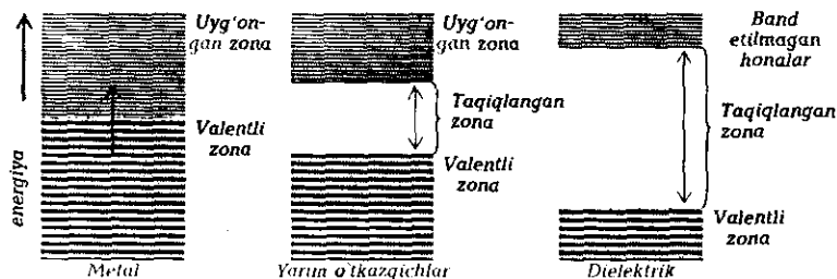
27.5-rasm. Metall, dielektrik va yarim o'tkazgichlar uchun taqiqlangan va o'tkazuvchan zonalar.
