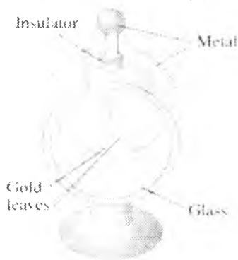
13.4-rasm. Elektroskop
