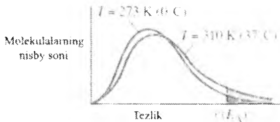
11-1-rasm. Ikki xil temperatura uchun molekulalar tezliklarining taqsimoti
