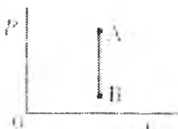
10-6-rasm. a) Izobarik jarayon. B) Izoxorik jarayon.
