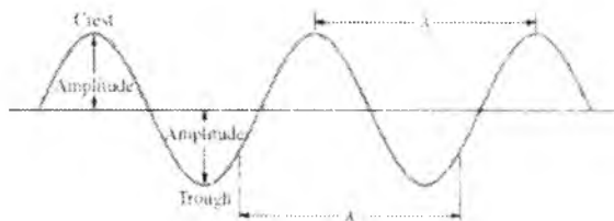
8-8-rasm. Davriy to'lqinni xarakterlovchi kattaliklar.
