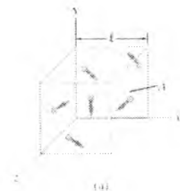
9-4(a)-rasm. To'g'ri burchakli idishda gaz molekulalari joylashgan.
