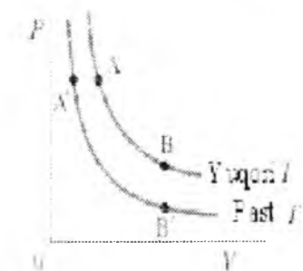
10-4 PV diagrammada ideal gazning izotermik jarayonda ikki xil temperaturada pasayishi
