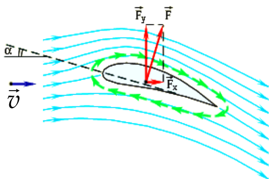
Рис.10.18. Подъемная сила крыла самолета
