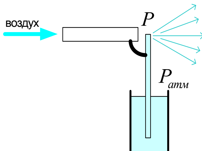
Рис.10.19. Пульверизатор
