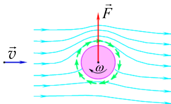
Рис.10.20. Полет закрученного мяча
