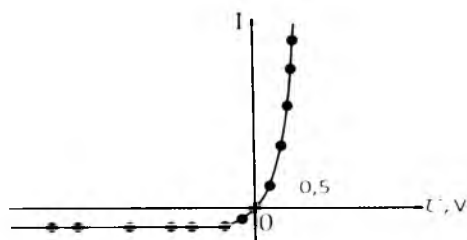
343 - rasm. Elektron - kavakli o'tishning volt - amper xarakteristikasi
