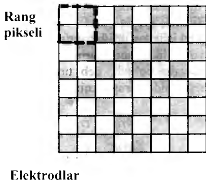
198 - rasm. Bayerning matritsali sensorining bir qismi. To'rtburchak ichidagi to'rt pikselarni \begin{matrix} R & G \\ G & B \end{matrix} "rang" pikseli ham deyishadi
