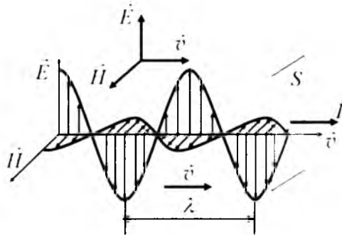
179 - rasm. Elektromagnit to'lqinning elektr va magnit kuchlanganlik vektorlari yo'nalishlari
