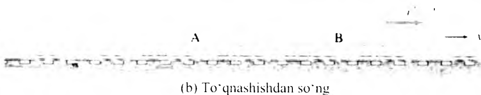
20 - rasm. Vagonlar to'qnashishi
