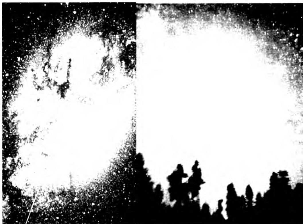
352 - rasm. Somon yo'li galaktikasining bir qismi. (a) rasmdagi ingichka chiziqli qorong'i diagonal soha yorug'likning galaktika changlari tomonidan yutilishi hisobiga hosil bo'lgan. (b) rasm galaktika markazi tomonidan ko'rinishi (Arizona (AQSH) yozida tasvirga olingan)
