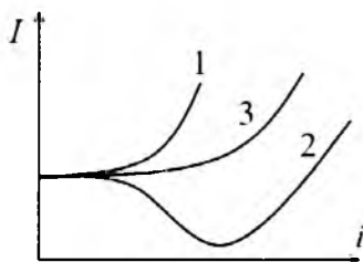
224 - rasm. Qaytgan yorug'lik nuri jadalligining tushish burchagiga bog'liqligi
