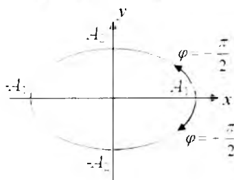
159 -rasm. Fazalar farqi \pm \frac{\pi}{2} ga teng bo'lgan tebranishlar qo'shilishidagi natijaviy tebranish
