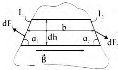
115 - rasm. Yassi kontur tekisligiga parallel bo'lgan magnit maydonining ta'siri
