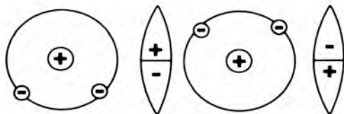
278 - rasm. Geliy atomlarida tortishish kuchlarini hosil boʻlishi
