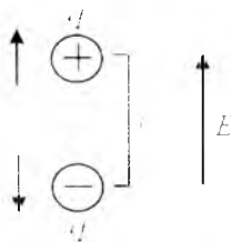
53 - rasm. Tashqi elektrostatik maydon taʼsirida qutbsiz molekulaning dipol momentiga ega boʻlishi
