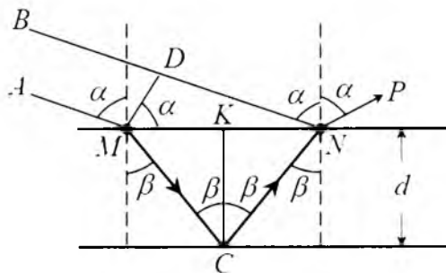
204 - rasm. Yupqa tiniq plastinkadagi yorugʻlik interferensiyasi
