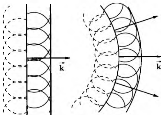
176 - rasm. Ikkilamchi to'liqlarning hosil bo'lish markazlari
