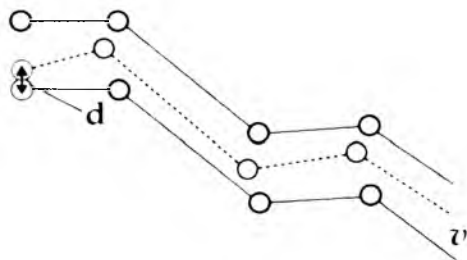
257 - rasm. Molekulalarning oʻzaro toʻqnashish xarakteri
