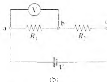
95 - rasm. Qarshiliklar ketma-ket ulangan zanjir
