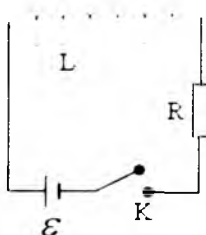
137 - rasm. Induktivlik va qarshilikdan iborat elektr zanjiri
