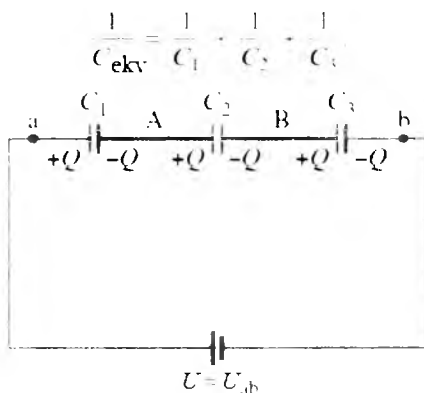
86 - rasn. Ketma-ket ulangan kondensatorlar
