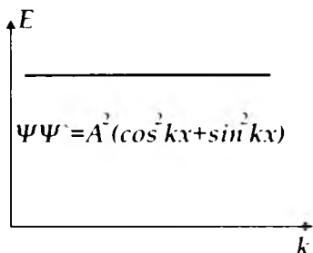
300 - rasm. Erkin elektronning fazoda bo'lish ehtimoligi
