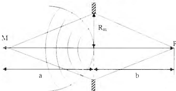
210 - rasm. Dumaloq teshikli ekrandagi difraksiya
