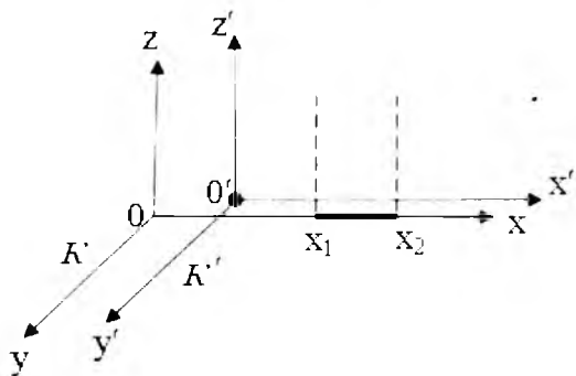
28 - rasm. Bir-biriga nisbatan harakatda bo'lgan sanoq tizimida uzunlik o'lchamining o'zgarishi
