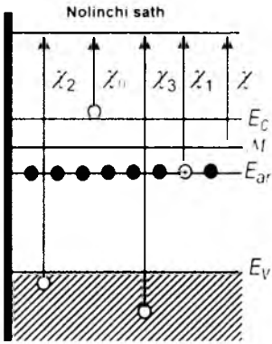
328 - rasm. Elektron tipli yarim oʻtkazgichda elektronlarning vakuumga chiqish yoʻllari
