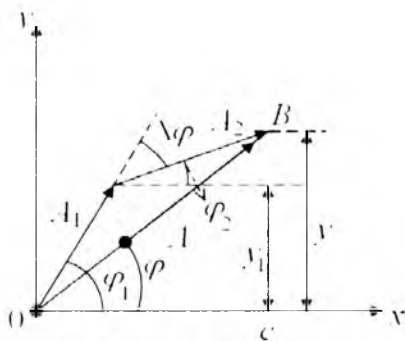
155 - rasm. Bir yo'nalishdagi tebranishlarni vektorlar diagrammasi usulida qo'shish
