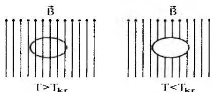
320- rasm. O'ta o'tkazuvchanlik hodisasida qattiq jismlarda magnit maydonini siqib chiqarish
