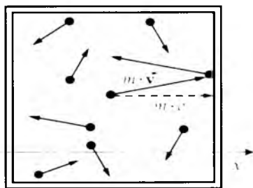
251 - rasm. Yuzaga perpendikulyar harakat qilayotgan molekular urilganda yuzaga keluvchi impuls
