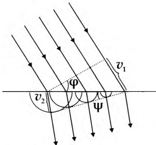
200 - rasm. Ikkita tiniq muhit chegarasida ikkilamchi toʻlqinlar manbalarining hosil boʻlishi
