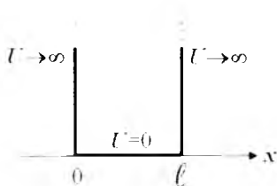
238 - rasm. Devorlari cheksiz baland bo'lgan potensial chuqurlik
