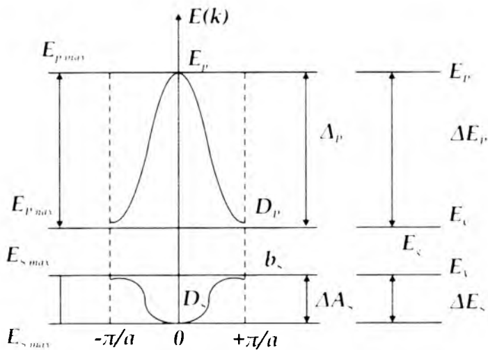
302 - rasm. S – va P – sohalarining dispersiya chiziqlari
