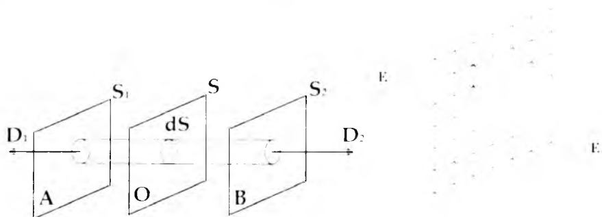
42 - rasm. Bir tekis zaryadlangan cheksiz tekislik
