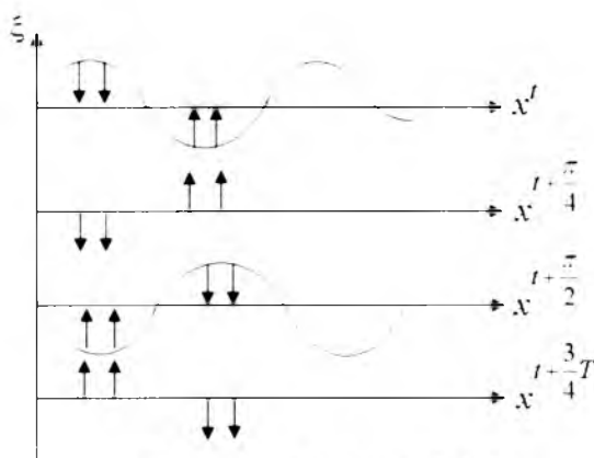
175 - rasm. Turg'un to'liqlar
