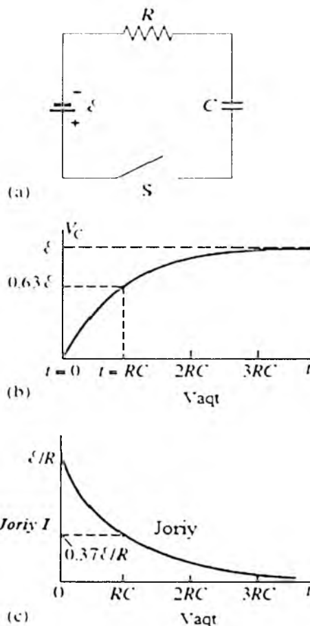
88 - rasm. (a) S kalit ulanganda RC -zanjir qisqa tutashadi; (b) kondensatordagi kuchlanish U_C vaqt o'tishi bilan ortaboradi; (c) qarshilik orqali o'tayotgan tok \mathcal{E}/R vaqt o'tishi bilan kamayadi
