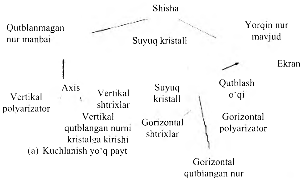
228 - rasm. (a) Suyuq kristallning "o'ralgan" shakli. Nurning qutblamish tekisligi 90^\circ ga aylantirilgan va gorizontall polyarizatorga yuborilgan. Faqatgina bir qator molekulalar tasvirlangan. (b) Molekulalar elektr maydoni ta'sirida tartibsizlanadi. Qutblanish tekisligi o'zgarmadi, shuning uchun nur gorizontall polyarizator orasidan o'tmadi
