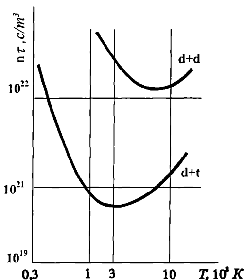
5.15-rasm. Deyteriy-tritdiy, deyteriy-deyteriy reaksiyalari uchun plazmani ushlab parametrlarining temperaturaga bog'liqligi.
