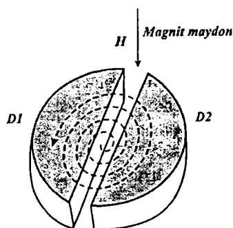
5.1-rasm. Siklotron. Siklotronda ionlar harakati.
