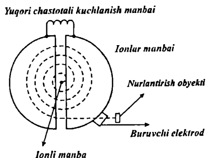
5.1-rasm. Siklotron. Siklotronda ionlar harakati.
