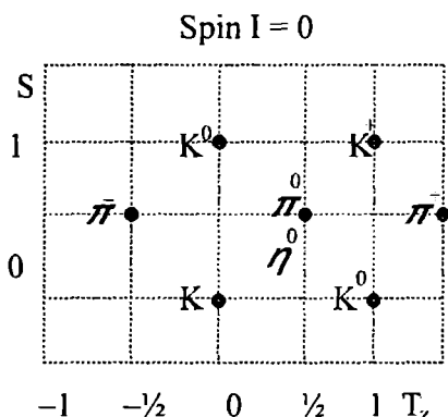
b) Mezon oktet
