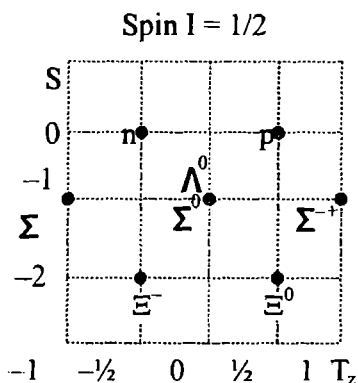
a) Barion oktet
