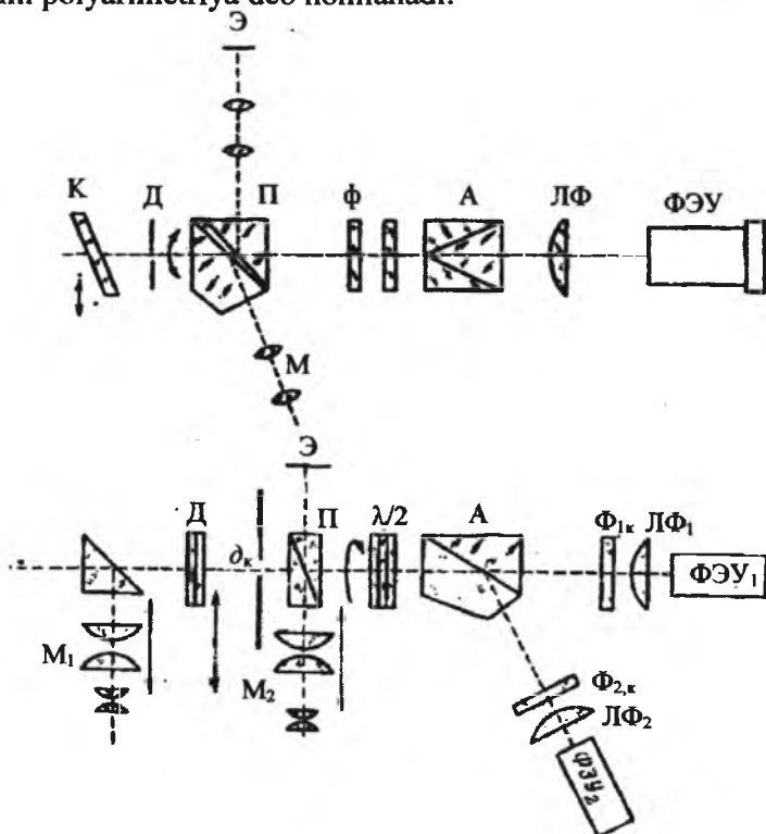
44-rasm. Bir va ikki nurlı elektropolyarimetrlar.
