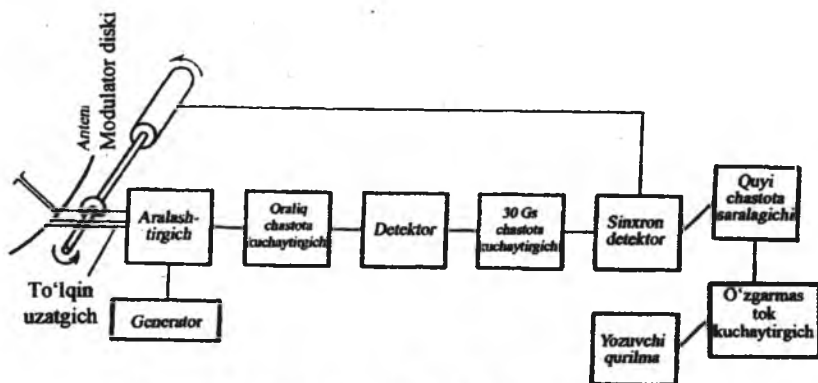
40-rasm. Modultatsiyali radiometrning sxemasi
