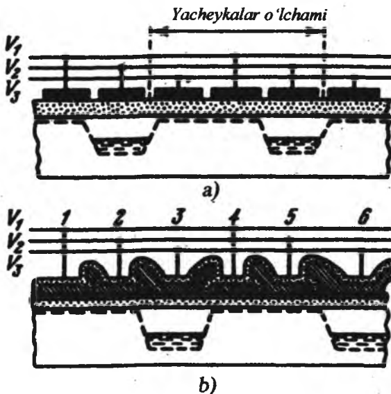
33-rasm. ZO'A lanning bir qatlamli va uch qatlamli strukturalari.
