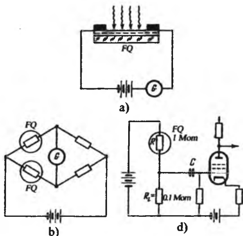
29-rasm. Fotoqarshilikni ulash sxemalari.
