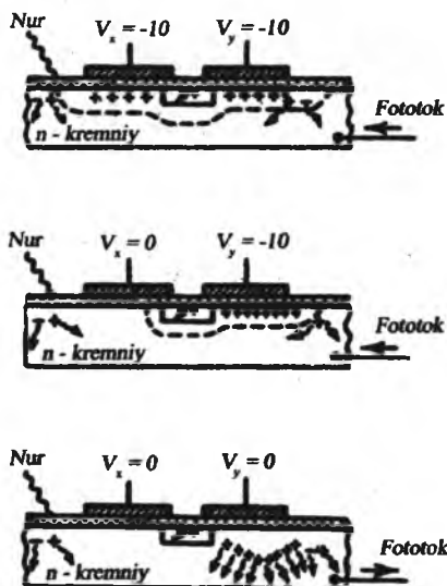
36-rasm. Zaryadlari injeksiya qilinadigan ZO'A uyachaning ishlash sxemasi.
