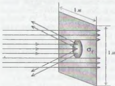
20.6-расм. Sochilishning Tompson kesimi ( \sigma_T ).
