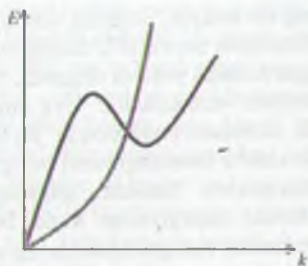
28.4-rasm. Real zarra va kvazizarralar uchun energiya va implus bog'liqligi grafigi.
