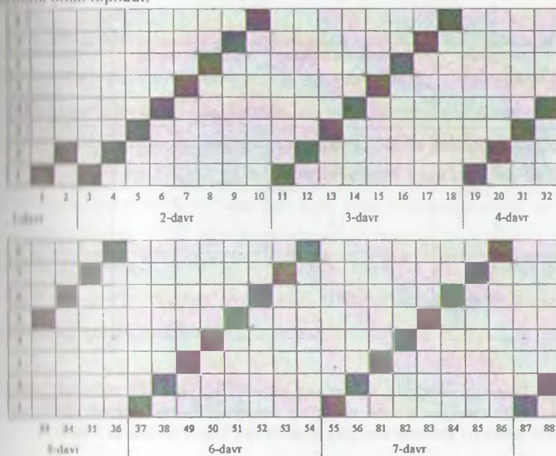
26.3-rasm. Elementlar atomlari tuzilishining davriy o'zgarishi.
