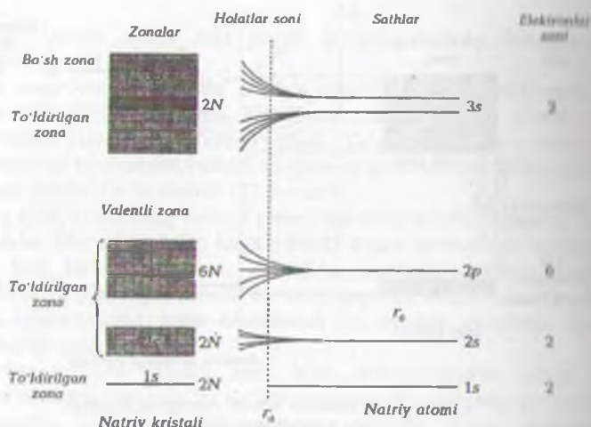
27.7-rasm. Natriy atomlarini bir-biriga yaqinlashganda atom sathlarining zonalariga ajralishi.
