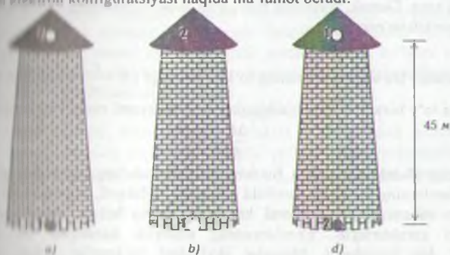
21.16-rasm. Gravitatsion maydonida gamma kvantni qizil siljishi. R.V.Paund va G.A.Rebke tajribasi.
