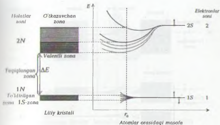
27.6-расм. Литий кристалли uchun energetik zonalar. r_0 - кристалл доимийси
