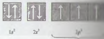
Azot atomining elektron konfiguratsiyasi
