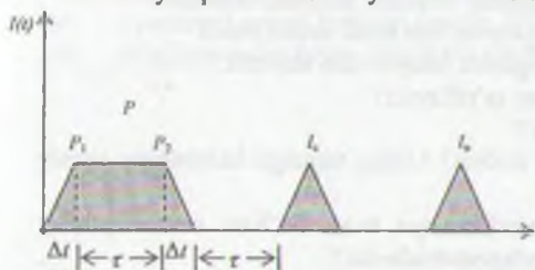
32.12-rasm. Chekkaviy va ko'p karrali sado. R uyq'otuvchi impuls, \Delta t va T chekkani davomligi va davomlilik. I_K - chekkaviy sado, I_K - ko'p karrali sado.
