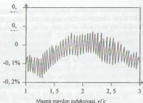
30.6-rasm Aaronov-Bom effektini oltin uzukcha bilan qilingan eksperiment grafiqi.
