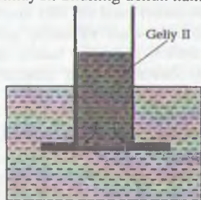
28.1-rasm. He-II ni o'ta oquvchanligi Ikkita silliq shisha plastinka orasiidagi tor kanaldan Geliy-II bemolol oqib o'tadi. Suv esa bu kanaldan o'ta olmaydi.
