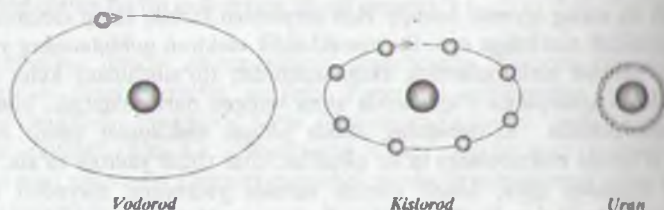
26.1-rasm. Energiya minimumi prinsipi asosida atomlarning qobig'ini elektronlar bilan to'ldirishi.
