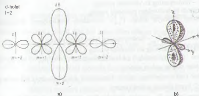
17.9-rasm. a) \theta - burchakka bog'liq bo'lgan p_{\theta} = |\theta'_{2,1}, \theta'_{2,-1}| va p_{\theta} = |\theta'_{2,0}, \theta'_{2,2}| holat uchun ehtimol zichligi; b) To'la ehtimol zichlik, burchak ehtimol zichligi p_{\theta} bilan radial ehtimol zichligi p_r ga ko'paytmasi.
