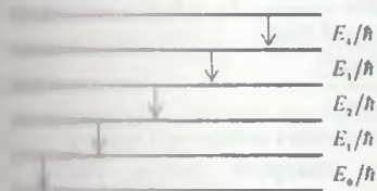
10.8-rasm. Garmionik ossillator uchun ruzat etilgan o'tishlar
