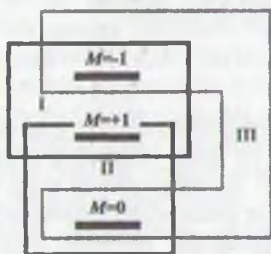
32.10-rasm. Ko'p sathli sistemalar dinamikasi Spektr turlari: a) ekvidistant, b) noekvidistant, d) aynigan; v_1, v_2, v_3, v_+ = v_- sistemaning rezonans chastotalari, e), f) turli doiraviy qutblangan fotonlar. \vec{v} - harakat yo'nalishidagi tezlik. M - burchak momenti vektorining yo'nalishi.
