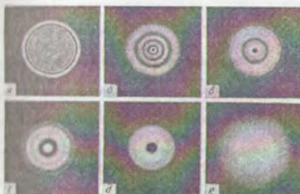
22.19-rasm. Doiraviy tirqishda Frenel difraksiyasi.
