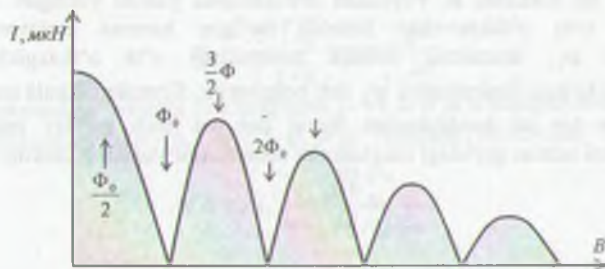
29.20-rasm. Djozefson tokiini B magnit maydon induksiya B ga bog'liqligi.
