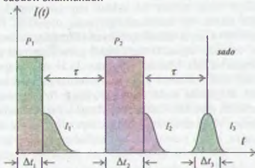
32.8-rasm. Vaqt bo'yicha foton sadosi. I(t) – javoblar (sadolar) intensivligi; I_1 , I_2 va I_3 mos ravishda, 1–, 2–, 3– induksiya va sado intensivliklari; \tau –vaqt, R_1 va R_2 uyg'otuvchi impuls; \Delta t_1 va \Delta t_2 ularning davomiyligi.
