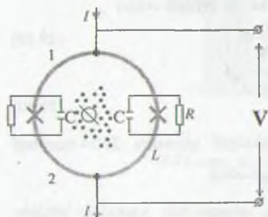
29.26-rasm. Magnit oqimi \Phi va o'rtacha tok I bo'lgan o'zgarmas tok SKVID sxemasi.
