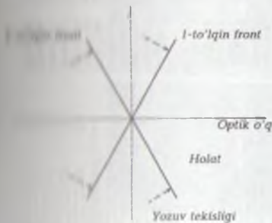
22.38-rasm. Optik o'qqa nisbatan simmetrik joylashgan ikkita yassi to'lqinlarni qo'shish.
