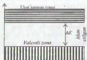
27.4-rasm. Kristallda energetik zonalarini soddalashtirilgan chizmasi.
