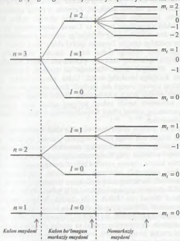
19.1-pasm. Vodorod atomining energetik sathlarni aynishi va yo'qolishi yo'llari.
