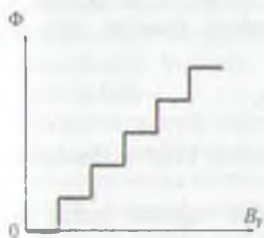
29.11-rasm. Halqa teshigida ushlanib qolgan magnit oqimi tashqi magnit maydon induksiyasiga bog'liqlik grafiki.
