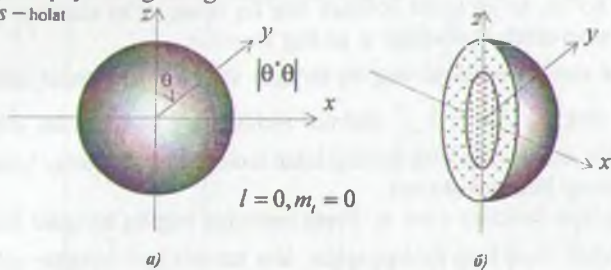
17.7-rasm. a) \theta - burchakka bog'liq bo'lgan p_\theta = |\theta|^2 holat uchun ehtimol zichligi; b) To'la ehtimol zichlik, burchak ehtimol zichligi p_\theta bilan radial ehtimol zichligi p_r ga ko'paytmasi
