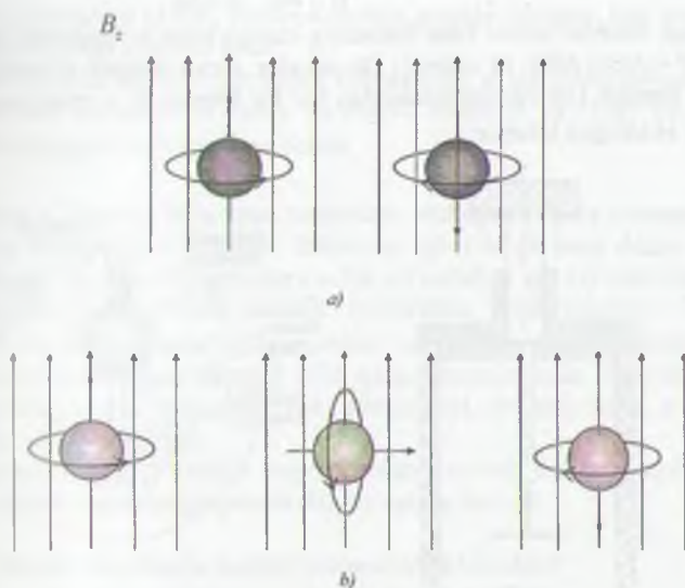
18.3-rasm. a) Spini \frac{1}{2} ga teng bo'lgan zarralarning tashqi magnit maydonga nisbatan olgan holatlari. Oqizil ko'rsatkichlar tashqi magnit maydon yo'nalishini ko'rsatadi. Bunday holat elektron, proton, neytron kabi zarralar uchun o'rinalidir.
