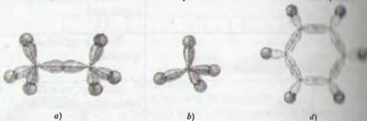
24.6-rasm. Molekula strukturalari.
