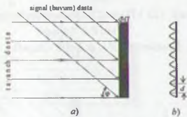
22.11-rasm. Qo'shni interferensiya tasmlar orasidagi masofa.
