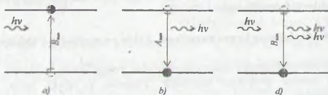
20.7-рису. Atomda pastdan yuqoriga ( n \rightarrow m ) va yuqoridan pastga ( m \rightarrow n ) o'tishlar. a) yutilish; b) spontan nurlanish; d) induksirlangan (majburlangan) nurlanish.
