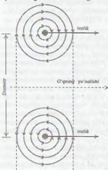
28.8-rasm. Suva uyurma halqalari.
