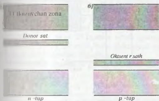
27.16-rasm. Aralashmaga yarimo'tkazgichlarda donor va akseptor energetik sathlar.
