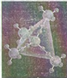
27.14-rasm. Germaniy strukturasini.
