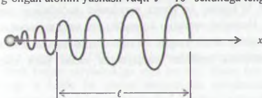
20.2-rasm. Yorug'lik impuls yoki to'lqinlar sistemasi - sug.
