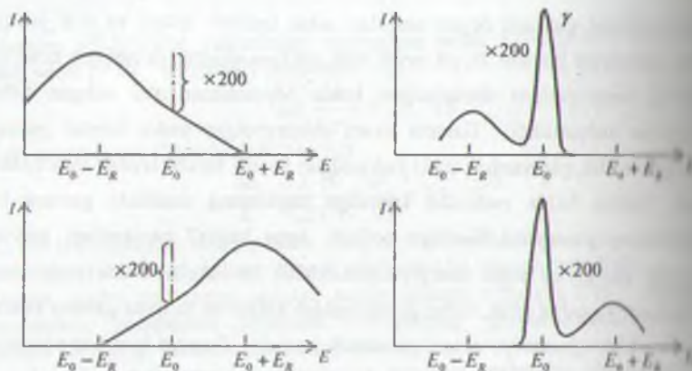
23.7-rasm. 88 K temperaturada ^{191}_{77}\text{Ir} -iridiy izotopi uchun gamma kvantlarini chiqarilishi va yutilishi.
