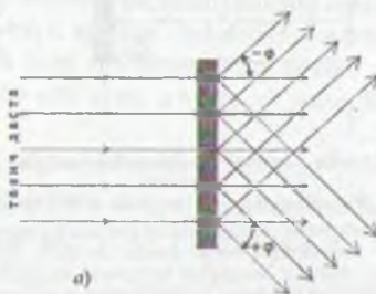
22.12-rasm. Gologrammada faqat tayanch dasta o'tishi ratijasida uchta to'qlin hosil bo'lishi.
