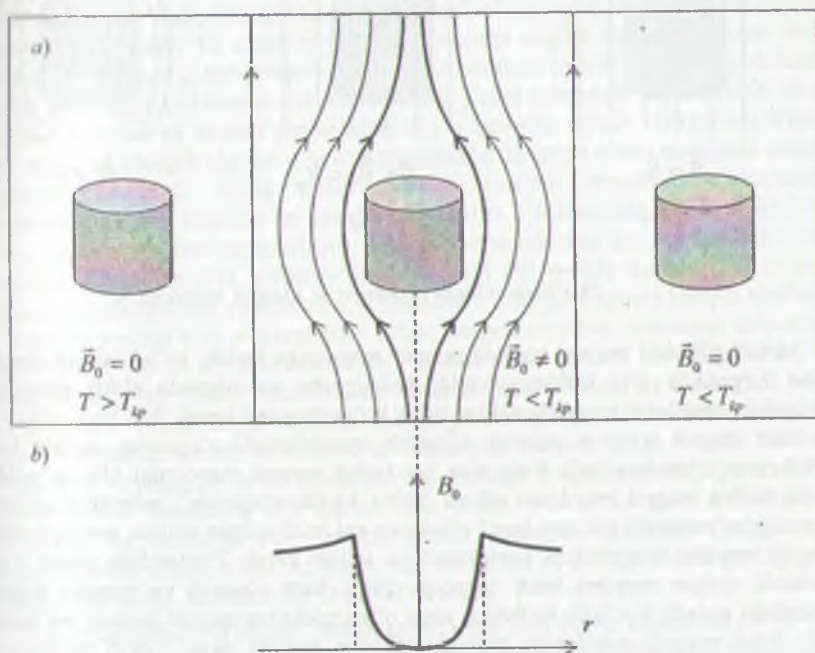
29.4- rasm a) Magnit maydonda o'ta o'tkazuvchan tsilindr b) \vec{B} magnit induksiyaning r ga bog'liqlik grafigi.
