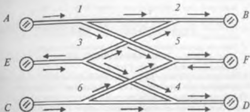
7.11-rasm. Tolali optik tarmoqlagichlar blokining tuzilish sxemasi
