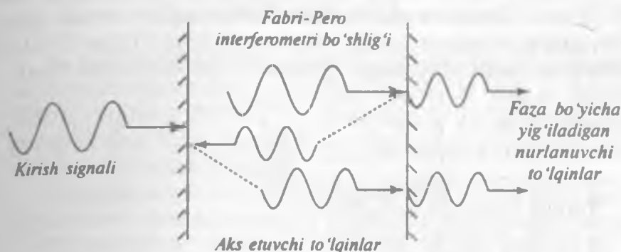
8.1-rasm. Yorug'lik nurlanishini Fabri-Pero rezonatori yordamida filtrlash
