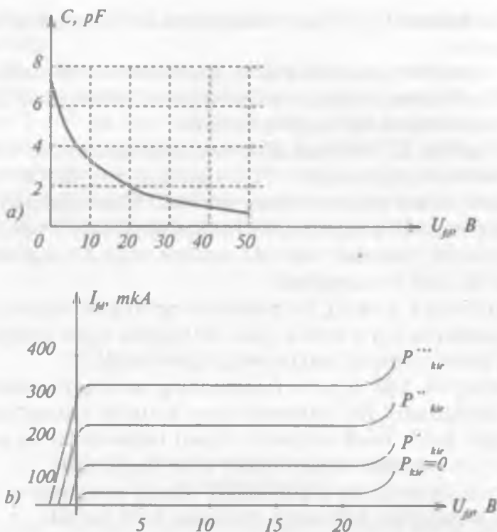
4.7-rasm. SP109 fotodiodining volt-farada (a) va volt-ampér (b) xarakteristikalari
