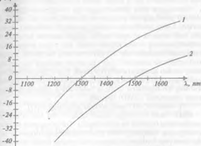
2.21- rasm. Xromatik dispersiyaning to‘lqin uzunligiga bog‘liqligi:
