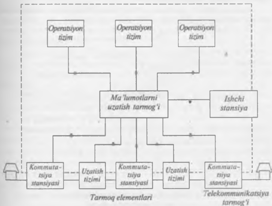
13.4-rasm. Telekommunikatsiyalarni boshqarish tarmog'i va aloqa tarmog'i o'rtasidagi o'zaro bog'liqlik
