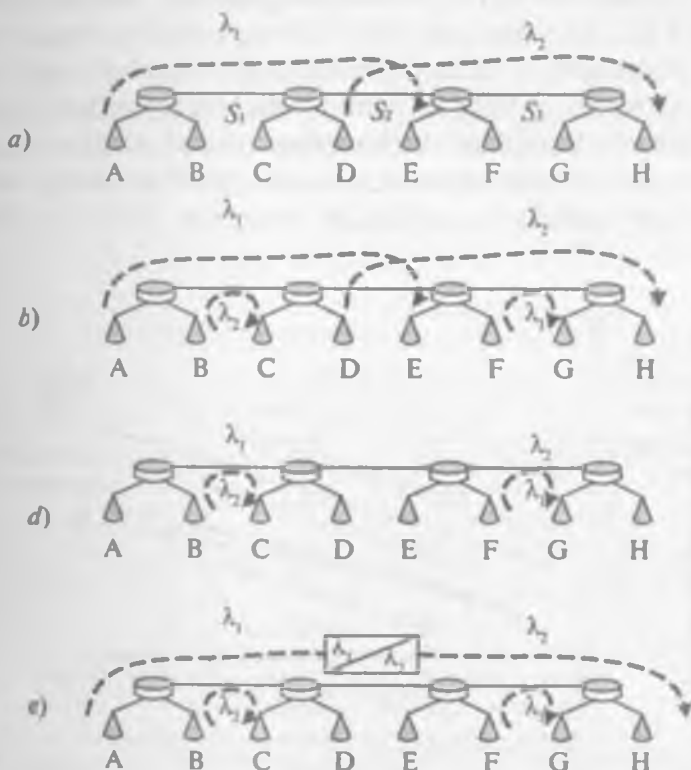
12.5-rasm. Dinamik to'liqin marshrutlashtirishli optik tarmoq: a – tarmoqda to'liqin konversiyasiz vujudga keladigan cheklanishlar; c – to'liqin konversiyasi tarmoqni yanada o'zgaruvchan qiladi
