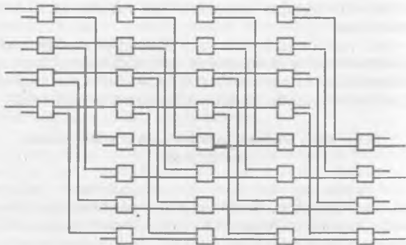
10.5-rasm. Karrali matritsa sxemasi
