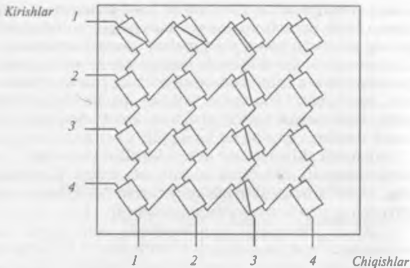
10.4.-rasm. Matritsali kommutator sxemasi
