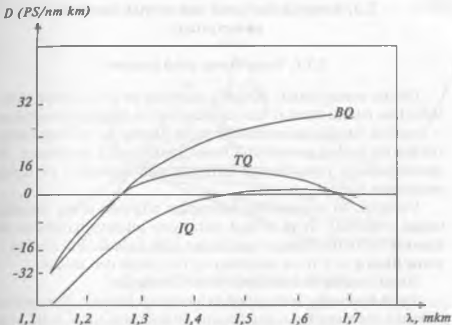
2.8-rasm. Dispersiyaning to'liqin uzunligi va qobiqlar soniga bog'liqligi:
