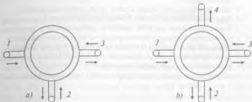
8.7-rasm. Optik sirkulatorning sxemasi
