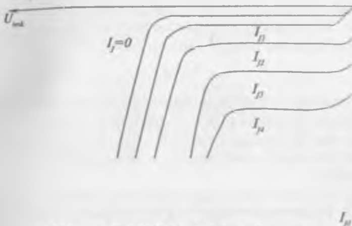
4.11-rasm. Ko'chkili fotodiodning volt-ampyer xarakteristikalarlari oilasi
