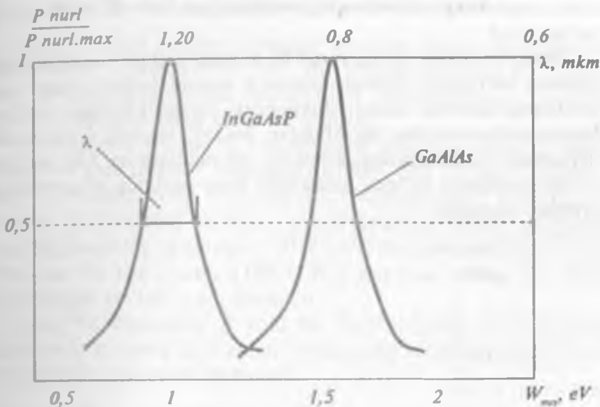
3.5-rasm. InGaAsP va Ga As asosidagi yorug'lik diodlarining spektral xarakteristikalari
