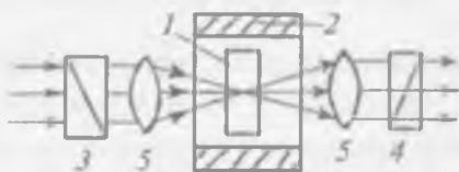
6.10- rasm. Magnitooptik modulyatorning tuzilish sxemasi: 1 – aktiv muhit (magnitooptik moda); 2 – induksiyalovchi g'altak; 3 – qutblagich; 4 – tahlillagich (analizator); 5 – linza.
