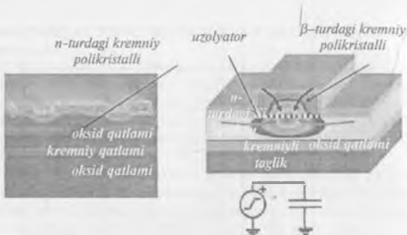
6.12-rasm. Kremniyli fazaviy optik modulnya torning tuzilishi
