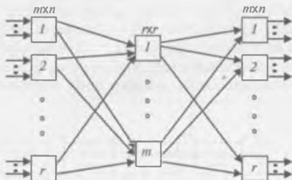
10.7-rasm. Uch tekislikli fazoviy kommutator
