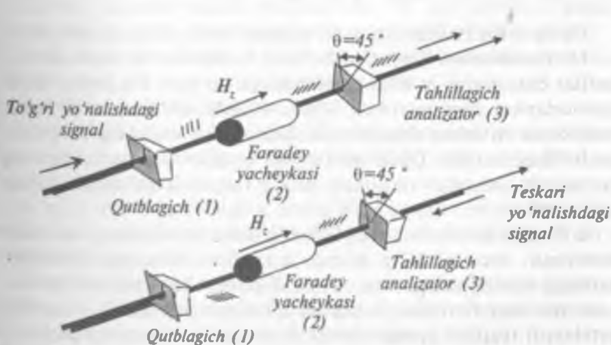
8.6-rasm. Optik izolatorning tuzilish sxemasi va ish prinsipi: a – to'g'ri yo'nalishdagi foydali optik signal undan to'siqsiz o'tadi; b – teskari yo'nalishdagi zararli signal qutblagich orqali o'tmaydi
