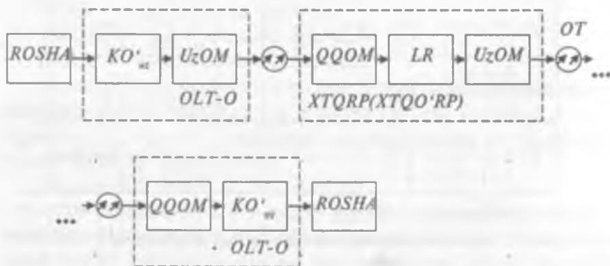
11.4-rasm. Raqamli TOATda regeneratori qo'llanilgan optik liniya traktining tuzilish sxemasi
