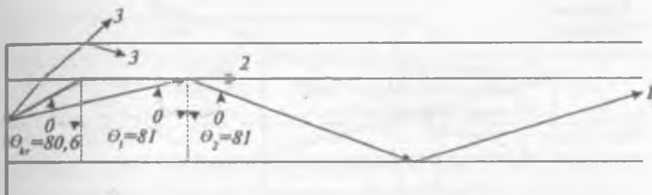
2.12-rasm. Optik to'ida to'liq ichki qaytish jarayoni
