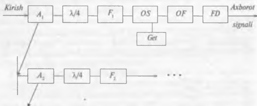
1.12-rasm. Chastota bo'yicha (geterodinli) zichlashtirishda guruhli optik signallarni qabul qilish sxemasi
