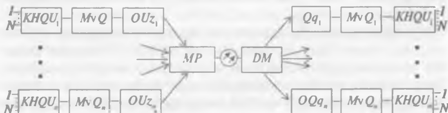
1.8-rasm. To'liqin uzunligi bo'yicha zichlashtirilgan TOATning tuzilish sxemasi
