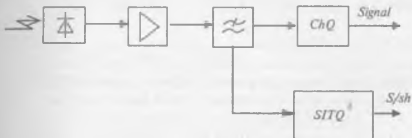
6.13-rasm. Raqamli signal bilan modulyatsiyalangan optik nurlanishni qabul qiluvchi fotoqabulqilgich
