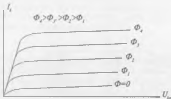
4.13-rasm. Bipolar fototranzistorning volt-ampere xarakteristikalar oilasi
