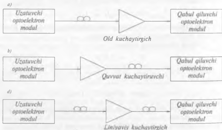
5.11-rasm. Optik kuchaytirgichlarning tolali optik uzatish tizimlarida qo'llanish usullari:
