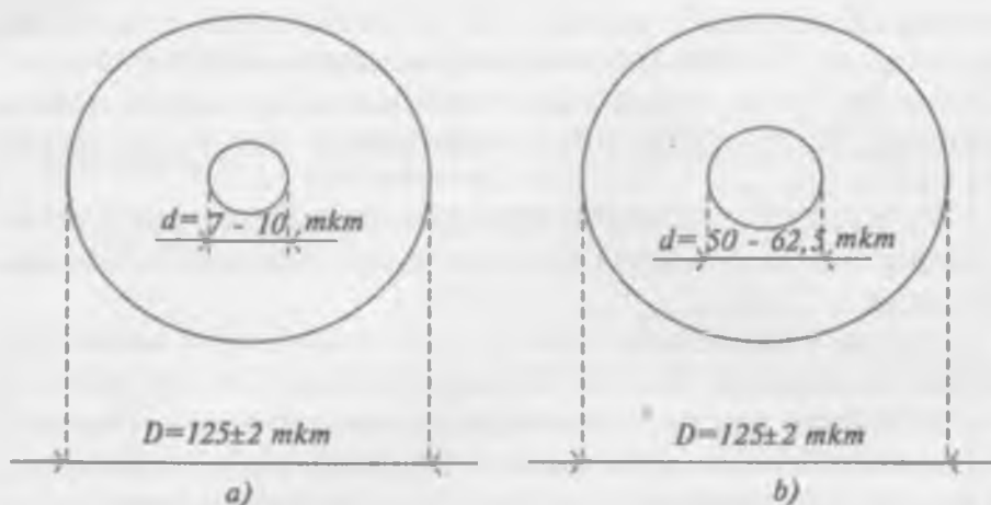
2.3-rasm. Bir modali (a) va ko'p modali (b) optik tolalarning ko'ndalang kesimi
