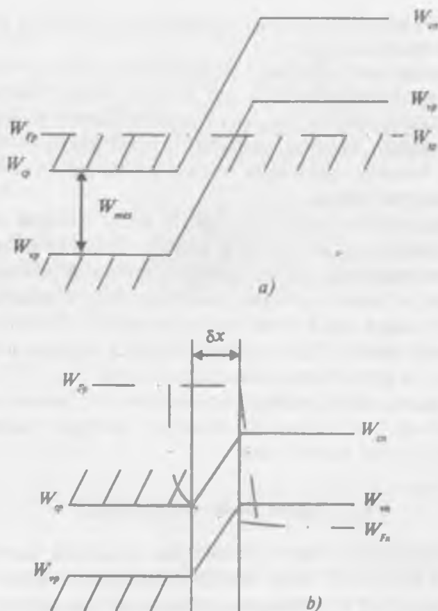
3.13-rasm. Aynigan yarimo'tkazgichlardan tayyorlangan p - n o'tishning termodinamik muvozanat holatdagi (a) va to'g'ri ulangan holdagi (b) energetik diagrammasi
