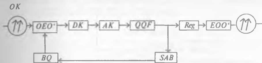
11.1-rasm. Raqamli retranslyator-regeneratorning umumlashgan tuzilish sxemasi
