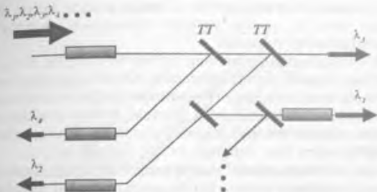
9.3-rasm. Guruhiiy signalni demultipleksorlash uchun ishlatiladigan yupqa pardali filtrlarning ko'p pog'onali tizimi
