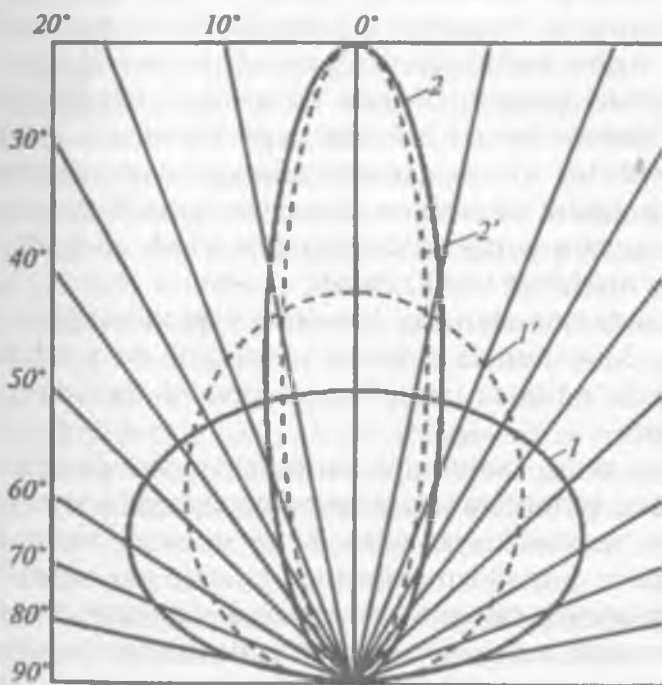
3.7-rasm. Yorug'lik diodlarining yo'nalganlik diagrammalari: 1,1' – qaytargichsiz, 2,2' – qaytargichli GaAs va GaP diodlari
