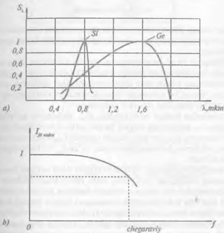
4.4-rasm. Fotodiodning spektral (a) va chastotaviy (b) xarakteristikallari
