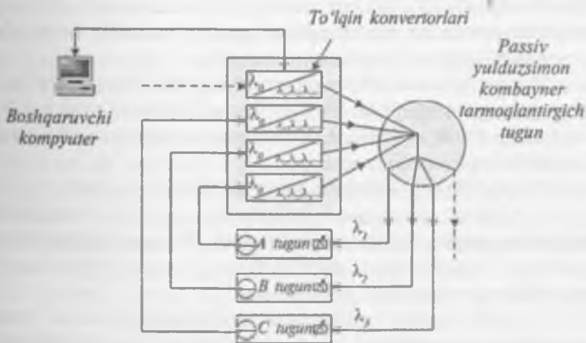
12.7-rasm. Kanallar kommutatsiyasi bo'lgan optik tarmoq: tarmoqning markaziy bo'g'ini to'lqin konverterlari asosida bajarilgan
