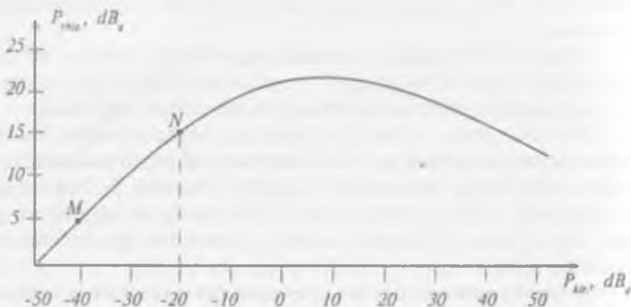
5.4-rasm. Aralashmali tolali optik kuchaytirgichning amplitudaviy xarakteristikasi
