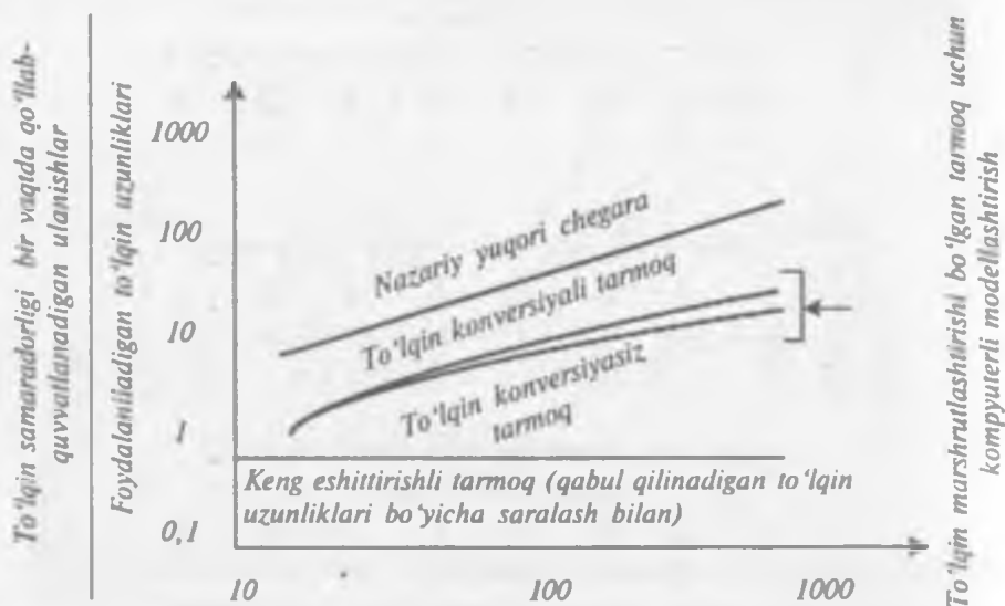
12.6-rasm. Optik tarmoq kanallar kommutatsiyasi bilan. Keng eshittirishli optik tarmoqlarni taqqoslash va to'lqin marshrutlashtirishi bo'lgan optik tarmoq
