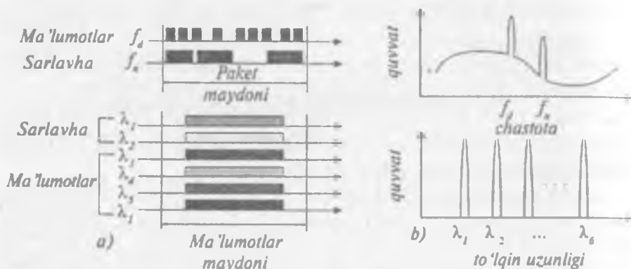
12.9-rasm. Tarmoqlarda paketning tuzilmasi:
