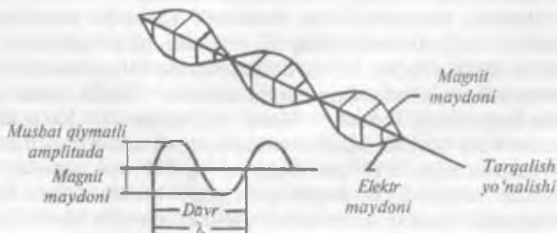
1.1-rasm. Elektromagnit to'lqin
