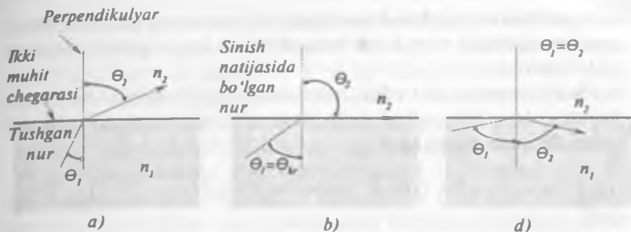
2.11-rasm. Bir necha tushish burchaklari uchun nurning tarqalish yo'lli, n_1 > n_2 , bunda n_1 va n_2 ikki xilli muhitlarning sindirish ko'rsatkichlari
