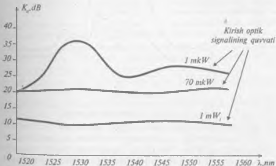
5.5-rasm. Erbiy aralashmali tolali optik kuchaytirgich kuchaytirish ko'effitsiyentining optik signal to'lqin uzunligiga bog'liqligi
