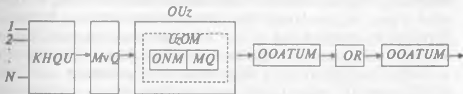
a) a — OOAT uzatish traktining tuzilish sxemasi
