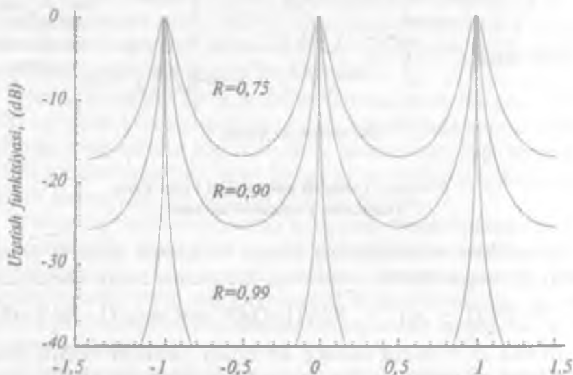
8.2-rasm. Fabri-Pero rezonatorli filtrning uzatish funksiyasi
