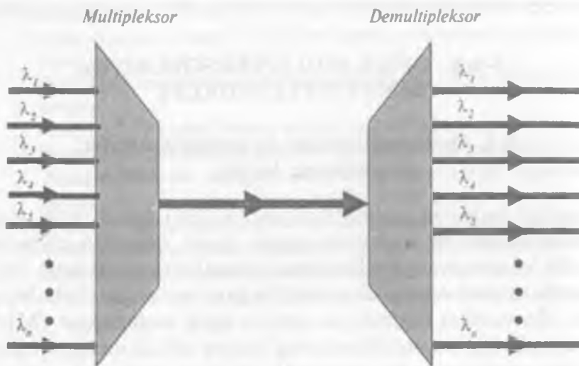
9.1-rasm. Spektr bo'yicha zichlashtirilgan tolali optik aloqa tizimlarida multiplekslash va demultiplekslash jarayonlari
