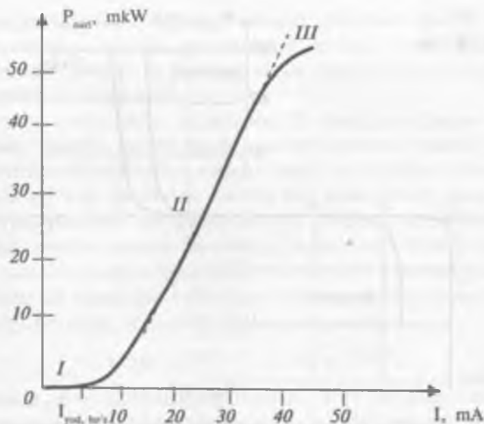
3.4-rasm. Yorug'lik diodining vatt-ampere xarakteristikasi
