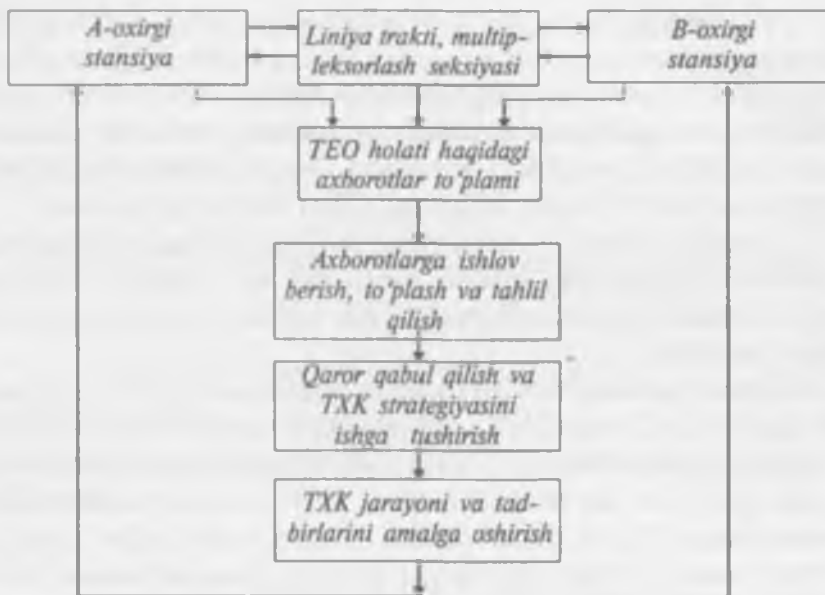
13.3-rasm. To'g'rilovchi texnik xizmat ko'rsatishning umumiy sxemasi
