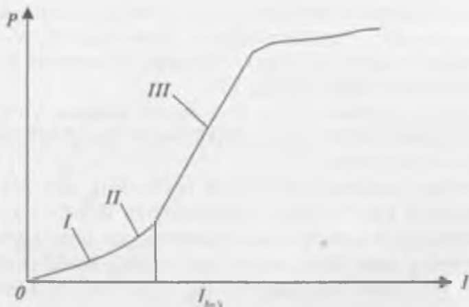
3.14-rasm. Yarimo'tkazgichli injeksion lazerning vatt-amper xarakteristikasi
