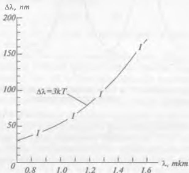
3.6-rasm. Yorug'lik diodi spektral diapazoni \Delta\lambda ning kengligi va to'liq uzunligi \lambda orasidagi bog'lanish (uzluksiz chiziq (3.8) munosabat bo'yicha hisoblash yo'li bilan olingan natijalarni ifodalaydi)
