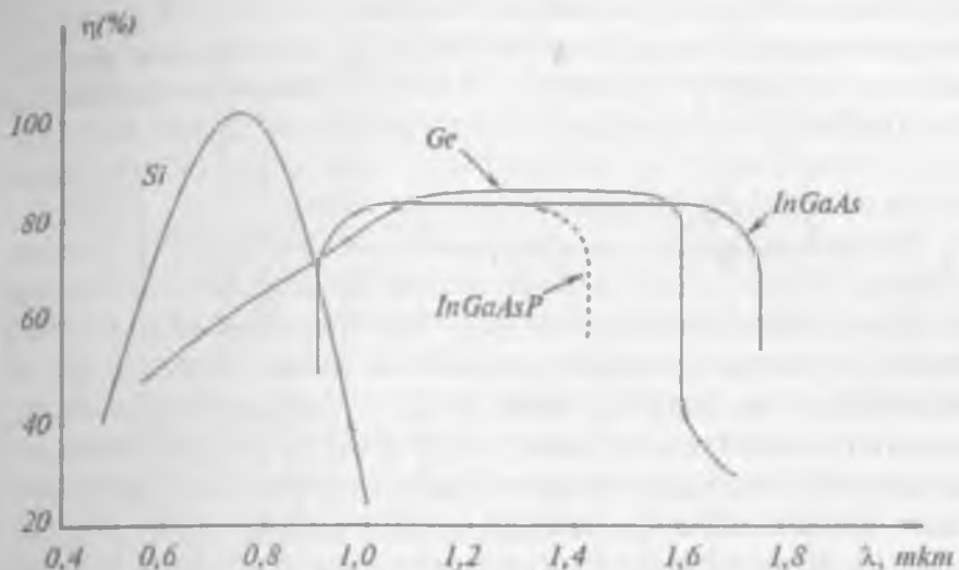
4.15-rasm. Yarimo'tkazgichlarning kvant samaradorligi va to'liqin uzunligi orasidagi bog'lanish grafigi
