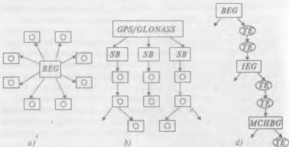
1.13-rasm. Taktli tarmoq sinxronizatsiyasini tuzish usullari: bir sathli yulduzcha sxemasi (a), bir sathli taqsimlangan sxema (b), iyerarxik ko'p sathli sxema (d)
