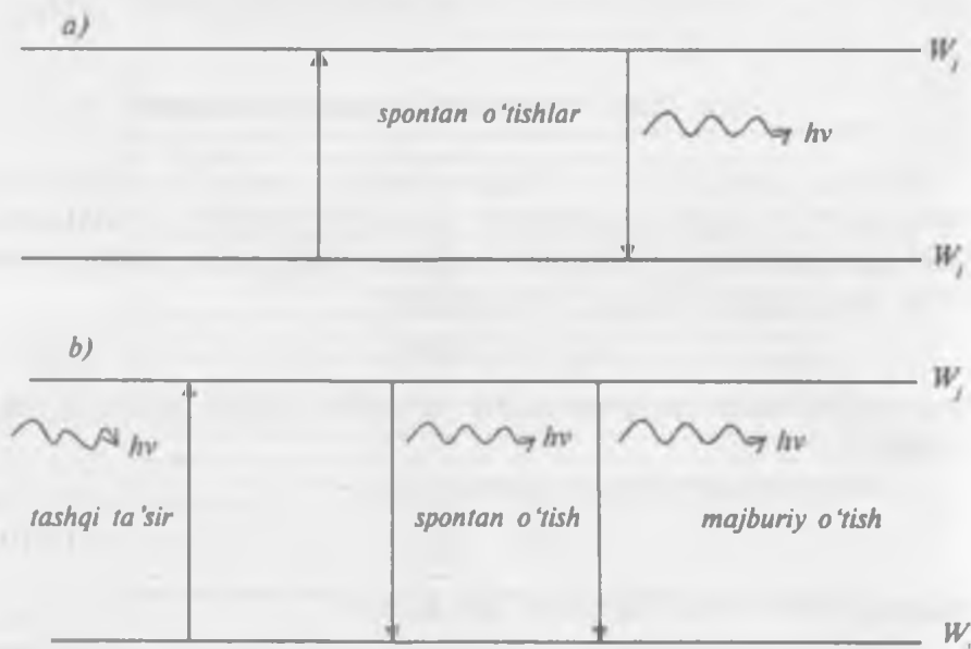
3.12-rasm. Spontan va majburiy o'tishlar
