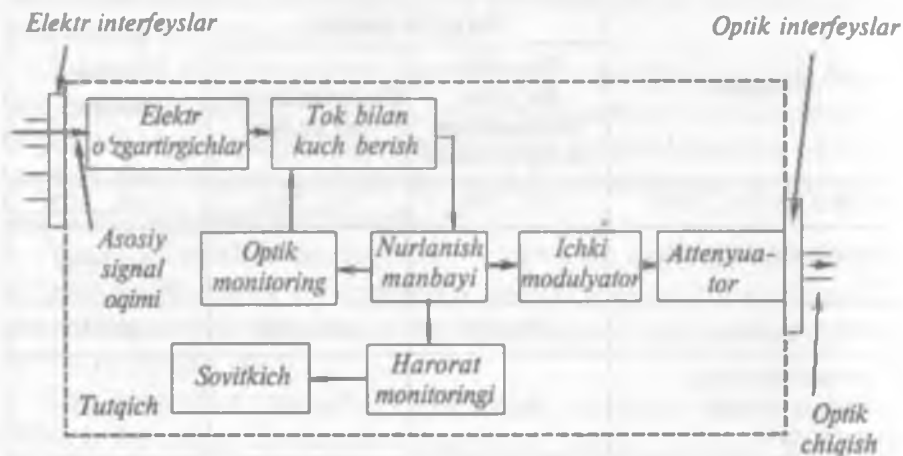
3.26-rasm. Optoelektron uzatuvchi modulning tuzilish sxemasi va tarkibiy elementlari
