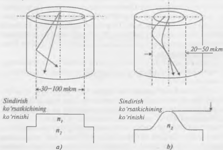
2.4-rasm. Pog'onali (a) va gradiyentli (b) ko'p modali optik tolalarning tuzilishi va sindirish ko'rsatkichi ko'rinishlari
