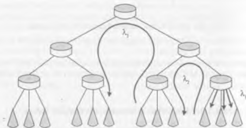
12.4-rasm. Kanallar kommutatsiyali optik tarmoq arxitekturasiga misol
