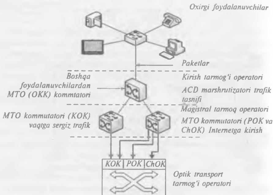
12.11-rasm. Multiservis foton tarmog'i foydalanuvchilari
