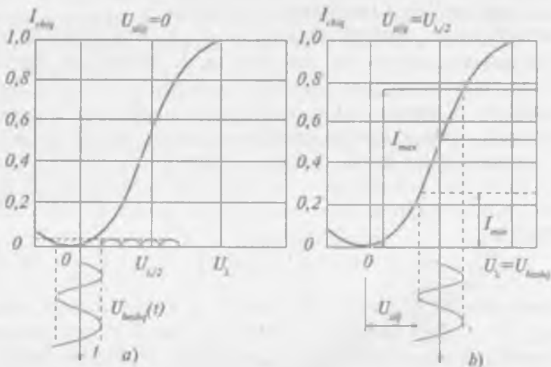
6.6-rasm. Elektrooptik modulyatorning boshqarish xarakteristikalari:
