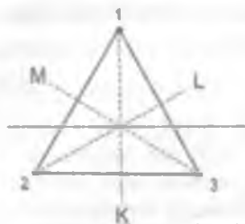
IV.1-rasm: Uch atomli molekula
