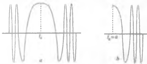
III 5-rasin f'(t_0) = 0 holdagi integral ostidagi ifodaga t_0 nuqta atrofida mos keluvchi grafik
