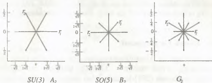
IV.9-rasm: Ikkinchi rang gruppalarining ildiz diagrammalari
