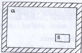
3-chizma. A-termostat; B-termostat ichida joylashgan tekshiriluvchi tizim.
