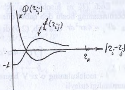
7-chizma. O'zaro ta'sir potentsial energiyasi \phi(r_{ij}) va f(r_{ij}) -funktsiyalarining zarralar orasidagi masofaga bog'liqligi
