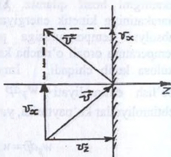
6-chizma. \vec{v} tezlikka ega bo'lgan zarraning proektsiyalari v_x = v_z . v_y = v_y , v_z = -v_z
