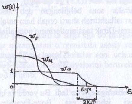
9-chizma. Kvant va klassik taqsimot funksiyalarining shartli grafigi
