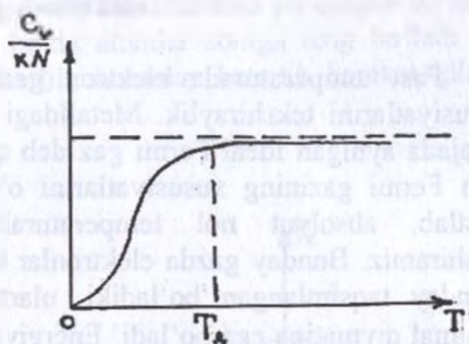
11-chizma. Kristallik panjara issiqlik sig'iminin temperaturaga bog'liqlik grafigi
