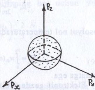
12b-chizma. Absolyut nol temperaturalarda barcha elektronlar joylashgan Fermi-sfera
