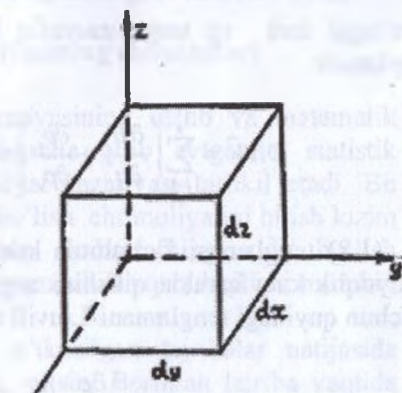
1-chizma. Uch o'lchamli Dekart koordinat sistemasi uchun dV = dx dy dz
