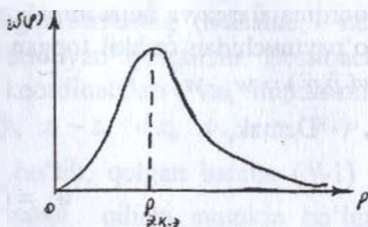
4-chizma. Impulsning absolyut qiymati bo'yicha Maksvell taqsimotining impulsiga bog'liqlik grafigi
