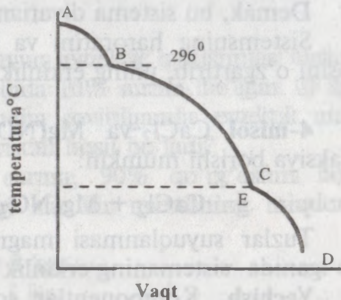
4.3-rasm. Tarkibida 8% surma bor qotishmaning sovish diagrammasi.
