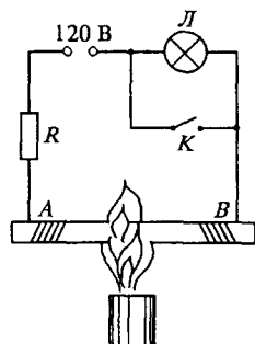
Рис. 106. Демонстрация электропроводности стекла при нагревании
