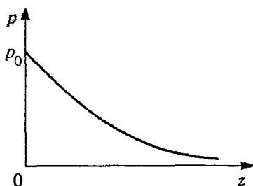
Рис. 71. Зависимость давления газа
