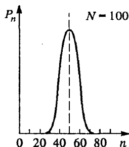
Рис. 78. Та же вероятность в случае, когда сосуд содержит 100 моле-
