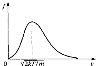
Рис. 74. График максвелловского распределения молекул газа по скоростям
