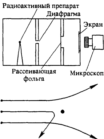
Рис. 24. Схема опытов Резерфорда
