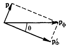
Рис. 18. К объяснению эффекта Комптона.
