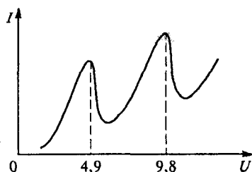
Рис. 105. Зависимость тока от ускоряющего напряжения в опытах
