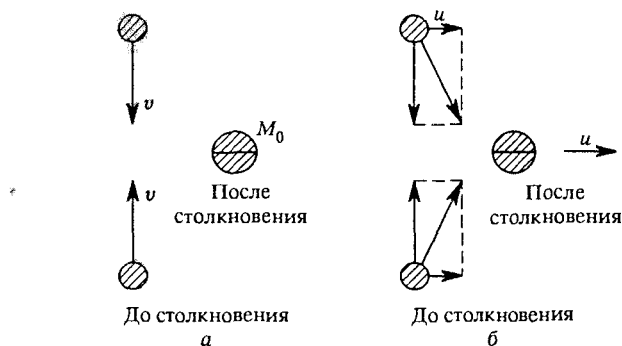
Рис. 11. Неупругое столкновение, наблюдаемое в разных системах отсчета
