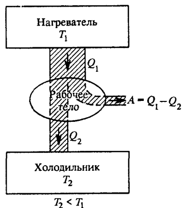
Рис. 53. Принципиальная схема тепловой машины
