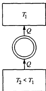
Рис. 56. Принципиальная схема гипотетического устройства, в котором нарушается постулат Клаузиуса
