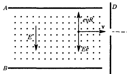
Рис. 29. Схема фильтра скоростей заряженных частиц
