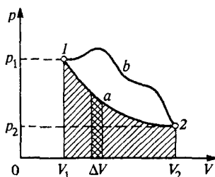
Рис. 50. p - V -диаграмма идеального газа
