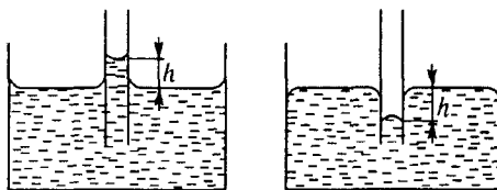
Рис. 84. Жидкость в капиллярах
