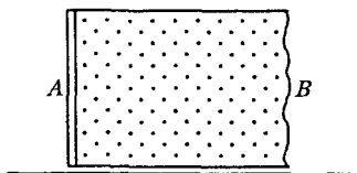
Рис. 69. Стенки сосуда A и B разные: удар молекул о стенку A абсолютно упругий, о стенку B — неупругий
