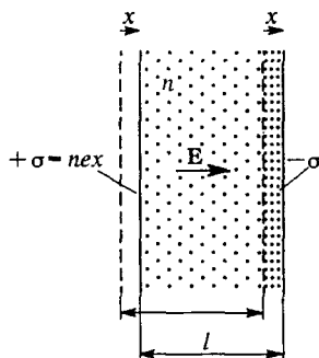
Рис. 108. К выводу формулы для частоты плазменных колебаний
