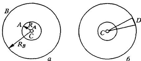
Рис. 76 Схема опытов Штерна
