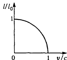
Рис. 6. Зависимость сокращения длины от относительной скорости
