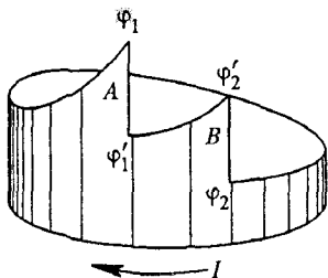
Рис. 107. Распределение потенциала вдоль цепи, содержащей химический элемент
