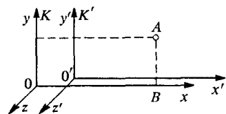
Рис. 7. Координаты одного и того же события A в двух системах отсчета
