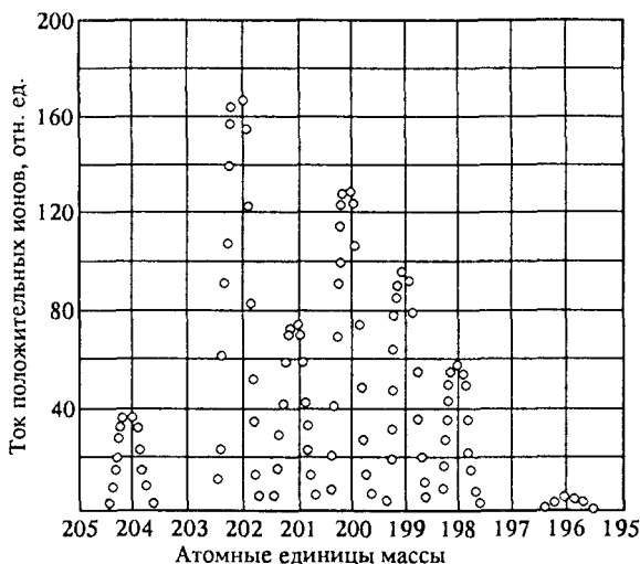
Рис. 32. Спектр масс изотопов ртути
