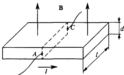
Рис. 118. К объяснению эффекта Холла
