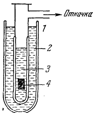
Рис. 5.4. Типичное устройство из двух сосудов Дьюара для работы вблизи 1°K. Дьюар, наполненный жидким гелием, помещен в другой дьюар, наполненный жидким азотом. Такое устройство уменьшает проникновение тепла в жидкий гелий. 1 — окружающая среда при 295°K, 2 — жидкий азот при 77°K, 3 — жидкий гелий при 4,2°K, 1 атм, 4 — охлажденный образец при низкой температуре.
