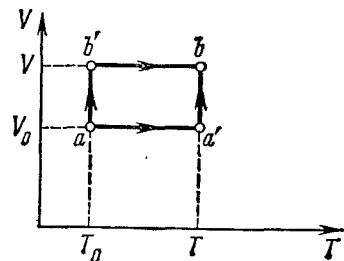
Рис. 7.5. Два различных квазистатических процесса, переводящие систему из начального макросостояния a (температура T_0 , объем V_0 ) в конечное макросостояние b (температура T , объем V ).
