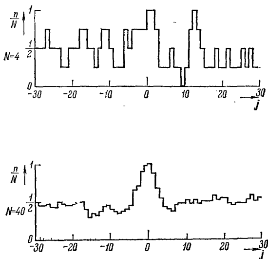
Рис. 1.20. Относительное число n/N частиц в левой половине ящика в зависимости от номера кадра j или времени t=j\tau_0 . Эти графики содержат ту же информацию, что и рис. 1.19
