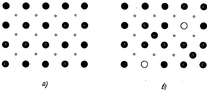
Рис. 1.15. а) Все атомы твердого тела (черные кружки) находятся в своих нормальных положениях, а возможные промежуточные положения (белые точки) не заняты. б) При более высоких температурах часть промежуточных положений может быть занята, как показано на рисунке.
