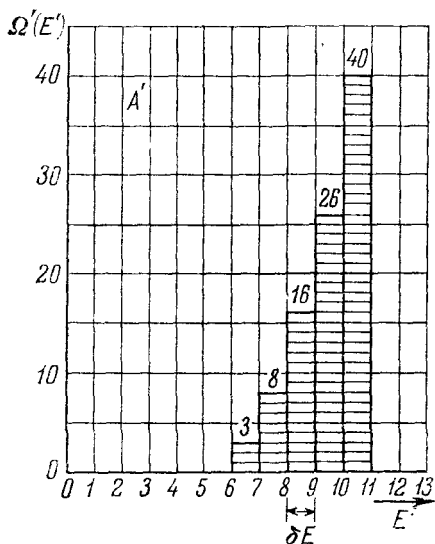
Рис. 4.1. На графиках показано (для частного случая двух очень малых систем A и A' ) числа состояний \Omega(E) и \Omega'(E') , доступных системам A и A' , в зависимости от энергии систем E и E' соответственно. Энергии измерены в произвольных единицах.
