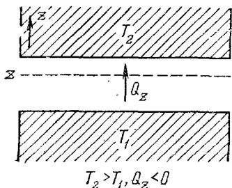
Рис. 36. Вещество, находящееся в тепловом контакте с двумя телами, абсолютная температура которых равна T_1 и T_2 . Если T_2 > T_1 , тепло течет в направлении -z , от тела с большей температурой к телу с меньшей температурой, таким образом, величина Q_z отрицательна.
