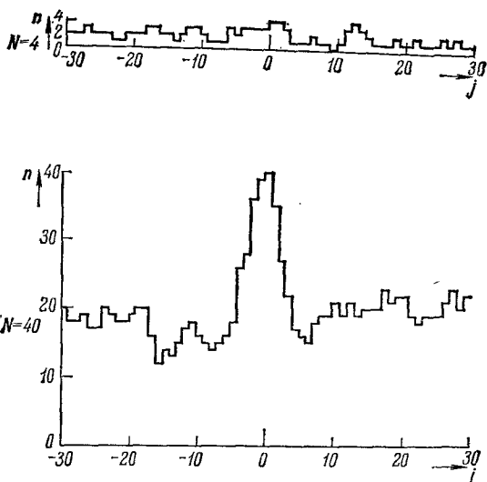
Рис. 1.19. Число n частиц в левой половине ящика в зависимости от номера кадра j или от времени t=j\tau_0 . Число частиц n на j -м кадре указано горизонтальной чертой, идущей от j до j+1 . Графики иллюстрируют рис. 1.15 и 1.16 для N=4 и рис. 1.17 и 1.18 для N=40 частиц, но содержат информацию о большем числе кадров, чем показано на этих рисунках. Правая половина каждого рисунка показывает приближение системы к равновесию. Весь рисунок иллюстрирует возникновение редкой флуктуации, возможной в состоянии равновесия.
