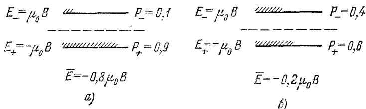
Рис. 3.12. Влияние теплового взаимодействия на весьма простую систему A , состоящую из единственного спина 1/2 с магнитным моментом \mu_0 , помещенного в магнитное поле B . На диаграмме показаны два возможных уровня энергии системы A . Этим двум квантовым состояниям соответствуют энергии E_+ и E_- . Вероятность обнаружить A в соответствующих состояниях обозначена через P_+ и P_- , и величина этих вероятностей пропорциональна заштрихованной части горизонтальных линий. Уровни энергии остаются неизменными, если внешнее магнитное поле (единственный внешний параметр системы) фиксировано. Начальное равновесное состояние (а) соответствует спину, помещенному в некое твердое тело. Твердое тело затем помещается в жидкость, и мы ждем наступления конечного равновесного состояния (б). В этом процессе спин системы A поглощает тепло от системы A' , состоящей из твердого тела и жидкости. При указанных на диаграмме изменениях вероятности тепло Q , поглощенное системой A , равно Q = 0,6 \mu_0 B .
