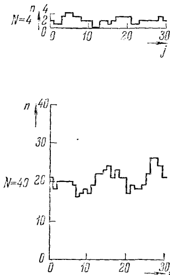
Рис. 1.5. Число n частиц в левой половине ящика в зависимости от номера кадра j или текущего времени t = jt_0 . Число частиц на кадре представлено горизонтальной чертой, простирающейся от j до j+1 . Графики иллюстрируют рис. 1.3 для N=4 и рис. 1.4 для N=40 , но содержат информацию о большем числе кадров, чем показано на этих рисунках.
