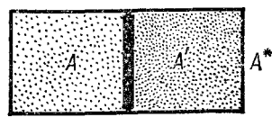
Рис. 3.10. Два газа, A и A' , разделенные подвижной перегородкой. Объединенная система A^* состоит из двух систем, A и A' , и является изолированной.
