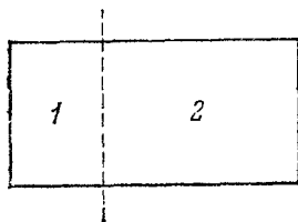
Рис. 5.1а Разделение однородной макроскопической системы на две части
