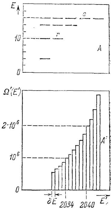
Рис. 4.6. Схема доступных состояний некоторой системы A и специального (очень маленького) теплового резервуара A' . На верхней части рисунка показаны уровни энергии для нескольких состояний системы A , на нижней — число доступных состояний \Omega'(E') системы A' в зависимости от ее энергии E' . Энергия измерена в произвольных единицах.
