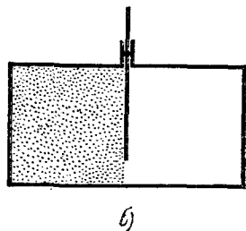
Рис. 1.13. Перегородка неожиданно поднята, но не до конца.
