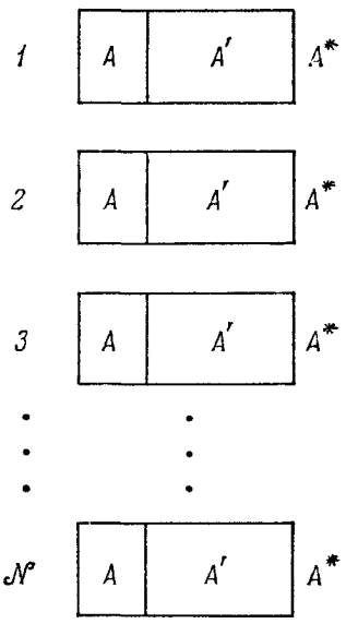
Рис. 3.11. Ансамбль систем A^* . Каждая система A^* состоит из двух систем, A и A' , которые могут взаимодействовать друг с другом.
