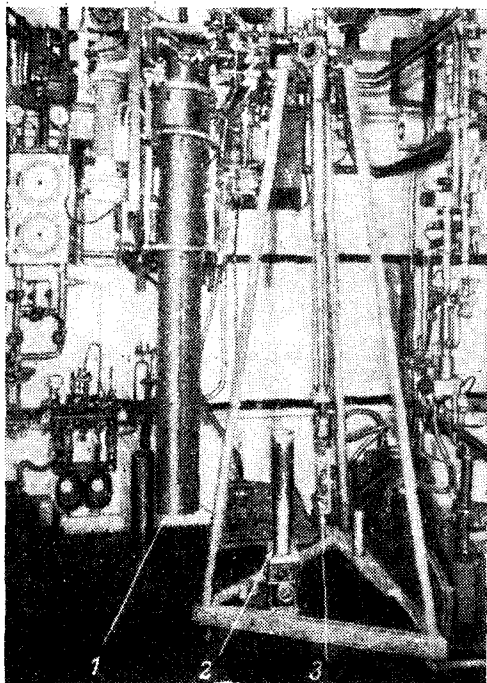
Рис. 5.14. Фотография всей аппаратуры для измерения удельной теплоемкости вблизи 0,1^\circ\text{K} . Внутренняя часть прибора (на рис. 5.13 она показана в увеличенном виде) здесь подвешена на треножке, сделанном из труб нержавеющей стали, через которые происходит откачка системы и проходят электрические провода. Откачиваемый сосуд при измерениях окружает внутреннюю часть прибора; на рисунке он показан отдельно. Для измерений весь прибор погружается в сосуд Дьюара, показанный слева. 1 — устройство с сосудом Дьюара, 2 — оболочка, 3 — внутренняя часть аппаратуры.
