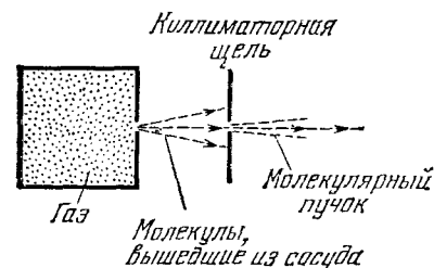
Рис. 1.37. Сосуд, наполненный газом, имеет очень маленькое отверстие, через которое молекулы могут выходить в окружающий вакуум. С помощью одной или нескольких коллимирующих щелей можно выделить молекулярный пучок. Распределение молекул по скорости в пучке определяется распределением в сосуде. Метод молекулярного пучка позволяет изучать поведение изолированных атомов или молекул. Его очень часто используют в современных физических экспериментах.
