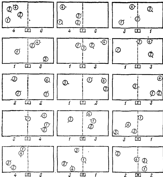
Рис. 1.16. Кадры, полученные с помощью электронной вычислительной машины, показывают положения четырех частиц в ящике. Началом этой последовательности кадров является специальный случай, когда частицы находятся в левой половине ящика и имеют некоторые произвольно заданные скорости (кадр j=0 ). Эволюция системы во времени показана последовательностью кадров j=0, 1, 2, \dots, 14 . Число частиц в каждой половине ящика записано непосредственно под кадром. Короткая черточка у каждой частицы показывает направление ее скорости.
