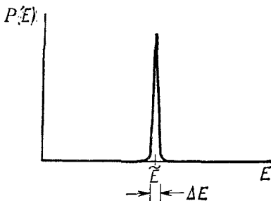
Рис. 4.2. Характер зависимости вероятности P(E) от энергии E .
