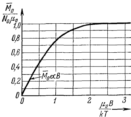
Рис. 4.10. Зависимость намагниченности \bar{M}_0 от магнитного поля B и температуры T в случае слабо взаимодействующего атома со спином 1/2 и магнитным моментом \mu_0 .
