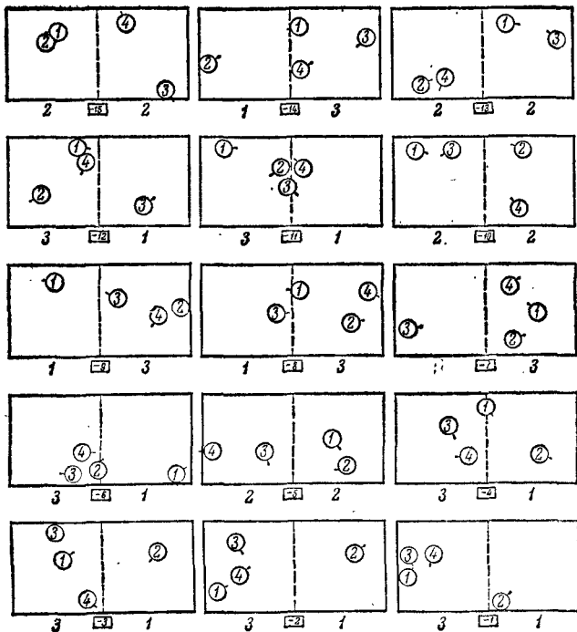
Рис. 1.15. Здесь показана возможная предыстория событий, рассматриваемых на рис. 1.16. Рисунки получены из исходного кадра j=0 (см. рис. 1.16), на котором скорости всех четырех частиц (находящихся в левой половине ящика) изменены на обратные. Эволюция системы во времени представлена последовательностью кадров j = -1, -2, \dots, -15 . Короткая черточка у каждой частицы показывает направление ее скорости. Если теперь представить себе, что скорости всех частиц на этом рисунке изменены на противоположные, то последовательность кадров j = -15, -14, \dots, -1, 0, 1, \dots, 14 (т. е. кадры на рис. 1.15 и 1.16) представляет собой возможное движение частиц.
