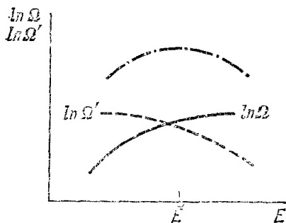
Рис. 4.3. Зависимость \ln \Omega(E) и \ln \Omega'(E') \equiv \ln \Omega'(E^* - E) от энергии E . Из (3.38) следует, что \ln \Omega(E) \sim f \ln(E - E_0) + \text{const.} Обе кривые обращены выпуклостью вверх и их сумма (показанная штрих-пунктирной линией) имеет единственный максимум при некотором значении \tilde{E} . Широкий максимум для медленно меняющегося логарифма P(\tilde{E}) в формуле (6) соответствует крайне резкому максимуму самой величины P(E) .
