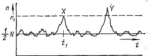
Рис. 1.8. Диаграмма, показывающая редко возникающие большие флуктуации числа молекул n в одной половине сосуда относительно равновесного значения \frac{1}{2}N .
