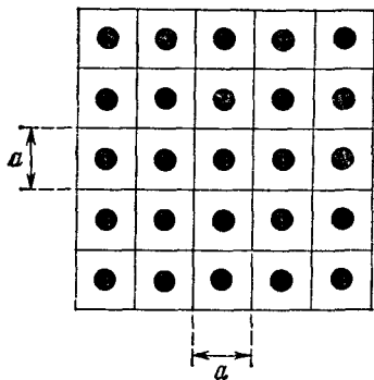
Рис. 6.14. Поверхность твердого тела, поверхность которого образуют простую кубическую решетку.
