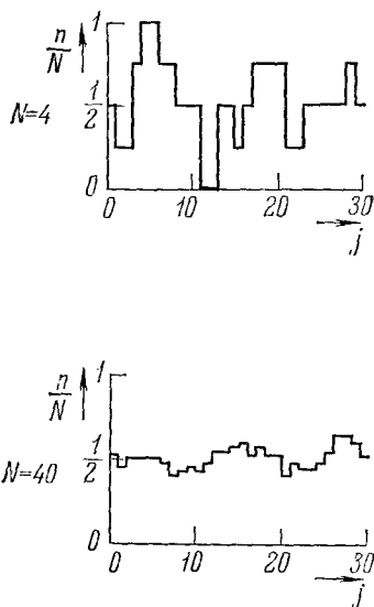
Рис. 1.6. Относительное число n/N частиц в левой половине ящика в зависимости от номера кадра j или текущего времени t = jt_0 . Эти графики содержат ту же информацию, что и рис. 1.5
