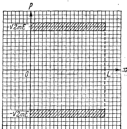
Рис. 6.3. Классическое фазовое пространство частицы, движущейся в одном измерении в ящике длиной L . Состояние частицы характеризуется координатой x и импульсом p ; ее энергия лежит между E и E+\delta E . Состояния, доступные частице, соответствуют ячейкам, находящимся в заштрихованных областях.
