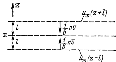
Рис. 8.5. Молекулы, пересекающие плоскость, осуществляют перенос импульса.
