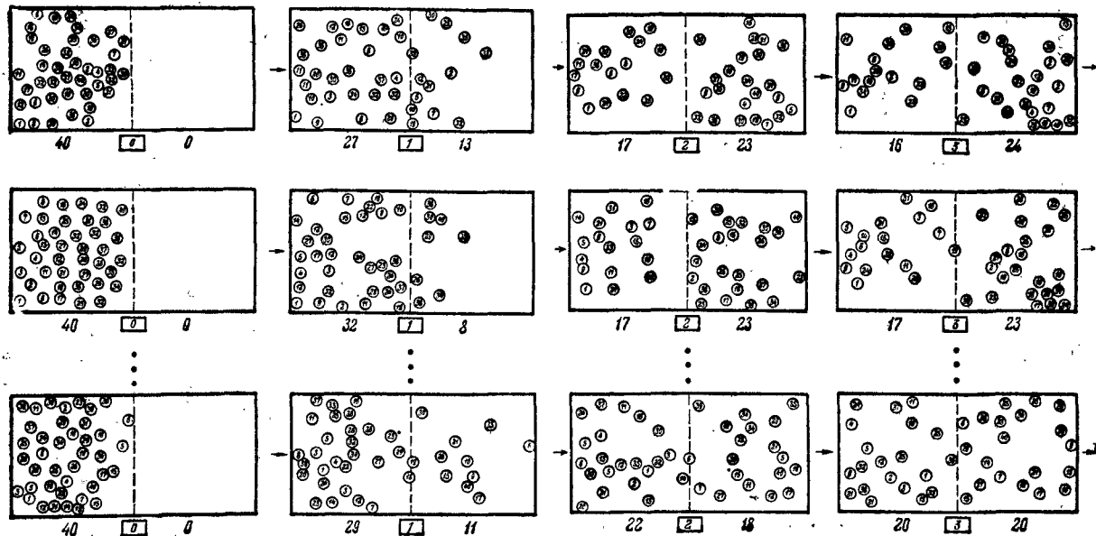
Рис. 2.3. Полученные с помощью вычислительной машины рисунки образуют статистический ансамбль систем. Этот ансамбль должен отразить поведение системы, состоящей из 40 частиц, заключенных в ящик. Доступная нам информация о системе заключается в следующем: в начальный момент времени (кадр j=0 ) все частицы находятся в левой половине ящика, но ничего больше об их положении и скорости мы не знаем. Чтобы проследить эволюцию во времени k -й системы ансамбля, нужно рассмотреть горизонтально расположенные в k -м ряду кадры j=0, 1, 2, \dots . Чтобы высказать какие-нибудь статистические утверждения о системе в момент времени, отвечающий j -му кадру, необходимо рассмотреть расположенные по вертикали j -е кадры и произвести счет числа систем, необходимый для определения вероятности.
