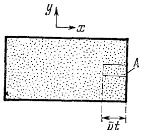
Рис. 1.34. Этот рисунок иллюстрирует столкновение молекул газа с площадкой A на одной из стенок сосуда. (Ось z перпендикулярна к плоскости чертежа.)
