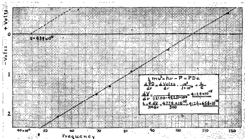
Рис. 44В. График из работы: Millikan R. A. — Phys. Rev., 1916, v. 7, p. 355, показывающий линейную зависимость критического значения задерживающего потенциала от частоты света для fotocувствительной поверхности натрия. Внизу справа приведены вычисления отношения h/e , сделанные Милликаном по этому графику
