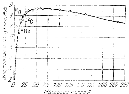
Рис. 33А. Зависимость энергии связи на нуклон \Delta(A, Z)c^2 от массового числа A . Точки отвечают определенным ядрам, часть которых указана на графике. В области легких ядер существуют нерасулярности, но при A > 25 экспериментальные точки хорошо ложатся на сплошную кривую. Энергия связи на один нуклон в среднем близка к 8 МэВ и при возрастании массового числа постепенно уменьшается. Это систематическое уменьшение происходит из-за увеличения электростатического отталкивания между протонами ядра.
