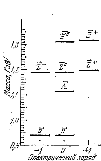
Рис. 27С. Спектр масс антибарионного октета, который образован античастицами октета, приведенного на рис. 27В. Все частицы антибарионного октета имеют барионное число -1 и спин, равный 1/2 . Отразив барийную диаграмму вокруг вертикали, проходящей через нуль заряда, получим антибарионную диаграмму, и наоборот
