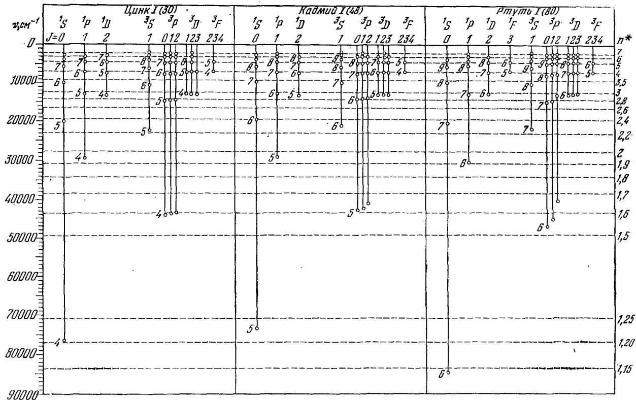
Рис. 35А. Схема уровней цинка, кадмия и ртути. Приведенные вместе, они показывают, что химически сходные элементы имеют аналогичные схемы уровней (из книги Гроттриана, см. рис. 28А)
