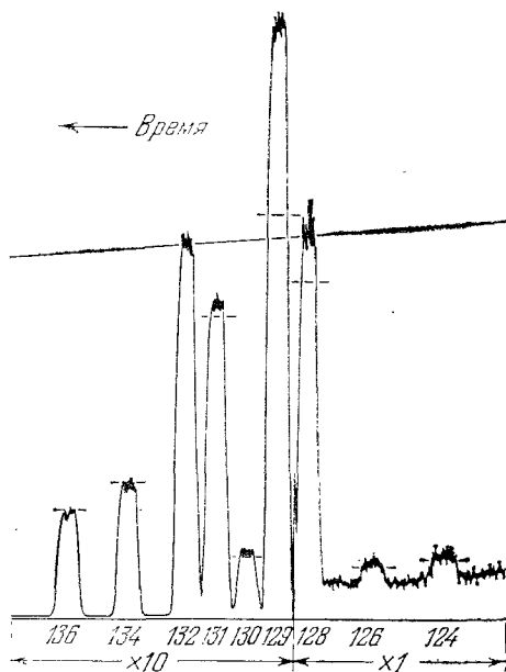
Рис. 34 В. Спектр масс, полученный с помощью прибора, показанного на рис. 34 А, для ксенона в метеоритах. Короткими горизонтальными линиями показана распространенность изотопов ксенона в земных образцах. Мы видим, что метеоритный ксенон обогащен изотопом ^{129}\text{Xe} . Заметим, что кривая распространенности изображена в двух различных вертикальных масштабах
