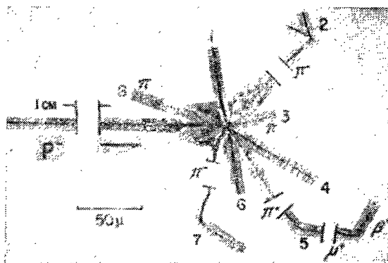
Рис. 29А. Звезда, возникшая от аннигиляции протона и антипротона в ядерной эмульсии. Этот рисунок является мозаикой из миксфотопрографий многих полей зрения, позволяющей увидеть следы различных частиц. Масштаб снимка показан в нижнем левом углу. У четырех следов слева пробег выброшен, чтобы придать рисунку удобные размеры. Горизонтальный след слева принадлежит антипротону. Перемещаясь в эмульсии, антипротон теряет энергию и замедляется. В конце концов он поглощается ядром эмульсии (по-видимому, ядром углерода) и аннигилирует с одним из протонов ядра. При этом рождается несколько пионов (следы 2, 3, 5, 7, 8) и ядро разваливается на осколки. Следы 1 и 3, вероятно, принадлежат протону, а след 6 — более тяжелой частице, возможно ядру ^3\text{H} . Сумма полной кинетической энергии видимых (заряженных) частиц и энергии покоя пионов на этом снимке близка к 1,3 ГэВ. След 5 принадлежит положительному пиону, который после остановки распадается на нейтрино (его след на снимке, конечно, не виден) и положительный мюон, в свою очередь распадающийся на позитрон и два нейтрино (Segrè E. Antinucleons.— Annual Rev. Nucl. Sci. 1958, } ч. 8, р. 127; эта работа является обзором ранних исследований антинуклонов)
