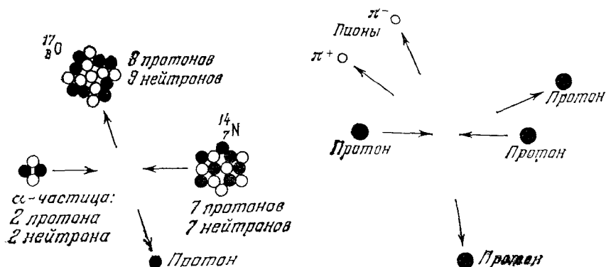
Рис. 11А. Схематическое представление ядерной реакции: α-частица (ядро гелия) сталкивается с ядром азота, в результате образуется ядро кислорода и протон. Именно эта реакция, открытая Резерфордом в 1919 г., была первым наблюдением превращения одних стабильных ядер в другие (Rutherford E. — Phil. Mag., 1919, v. 37). В опыте Резерфорда азот бомбардировался α-частицами радиоактивного источника, а реакция идентифицировалась по наблюдению испущенных протонов. Этот рисунок аналогичен рис. 9А и показывает, что ядра состоят из протонов и нейтронов, а ядерная реакция заключается (при малых энергиях) в перераспределении этих частиц между ядрами. Такой рисунок не следует понимать буквально: ядра «не похожи» на то, что показано на рисунке
