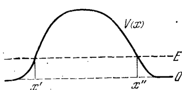
Рис. 35А. Как получить выражение для коэффициента пропускания такого барьера?
