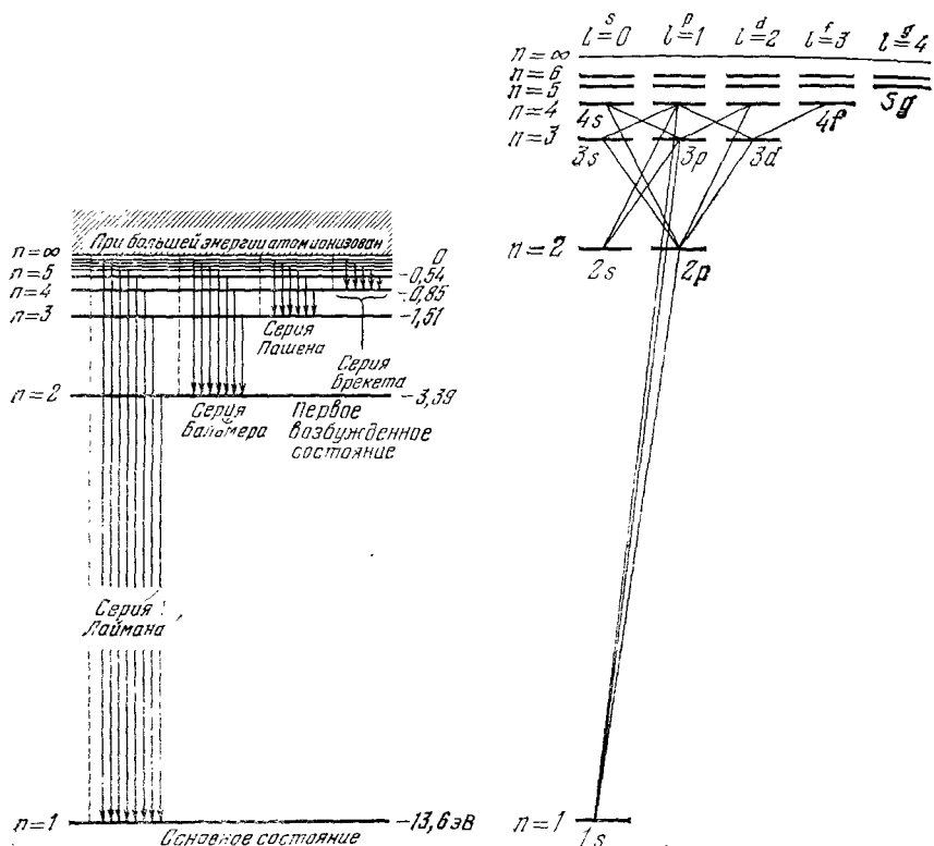
Рис. 45А. Схема уровней атома водорода. С очень хорошим приближением энергия E_n уровня с главным квантовым числом n равна E_n = -R_H/n^2 , где R_H = (1 + m/M_p)^{-1} R_\infty = 13,5976 эВ. Вертикальными линиями показаны возможные электрические дипольные переходы. Эти переходы группируются в четыре серии, названные именами известных спектроскопистов. Вся серия Лаймана лежит в ультрафиолетовой области; серия Бальмера — в видимой области. На рис. 1В гл. 3 показан спектр водорода, на котором видны некоторые линии серии Бальмера
