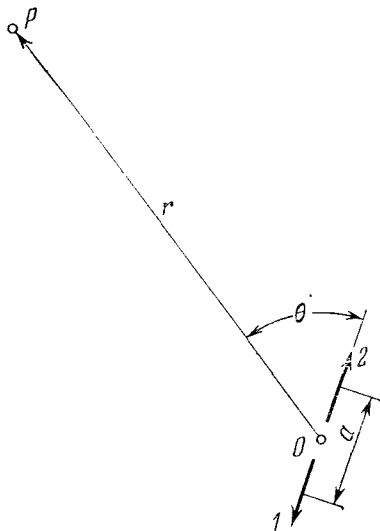
Рис. 50А. Схематическое изображение электрического квадрупольного излучения. Стрелки 1 и 2 соответствуют двум одинаковым электрическим диполям, осциллирующим с одинаковой частотой \omega и направленным в противоположные стороны. У такой системы нет ни электрического дипольного, ни магнитного дипольного момента, но имеется электрический квадрупольный момент. Если расстояние a мало по сравнению с длиной волны \lambda , то мощность излучения такого источника меньше мощности излучения диполя на множитель порядка (a/\lambda)^2 .
