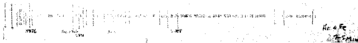
Рис. 5В. Спектр гелия (длинные линии), наложенный на спектр железа (короткие линии). На этой спектрограмме поражает сложность спектра железа по сравнению с простым спектром гелия
