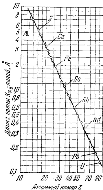
Рис. 37А. График зависимости \ln \lambda от \ln Z . Здесь \lambda — длина волны так называемой K\alpha_2 -линии рентгеновского
