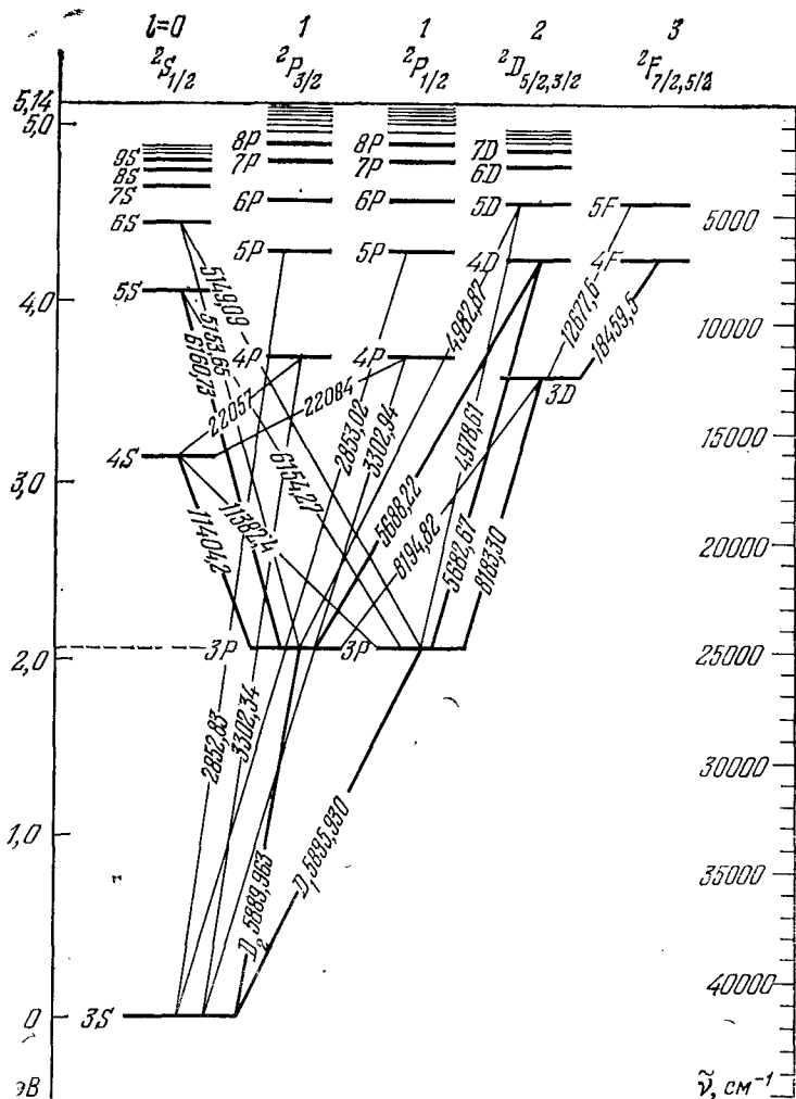
Рис. 32А. Схема уровней нейтрального атома натрия (из книги Гроттриана, см. рис. 28А;
