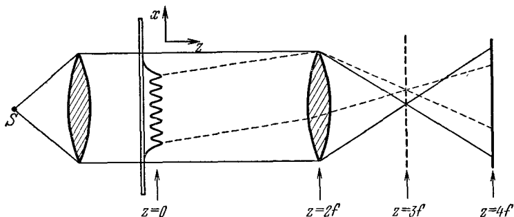
Рис. к задаче 9.56. Фазово-контрастный микроскоп.
