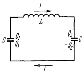
Рис. 1.5. Последовательное соединение самондукции L и емкостей C .
