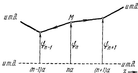
Рис. 2.11. Общая конфигурация нагруженной струны, совершающей поперечные колебания по оси x .
