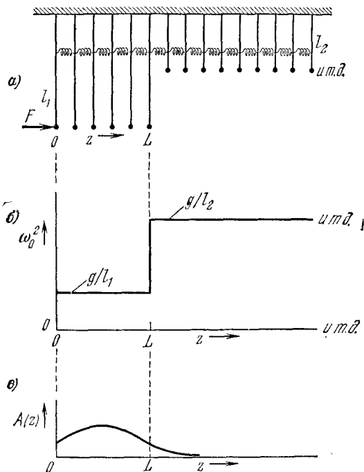
Рис. 3.12. Система связанных маятников с внезапным изменением \omega_0^2 в точке z=L .
