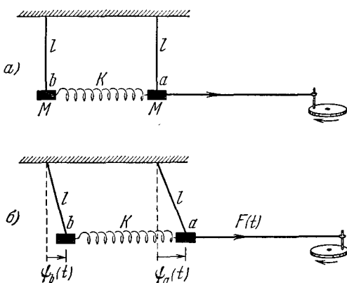
Рис. 3.3. Вынужденные колебания связанных маятников.
