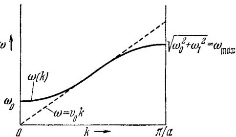
Рис. 2.18. Дисперсионное соотношение для связанных маятников.
