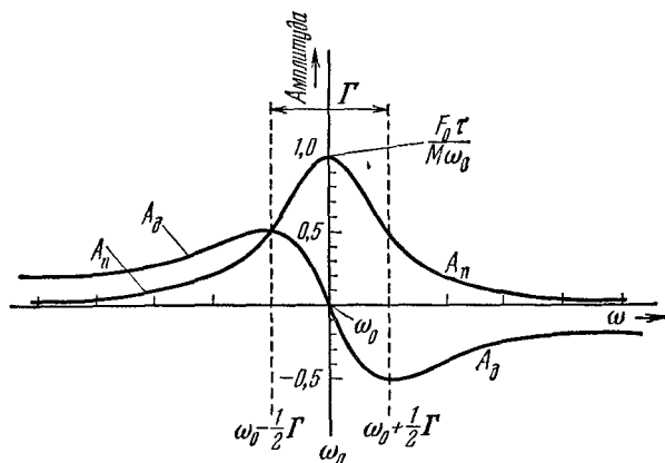
Рис. 3.1. Резонанс вынужденных колебаний. Если на осциллятор действует внешняя сила F_0 \cos \omega t , то в установившемся состоянии x_s(t) = A_n \sin \omega t + A_d \cos \omega t .
