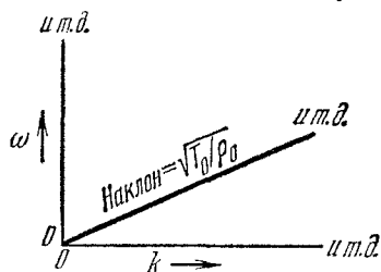
Рис. 2.4. Дисперсионное соотношение для непрерывной однородной струны.
