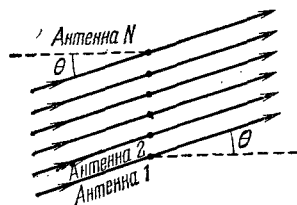
Рис. 9.17. Ряд антенн, возбуждаемых наклонно падающей волной.
