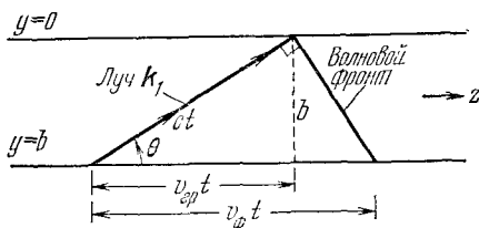
Рис. 7.2. Одна из бегущих волн в волноводе.
