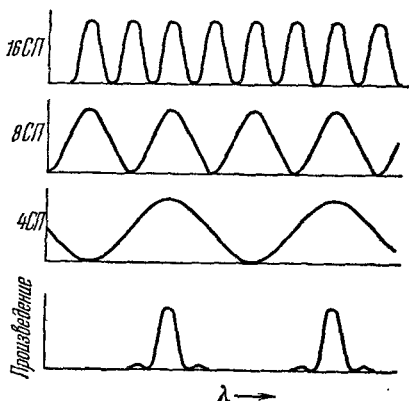
Рис. к задаче 8.17. Фильтр.
