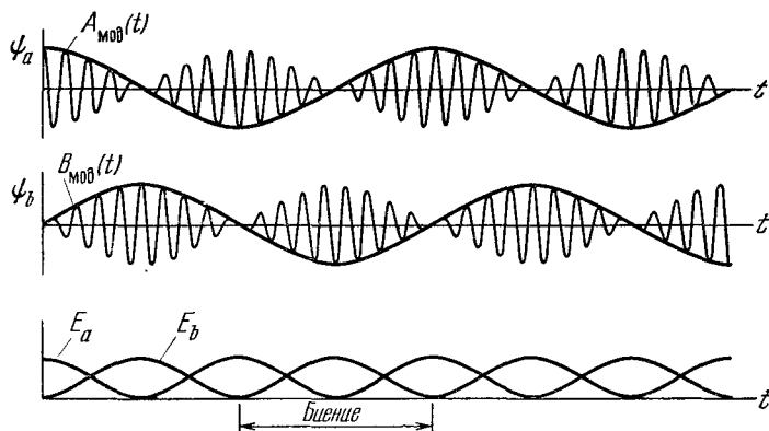
Рис. 1.15. Перемещение энергии между двумя слабо связанными одинаковыми маятниками. Энергия переходит от a к b и от b к a с частотой |v_1 - v_2| биений обоих мод.
