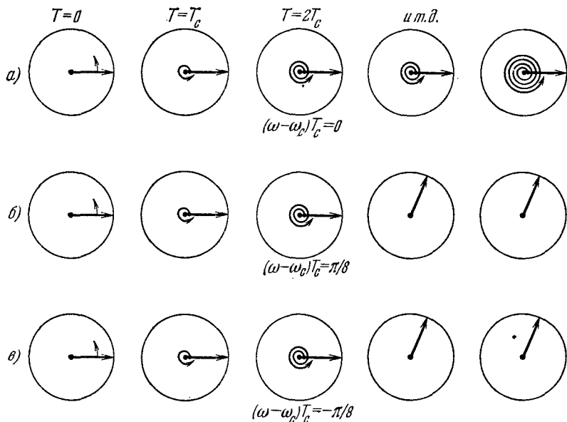
Рис. 6.2. Стробоскопические моментальные «снимки» вращающегося комплексного вектора \exp i\omega t .
