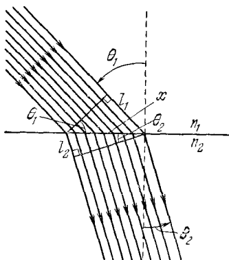
Рис. 4.7. Преломление.
