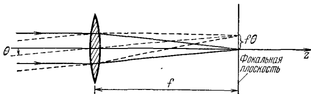
Рис. 9.27. Фокальная плоскость.
