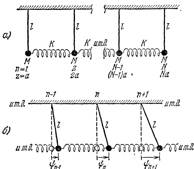
Рис. 2.17. Связанные маятники.
