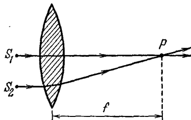
Рис. 9.3. Собирающая линза.
