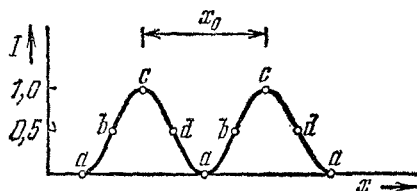
Рис. 9.7. Зависимость интенсивности от x в данный «момент» времени, продолжительность которого меньше (\Delta\nu)^{-1} .
