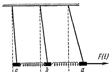
Рис. 3.7. Механический фильтр.
