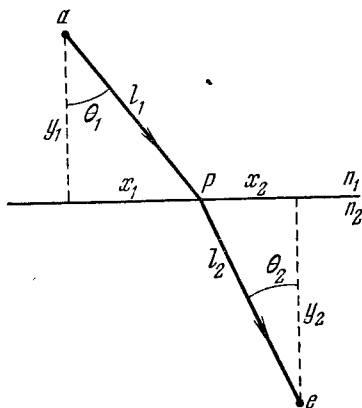
Рис. 9.21. Преломление.
