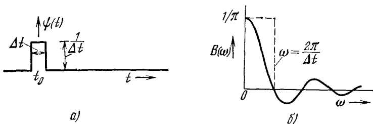
Рис. 6.10. Прямоугольный импульс \psi(t) и его фурье-коэффициент B(\omega) .
