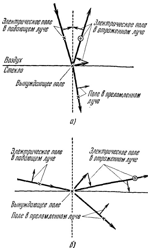
Рис. 8.8. Фазовые соотношения для света, отраженного от стекла. а) Угол \theta_1 меньше угла Брюстера; б) \theta_2 больше угла Брюстера. Кружками показана поляризация, перпендикулярная плоскости чертежа. Крест и точка означают, что вектор E направлен от нас или на нас соответственно. Стрелками показано направление E в плоскости рисунка.
