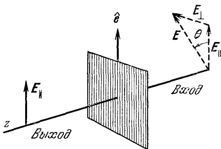
Рис. 8.5. Идеальный поляризатор.
