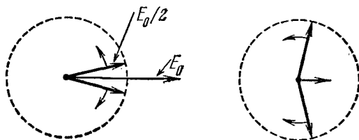
Рис. 8.12. Линейно-поляризованные колебания с амплитудой E_0 можно рассматривать как суперпозицию левой и правой круговой поляризации с амплитудами E_0/2 .
