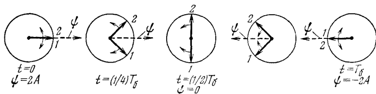
Рис. 6.3. Биение в суперпозиции \psi(t) = A \exp i\omega_1 t + A \exp i\omega_2 t . Стробоскопические «снимки» производятся с частотой \omega_{\text{с}} = \omega_{\text{ср}} и покрывают целый период биений T_\delta .
