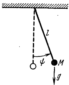
Рис. 1.2. Простой маятник.
