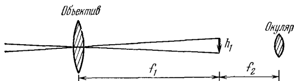
Рис. 9.32. Телескоп.
