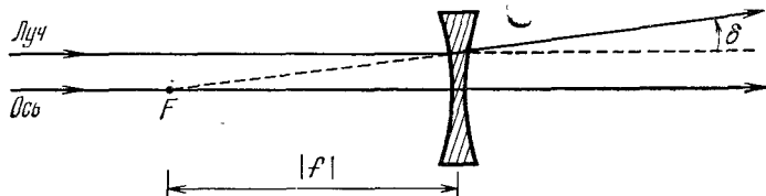
Рис. 9.30. Рассеивающая линза.
