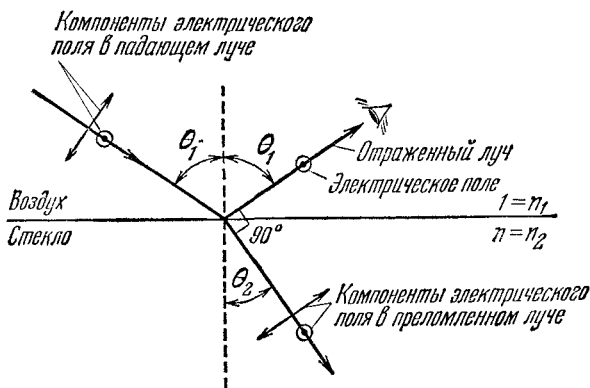
Рис. 8. 7. Угол Брюстера.
