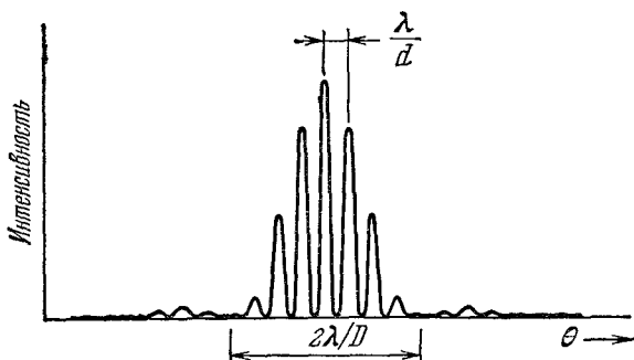
Рис. 9.15. Дифракция от двух щелей для случая, когда расстояние между щелями d в 4 раза больше ширины каждой щели.
