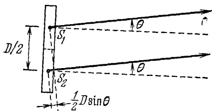
Рис. 9.11. Плоский излучатель.
