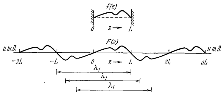
Рис. 2.5. Образование периодической функции F(z) с периодом \lambda_1=2L из функции f(z) , исчезающей на концах отрезка z=0 и z=L .
