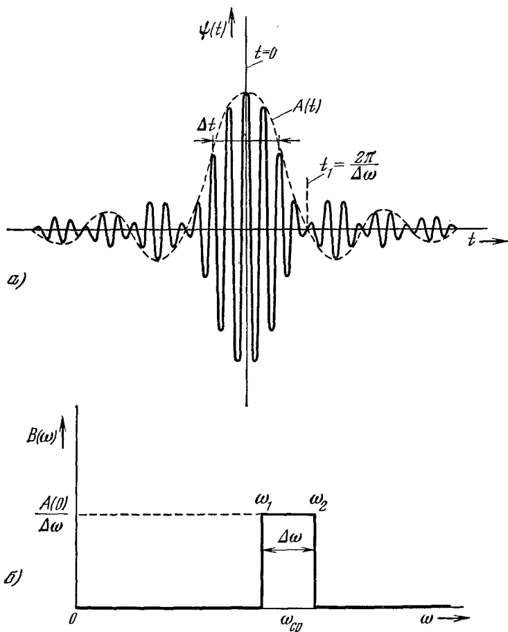
Рис. 6.6. Фурье-анализ непериодической функции.
