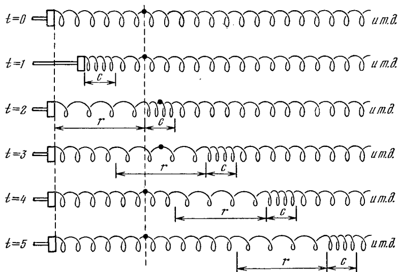
Рис. 4.2. Продольные бегущие волны сжатия (с) и разрежения (r) в пружине. Шестой виток спирали отмечен, что позволяет следить за его движением.
