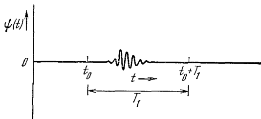
Рис. 6.8. Импульс \psi(t) .
