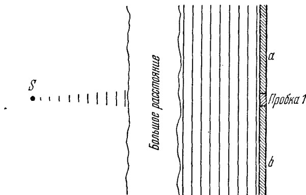
Рис. 9. 12. Плоские волны от далекого точечного источника падают на непрозрачный экран. Нулевая интенсивность за экраном является результатом суперпозиции полей от S и от частей экрана a и b и пробки 1 .
