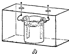
Рис. 4.8. Различные устройства, эквивалентные для постоянного тока сопротивлению 65 ом. а) Нихромовая проволока № 40 длиной 28 см. б) Катушка эмалированного медного провода № 28 для магнитов длиной 1030 футов (301,4 м) и весом 1/2 фунта (227 г). в) Два сопротивления по 70 ом и одно сопротивление 30 ом. г) Вольфрамовая лампа накаливания 25 вт, 115 в (холодная). д) 0,5 н-раствор KCl с электродами определенного размера на определенном расстоянии.
