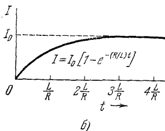
Рис. 7.24. а) Характер изменения тока в начале и через очень большой промежуток времени. б) Изменение тока во времени в контуре рис. 7.23.
