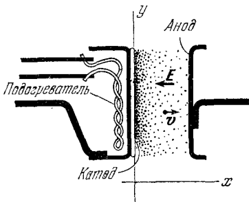
Рис. 4.2. Вакуумный диод с плоскопараллельными катодом и анодом.
