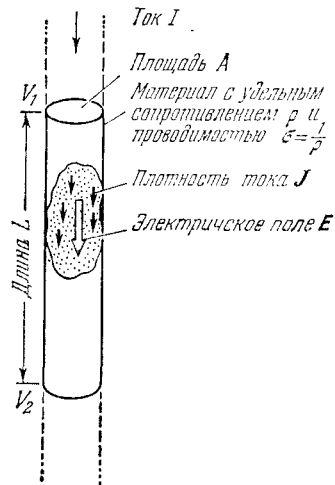
Рис. 4.3. Ток в проводнике. Соотношение J = \sigma E между плотностью тока J и электрическим полем E заключает в себе закон Ома: V = IR , I = AJ = A\sigma E , V = V_1 - V_2 = EL ,
