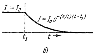
Рис. 7.25. а) Контур LR . б) Экспоненциальное спадание тока в контуре LR .
