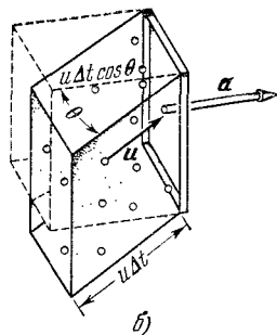
Рис. 4.1. а) Поток заряженных частиц, движущихся с одинаковой скоростью \mathbf{u} . Площадь рамки \mathbf{a} . В ближайшие \Delta t сек через рамку пройдут частицы, заключенные внутри косої призмы. б) Площадь основания призмы равна \mathbf{a} , высота u \Delta t \cos \theta , следовательно, объем призмы \mathbf{a} u \Delta t \cos \theta или \mathbf{a} \cdot \mathbf{u} \Delta t .
