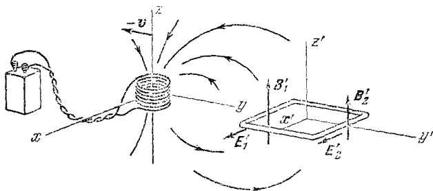
Рис. 7.14. Рамка неподвижна в системе координат F' , источник поля движется. Поля \mathbf{B}' и \mathbf{E}' меняются как в пространстве, так и во времени.
