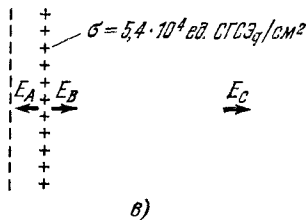
Рис. 9.21. а) Диск, состоящий из полярных молекул с дипольными моментами, направленными параллельно оси. б) Поперечное сечение диска. в) Поперечное сечение эквивалентных заряженных слоев.
