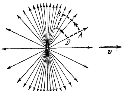
Рис. 5.13. Другое представление поля равномерно движущегося заряда.
