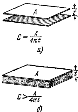
Рис. 9.1. а) Конденсатор, состоящий из параллельных проводящих пластин. б) Тот же конденсатор с изолирующим слоем между пластинами.
