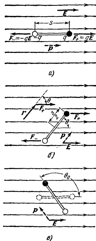
Рис. 9.7. а) Диполь в однородном поле. б) Вращающий момент, действующий на диполь, \mathbf{N} = \mathbf{p} \times \mathbf{E} ; \mathbf{N} — это вектор, направленный перпендикулярно к плоскости рисунка («от нас»). в) Работа, затраченная на поворот диполя из положения, параллельного полю, в положение, показанное на рисунке, равна pE(1 - \cos \theta_0) .
