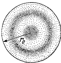
Рис. 1.18. Сферически симметричное распределение заряда.
