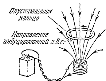
Рис. 7.12. Во время опускания кольца увеличивается поток сквозь кольцо, направленный вниз. Индуцированная э.д.с. будет, согласно закону Ленца, направлена по стрелкам, так как ток, текущий в этом направлении, создает поток, направленный вверх сквозь кольцо. Система противодействует происходящему изменению.
