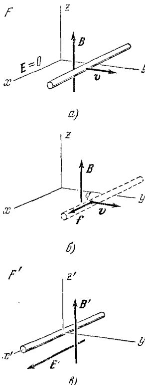
Рис. 7.2. а) Проводящий стержень движется в магнитном поле. б) На произвольный заряд q , движущийся вместе со стержнем, действует сила (q/c)\mathbf{v} \times \mathbf{B} . в) Система координат F' движется вместе со стержнем, электрическое поле в этой системе обозначено через \mathbf{E}' .
