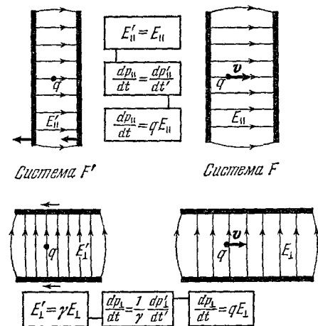
Рис. 5.19. В системе, где заряды, создающие поле \mathbf{E} , неподвижны, сила, действующая на движущийся с любой скоростью заряд q , равна просто q\mathbf{E} .
