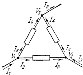
Рис. 4.14. Токи и потенциалы в узлах цепи.
