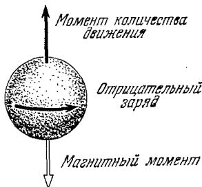
Рис. 10.14. Внутренний момент количества движения, \frac{h}{4\pi} = 0,5 \cdot 10^{-27} г·см 2 /сек (спин), и связанный с ним магнитный момент электрона, \frac{e\hbar}{4\pi mc} = 0,93 \cdot 10^{-20} эрг/гс.
