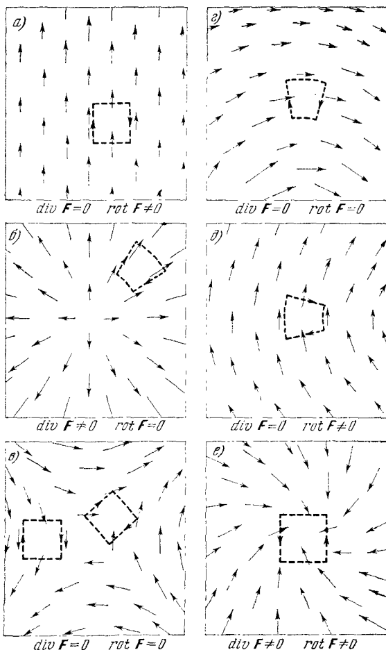
Рис. 2.33. Обсуждение рис. 2.32. а) Заметьте, что вектор остается постоянным, когда вы продвигаетесь в его направлении, т. е. \partial F/\partial y=0 , F_x=0 . Следовательно, \text{div } F=0 . Обратите внимание на то, что линейный интеграл вдоль штрихового контура не равен нулю. б) Поле является центральным. Это значит, что функция F радиальна и что для данного r ее величина постоянна. Ротор любого центрального поля равен нулю; циркуляция равна нулю вокруг пунктирного и любого другого контура. Но дивергенция, очевидно, не равна нулю. в) Циркуляция, очевидно, могла бы быть равна нулю вокруг изображенных контуров. Действительно, это то же самое возможное электростатическое поле, как на рис. 2.2. Из одного этого рисунка не очевидно, что \text{div } F=0 , но видно, что она также могла бы быть равна нулю. г) Заметьте, что, с точностью до первого порядка, здесь нет изменения в величине F , если вы продвигаетесь в направлении вектора F . Этого достаточно для того, чтобы дивергенция была равна нулю. Оказывается, что циркуляция могла бы быть равна нулю вокруг изображенного контура, так как F слабее на длинной стороне, чем на короткой. Действительно, это есть возможное электростатическое поле с F , пропорциональным 1/r , где r — расстояние до точки, расположенной вне чертежа. д) По той же причине, что и выше, мы приходим к заключению, что \text{div } F=0 . В данном примере величина F всюду одинакова, поэтому линейный интеграл по длинной стороне контура не уничтожается интегралом по короткому пути и циркуляция не равна нулю. е) Ясно, что циркуляция вокруг штрихового контура не равна нулю. Оказывается также, что и дивергенция не равна нулю, так как векторы сходятся к центру со всех сторон.
