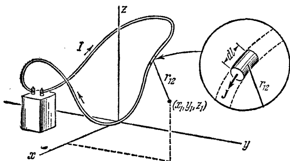
Рис. 6.12. Каждый элемент петли с током вносит вклад в векторный потенциал A в точке (x_1, y_1, z_1) .
