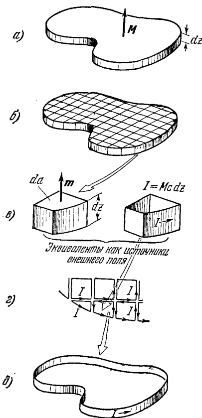
Рис. 10.16. Внешнее поле тонкой пластины, намагниченной перпендикулярно к ее широкой поверхности, эквивалентно внешнему полю ленты с током.
