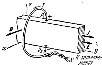
Рис. 6.29. Эффект Холла. Если проводник с током помещен в перпендикулярное к нему магнитное поле, то между точками, расположенными на противоположных сторонах бруска, возникает разность потенциалов. Если бы поля не было, эти точки имели бы одинаковые потенциалы. Это означает существование поля внутри бруска! Измеряя «потенциал Холла», можно определить число носителей заряда на кубический сантиметр и их знак.
