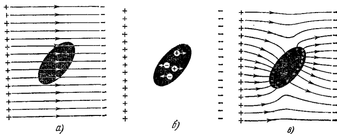
Рис. 3.1. Тело на рис. а является нейтральным и непроводящим. Положительные и отрицательные заряды, находящиеся в нем, неподвижны. На рис. б заряды свободны и начинают двигаться. Они будут продолжать движение до тех пор, пока не установится конечное состояние, изображенное на рис. в .
