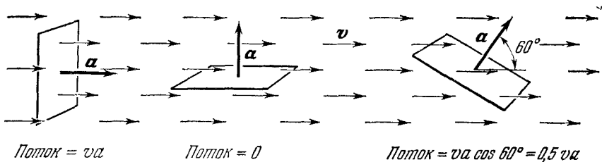
Рис. 1.14. Поток через рамку площадью a равен \mathbf{v} \cdot \mathbf{a} . Если \mathbf{v} — скорость жидкости, то поток равен объему жидкости, проходящей через рамку в единицу времени.
