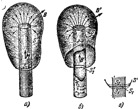
Рис. 10.18. а) Однородно намагниченный цилиндрический стержень. б) Эквивалентный полевой цилиндр, или трубка с током. в) Мы можем исследовать внутреннюю часть стержня и получить усредненное по объему микроскопическое поле с помощью близко расположенных параллельных поверхностей S_1, S_2, \dots
