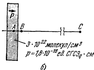
Рис. 9.21. а) Диск, состоящий из полярных молекул с дипольными моментами, направленными параллельно оси. б) Поперечное сечение диска. в) Поперечное сечение эквивалентных заряженных слоев.
