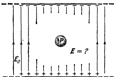
Рис. 9.28. Источники поля E_0 остаются неподвижными. В диэлектрическом шаре возникает поляризация P . Полное поле E является суперпозицией поля E_0 и поля этого поляризованного шара.
