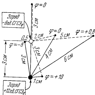
Рис. 2.6. Электрический потенциал \varphi в различных точках системы из двух точечных зарядов, \varphi стремится к нулю на бесконечно большом расстоянии. Заряд выражен в единицах СГСЭ _q , потенциал \varphi выражен в единицах СГСЭ _V , или в эргах на единицу заряда.
