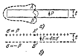
Рис. 9.19. а) Линейный интеграл от E на пути от A до B должен быть одинаковым для всех путей, внутренних и внешних, так как внутренние («микроскопическое», или «атомное») электрические поля также консервативны ( \text{rot } E = 0 ). Эквивалентные заряженные слои (б) имеют такое же внешнее поле.
