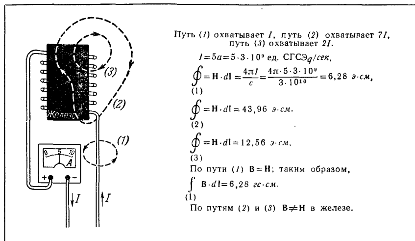
Рис. 10.24. Иллюстрация соотношения между свободным током и линейным интегралом от H .
