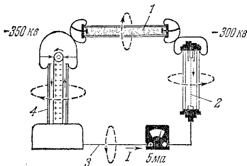
Рис. 6.7. Линейный интеграл от B имеет совершенно одинаковые значения вокруг любой части этого контура, несмотря на то, что скорости носителей зарядов в каждой части совершенно различны. 1 — чистая вода; отрицательные ионы движутся вправо со скоростью 3,5 см/сек; положительные ионы движутся влево со скоростью 2 см/сек. 2 — высоковольтный пучок электронов в вакууме; скорость электронов 2,4 \cdot 10^{10} см/сек. 3 — медный провод; электроны проводимости дрейфуют влево со средней скоростью 10^{-4} см/сек. 4 — генератор Ван-де-Граафа; отрицательные заряды движутся вверх, положительные — вниз, v \sim 2000 см/сек.
