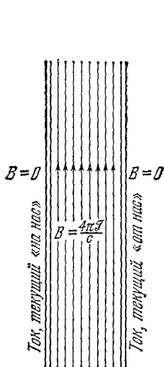
Рис. 6.23. Магнитное поле между двумя плоскопараллельными листами с током.
