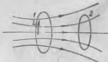
Рис. 299. Поток индукции, пронизывающий два контура.
