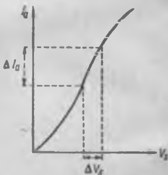
Рис. 357. Характеристика трехэлектродной лампы.
