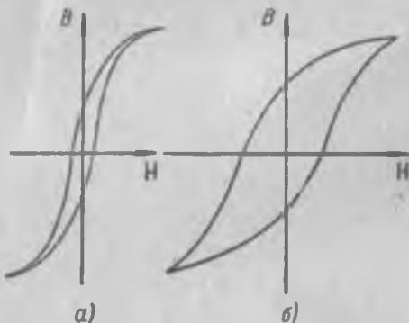
Рис. 223. Петля гистерезиса для: а — „мягкого“ материала; б — „жесткого“ материала.
