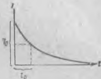
Рис. 297. Зависимость силы экстратока размыкания от времени.
