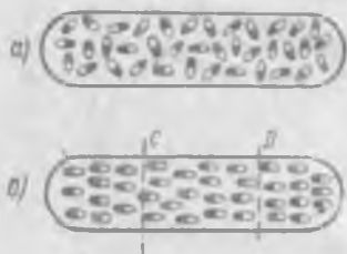
Рис. 6. Поляризация диэлектрика.
