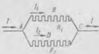
Рис. 114. Параллельное соединение двух проводников B и D .
