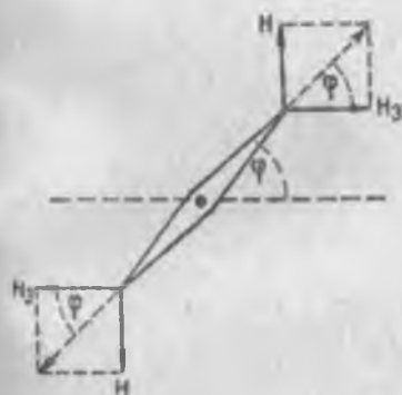
Рис. 252. К определению положения равновесия стрелки тангенс-гальванометра.
