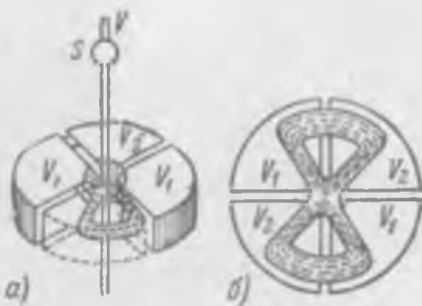
Рис. 79. Квадрантный электрометр.
