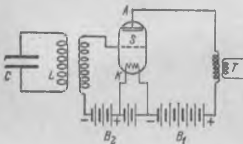
Рис. 356. Схема усиления электромагнитных колебаний.
