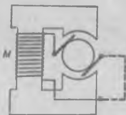
Рис. 314. Схема динамомашины с последовательным возбуждением.
