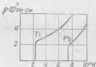
Рис. 82. Падение удельного сопротивления до нуля при переходе в сверхпроводящее состояние.
