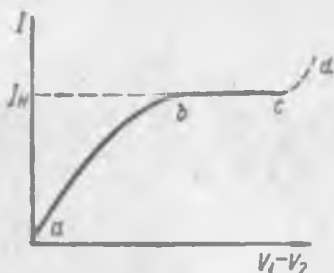
Рис. 154. Зависимость силы тока I от разности потенциалов V_1 - V_2 для случая несамостоятельной проводимости.
