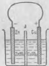
Рис. 104. Элемент Даниэля.
