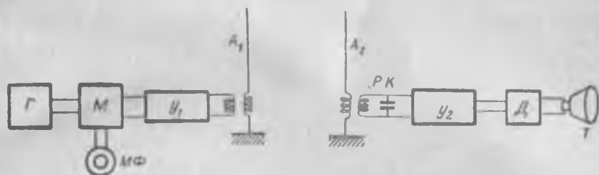
Рис. 359. Схема передающей и принимающей радиостанций.
