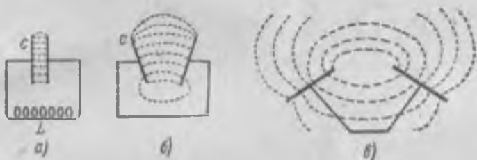
Рис. 343. Колебательные контуры различной степени открытости.
