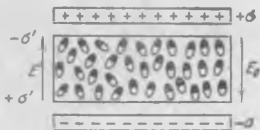
Рис. 53. Диэлектрик в конденсаторе.
