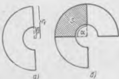
Рис. 74. Пластины конденсатора переменной емкости.
