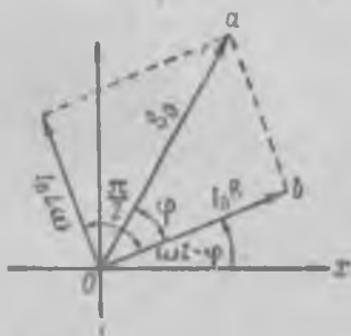
Рис. 305. Векторная диаграмма для цепи переменного тока с самоиндукцией.
