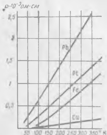
Рис. 81. Зависимость удельного сопротивления металлов от абсолютной температуры T .
