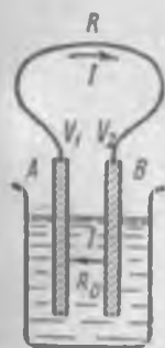
Рис. 106. Цепь гальванического элемента и внешнего со- противления.
