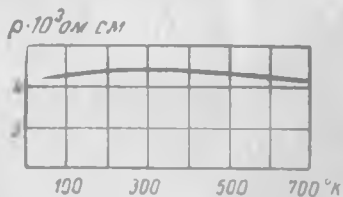
Рис. 93. Зависимость удельного сопротивления \rho манганина от абсолютной температуры T .
