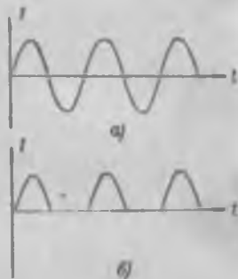
Рис. 320. Изменение со временем силы: а — переменного тока; б — тока, пропущенного через выпрямитель.
