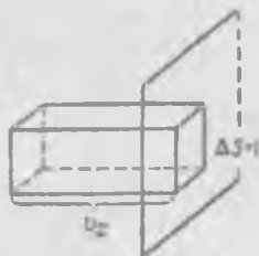
Рис. 141. К подсчету числа электронов, вылетающих с единицы поверхности в единицу времени.
