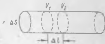
Рис. 84. К выводу выражения для плотности тока.
