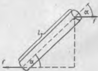
Рис. 230. К определению момента сил, действующего на магнит.
