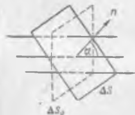
Рис. 20. Площадка \Delta S , расположенная наклонно по отношению к линиям напряженности.
