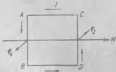
Рис. 198. Силы, действующие на рамку с током, расположенную параллельно линиям магнитной напряженности.
