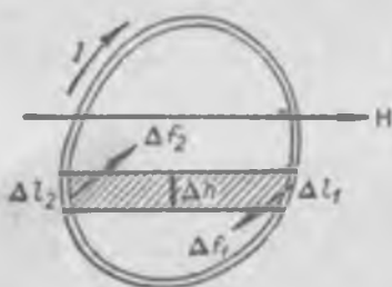
Рис. 202. К подсчету момента сил, действующих на контур с током, расположенный параллельно напряженности магнитного поля.
