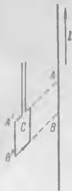
Рис. 176. Свободно поворачивающаяся рамка располагается в плоскости AA'BB' , проходящей через провод.
