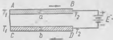
Рис. 134. Метод обнаружения явления Томсона.
