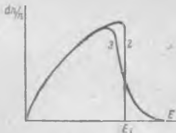
Рис. 103. Распределение электронов по энергиям: 2 — при T=0 ; 3 — при T \neq 0 .
