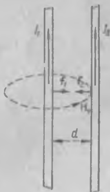
Рис. 199. Взаимодействие двух прямолинейных бесконечных токов.
