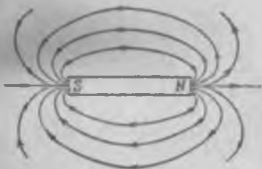
Рис. 228. Линии напряженности постоянного прямого магнита.
