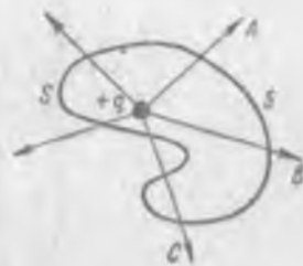
Рис. 23. Пересечение линиями напряженности произвольной замкнутой поверхности.
