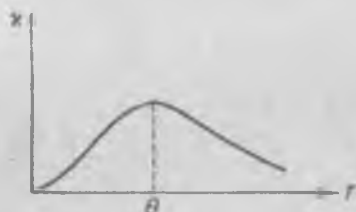
Рис. 226. Зависимость коэффициента намагничения \chi от температуры для антиферромагнетиков.
