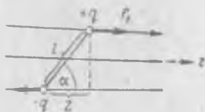
Рис. 49. Диполь во внешнем неоднородном поле.
