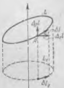
Рис. 209. К расчету циркуляции вектора магнитной напряженности H .
