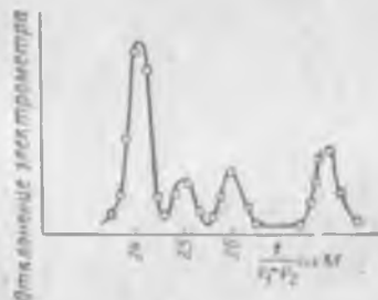
Рис. 279. Кривая для изотопов магния.
