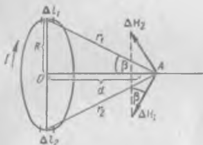
Рис. 191. К подсчету напряженности магнитного поля на оси кругового тока.
