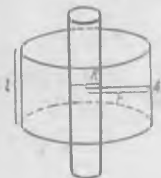
Рис. 31. К определению напряженности поля заряженного цилиндра.
