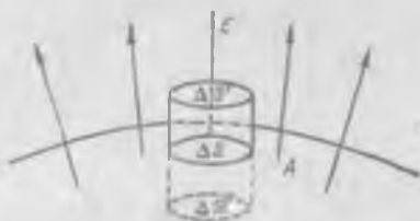
Рис. 45. К определению напряженности поля E вблизи поверхности заряженного проводника.
