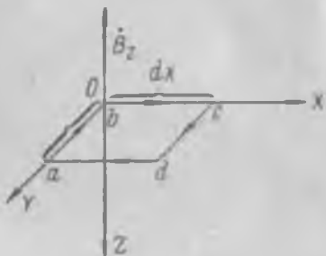
Рис. 342. К определению второй системы уравнений Максвелла.
