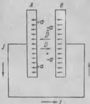
Рис. 338. Возникновение тока смещения между обкладками конденсатора.
