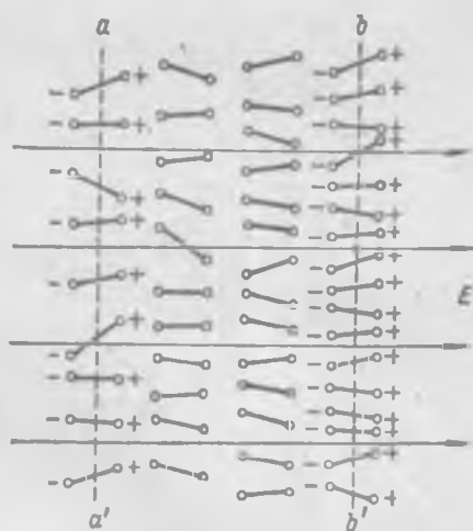
Рис. 54. Появление объемных зарядов при поляризации неоднородного диэлектрика.
