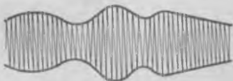
Рис. 358. Огибающая высокочастотных колебаний.
