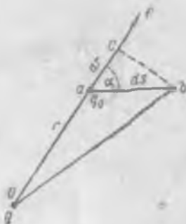
Рис. 32. К определению работы перемещения заряда q_0 на пути ds .
