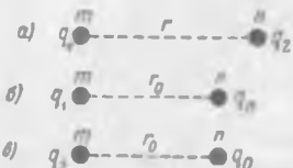
Рис. 8. К обоснованию закона Кулона.
