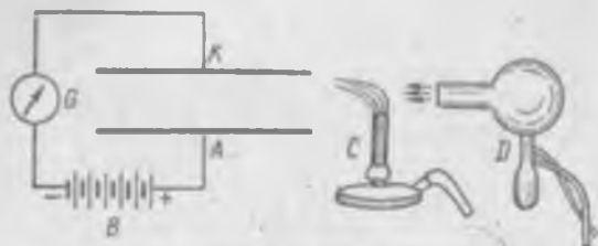
Рис. 151. Увеличение ионов потоком воздуха.
