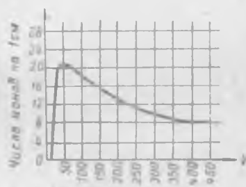
Рис. 165. Зависимость числа образуемых ионов ртути ( \text{Hg}^+ ) от скорости электронов.
