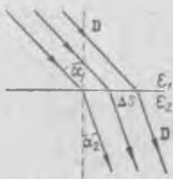
Рис. 63. Непрерывность линий индукции при прохождении через границу двух диэлектриков.
