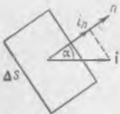
Рис. 83. К определению нормальной составляющей плотности тока I_n .
