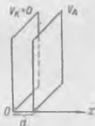
Рис. 160. К выводу формулы Богуславского — Ленгмюра.
