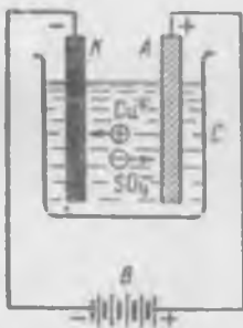
Рис. 142. Движение ионов \text{Cu}^{++} и \text{SO}_4^{--} при электролитической проводимости раствора медного купороса.
