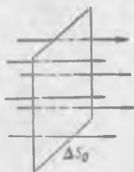
Рис. 19. Площадка \Delta S_0 , перпендикулярная к линиям напряженности.
