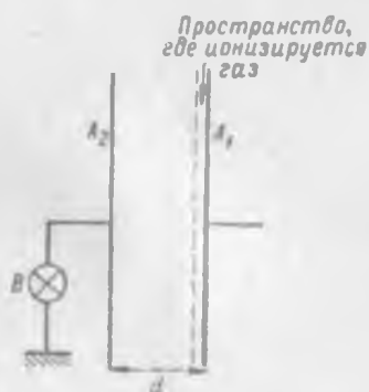
Рис. 158. Схема метода определения подвижности ионов.
