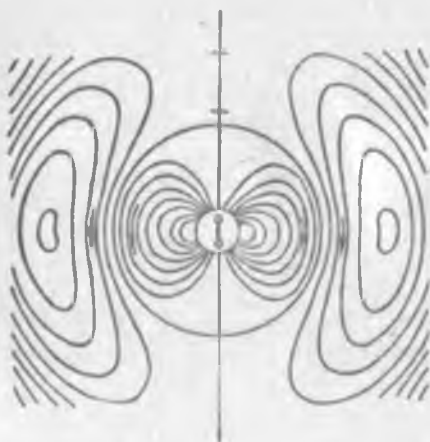
Рис. 348. Линии напряженности около диполя.
