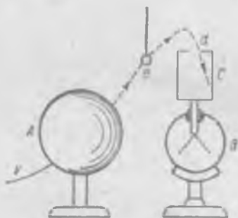
Рис. 44. Опыт с цилиндром Фарадея.
