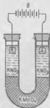
Рис. 146. Метод наблюдения подвижности ионов.
