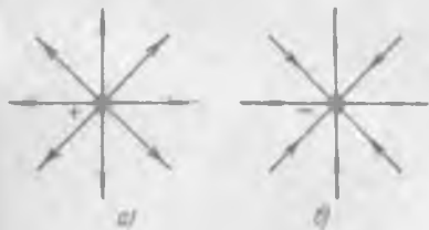
Рис. 16. Линии напряженности точечного заряда: а — положительного; б — отрицательного.
