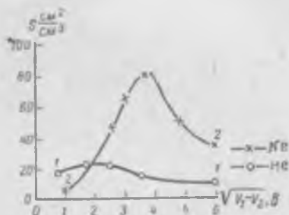
Рис. 163. Зависимость от скорости электронов эффективного сечения S атомов He и Ne, находящихся в 1 см 3 при 0°C и при давлении 1 мм Hg.
