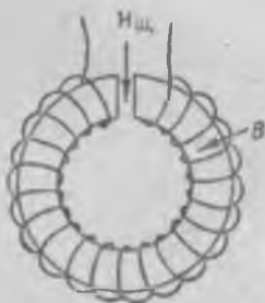
Рис. 218. Напряженность магнитного поля H_{щ} в щели равна магнитной индукции B в ферромагнетике.
