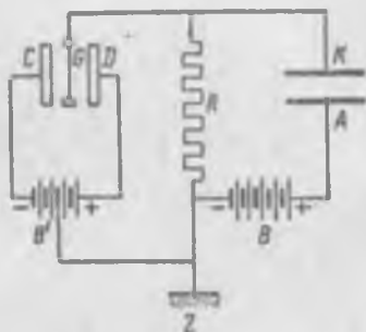
Рис. 153. Измерение малых токов методом постоянного отклонения.
