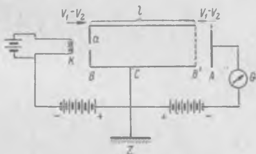
Рис. 161. Схема метода определения средней длины свободного пути электронов.
