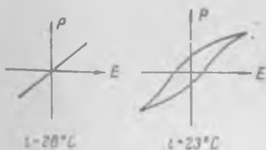
Рис. 66. Зависимость поляризации сегнетовой соли от меняющейся со временем напряженности поля.
