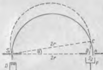
Рис. 278. Схема отклонения частиц в поперечном магнитном поле.
