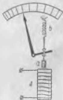
Рис. 254. Амперметр Доливо-Добровольского.
