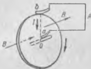
Рис. 295. Возникновение индукционного тока во вращающемся диске.
