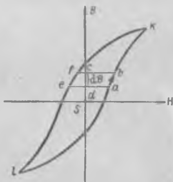
Рис. 300. К подсчету работы перемагничивания.
