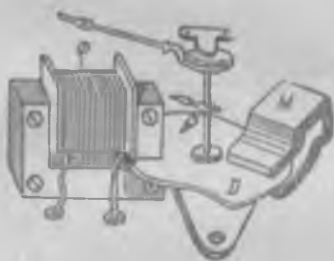
Рис. 323. Схема индукционного амперметра.
