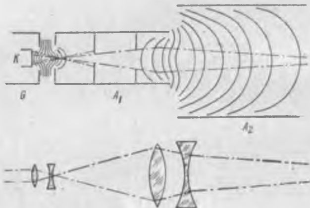
Рис. 284. Фокусирующая система осциллографа.
