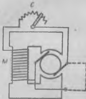
Рис. 315. Схема динамомашины с параллельным возбуждением.
