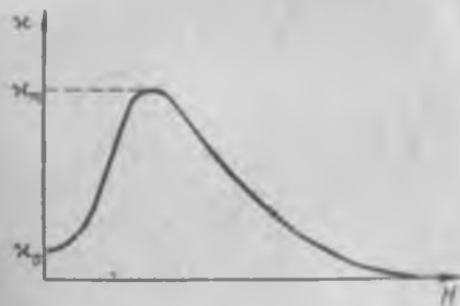
Рис. 221. Зависимость для ферромагнетика коэффициента намагничивания \kappa от напряженности поля H .
