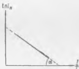
Рис. 140. Линейная зависимость логарифма тока насыщения от 1/T .
