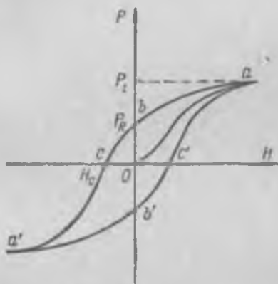
Рис. 222. Петля гистерезиса.
