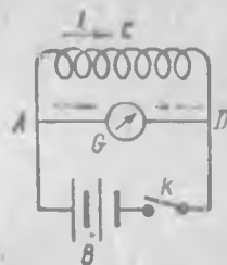
Рис. 296. Обнаружение экстратока размыкания.
