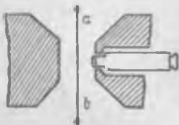
Рис. 258. Струнный гальванометр.
