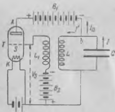
Рис. 337. Схема возбуждения незатухающих колебаний с помощью трехэлектродной лампы.
