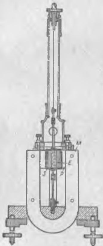
Рис. 257. Зеркальный гальванометр.
