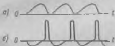
Рис. 318. Кривая зависимости силы тока от времени в индукционной катушке: а — в первичной обмотке; б — во вторичной обмотке.
