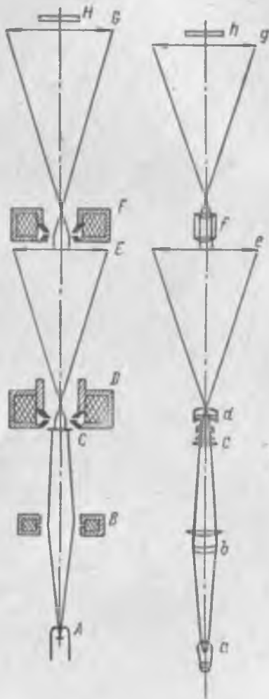
Рис. 286. Схемы микроскопов: электронного (слева) и оптического.
