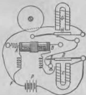
Рис. 354. Схема приемника А. С. Попова.
