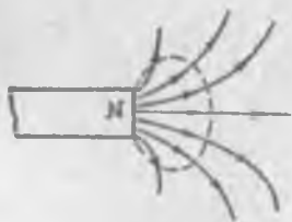
Рис. 238. Линии магнитной напряженности вблизи конца прямого и длинного магнита.
