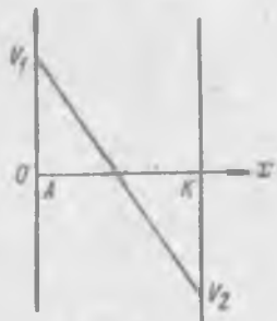
Рис. 155. Распределение потенциала V между электродами при отсутствии ионизации.
