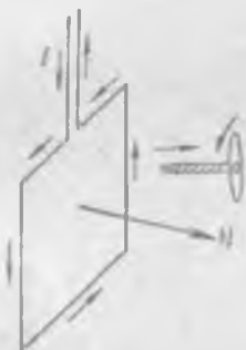
Рис. 177. Направление положительной нормали к рамке с током.
