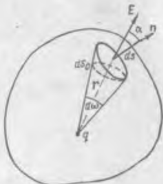
Рис. 24. К более точному выводу теоремы Остроградского — Гаусса.
