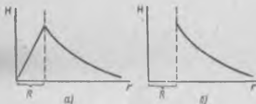
Рис. 213. Зависимость напряженности магнитного поля H от расстояния до оси цилиндра: а — для тока, текущего равномерно по сечению проводника; б — для тока, текущего по поверхности проводника.
