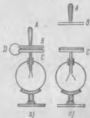
Рис. 121. Обнаружение контактной разности потенциалов.
