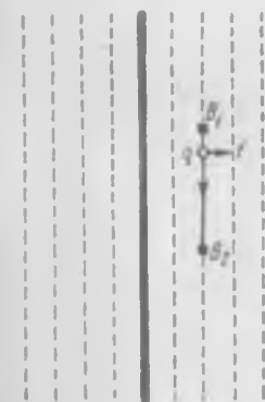
Рис. 37. Поверхности уровня потенциала бесконечной заряженной плоскости.
