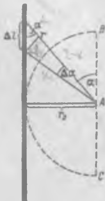
Рис. 188. К подсчету напряженности магнитного поля прямого тока.
