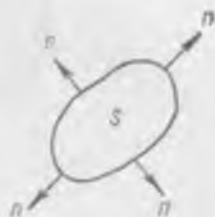
Рис. 85. Внешние нормали к замкнутой поверхности S .
