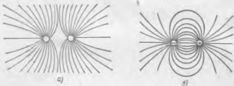
Рис. 17. Линии напряженности двух точечных зарядов: а — одноименных; б — разноименных.
