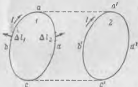
Рис. 242. К подсчету работы перемещения замкнутого контура с током в магнитном поле.
