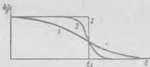
Рис. 102. Распределение электронов по энергетическим уровням: 1 — по Больцману при T \neq 0 ; 2 — по Ферми при T=0 ; 3 — по Ферми при T \neq 0 .
