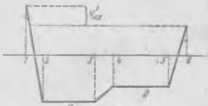
Рис. 124. Потенциальная яма двух соприкасающихся металлов.
