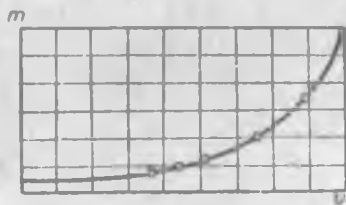
Рис. 272. Зависимость массы электрона от скорости.
