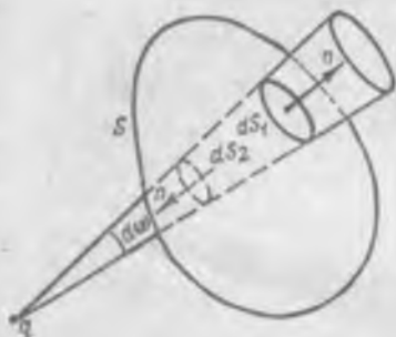
Рис. 25. К определению потока от заряда, находящегося вне замкнутой поверхности.
