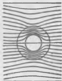
Рис. 237. Расположение линий магнитной индукции в теле с полостью.
