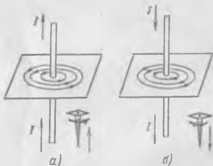
Рис. 179. Направление линий напряженности магнитного поля прямого тока.
