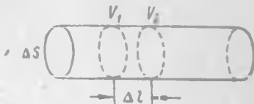
Рис. 84. К выводу выражения для плотности тока.
