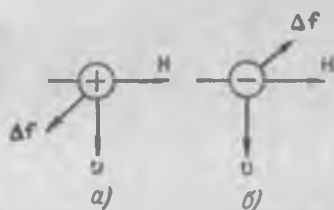
Рис. 261. Направление силы Лоренца \Delta f , действующей на заряд, движущийся со скоростью v в магнитном поле напряженности H .
