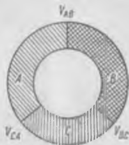
Рис. 125. Замкнутая цепь из трех металлов.
