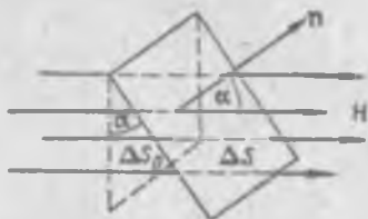
Рис. 184. Линии напряженности, проходящие через косо расположенную площадку \Delta S .
