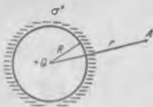
Рис. 56. Влияние диэлектрика на поле заряженного шара.
