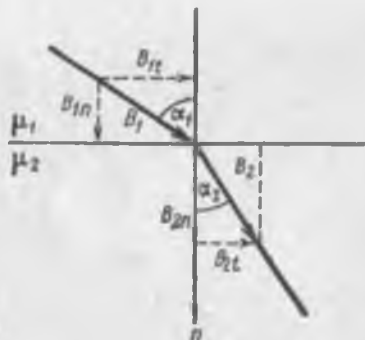
Рис. 236. Преломление линий магнитной индукции B на границе двух магнетиков.
