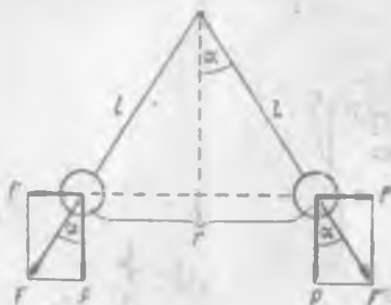
Рис. 10. Силы, действующие на наэлектризованные шары.
