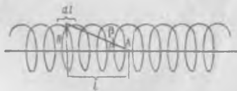
Рис. 192. К подсчету напряженности магнитного поля внутри соленоида.
