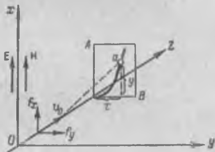
Рис. 275. Схема метода парабол.
