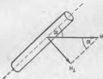
Рис. 229. Составляющая напряженности поля H , перпендикулярная оси магнита.
