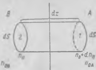
Рис. 126. К подсчету давления электронного газа.
