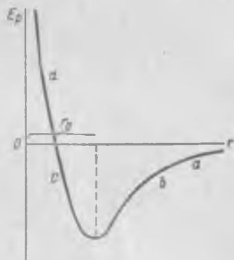
Рис. 144. Зависимость потенциальной энергии E_p от расстояния r .
