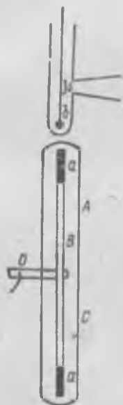
Рис. 264. Схема опыта Эйхенвальда.
