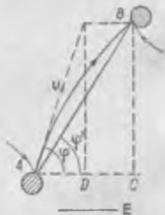
Рис. 169. К определению пути электрона между двумя столкновениями.
