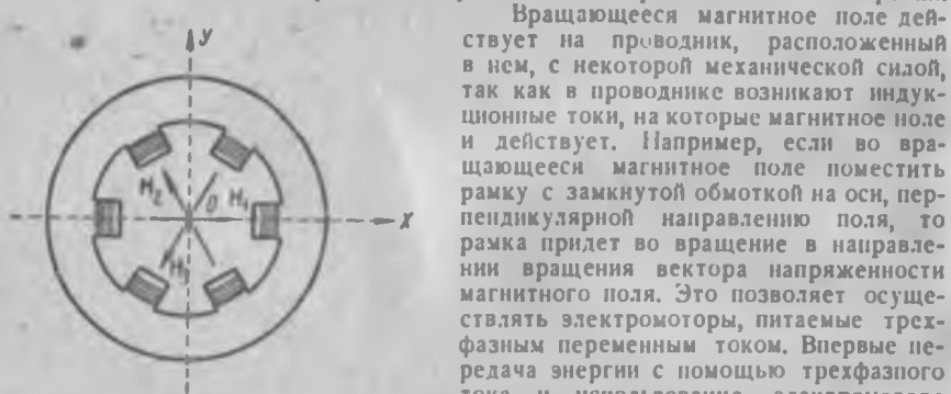
Рис. 328. Кольцевая магнитная цепь.
