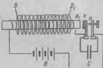
Рис. 317. Индукционная катушка.
