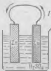
Рис. 128. Гальванический элемент из пластинок цинка и меди, погруженных в раствор серной кислоты.
