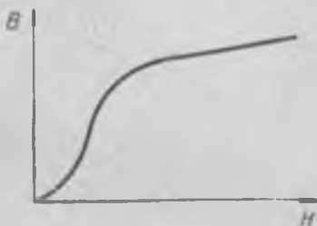
Рис. 220. Зависимость для ферромагнетика магнитной индукции B от напряженности поля H .
