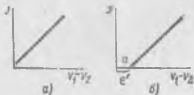
Рис. 147. Зависимость силы тока I от разности потенциалов. а — для проводника первого рода; б — для проводника второго рода (электролита).
