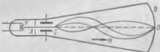
Рис. 273. Схема метода магнитной фокусировки.
