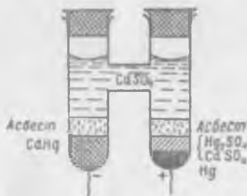
Рис. 119. Нормальный элемент.
