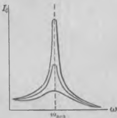
Рис. 333. Резонансные кривые силы тока I .
