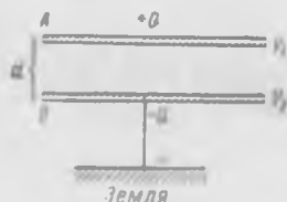
Рис. 50. Плоский конденсатор.
