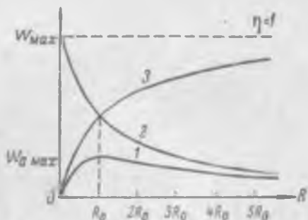
Рис. 109. Зависимость от сопротивления внешней части цепи R : 1 — мощности W_a , выделяемой во внешней части цепи; 2 — полной мощности W ; 3 — коэффициента полезного действия \eta .
