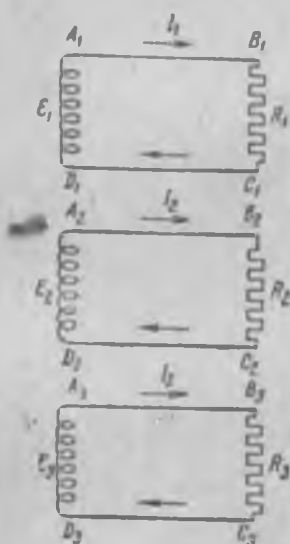
Рис. 325. Схема возбуждения трехфазного тока.
