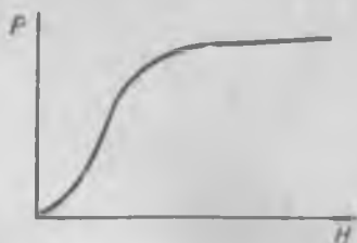
Рис. 219. Зависимость для ферромагнетика вектора намагничивания \mathbf{P} от напряженности поля \mathbf{H} .
