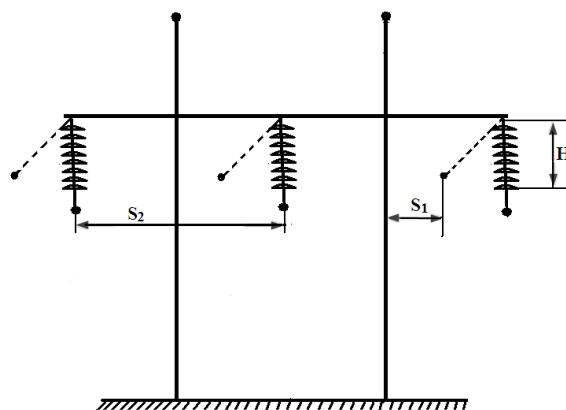
4.1- rasm. Portal rusumidagi tayanchda bajarilgan liniyaning izolyatsiya oraliqlarining ko'rinishi.
