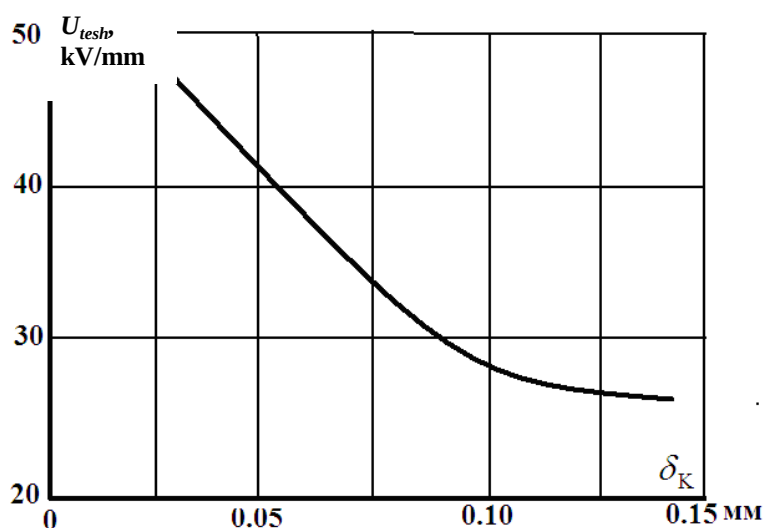
4.13- rasm. Qog'ozli moyli izolyatsiya uchun elektr maydonining teshilish kuchlanganligining qog'oz qalinligiga bog'liqliligi.
