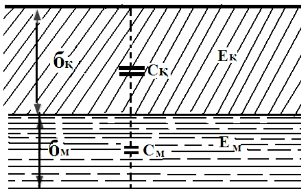
4.12- rasm. Qog'ozli – moyli izolyatsiyaning ekvivalent sxemasi.
