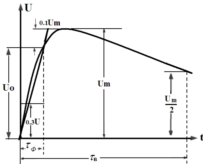
2.7- rasm. Standart impuls to'liqining va frontining uzunligini aniqlash
