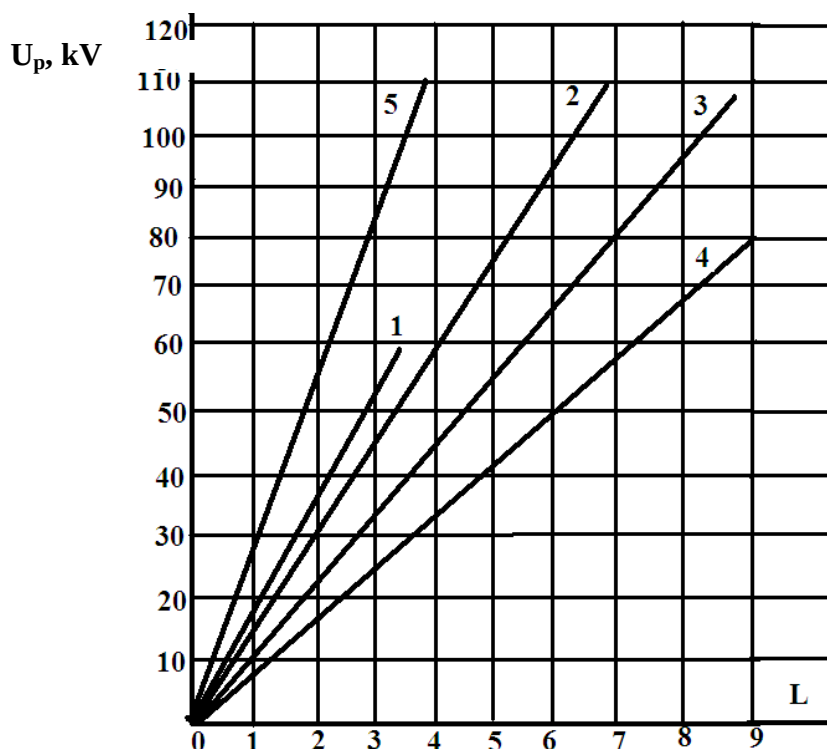
2.11-rasm. Namunalar sirti bo'ylab razryadlanish kuchlanishining elektrodlar orasidagi masofaga bog'liqligi. Oraliqning konstruksiyasi (2.10- rasm): 1 – toza havo oralig'i; 2 – elektrotehnika; 3 – shisha; 4- shisha va chini dielektriklarning elektrodlanga gips joylashmagan holatida.
