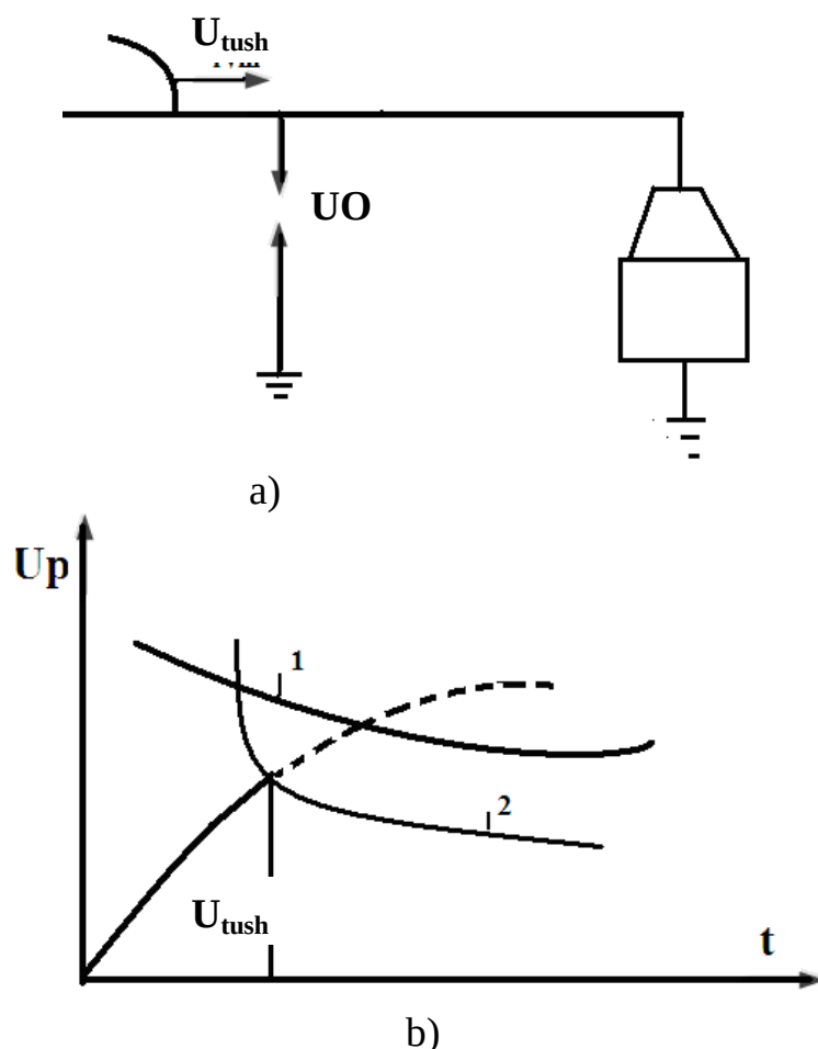
8.9- rasm. Himoya uskunasi ishlash prinsipi: a– uchqun oralig'i (UO)ning sxemasi; b– himoyalananayotgan element (1) va uchqun oralig'i (UO)ning volt–sekund xarakteristikalarini moslashtirish.
