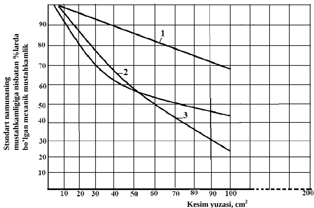
3.4- rasm. TSilindr shaklidagi chinnining mexanik mustahkamligini ko'ndalang kesim yuzasiga bog'liqligi: 1 – siqishga; 2 – cho'zishga; 3 – egishga.
