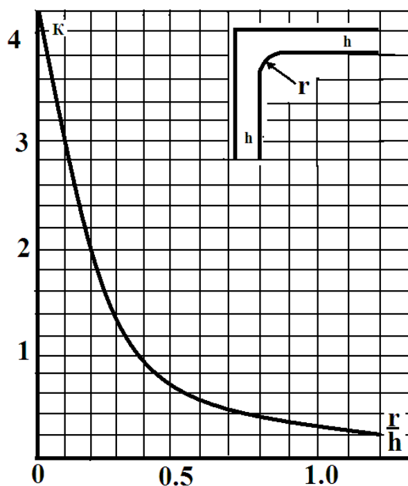
5.2- rasm. Elektr maydon notekisligi K ni o'tmaslashtirish radiusi r ning izolyatsiya qalinligi h ga nisbatiga bog'liqligi
