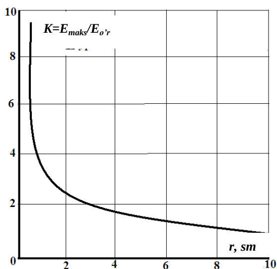
2.1- rasm. Silindrik kondensatorning tashqi radiusi R = 10 \text{ sm} va oʻzgarmas boʻlganda bir jinsli boʻmaganlik koeffitsienti K ning ichki tsilindr radiusi r ga bogʻliqligi
