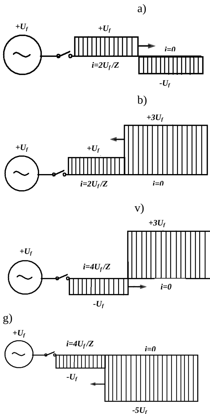
7.12- rasm. O'chirilayotgan liniya bo'ylab kuchlanishning har xil momentlar uchun taqsimlanishi. a – birinchi yoy yongandan so'ng uning liniya oxiridan qaytgunicha; b – xuddi to'lqinning liniya oxiridan qaytgandagisi; v - ikkinchi yoy yongandan so'ng uning liniya oxiridan qaytgunicha; g - xuddi to'lqinning liniya oxiridan qaytgandagisi hisoblanadi.
