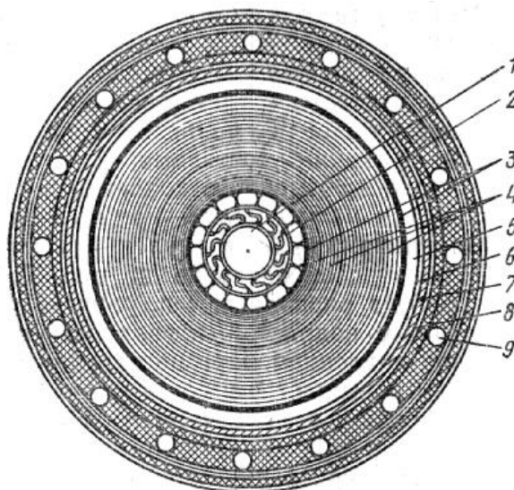
4. 18- rasm. Kuchlanishi 220 kVga muljallangan o'rta bosimli kabel: 1 – moy o'tkazuvchi kanal; 2 – fasonli o'tkazgichdan yasalgan pay; 3 – yarim utkazgichli va metallashtirilgan qog'ozdan tashkil topgan pay bo'ylab joylashtirilgan ekran; 4 – xar xil qalinlikda va xar xil zichlikdagi qog'ozdan yasalgan izolyatsiya; 5 – qo'rg'oshin qobiq; 6 –plastikatdan yasalgan lenta; 7 – misdan yasalgan kuchaytiruvchi lenta; 8 – ximoya jobdig'i; po'lat sim.
