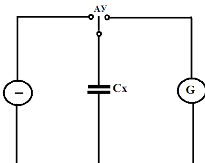
6.5- rasm. Ikkita chastotada izolyatsiyaning sig'imini o'lchashning printsipl sxemasi.
