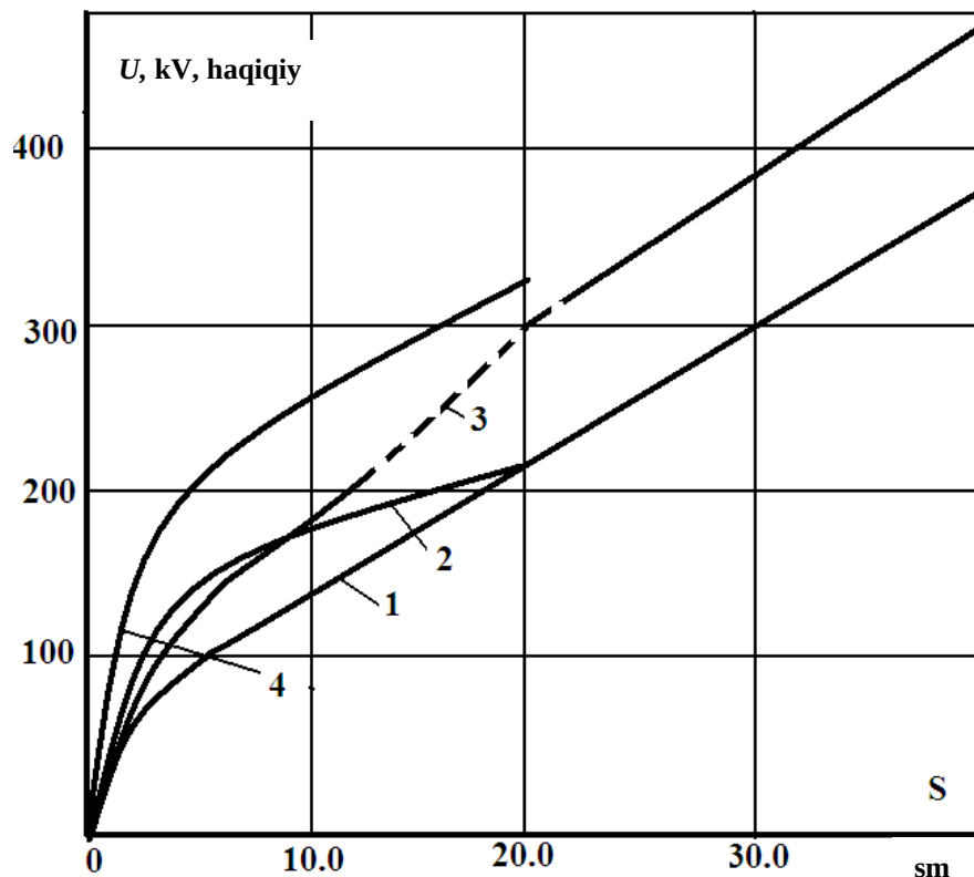
5.4- rasm. Sanoat chastotasida elektrodnlarni yupqa qatlamli dielektrik bilan qoplanishining ta'siri. Elektrodlar parallel:
