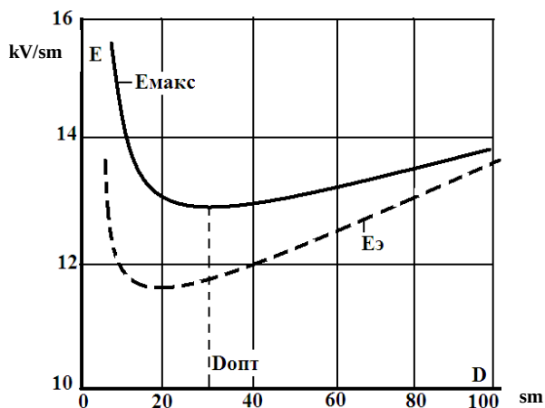
1.8- rasmda. Parchalangan o'tkazgich sirtidagi maksimal va ekvivalent elektr yurituvchi kuchining o'tkazgichlar orasidagi masofaga bog'liqligi.
