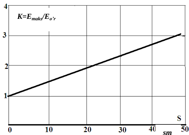
2.2- rasm. Diametri D = 20 \text{ sm} boʻlgan sharlar orasidagi elektr maydon bir jinsli boʻmaganlik koeffitsientining sharlar orasidagi masofaga bogʻliqligi.
