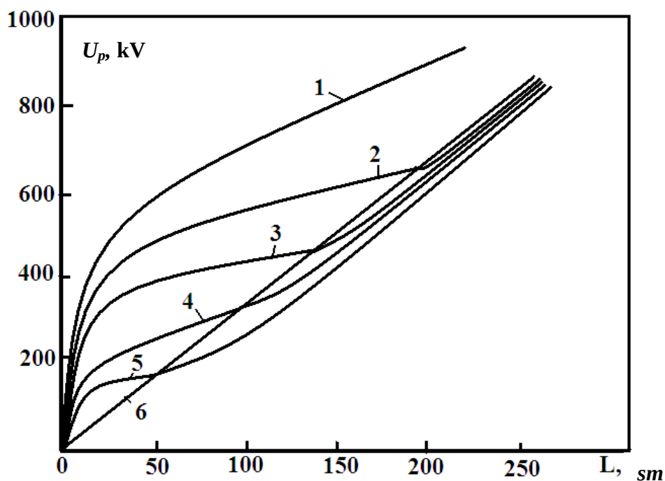
3.15- rasm. Razryadlanish kuchlanishining «shar – tekislik» elektrod-lari orasidagi havo oralig'ining uzunligiga bog'liqligi: 1 – shar diametri 100 sm; 2 – 75 sm; 3 – 50 sm; 4- 25 sm; 5 – 12.5 sm; 6 - «sterjenъ – tekislik» oralig'i.
