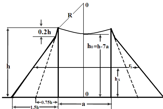
8.4- rasm. Ikkita sterjen ko'rinishidagi YAQning himoyalash sohasi.
