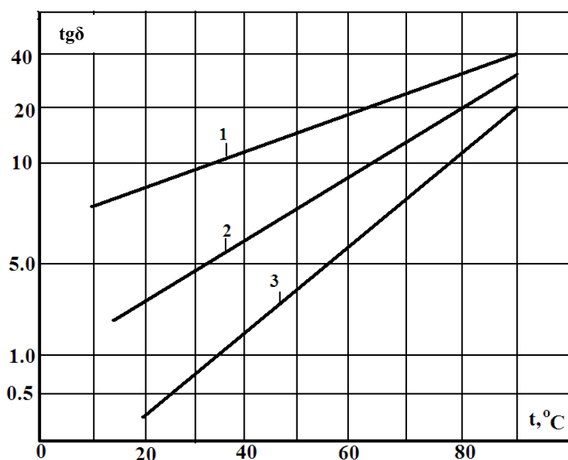
6.6- rasm. Transformatorlar izolyatsiyasi uchun \operatorname{tg} \delta = f(t^{\circ}) funktsional bog'lanishlarning grafigi: 1 va 2 – ho'llangan holatlar ; 3 – quruq xolat.
