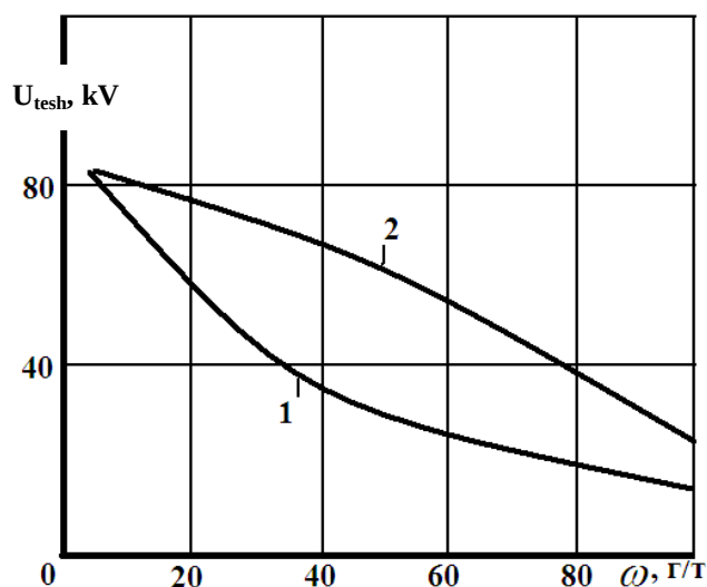
3.5- rasm. Atrof muhit temperasturasi 25 0 S va 50 Gts da transformator moyining teshilish kuchlanishini namlikka bog'liqligi: 1 – tarkibida 50 g/t kontsentatsiyali qattiq birkmalar mavjud bo'lgan texnik toza moy uchun; 2 – tarkibida 0,5 g/t kontsentatsiyali qattiq birkmalar mavjud bo'lgan texnik toza moy uchun.
