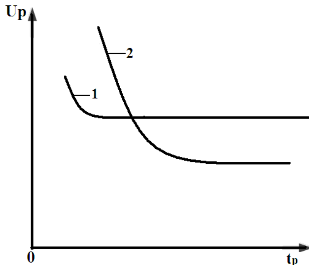
2.7- rasm. Birjisli (1) va keskin bir jinsli bo'magan (2) elektr maydonli (chaqmoqli impuls) oraliq uchun volt–sekund harakteristikasining ko'rinishi
