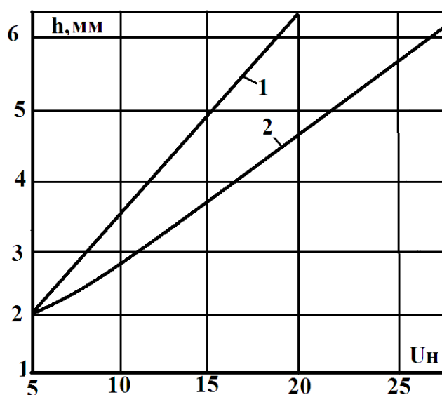
5.3- rasm. Korpus izolyatsiyasi qalinligining generatr nominal kuchlanishiga bog'liqligi: 1 – kempoundlangan mikalent; 2 – termoreaktiv.
