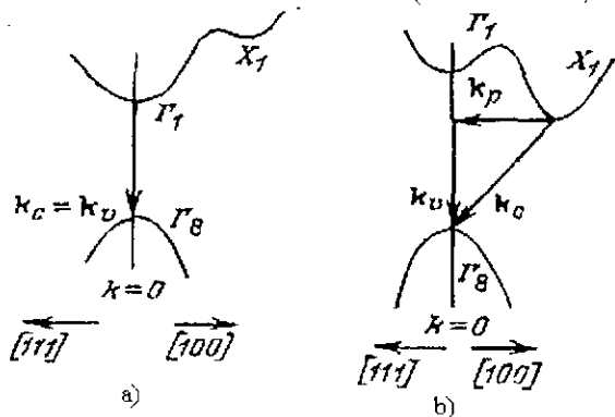
YIII. 1-rasm. To'g'ri (a) va noto'g'ri (b) elektron o'tishlar.
