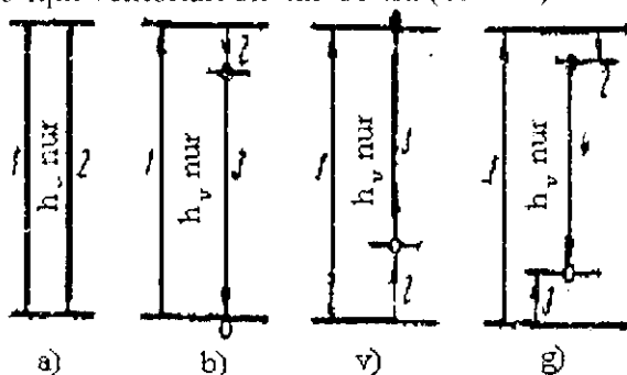
IV.2-rasm. Energetik diagrammalar. a-to'g'ri nurlanish rekombinatsiyasi; b,v,g-lokal markazlar ishg'ol qilgan nurlanish rekombinatsiyasi.
