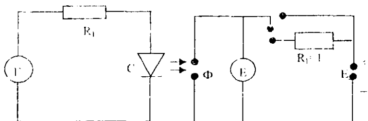
2-rasm. Fotoasboblarning inersion xususiyatlarini o'rganish qurilmasi.
