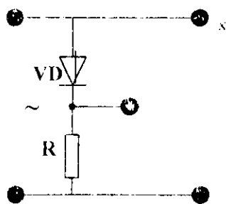
2- rasm. Volt-ampér xarakteristikasini ossillograf ekranida ko'rish sxemasi.
