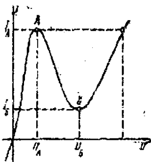
VI.3-rasm. Tunnel diodning volt-ampér xarakteristikasi
