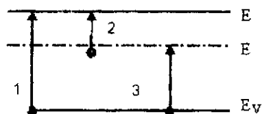
III.1 rasm. Ta'qiqlangan zonadagi elektronning mumkin bo'lgan optik o'tishlari sxemasi.
