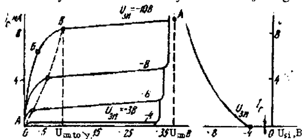
VII.12-rasm. Induksiyalangan kanalli maydon tranzistorining chiqish xarakteristikasi
