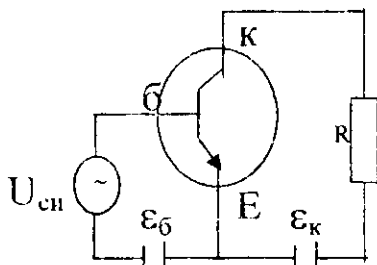
2 - rasn. Umumiy emmitterli ulash sxemasi.
