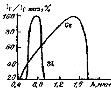
VIII.5–rasm. Germaniy va kremniy asosidagi fotodiodlarning spektral xarakteristikalar.
