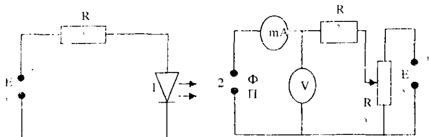
1-rasm. Fotoasboblar statistik xarakteristikalarini o'rganish qurilmasi.
