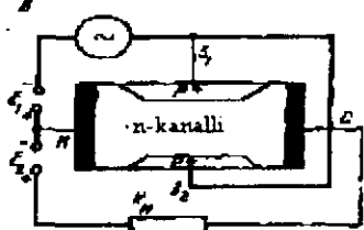
VII.8-rasm. Boshqariladigan p-n o'tishli maydon tranzistori.
