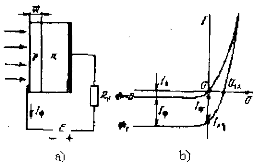
YIII.4 rasm. Fotodiodning ulash sxemasi (a) va volt-amper xarakteristikasi (b).
