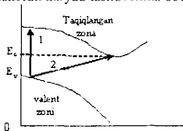
III. 2-rasm. To'g'ri 1 va noto'g'ri 2 zonalarda optik o'tish.
