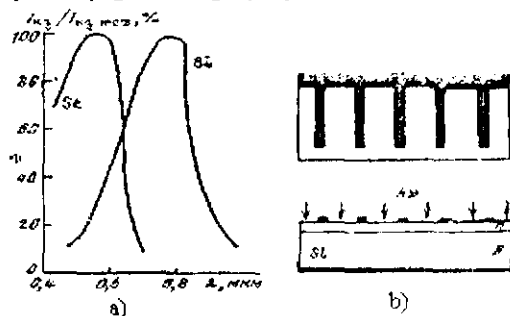
VIII.7 - rasm. Quyosh elementining spektral xarakteristikasi (a) va struktyravii tuzilishi.
