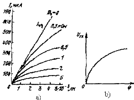
VIII.6 - rasm. Iste'molchi qarshiligining qiymatlarida fotoelementning yorug'lik xarakteristikalarini (a) va salt yurish kuchlanishining yorug'lik oqimidan bog'liqligi (b).
