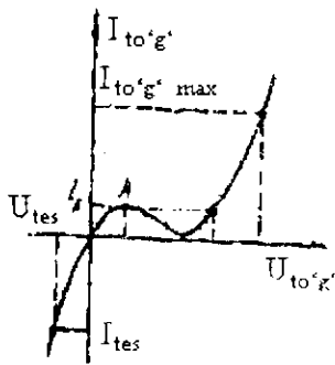
VI.4-rasm. Aylantirilgan diodning volt-ampér xarakteristikasi
