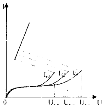
3 - rasm. Boshqaruv tokining turli qiymatlarida tiristorning volt - amper xarakteristikasi.
