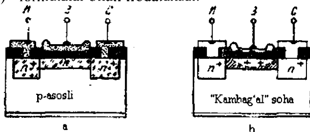
VII.10-rasm. Kanal o'rnatilgan maydon tranzistorining tuzilishi.
