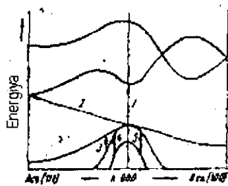
II.- 2-rasm Germaniyning Energetik zonalari.
