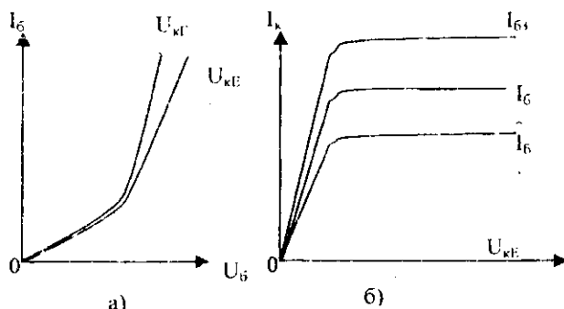
3 - rasn. Tranzistorning kirish va chiqish xarakteristikallari.
