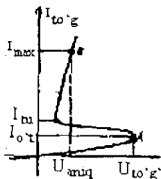
VII.15-rasm Tranzistorning amper xarakteristikasi.
