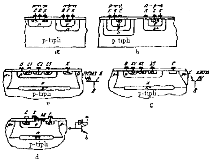
VII.7 rasmi. Integral tranzistorlar: a-gorizontual strukturali komplementar tranzistorlar; b- vertikal strukturali komplementar tranzistorlar; v-ko'p emitterli tranzistor; g-ko'p kollektorli tranzistor; d-Shotki to'sig'iga ega bo'lgan tranzistor.
