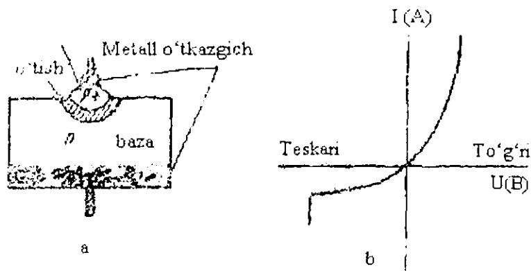
VI.1- rasn. Yarim o'tkazgichli diodning tuzilishi (a) va uning volt-ampér xarakteristikasi (b).
