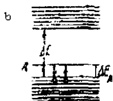
V.3-rasm. n-tipli yarimo'tkazgichning hosil bo'lishi
