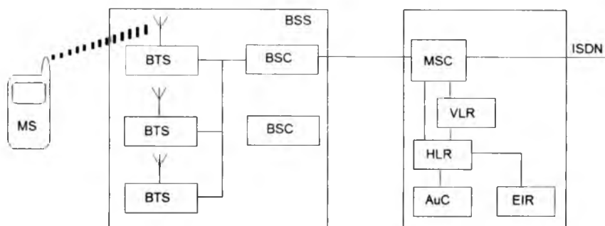
4.2-rasm. GSM tarmogʻining tuzilish sxemasi.
