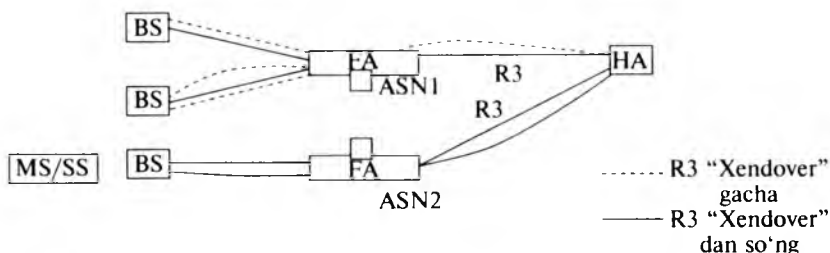
31.5-rasm. Mobillikni boshqarish turlarining aralash o'zaro ta'sirlashishi.
