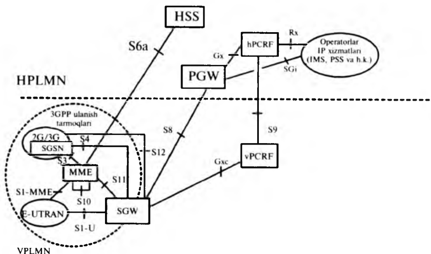
17.1-rasm. “Rouming” jarayonida LTE tarmoqlarining 3GPP tarmoqlari bilan PMIPv6 protokoli asosida o'zaro hamkorligi.
