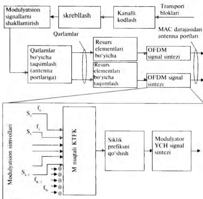
20.4-rasm. “Pastga” kanalda signalning shakllanish sxemasi.
