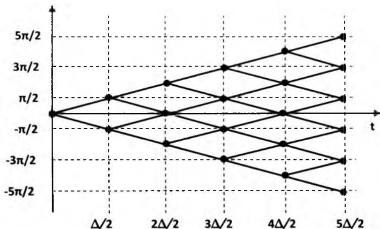
6.6-rasm. MCHM signalning oniy fazasining traektoriyalari.
