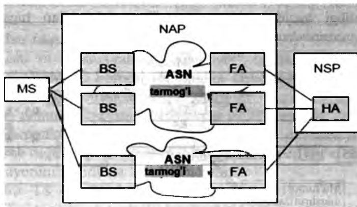
31.3-rasm. WiMAX tarmog'ida MIPning shakllantirilishi.
