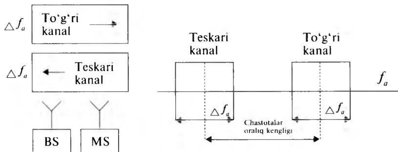
9.4-rasm. Chastotalarni dupleksli tarqoqlash prinsipida tashkillashtirish.
