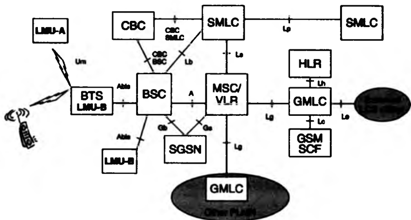
4.5-rasm. Arxitektura LVP.
