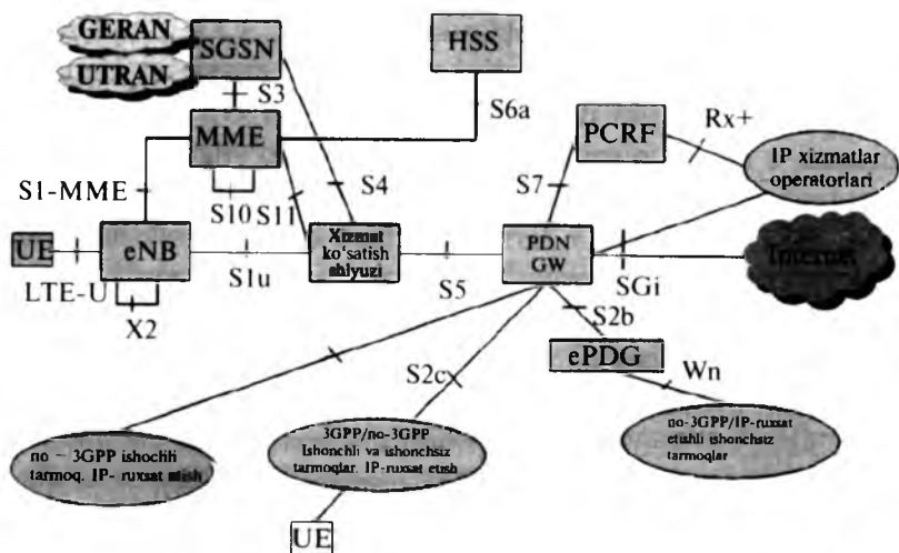
14.3-rasm. LTE/SAE tizimi arxitekturasini.
