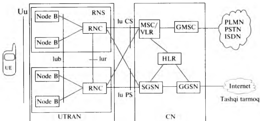
4.4-rasm. UMTS tizimlarining arxitekturası.
