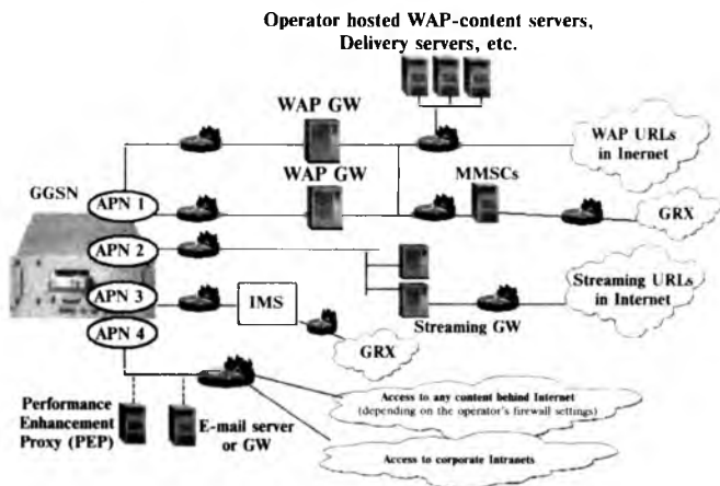
3.7-rasm. APNni proksiserverga bog‘lliqi.
