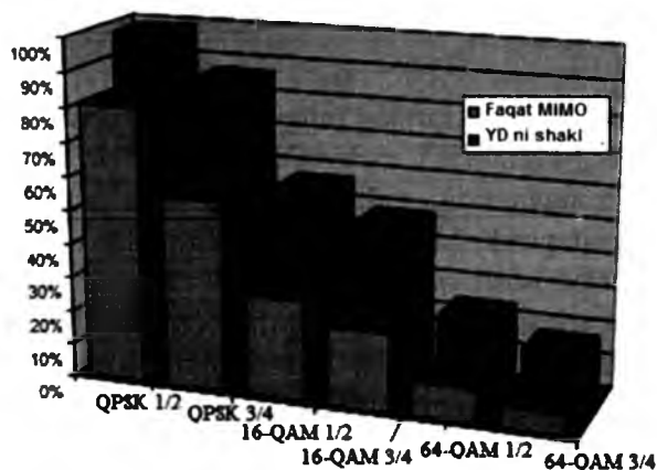
33.3-rasm. Har xil modulyatsiya va kodlash sxemalari turlarida ASS va MIMO texnologiyalari qo'llanilganda qamrab olinadigan hudud foizi.
