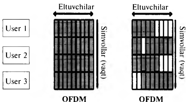
20.1-rasm. OFDM va OFDMA prinsiplari.
