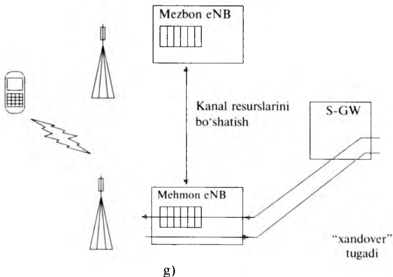
16.6-rasm. LTE tarmog'ida “xendover” jarayoni.
