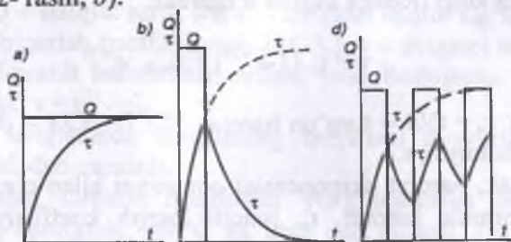
7.2- rasm. Elektr yuritmaning yuklama diagrammalari va dvigatel harorati o'zgarishining egri chiziqlari:
