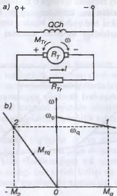
2.8-rasm. Dvigatelnining dinamik tormozlash rejimidagi elektr sxemasi (a) va mexanik tavsiflari (b).
