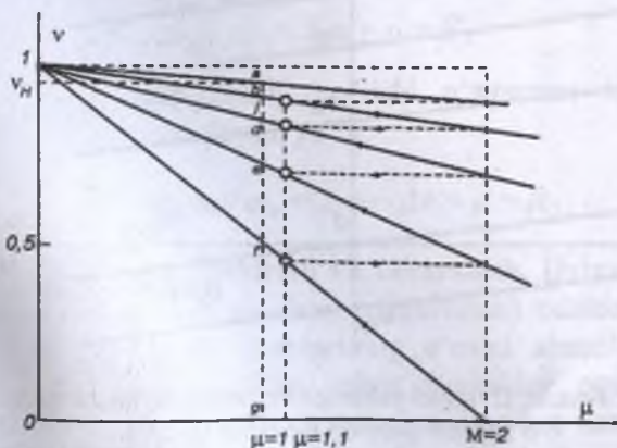
2.3-rasm. Mustaqil qo'zg'atishli o'zgarmas tok dvigateli ishga tushirish reostatlari qiymatini hisoblash.
