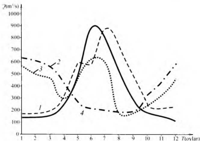
2-rasm. Har xil rejimda ishlayotgan suv omborining suv sarflari: 1 – irrigatsion; 2 – energetik; 3 – birliglikda (irrigatsion-energetik); 4 – suv omboriga o'rtacha ko'p yillik suvning oqib kelishi.
