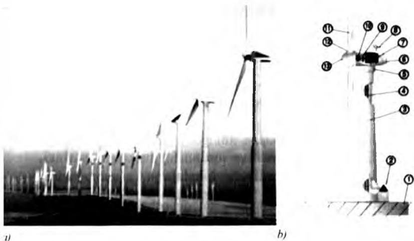
59-rasm. Sanoatda ishlab chiqariladigan shamol energetik qurilmalarining joylashishi (a) va tuzilishi (b):
