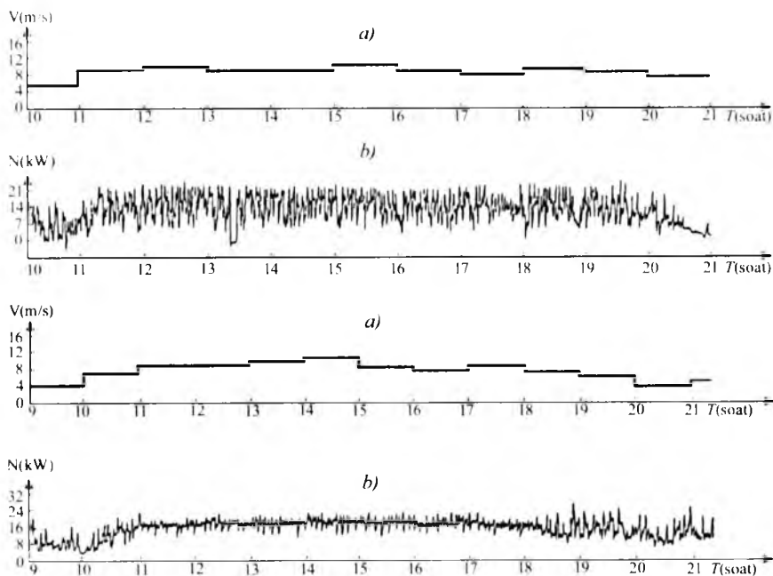
56-rasm. Shamol elektrostansiyasining ishlash grafigi:
