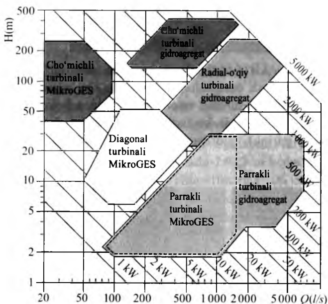
38-rasm. Kichik quvvatli turbinalar hamda mikroGESlarni tanlash diagrammasi.
