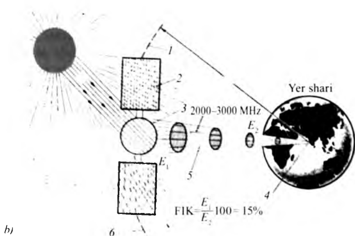
68-rasm. Yer sun'iy yo'ldoshiga o'rnatilgan quyosh elektrostansiyasining sxemasi: a – sxemasi; 1 – quyosh energiyasi oqimi; 2 – quyosh energiyasining sun'iy yo'ldosh kollektori; 3 – uzatuvchi antenna; 4 – qabul qiluvchi antenna; 5 – qisqa to'liqli nur; 6-energetik sun'iy yo'ldoshning doimiy orbitasi; b – sun'iy yo'ldoshga o'rnatilgan quyosh elektrostansiyasining umumiy ko'rinishi.
