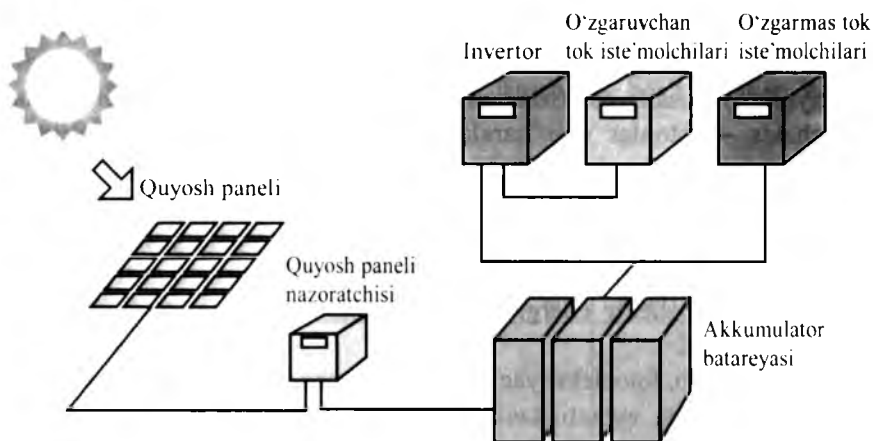
67-rasm. Quyosh batareyasidan elektr energiyasi olish sxemasi.
