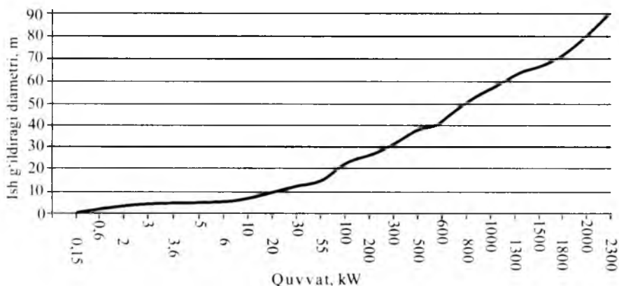
48-rasm. Shamol qurilmasi ish g'ildiragining diametri bilan uning quvvati orasidagi bog'lanish grafigi.
