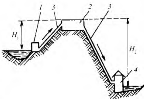
30-rasm. Suv bo'luvchi tepalikka o'rnatilgan hovuz suvi bilan ishlaydigan GAES sxemasi:
