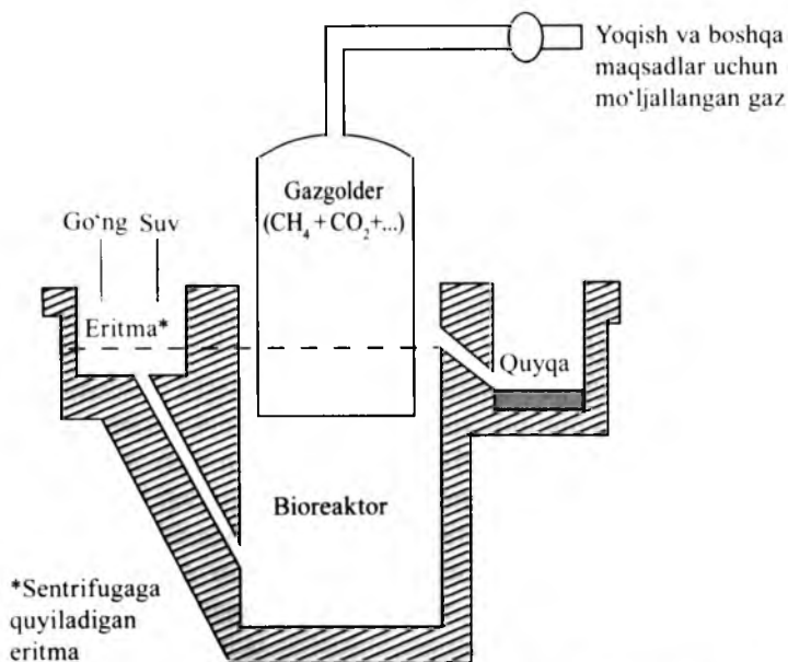
87-rasm. Biogaz reaktorining soddalashtirilgan sxemasi.
