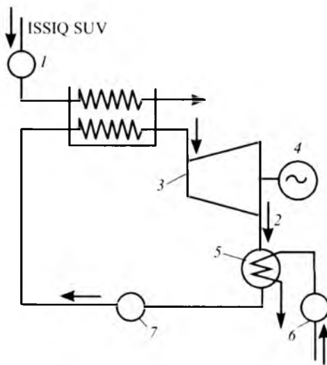
75-rasm. Okean issiqlik elektrostansiyasining sxemasi:
