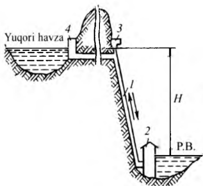
29-rasm. GAESning sxemasi:
