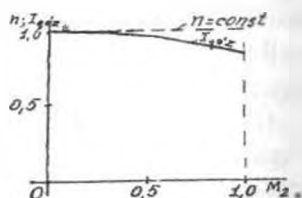
31.10-rasm. Parallel qo'zg'atishli motorning n=n_N=\text{const} va U=U_N=\text{const} bo'lgandagi I_{qz}=f(M_2) xarakteristikasi.
