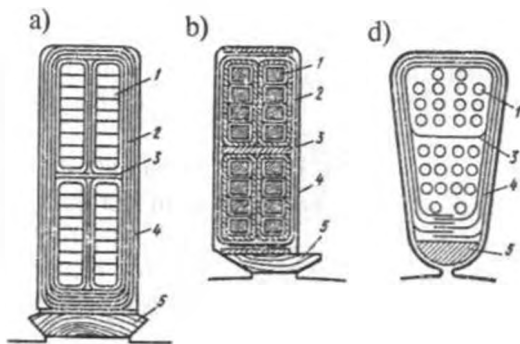
10.2-rasm. Statorning ochiq (a), yarim ochiq (b) va yarim yopiq (d) shaklli pazlari: 1 – o'tkazgichlar; 2 – qatlam izolatsiyasi; 3 – qatlamlararo isolatsiya; 4 – paz izolatsiyasi; 5 – pona.
