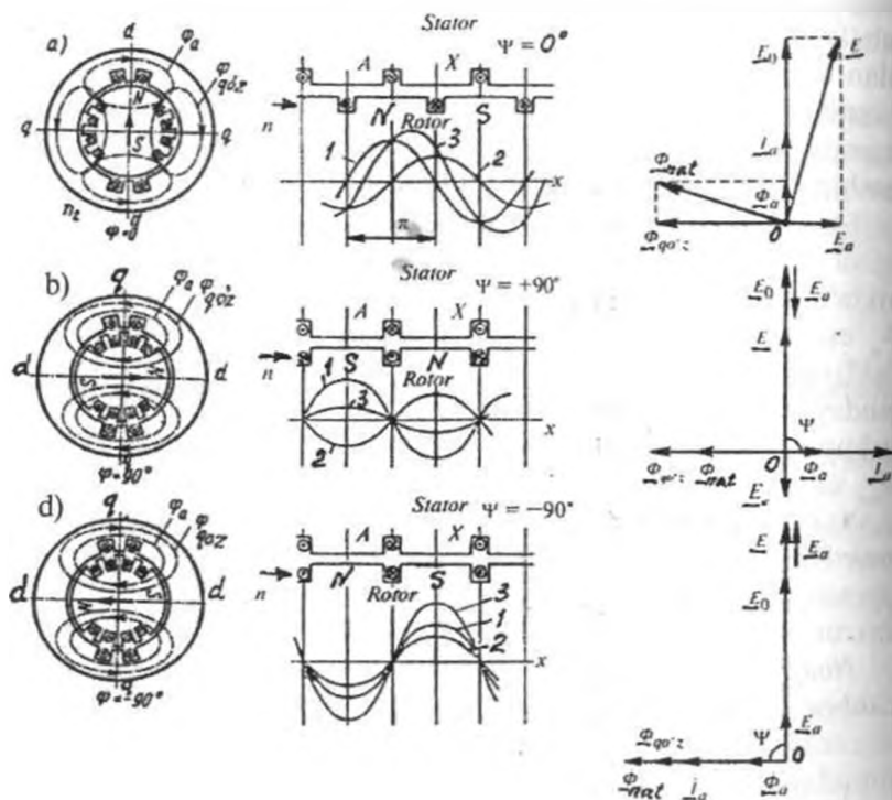
19.1-rasm. Noayon qutbli sinxron mashinada turli ( a — aktiv, b — induktiv va c — sig'imiyl) xarakterli yuklamadagi magnit oqimlar ( \Phi_{\varphi} — qo'zg'atish oqimi va \Phi_a — yakor reaksiyasi oqimi), magnit induksiyalari (1 — qo'zg'atish chulg'ami induksiyasi B_{\varphi} , 2 — yakor chulg'ami induksiyasi B_a va 3 — natijaviy induksiya B_{nat} ) ning taqsimlanish egri chiziqlari hamda vagnit oqimlar va EYKlarning vektor diagrammalari; \Phi_{nat} — natijaviy oqim.
