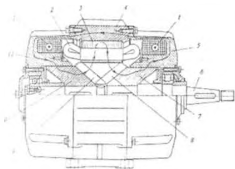
26.3-rasm. Rotori changalsimon qutblardan iborat bo'lgan kontaksiz sinxron generator, bunda: 1 – halqasimon qo'zg'atish g'altaklari; 2 – yakor chulg'ami; 3 – yakorning magnit o'tkazgichi; 4 – stanina (tana gardishi); 5, 11 – podshipnik qalqonlari; 6 – val; 7, 10 – janubiy va shimoliy qutblarning yarmosi; 8, 9 – janubiy va shimoliy qutblar.
