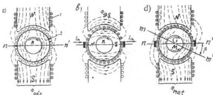
28.1-rasm. O'zgarmas tok mashinasining magnit maydoni: a) qo'zg'atish chulg'aming maydoni F ; 1 – qo'zg'atish chulg'ami, 2 – yakor; b) yakor chulg'aming maydoni F_a ; d) mashinaning natijaviy magnit maydoni F_{nat}
