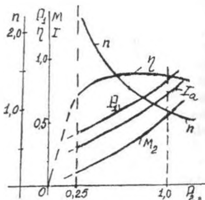
31.5-rasm. Ketma-ket qo'zg'atishli motorning foydali quvvat R_2 ga nisbatan olingan ish xarakteristikalari.
