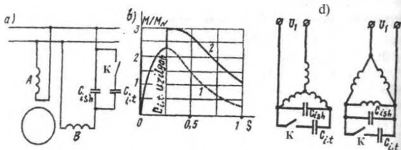
16.2-rasm. Kondensatorli asinxron motor sxemasi (a) va uning mexanik xarakteristikasi (b); uch fazali asinxron motorni bir fazali tarmoqdan ishlatishda stator chulg'omini ulash sxemalari(d); K — kalit.
