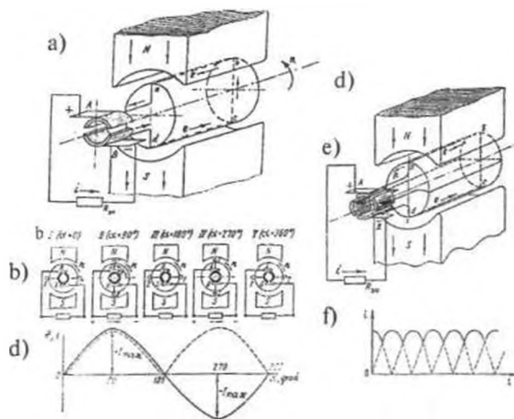
27.6-rasm. Yakor chulg'ami bitta o'ram (2 ta o'tkazgich)dan iborat bo'lgan eng oddiy o'zgarmas tok generatorining modeli (a); yakor bitta aylantirilganda o'tkazgichlarning magnit maydondagi holatlari (b) va o'zgarmas EYK (yoki tok) ning hosil bo'lishi (d); yakor chulg'ami fazoda bir-biriga nisbatan 90° da joylashgan ukkita o'ram (4 ta o'tkazgich)dan iborat bo'lganda (e), tashqi zanjirda EYK (yoki tok) pulsatsiyalanishining keskin kamayishi (f).
