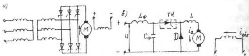
31.13-rasm. Boshqariladigan to'g'rilagichdan ta'minlanadigan mustaqil qo'zg'atishli motorning aylanish chastotasini rostlash sxemasi (a) va o'zgaras tok motorini impulsli rostlash (b): \alpha_f S_f — kirish filtri (tozalagichi); TK — tiristorli kalit; D — teskari diod; L_f — induktivlik.
