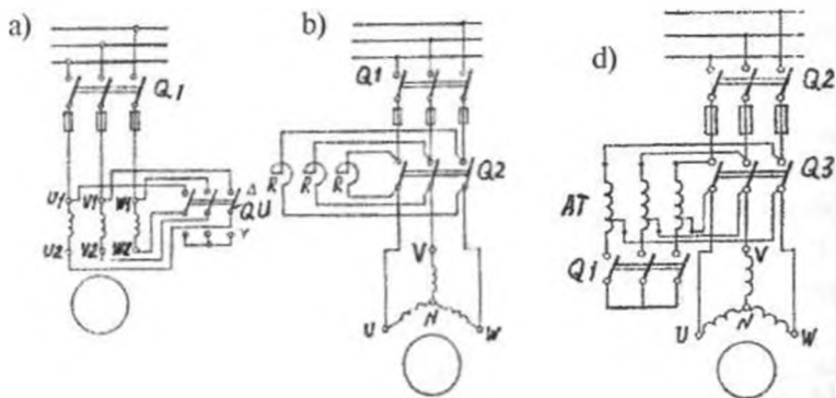
14.2-rasm. Tormoz kuchlanishini pasaytirib ishga tushirish sxemalari: stator chulg'omini yulduz ulanish sxemadan uchburchak ulanish sxemaga Yo'li bilan ishga tushirish (a); stator chulg'amiga reaktor R (reaktiv qarshilik) ulab (b) yoki AT — avtotransformator yordamida kuchlanishni pasaytirib (d) ishga tushirish sxemalari (hularda: QU — qayta ulagich; Q1, Q2 va Q3 — ishga tushirish kontaktorlari).
