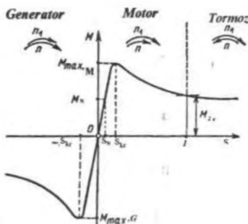
12.2-rasm. Asinxron mashinaning motor, generator va elektomagnit tormoz rejimlari uchun mexanik xarakteristikalari (a, b) — M = f(s) .
