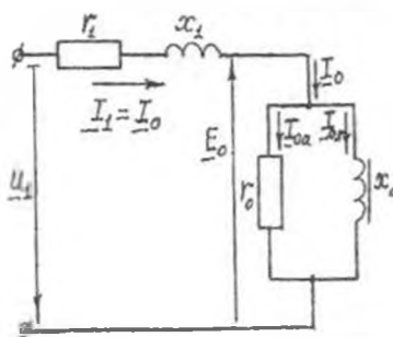
3.4-rasm. Transformatorning salt ishlash rejimi uchun almashtirish sxemasi.
