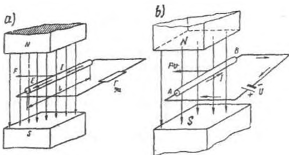
K.2-rasm. Elektr mashinalarida mexanik energiyaning elektr energiyaga (a) va elektr energiyaning mexanik energiyaga (b) aylantirilishiga oid chizmalar.
