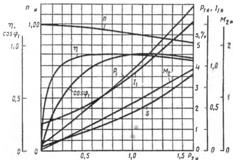
13.4-rasm. Quvvati 50 kW, 220/380 V, 1470 ayl./min bolgan qisqa tutashgan rotorli asinxron motorning ish xarakteristikalar.
