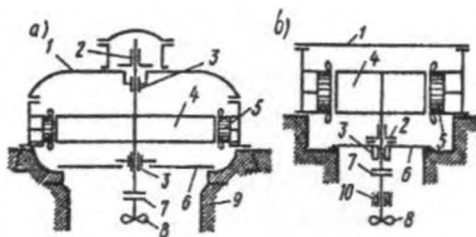
18.3-rasm. Gidrogeneratorlarning konstruktiv sxemalari — osma (a) va soyabon (b) tiplari:
