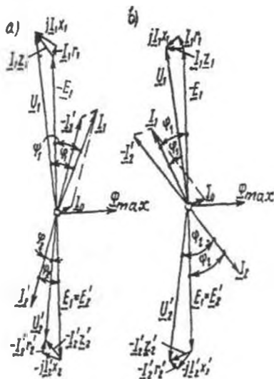
4.1-rasm. Transformatorning aktiv-induktiv (a) va aktiv-sig'imiyl (b) yuklamalar uchun vektor diagrammalari.
