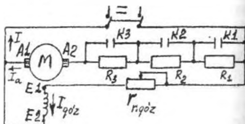
31.3-rasm. Avtomatlashtirilgan elektr yuritmasida parallel qo'zg'atishli O'TM ni ishga tushirishning prinsipl sxemasi.
