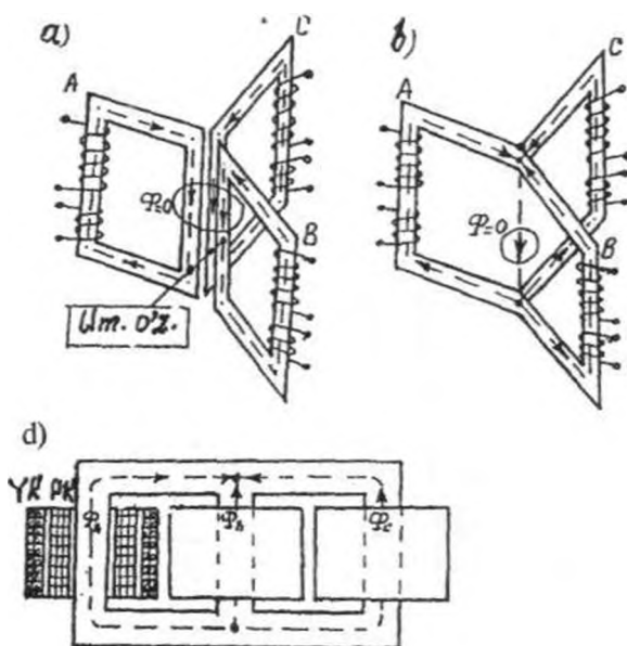
2.1-rasm. Magnit sistemasi umumiy bo'lgan uch fazali transformator konstruksiyasining hosil qilinishiga oid chizmalar:
