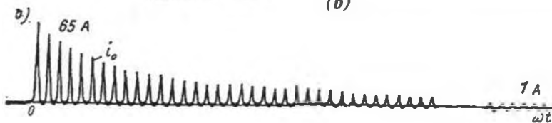
8.5-rasm. Yuklama ulanmagan o'rtta quvvatli bir fazali transformatorni elektr tarmog'iga bevosita qo'shish sxemasi (a) va bu jarayondagi tok ossillogrammasi (b)
