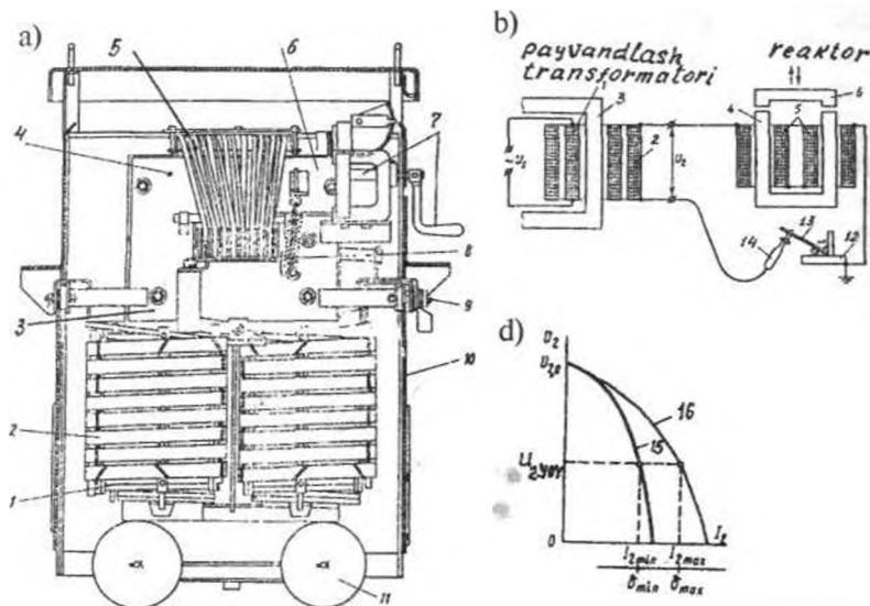
9.2-rasm. STN-500-1 tipli payvandlash transformatorining tuzilishi (a) va ishiniing prinsipial sxemasi (sxemada reaktor ajratib ko'rsatilgan) (b): [1, 2 – tegishli YK va PK chulg'amlar; 3 – magnit o'tkazgich; 4, 6 – reaktor magnit sistemasining qo'zg'almas (4) va qo'zg'aluvchi (6) qismlari; 5 – reaktor chulg'ami; 7 – qo'zg'aluvchi qismni harakatga keltirish uchun dastakli yurituvchi vint; 8 – qo'zg'aluvchi qismning titrashini kamaytirish uchun prujina; 9 – ikkilamchi chulg'am va reaktor chulg'ami qisqichi; 10 – kojux; 11 – g'ildirak; 12 – payvandlanadigan detal; 13 – elektrod; 14 – tokli simning izolatsion tutqichi]; payvandlash transformatorining tashqi xarakteristikalar (d): [minimal (1) va maksimal (2) zazorlar uchun; U_{2, \text{nom}} – elektr yoyining turg'un yonishi uchun zaruriy kuchlanish].
