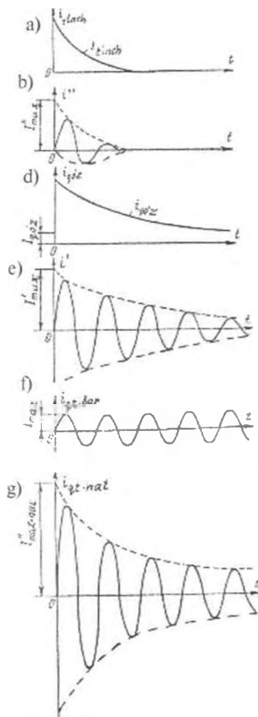
22.4-rasm. Sinxron generatorda to'saidan qisqa tutashuv toklari: a – tinchlantirish chulg'amdagi tok; b – bu tokning yakordagi tashkil etuvchisi; d – qo'zg'atish chulg'amidagi tok; e – bu tokning yakordagi tashkil etuvchisi; f – yakordagi barqaror qisqa tutashuv tok; g – yakordagi natijaviy qisqa tutashuv tok.
