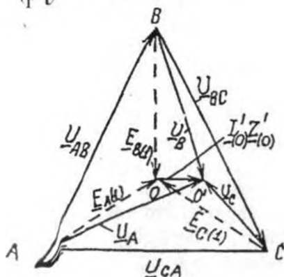
8.3-rasm. Chulg'amlari Y/Y_0 sxemaga ulanganda nol ketma-ketlikli toklarning ta'siridan transformator fazaviy kuchlanishlar sistemasining buzilishini ko'rsatuvchi vektor diagramma.
