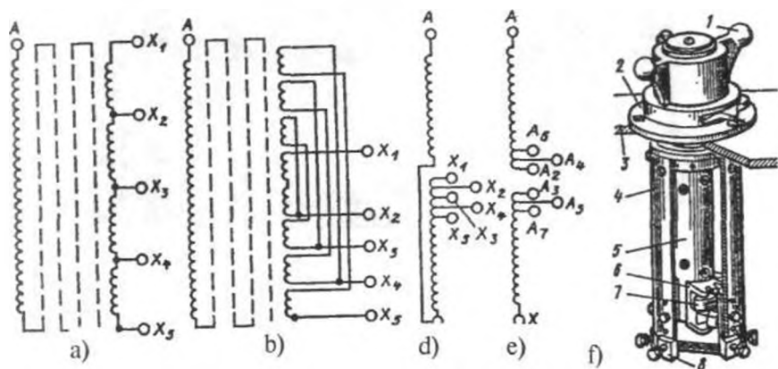
5.4-rasm. Yuqori kuchlanishli chulg'amda kuchlanishni rostdashning PBV turida shoxobchalarni bajarish sxemalari: a, b — ko'p qatlamli silindrik chulg'amlar uchun; d, e — ko'p qatlamli g'altakli silindrik va uzluksiz g'altakli chulg'amlar uchun; f — uch fazali qayta ulagich, bunda: 1 — yuritish dastagi; 2 — mahkamlash flanetsi; 3 — bak qopqog'i; 4 — qog'oz-bakelitli silindr; 5 — tayanch valning qog'oz-bakelitli izolyatsiyasi; 6 — tirsakli val; 7, 8 — qo'zg'aluvchi va qo'zg'almas kontaktlar.
