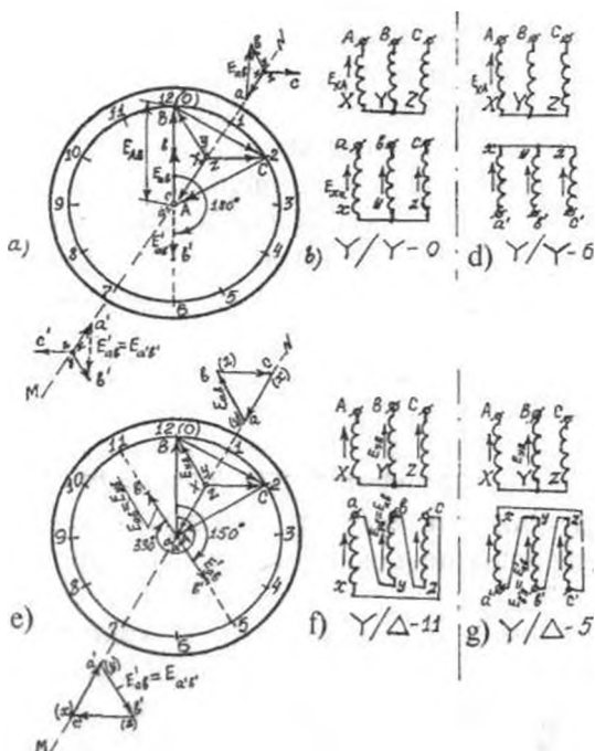
6.2-расм. «Yulduz-yulduz» (b, d) va «yulduz-uchburchak» (f, g) sxemalar uchun uch fazali transformator chulg'amlarining ulanish guruhini aniqlashga oid chizmalar (a, e).
