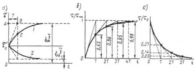
34.2-rasm. Umumiy hol uchun elektr mashinasida qizish (1) va sovish (2) jara-yonlarining vaqt bo'yicha o'zgarishi (a); \tau = 0 dan boshlab mashinaning qizishi (b); mashinaning 0^\circ\text{C} gacha sovish jarayonining vaqt bo'yicha o'zgarishi (c).
