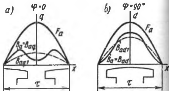
19.2-rasm. Ayon qutbli sinxron mashinaning ko'ndalang (a) va bo'yлама r'qlari bo'yicha yakor MYK larining hamda ular hosil qilgan magnit ksiyalarining taqsimlanish egri chiziqlari.
