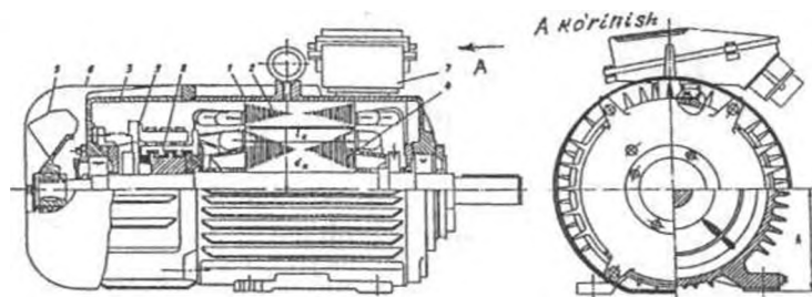
32.4-rasm. 4PO seriyali o'zgaras tok motorining bo'ylama va ko'ndalang qirgimlari:
