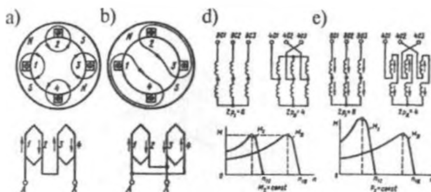
14.7-rasm. Stator faza chulg'aming qutblar sonini o'zgartirish uchun qayta ulash sxemasi: a — 2p = 4 da va b — 2p = 2 da uch fazali asinxron motor qutblar sonini qayta ulash sxemalari hamda uning aylantiruvchi sxemasi M = \text{const} ( d ) va aylanish chastotasi n = \text{const} ( e ) rejimlarida mexanik xarakteristikalari.
