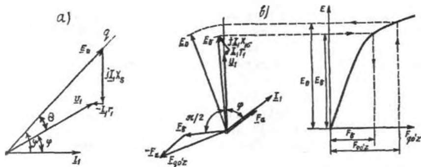
19.5-rasm. Noayon qutbli SG ning aktiv-induktiv xarakterli yuklamadagi vektor diagrammalari: a – magnit zanjirining to'yinishi hisobga olinmagan hol uchun; b – magnit zanjirining to'yinish darajasi hisobga olingan hol uchun; \underline{E}_{ad} – natijaviy magnit oqim F_{ad} ning mashina bo'ylama o'qi bo'yicha tashkil etuvchisi F_{ad} hosil qilgan EYK.
