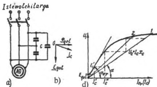
15.3-rasm. O'z-o'zini qo'zg'atishli asinxron generator(a), vektor diagramma (b) va AG ning o'z-o'zini qo'zg'atish jarayonini tushuntirishga oid(d).
