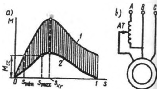
14.8-rasm. Asinxron motorga beriladigan uch fazali kuchlanish sistemasi simmetrikligini o'zgartirib aylanish chastotasini rostlashda mexanik xarakteristika (a), (bunda: 1 — simmetrik va 2 — nosimmetrik kuchlanishlarda) hamda b — tarmoqqa ulash sxemasi.
