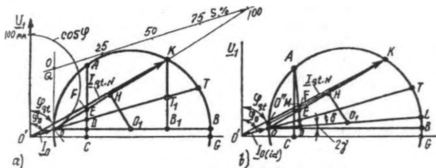
13.3-rasm. Asinxron motorninig soddalashgan (a) va aniqlashtirilgan (b) doiraviy diagrammalarini salt ishlash va qisqa tutashuv tajribalari ma'lumotlari bo'yicha qurish; \underline{I}_{0(id)} — ideal salt ishlash toki
