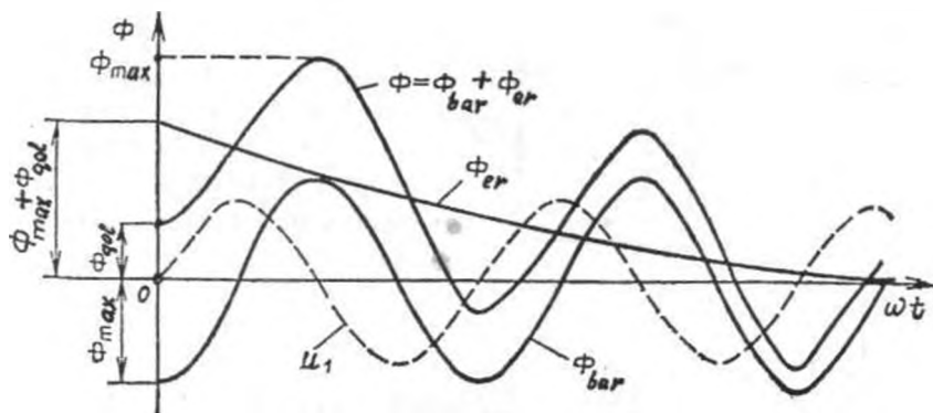
8.6-rasm. Nominal kuchlanish bilan ishlayotgan transformatorning ikkilamchi chulg'ami to'satdan qisqa tutashgandagi tokning vaqt bo'yicha o'zgarish grafigi.
