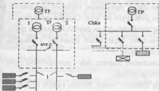
5.6-rasm. I toifali avariya yoritishni ta'minlash sxemasi.
