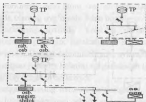
5.5-rasm. Avariya yoritishning bir transformatorli ta'minoti.
