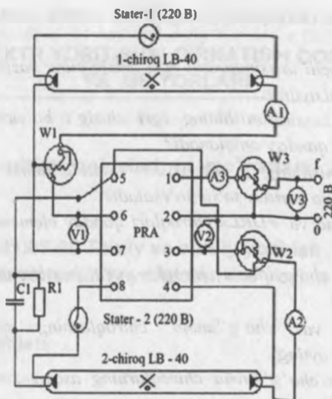
3.7-rasm. Ikki yoritgichli bir fazali ta'minotga ulangan lyuminescent chiroqlarning (2x20 W) antistroboskopik ulanish sxemasi.
