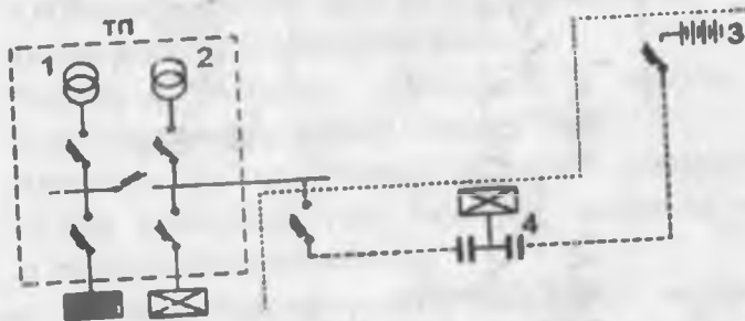
5.7 - rasmi. "O'zgacha" toifali avariyaaviy yoritishni ta'minlash sxemasi.
