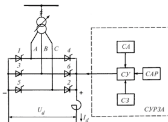
28-rasm. O'zgartiruvchi ko'priknining sxemasi
