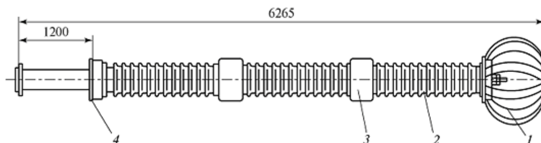
23-rasm. 500 kV kuchlanishli moy toʻldirilgan kabellarning tugallovchi muftalarining konstruksiyasi.
