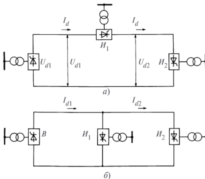
31-rasm. Oraliqda O'TUdan quvvat olish sxemasi:
