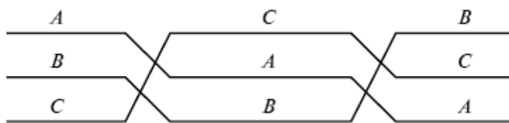
8-rasm. HL A, V, S fazalarining transpoziziya sikli.
