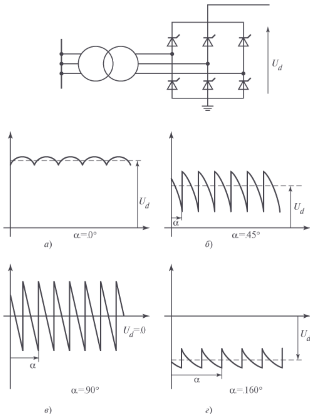
32-rasm. Rostlash burchagining turli qiymatlaridagi ko‘priknining to‘g‘rilangan kuchlanish qiymatlari; a, b – to‘g‘rilagich rejimi; v – inventar rejimiga o‘tish chegarasi; g – inventar rejimi
