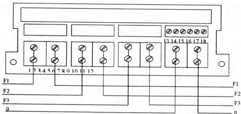
4.3-rasm. «Energiya – 9» CTK3-10A1HXR.VU hisoblagichi klemmlarining joylashishi.
