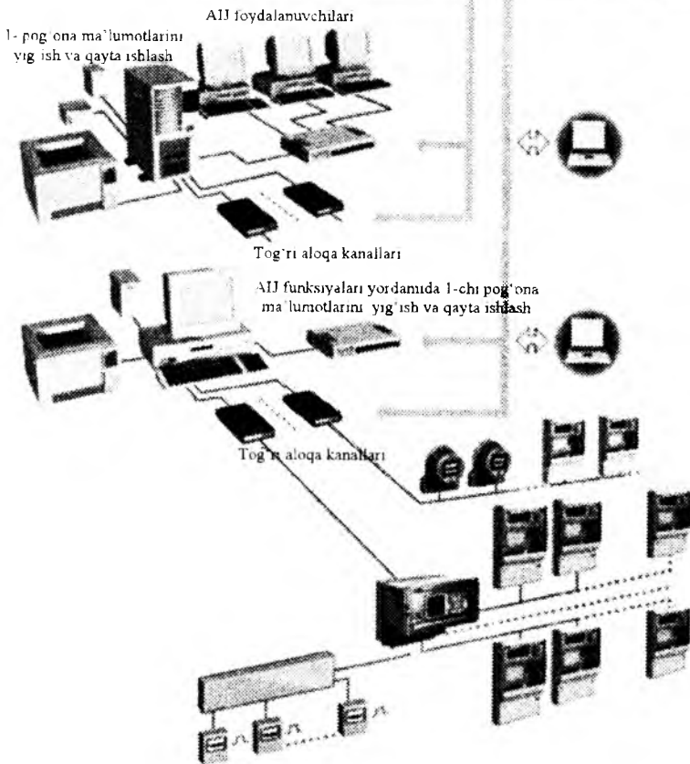
2.5-rasm. O'rta va yirik quvvatli sanoat korxonalari yoki energetika tizimi uchun ko'p pog'onali ENHAT ni tashkil etish.
