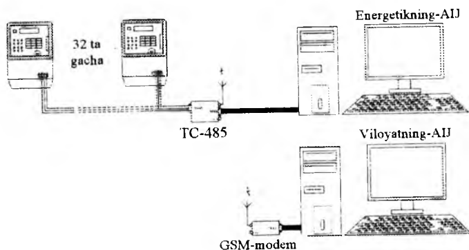
1.5-rasm. Ma'lumotlarni uzatish moduli asosidagi ENHAT
