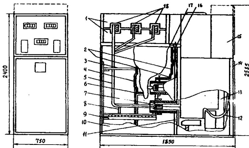
10.2-rasm. 3200 A li uzgichli KRU -KE- 10 shkafi;
