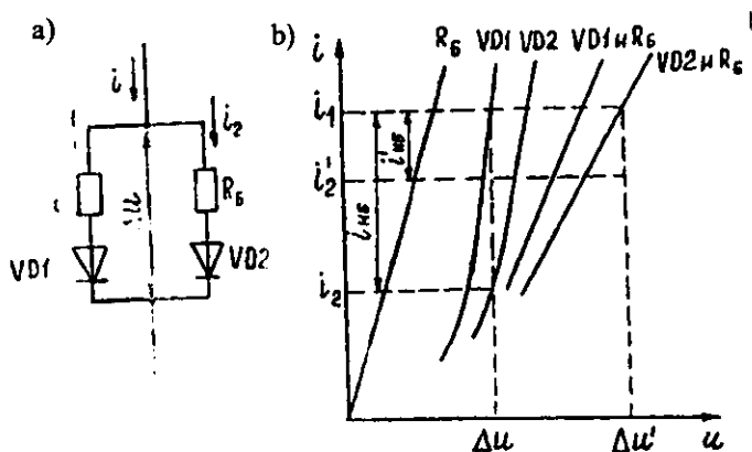
9.17-rasm. Ventillarni rezistor bilan ulanish sxemasi (a) va volt-amper tafsifi (6).
