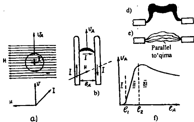
4.11-rasm. Magnit maydonidan elektr yoyining harakati (a–g); parallel elektrodlarda yoy harakati tezligining elektrod oralaridagi masofaga bog'liqligi.
