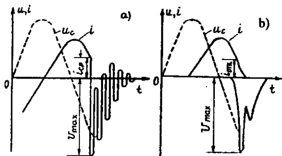
5.4-rasm. Moyli uzgich (a) va elektromagnitli uzgich (b) yordamida kichik qiymatli induktiv yuklama uzilganda tok va kuchlanishlarning o'zgarishi: i_{sr} — qir qish toki; U_{max} — o'takuchlanish amplitudasi.
