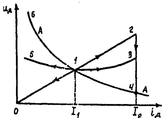
4.9-rasm. Yoyni statik va dinamik tavsiflari.
