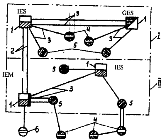
1.1-rasm. Energetik tizim: 1 — elektrstansiyalari; 2 — tizimlarni bog'lovchi elektr uzatish liniyalari; 3 — tizimning ichki bog'lovchi liniyalari; 4 — nimstansiyalar; 5 — tuman nimstansiyalari; 6 — loyihalananayotgan tortish nimstansiyalari.
