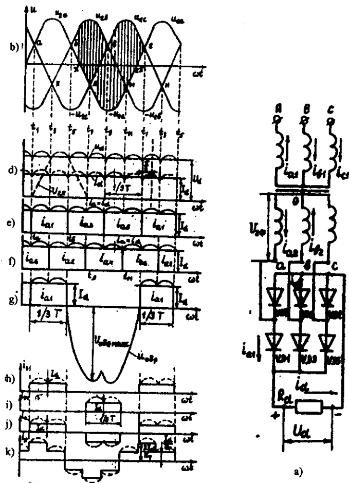
9.21-rasm. Uch fazali ko'prik sxemali to'g'irlagich (a) va undagi elektromagnit jarayonlar: b — uch fazali kuchlanish; d — to'g'irlangan kuchlanish.
