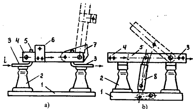
7.1-rasm. Vertikal aylanuvchi ajratgichlar konstruktiv sxemasi: 1—rama; 2— tayanch izolatori; 3—shinalar ulanadigan boshmoqlar; 4 —pichog (qo'zg'aluvchi kontakt); 5—qo'zg'almas kontakt; 6—tezkor shtanga «qulog'i»; 7—pichog harakatini cheklovchi tirgak; 8— izolatsiyali tortish.
