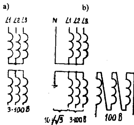
9.11-rasm. Uch fazali kuchlanish transformatorlarining ulanish sxemalari: a — uch oʻzakli magnit oʻtkazgichli transformator; b — toʻrt yoki besh oʻzakli magnit oʻtkazgichli transformator; ikkilamchi chulgʻamlarning bir guruhi ochiq uchburchak shaklida ulangan (kuchlanishning nol ketma-ketligini oʻlchash uchun).
