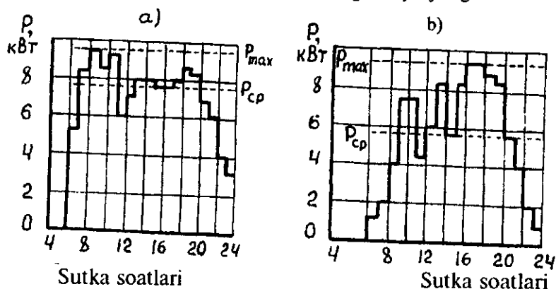
1.2-rasm. Elektr iste'molchilari ishlarining asosiy rejim grafiklari.
