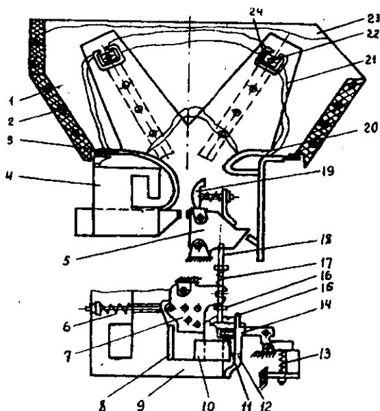
6.8-rasm. VAT—42 turidagi uzgichning yoy so'ndirgich kamerasi: 1—yoy so'ndirgich kamera; 2—yonbosh ulagich; 3,20,24 — elektrodlar (shoxchalar); 4—asosiy qo'zg'almas kontakt; 5 —asosiy qo'zg'aluvchi kontakt; 6—uzuvchi prujina; 7,11—yakor; 8,15 —tirkak,9 — magnit o'tkazgich; 10—g'altak; 12 —magnit o'tkazgich qisqich; 13 — prujina; 14 — zashyolka; 16 —richag; 17 —qaytuvchi prujina; 18—tortgich; 19 —yoy so'ndirgich kontakt; 21—to'siqlar; 22—P—simon magnit o'tkazgich; 23—shchitlar.
