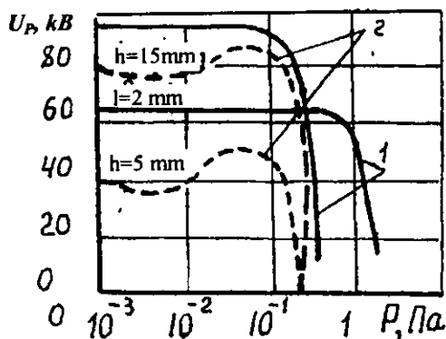
5.18-rasm. Vakuum oraliq'i elektr puxtaligining qoldiq gazlar bosimiga bog'liqligi: 1 – bir jismli maydondagi razryad (elektrodlar kislorodsiz misdan bo'lib, oraliq'i 1 ga teng); 2 – pleksiglas silindr yuzalaridagi razryad (silindr diametri 25 mm va balandligi h ga teng, ular bir jinsli maydonda nikellangan elektrodlar orasiga joylashgan).
