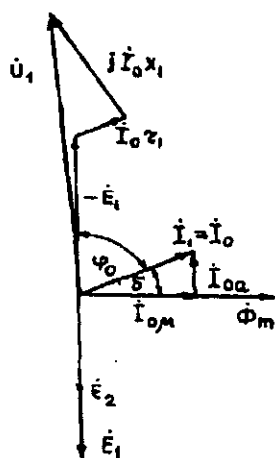
9.4-rasm. Transformatorning salt ishlashdagi vektor diagrammasi.
