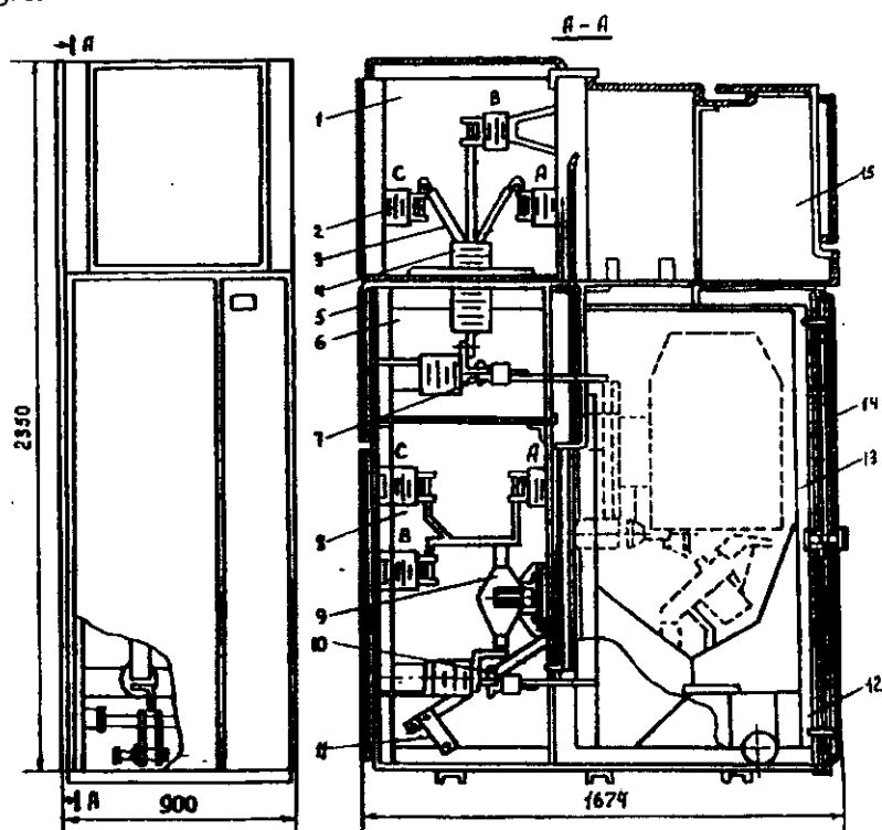
10.1-rasm. Elektr magnitli uzgich BEM-10Eli shkaf KRU-2 a 10E/E: 1 — yig'ma shinalar hujrasi; 2 — tayanch izolatori; 3 — yig'ma shinalar; 4 — o'tuvchi izolator; 5 — olinadigan qopqoq; 6 — asosiy kontakt zanjiri olinuvchi yuqori hujra; 7, 10 — yuqori va pastki asosiy kontaktlar; 8 — liniyaviy hujra; 9 — tok transformatori; 11 — yerlatuvchi ajratgich; 12 — shkaf korpusi; 13 — olinadigan element; 14 — fasad eshigi; 15 — rele shkafi.
