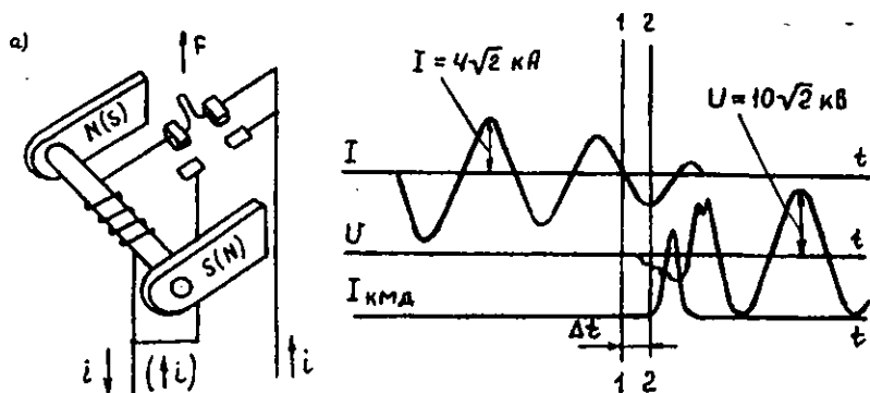
5.9-rasm. Yoyni magnit maydoni bilan o'zaro ta'siri sxemasi (a) va elektromagnitli uzgich bilan g'altak uzilganda tok va kuchlanish ossillogrammalari (b).
