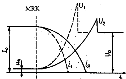
4.3-rasm. O'zgaras tok uzilganda tok va kuchlanishlar grafiklari.
