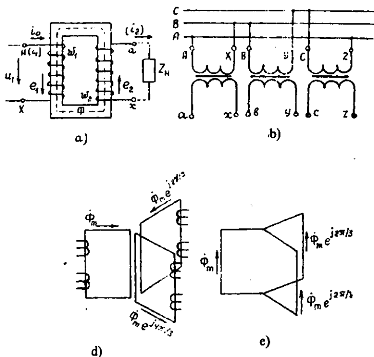
9.1-rasm. Transformatorning ishlash tamoyili: a—bir fazali taransformator; b—uch fazali guruh va g-uch fazali guruhdan yulduz—Y ko‘rinishli magnit o‘tkazgichga o‘tish.
