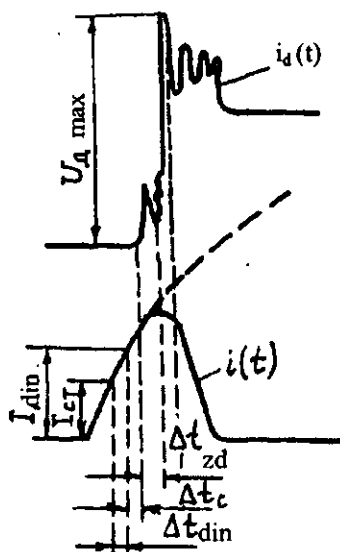
6.11-rasm. VAT—42 ( I_{nom} = 6300 A) turidagi uzgichning tok va kuchlanish ossillogrammalari.
