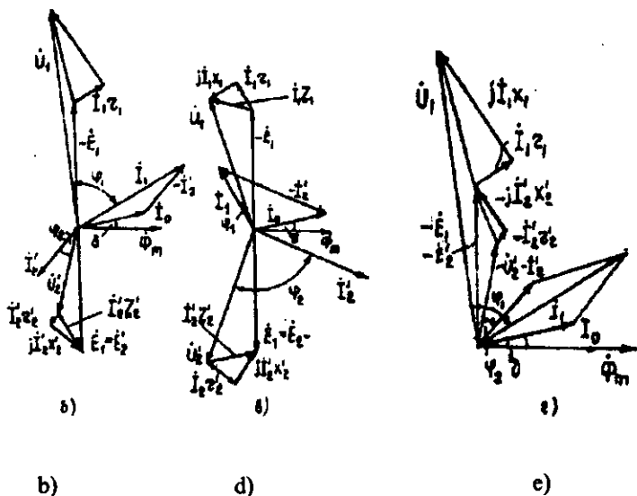
9.6-rasm. Transformatorning ekvivalent sxemasi (a), potensial (e) va vektor diagrammalari: b — aktiv induktiv yuklama uchun; d — aktiv sig'ım yuklama uchun.
