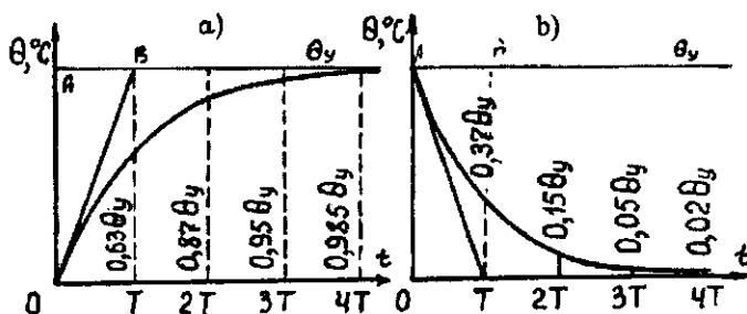
1.10-rasm. O'tkazgichning vaqt birligida qizish va sovush holatlarini aniqlovchi grafiklar: a – qizish; b – sovush.
