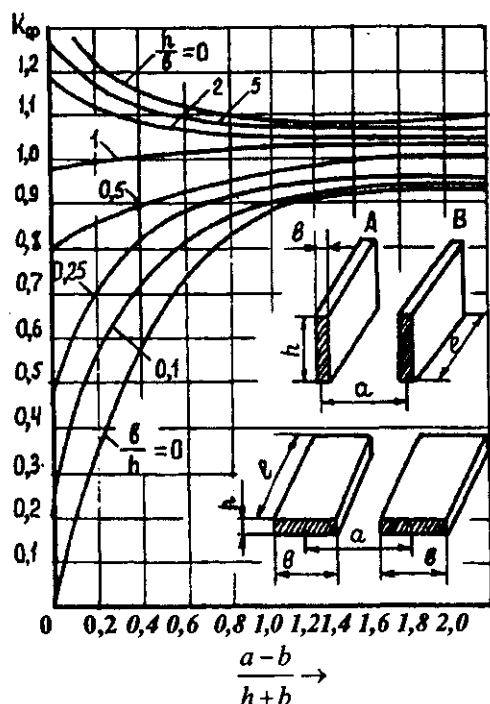
2.9-rasm. Shakl koeffitsiyenti K_\phi ni o'tkazgichning ko'ndalang kesim yuzasi o'lchamlariga bog'liqligi.
