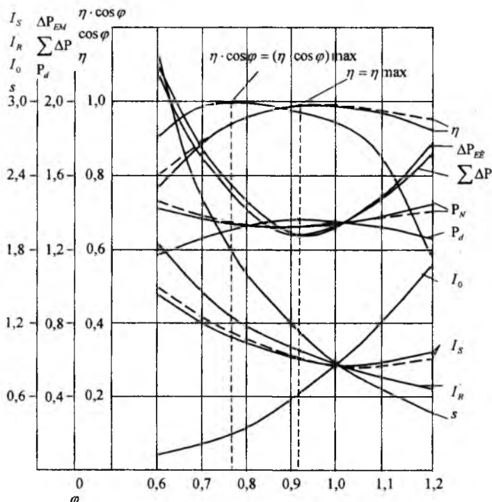
3.1- rasm. Tezligi chastotani o'zgartirib rostlanadigan elektr yuritmadagi 4A rusumidagi asinxron motorning chastota qiymati F = 1 bo'lgandagi elektrik va energetik ko'rsatkichlarining magnit oqimi o'zgarishiga bog'liq tavsiflari
