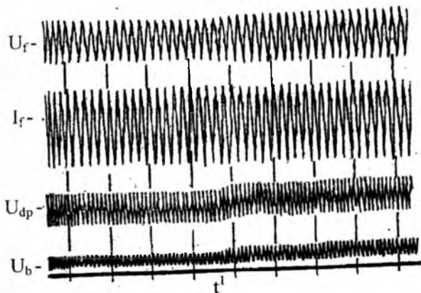
5.2-rasm. Boshqaruv signali musbat qiymatli chastotasi rostlanadigan elektr yuritmaning energiya tejamlar ish rejimlari ossillogrammalari
