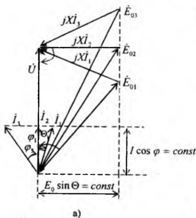
2.6-rasm. Sinxron elektr motorning vektor diagrammasi (a) va U ko'rinishdagi tavsifi (b)
