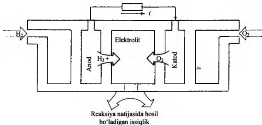
2.10-rasm. Yoqilg'i elementining ishlash sxemasi
