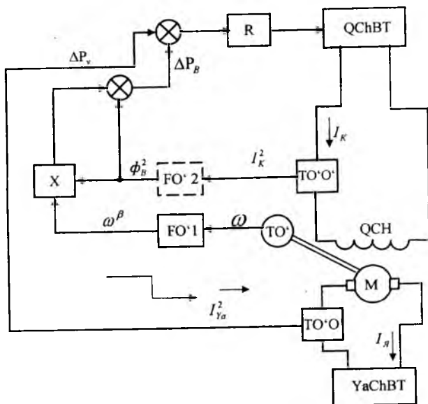
3.1 -rasm. Tarkibida toklarning qiymatini kvadratga o'zgartiruvchi o'lchov o'zgartkichi bo'lgan o'zgaras tok elektr yuritmasining tizim sxemasi
