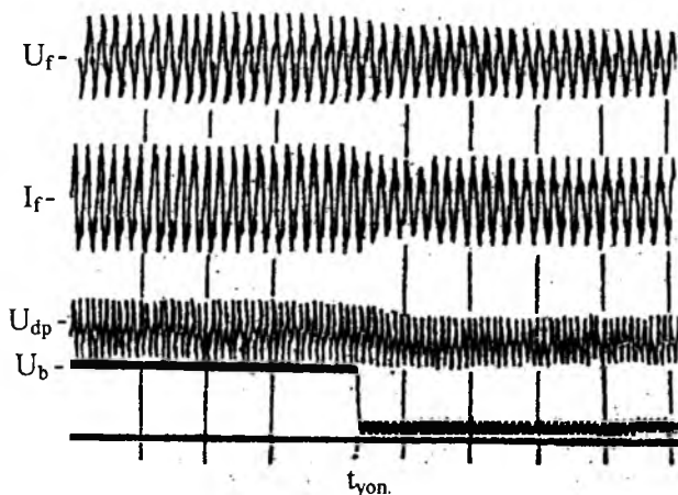
5.1-rasm. Boshqaruv signali manfiy qiymatli chastotasi rostlanadigan elektr yuritmaning energiya tejamlar ossillogrammalari
