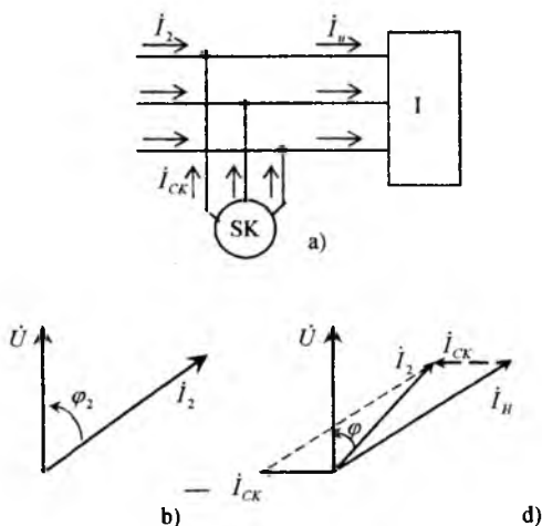
2.9-rasm. Iste'molchi va sinxron kompensatorlarning ulanish sxemasi: (a), kompensatsiyagacha (b) va kompensatsiyadan so'ngi (d) vektor diagrammalari
