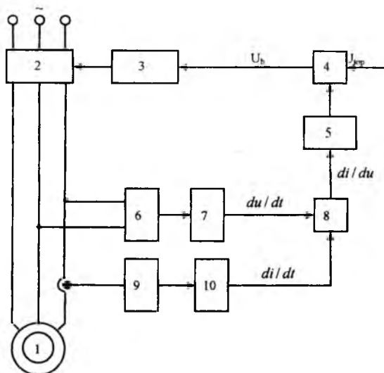
5.3-rasm. Kontrolyorli energiya tejakor asinxron elektr yuritmaning blok sxemasi
