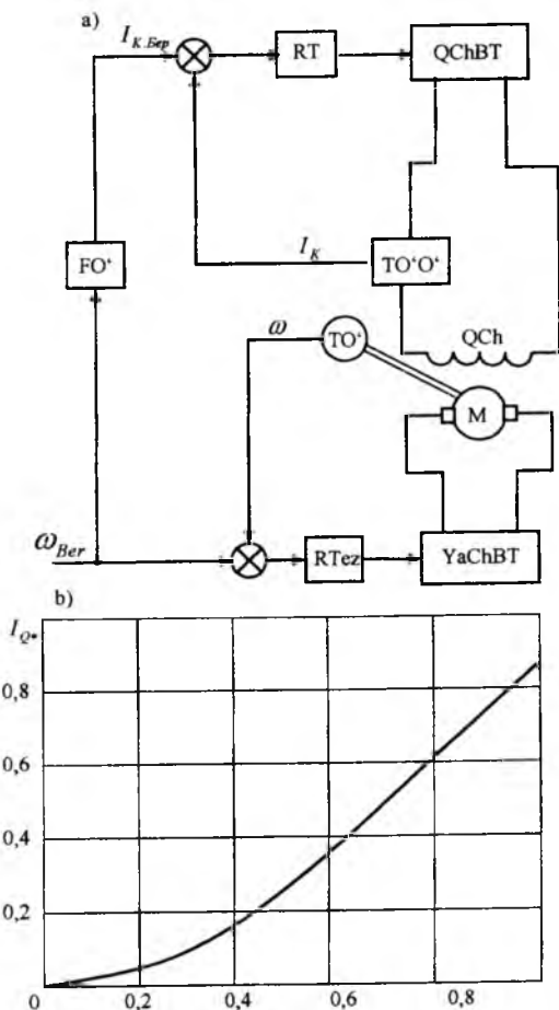
3.3-rasm. Ventilatorli yuklanishli mexanizmning oʻzgarmas tok elektr yuritmasi:
