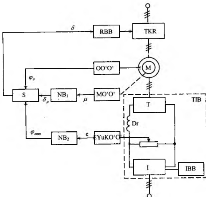
4.3-rasm. Energetik ko'rsatkichlari yaxshilangan energiya tejamlor asinxron-ventilli kaskad
