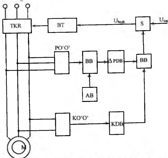
4.5-rasm. Energiya tejamkor asinxron elektr yuritmaning blok sxemasi
