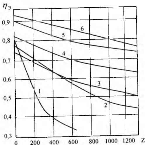
2.1-rasm. Kran elektr yuritmalarining ekvivalent FIK lari:
