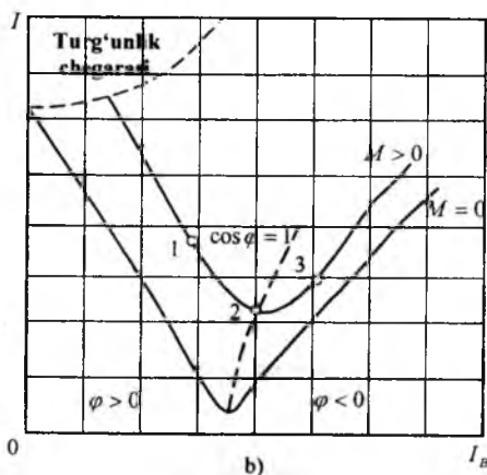
2.6-rasm. Sinxron elektr motorning vektor diagrammasi (a) va U ko'rinishdagi tavsifi (b)
