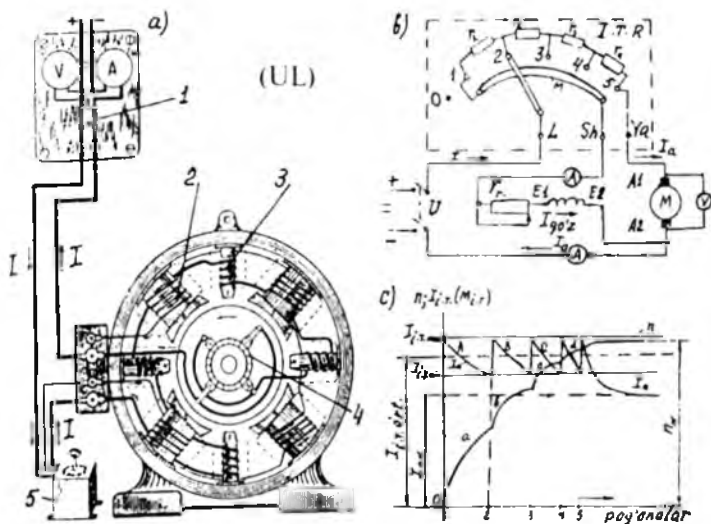
31.2-rasm. Parallel qo'zg'atishli o'zgarmas tok motorda: a – tajriba o'tkazish qurilmasi (bunda: 1 – ulab uzgich (UL); 2 – qo'zg'atish chulg'ami; 3 – qo'shimcha quth chulg'ami; 4 – kollektor; 5 – ishga tushirish reostati); b – motorni ishga tushirish sxemasi (ITR – ishga tushirish reostati, M – mis yoyi); d – «reostatli» ishga tushirish jarayonidagi tok, moment va aylanish chastotalarining o'zgarish xarakteri.
