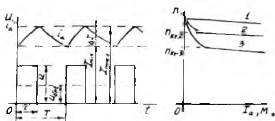
31.14-rasm. O'TM ing aylanish chastotasini impulsli rostlashda kuchlanish va toklarning (zgarish grafigi (a) va parallel qo'zg'atishli rotorni impulsli rostlashda tizlik va mexanik xarakteristikalar (b).
