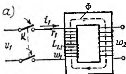
8.5-rasm. Yuklama ulanmagan o'rta quvvatli bir fazali transformatorni elektr tarmog'iga bevosita qo'shish sxemasi (a) va bu jarayondagi tok ossillogrammasi (b)
