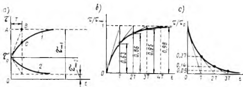
34.2-rasm. Umumiy hol uchun elektr mashinasida qizish (1) va sovish (2) jara-yonlarining vaqt bo'yicha o'zgarishi (a); \tau = 0 dan boshlab mashinaning qizishi (b); mashinaning 0^\circ\text{C} gacha sovish jarayonining vaqt bo'yicha o'zgarishi (c).
