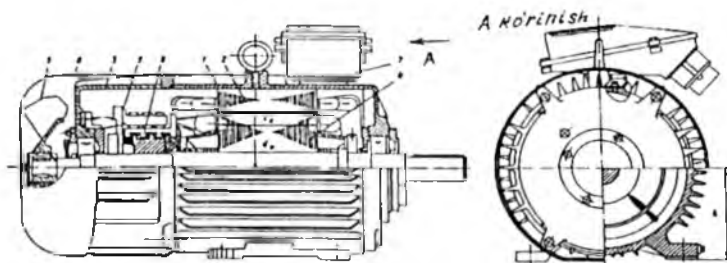
32.4-rasm. 4P seriyali o'zgarmas tok motorining bo'ylama va ko'ndalang qirg'irlari:
