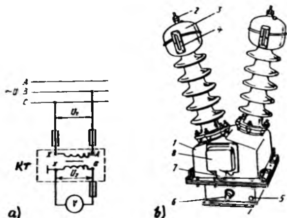
9.5-rasm. Kuchlanishi 35 kV bo'lgan tarmoqqa mo'ljallangan NOM-35 tipli kuchlanish transformatorini tarmoqqa ulash sxemasi (a) va uning tashqi ko'rinishi (b): (1 – korpus; 2 – yuqori kuchlanishli tarmoqdan ulanadigan sim uchun qisqich; 3 – o'tish izolatorining kengaytirgichi; 4 – moy ko'rsatkich; 5 – zaminlash uchun bolt; 6 – moyni to'kish uchun tiqinli teshik; 7 – ikkilamchi chulg'am uchlari chiqarilgan izolatsion taxtachaning qopqog'i va 8 – o'lchash asboblari sim ulash uchun shtutser (uchlariga rezba ochilgan biriktiruvchi qism); KT – kuchlanish transformatori.
