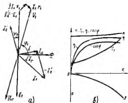
15.1-rasm. Asinxron generatorning vektor diagrammasi (a) va ish xarakteristikalari (b).
