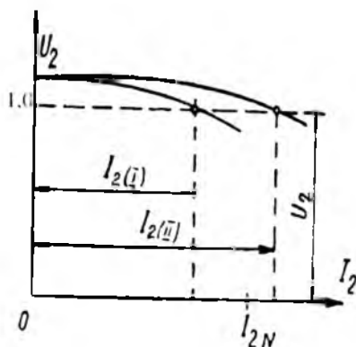
6.7-rasm. Qisqa tutashuv kuchlanishlari bir xil bo'lmagan holda parallel ishlayotgan ikkita transformatorning tashqi xarakteristikalar yordamida yuklama taqsimlanishini aniqlash.
