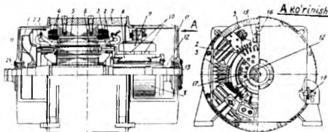
31.1-rasm. Umumiy maqsadli P seriyaga mansub bo'lgan o'zgarmas tok motori:
