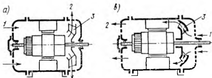
34.4-rasm. Mashinada qizigan havoni soʻrib kor-pusdan tashqariga chiqaruvchi (a) va sovituvchi havoni mashina ichiga haydovchi (b) ventilatsiya sistemalari: 1 – kiruvchi havo; 2 – chiquvchi havo; 3 – ventiliator.
