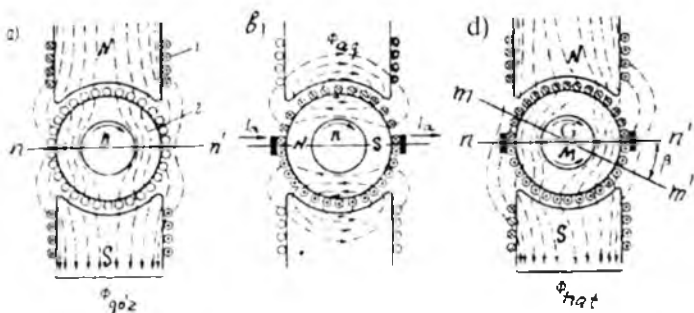
28.1-rasm. O'zgarmas tok mashinasining magnit maydoni: a) qo'zg'atish chulg'amingining maydoni F_{az} ; 1 – qo'zg'atish chulg'ami, 2 – yakor; b) yakor chulg'amingining maydoni F_a ; d) mashinaning natijaviy magnit maydoni F_{nat}
