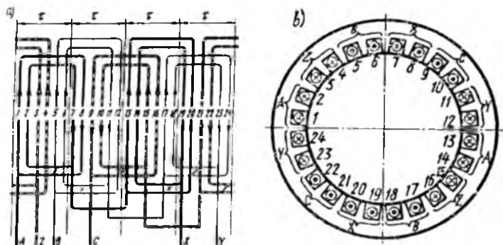
10.6-rasm. Uch fazali bir qatlamli konsentrik chulg'am sxemasi ( Z=24 , 2p=4 , q=2 , a=1 ) (a) va statorda g'altaklarning joylashishi (b).
