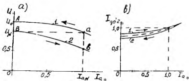
30.3-rasm. Mustaqil qo'zg'atishli o'zgarmas tok generatorining tashqi (a) va rostlash (b) xarakteristikalari.
