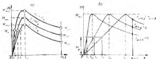
12.5-rasm. Kuchlanish nominaldan farqli bo'lganda (a)da juol rotorli asinxron motor rotor chulg'ami aktiv qarshiligining har xil qiymatlarida (b) mexanik xarakteristikalar
