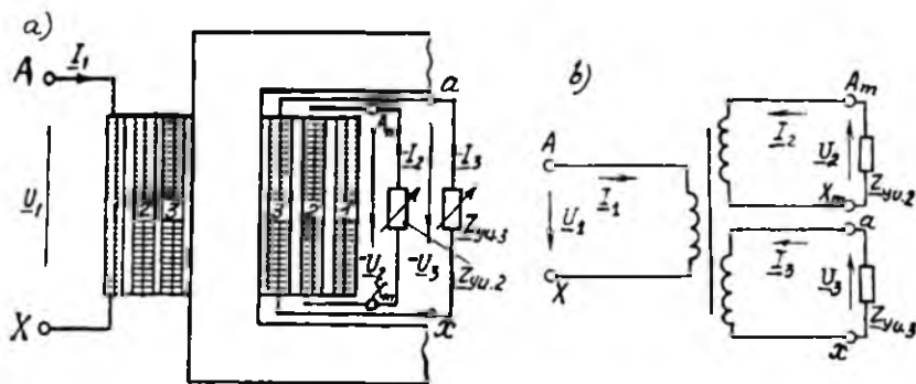
7.1-rasm. Uch chulg'amli pasaytiruvchi transformator o'zagida chulg'amlarning joylashirilishi (a) va prinsipial sxemasi (b).
