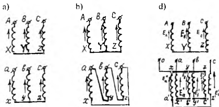
2.6-rasm. Uch fazali transformatorlar chulg'amlarining ulanish usullari: a – yulduz–yulduz (Y/Y); b – yulduz–uchburchak (Y/ \Delta ); d – yulduz–zigzag (Y/Z).
