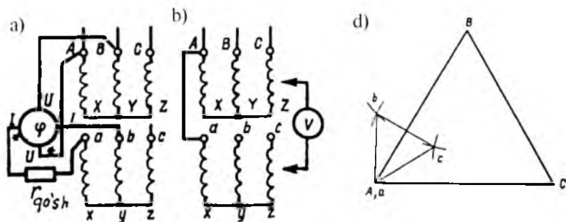
6.4-rasm. Transformorning ulanish guruhini tajriba yo'li bilan fazometr (a) va voltmetr (b) usullarida aniqlash sxemalari; d – tajribaviy-grafik usuli uchun diagramma qurish.
