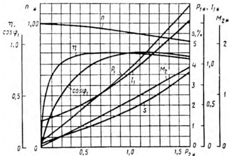
13.4-rasm. Quvvati 50 kW, 220/380 V, 1470 ayl./min boʻlgan qisqa tutashgan rotorli asinxron motorning ish xarakteristikalari.
