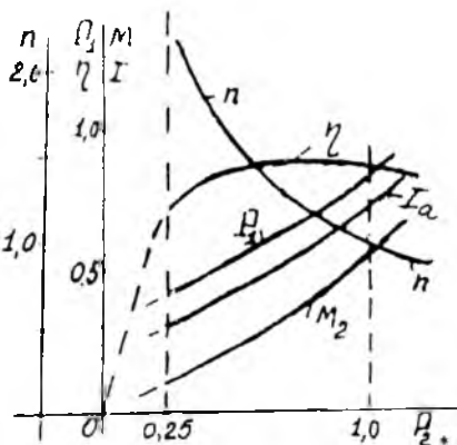
31.5-rasm. Ketma-ket qo'zg'atishli motorning foydali quvvat P_2 ga nisbatan olingan ish xarakteristikalari.
