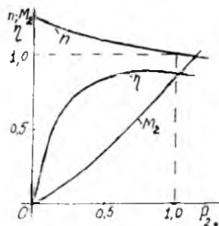
31.6-rasm. Mos ulangan aralash qo'zg'atishli motorning ish xarakteristikalarini (asosiy chulg'am - parallel qo'zg'atishli, qo'shimcha chulg'am - ketma-ket qo'zg'atishli).
