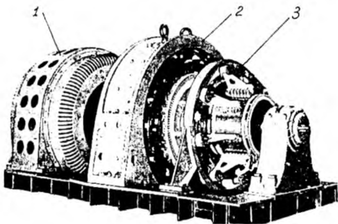
V.1-rasm. Quvvati 1000 kW, U = 250 V, I_n = 4000 A, n=750 ayl/min bo'lgan tayanch podshipnikli o'zgarmas tok generatori (ishlatishga o'rnatilgan holati): 1 — birlamchi motor; 2 — generator; 3 — cho'ikali qurilma.
