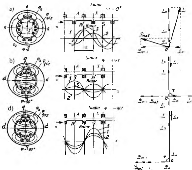
19.1-rasm. Noayon qutbli sinxron mashinada turli (a – aktiv, b – induktiv va c – sig'imiyy) xarakterli yuklamadagi magnit oqimlar ( \Phi_{qo'z} – qo'zg'atish oqimi va \Phi_n – yakor reaksiyasi oqimi), magnit induksiyalari (1 – qo'zg'atish chulg'ami induksiyasi B_{qo'z} , 2 – yakor chulg'ami induksiyasi B_n va 3 – natijaviy induksiya B_{nat} ) ning taqsimlanish egri chiziqlari hamda vagnit oqimlar va EYKlarning vektor diagrammalari; \Phi_{nat} – natijaviy oqim.
