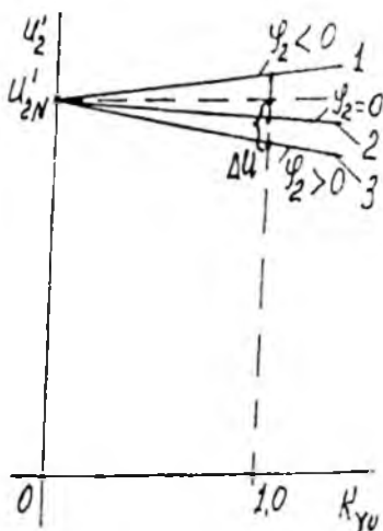
5.3-rasm. Transformatorning tashqi xarakteristikalari: 1 – aktiv-sig‘imiy; 2 – aktiv; 3 – aktiv-induktiv yuklamalar uchun.
