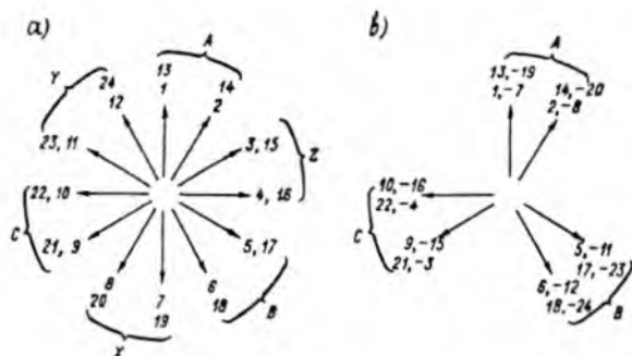
10.9-rasm. 10.8-rasmda tasvirlangan chulg'amning pazlardagi o'tkazgichlar EYK lari (a) va g'altaklar EYK lari yulduzlari (b).
