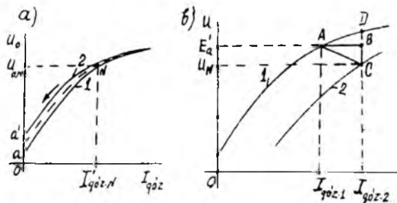
30.1-rasm. Mustaqil qo'zg'atishli o'zgarmas tok generatorining salt ishlash (a) va yuklanish (b) xarakteristikalari.
