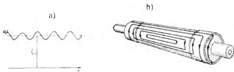
21.2-rasm. Sinxron generatorning nosimmetrik yuklamasida qo'zg'atish chulg'ami tokining o'zgarish shakli (a) va turbogenerator rotorida teskari ketma-ketlik maydoni hosil qilgan toklar o'tadigan yo'llar sxemasi (b).
