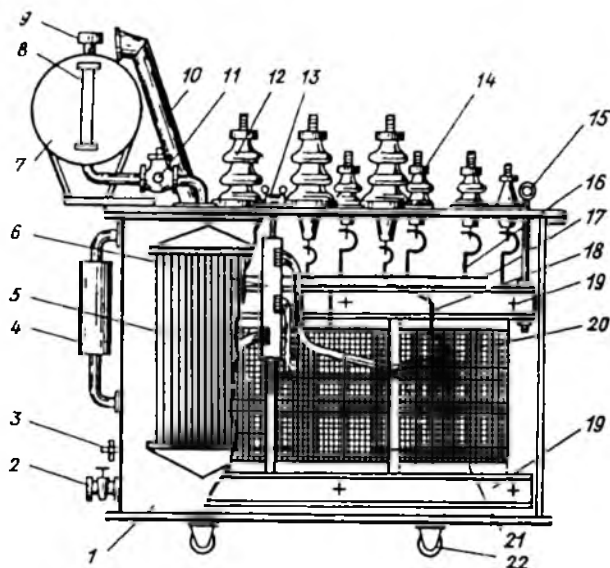
1.1-rasm. Kuchlanish klassi 35 kV quvvati 1000÷6300 kV·A konstruktsiyasiga mos keladigan pasaytiruvchi kuch transformatori:
