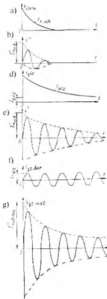
22.4-rasm. Sinxron generatorda to'satdan qisqa tutashuv toklari: a – tinchlantirish chulg'amidagi tok; b – bu tokning yakordagi tashkil etuvchisi; d – qo'zg'atish chulg'amidagi tok; e – bu tokning yakordagi tashkil etuvchisi; f – yakordagi barqaror qisqa tutashuv tok; g – yakordagi natijaviy qisqa tutashuv tok.
