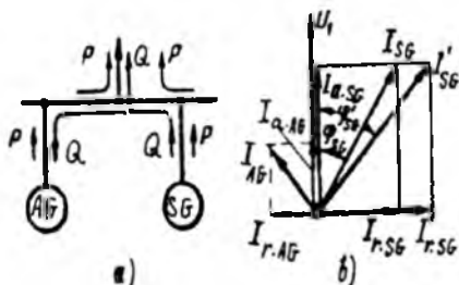
15.2-rasm. Asinxron va sinxron generatorlarning parallel ishlashi (a) va vektor diagrammasi (b); Q – reak.quvvat.
