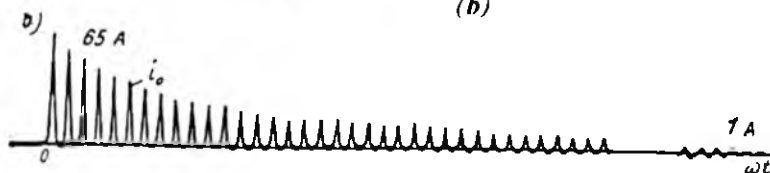
8.5-rasm. Yuklama ulanmagan o'rta quvvatli bir fazali transformatorni elektr tarmog'iga bevosita qo'shish sxemasi (a) va bu jarayondagi tok ossillogrammasi (b)
