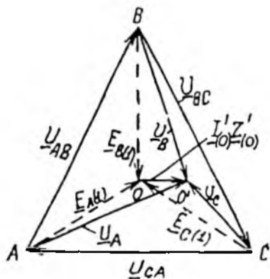
8.3-rasm. Chulg'amlari Y/Y_0 sxemaga ulanganda nol ketma-ketlikli toklarning ta'siridan transformator fazaviy kuchlanishlar sistemasining buzilishini ko'rsatuvchi vektor diagramma.
