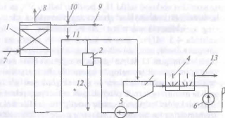
15.2- rasm. O'txona gazlarini oltingugurt oksidlaridan tozalash chizmasi (ohakli usul):
