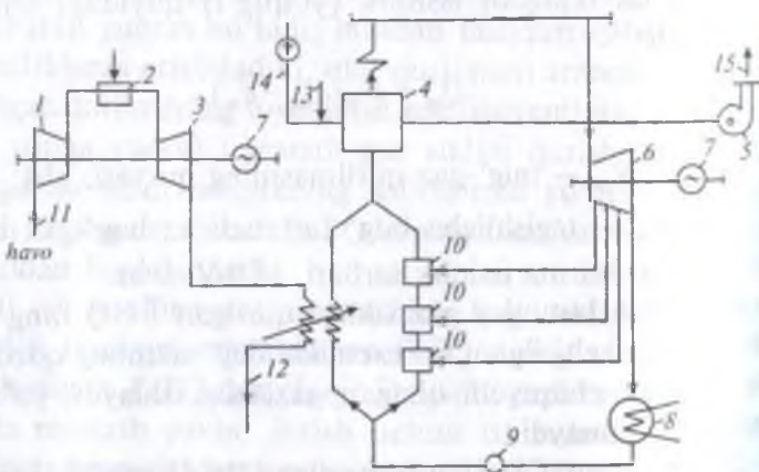
6.4- rasm. Bug' sikli ustiga gaz sikli qurilgan BGQ ning sxemasi: 1—kompressor; 2—yonish kamerasi; 3—gaz turbinasi; 4—bug' qozoni; 5—tutun tortkich; 6—bug' turbinasi; 7—elektr generatori; 8—kondensat; 9—ta'minlash nasosi; 10—regenerativ isitkichlar; 11—havo olish; 12—gazlar atmosferaga; 13—qozonga yoqilg'i berish; 14—havo berish; 15—tutun gazlari atmosferaga.
