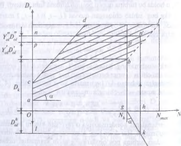
4.3- rasm. Ikki marta bug' olinadigan turbinaning ish holatlari diagrammasi.
