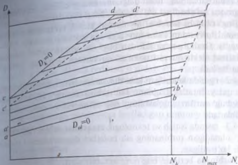
4.2- rasm. Bir marta bug' olinadigan kondensatorli turbinaning ish holatlari diagrammasi.
