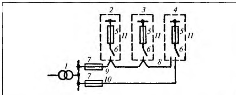
Рис. 2.3. Принципиальная схема электроснабжения жилых домов высотой до 5 этажей с резервной перемычкой:
