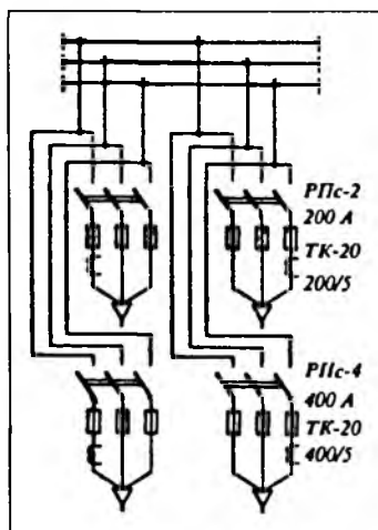
Рис. 3.4. Схема панели распределительного щита на четыре линии с рубильниками и предохранителями на напряжение 0,4 кВ
