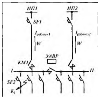
Рис. 4.19. Защита сети расцепителями автоматических выключателей
