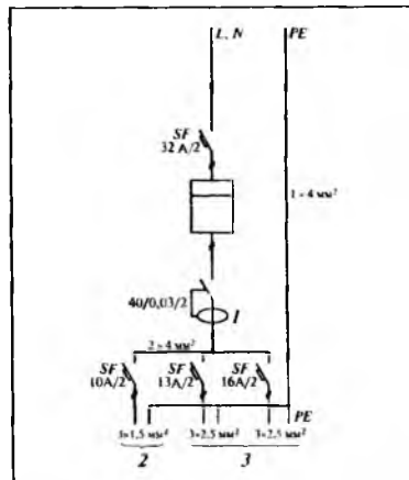
Рис. 4.13. Схема электроснабжения квартиры с газовой плитой с рекомендуемыми сечениями медных проводников (TN-S):
