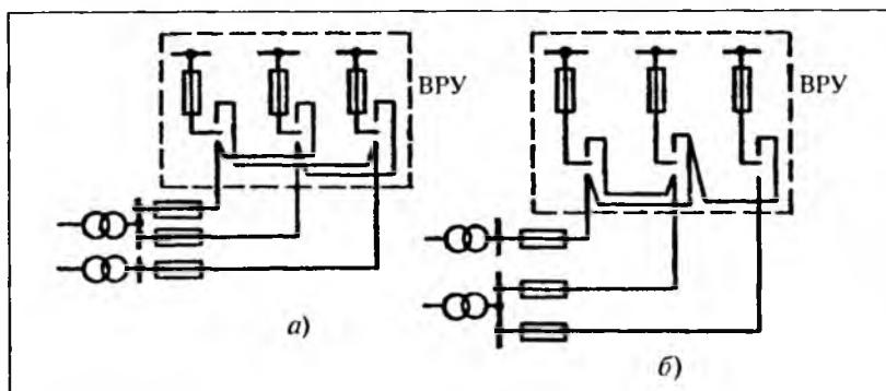
Рис. 2.6. Принципиальная схема электроснабжения жилых домов высотой 9 – 16 этажей с тремя вводами:
