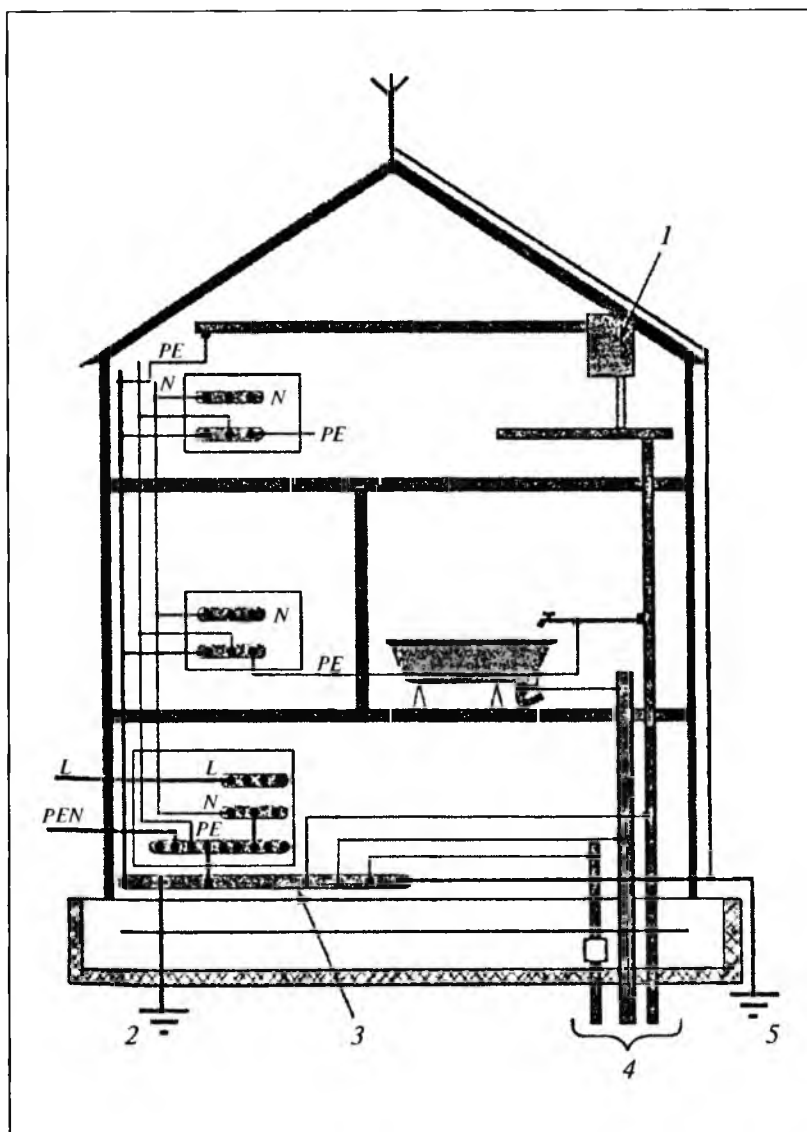
Рис. 4.5. Пример выполнения уравнивания потенциалов в электроустановке здания с системой TN-C-S :
