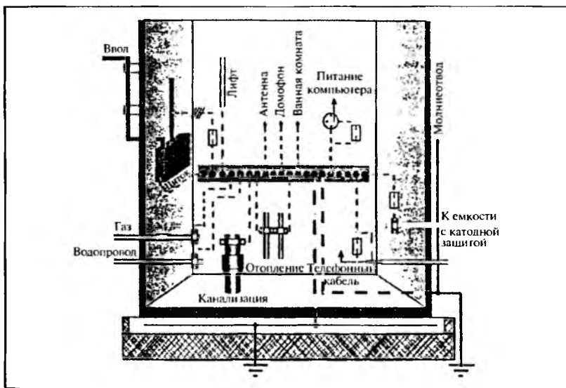
Рис. 4.4. Пример выполнения системы выравнивания потенциалов
