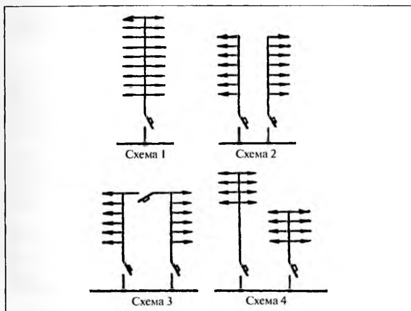
Рис. 2.8. Принципиальные схемы стояков, рекомендуемые по экономическим соображениям
