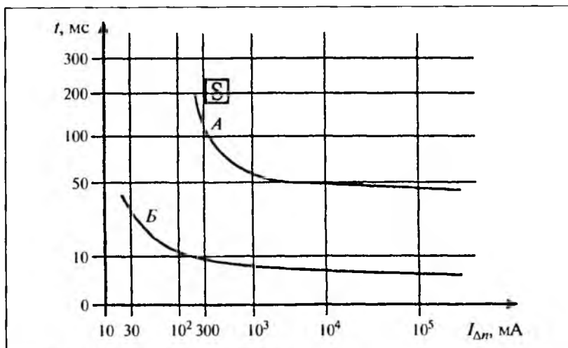
Рис. 4.16. Времятоковые характеристики УЗО:
