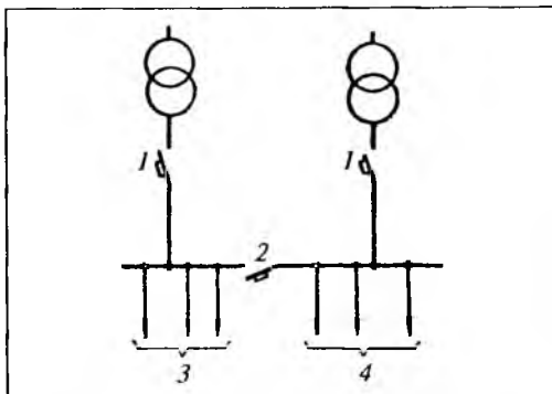
Рис. 2.12. Принципиальная схема электроснабжения общественного здания с встроенной ТП и абонентским щитом с АВР на автоматических выключателях:
