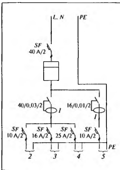
Рис. 4.8. Принципиальная схема электроснабжения квартиры с системой TN-S:
