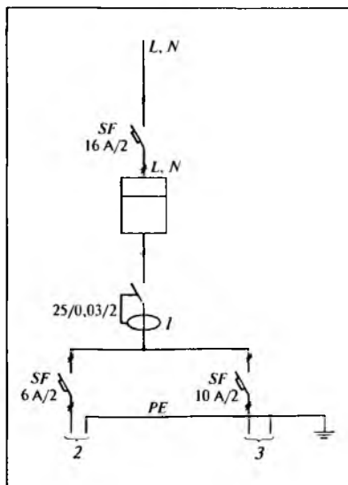
Рис. 4.9. Принципиальная схема электроснабжения мобильного здания с системой заземления TT:
