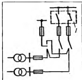
Рис. 2.7. Принципиальная схема электроснабжения жилых домов высотой 17 этажей и более:
