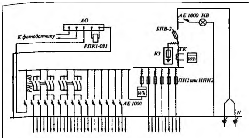
Рис. 3.3. Схема панели ВРУ на напряжение 0,4 кВ
