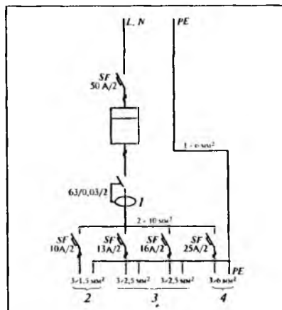
Рис. 4.12. Схема электроснабжения квартиры с электроплитой с рекомендуемыми сечениями медных проводников (TN-S):
