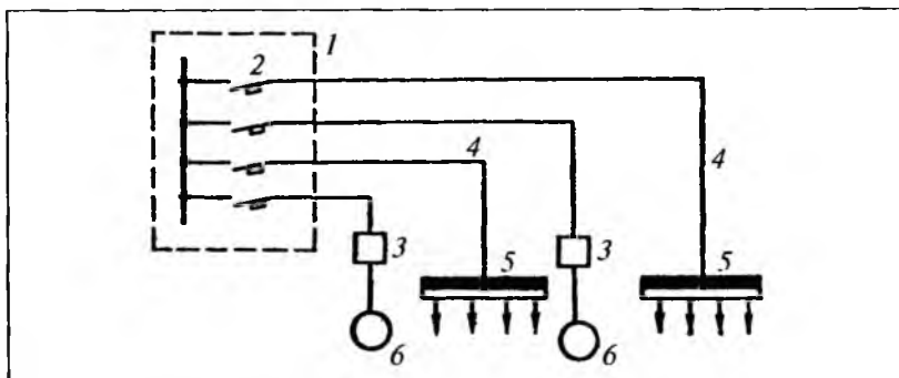
Рис. 2.1. Радиальная схема силовой сети:
