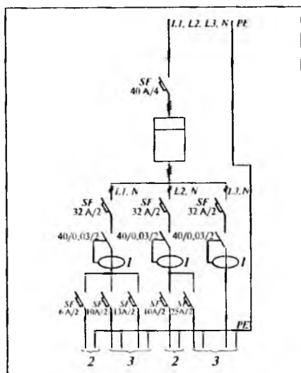
Рис. 4.10. Принципиальная схема электроснабжения здания с трехфазным вводом: 1 — УЗО; 2 — цепь освещения; 3 — розеточные цепи
