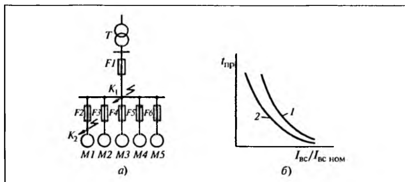
Рис. 4.18. Защита предохранителями радиальной сети с односторонним питанием
