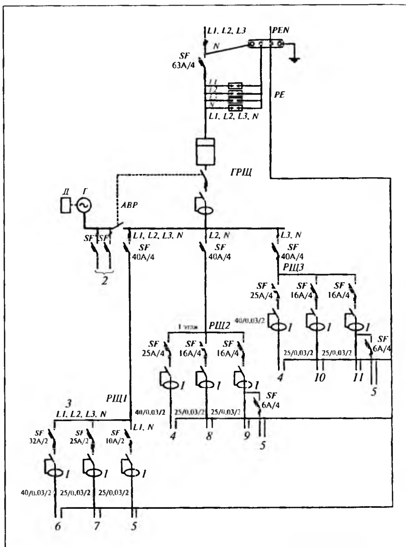
Рис. 4.15. Схема электроснабжения коттеджа с системой TN-C-S . При большом количестве групповых цепей рекомендуется применение этажных распределительных щитов — РЩ1, РЩ2, РЩ3, а также применение защиты от грозовых перенапряжений — ОПН:
