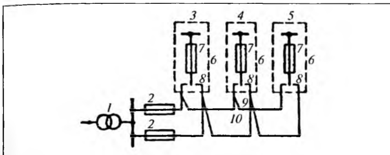
Рис. 2.4. Принципиальная схема электроснабжения жилых домов высотой до 5 этажей с переключателями на вводах:
