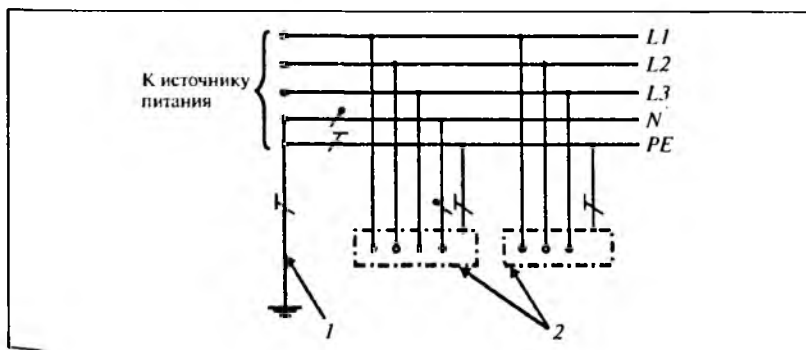
Рис. 4.3. Система TN-S переменного тока:
