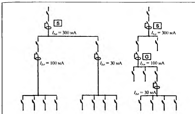
Рис. 4.17. Примеры схем с двумя и тремя уровнями селективности
