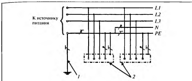
Рис. 4.2. Система TN-C-S переменного тока:
