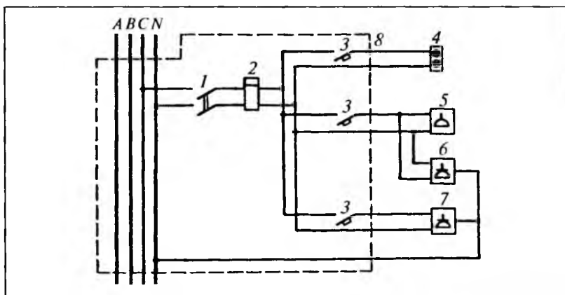
Рис. 2.9. Принципиальная схема групповой квартирной сети:
