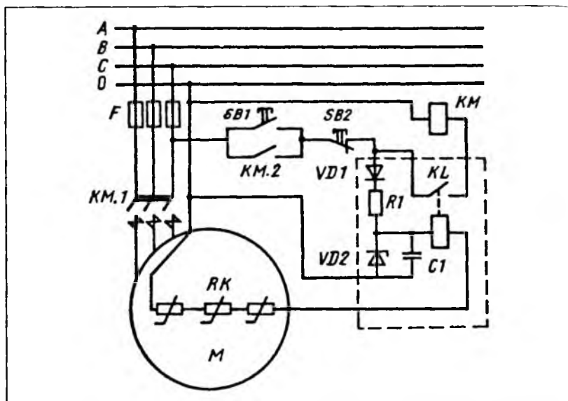
Рис. 3.2. Принципиальная схема температурной защиты электродвигателя напряжением до 1 кВ типа УВТЗ-2 с использованием терморезистора (позистора):
