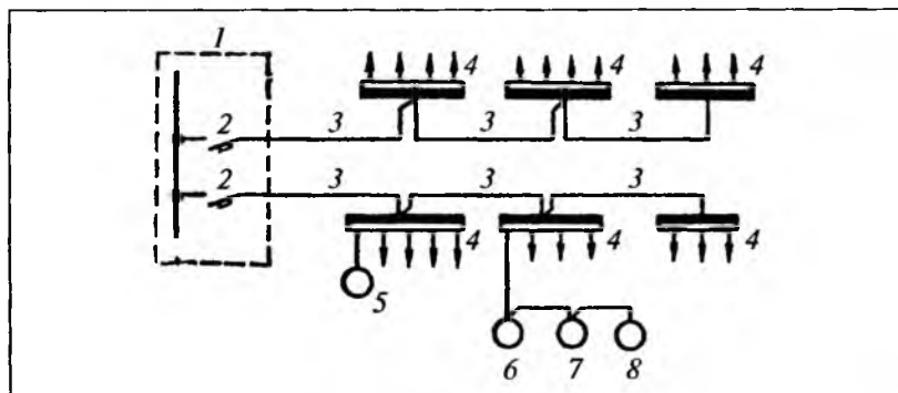
Рис. 2.2. Магистральная схема силовой сети:
