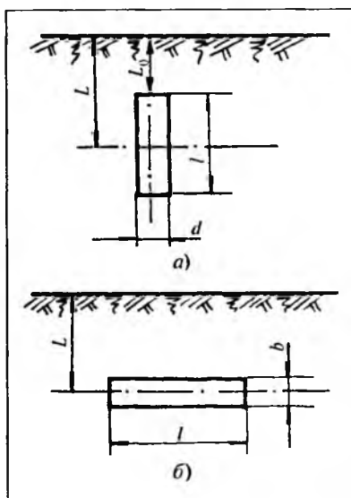
Рис. 4.6. К примеру расчета заземлителя: а — одиночный вертикальный заземлитель; б — горизонтальный протяженный электрод; L_0 — расстояние от уровня земли до верхнего конца электрода; L — расстояние от уровня земли до горизонтальной оси электрода; l — длина электрода; d — диаметр электрода; b — ширина полосы
