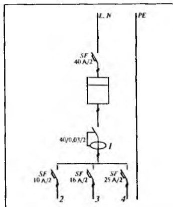
Рис. 4.11. Схема электроснабжения квартиры при отсутствии защитного проводника PE в розеточной цепи и цепи освещения (рекомендуемое временное решение для старого жилого фонда): 1 — УЗО; 2 — цепь освещения; 3 — розеточная цепь; 4 — электроплита
