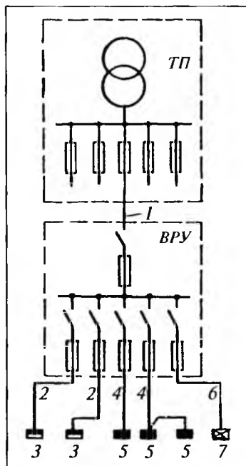
Рис. 2.10. Принципиальная схема электроснабжения общественного здания от однострансформаторной подстанции:
