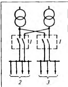
Рис. 2.11. Принципиальная схема электроснабжения общественного здания от двухтрансформаторной подстанции с АВР на контакторных станциях:
