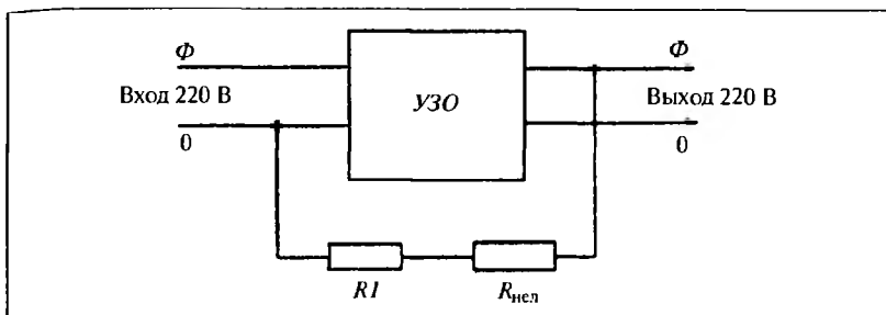
Рис. 4.7. Принципиальная схема включения УЗО для защиты от скачков напряжения в сети:
