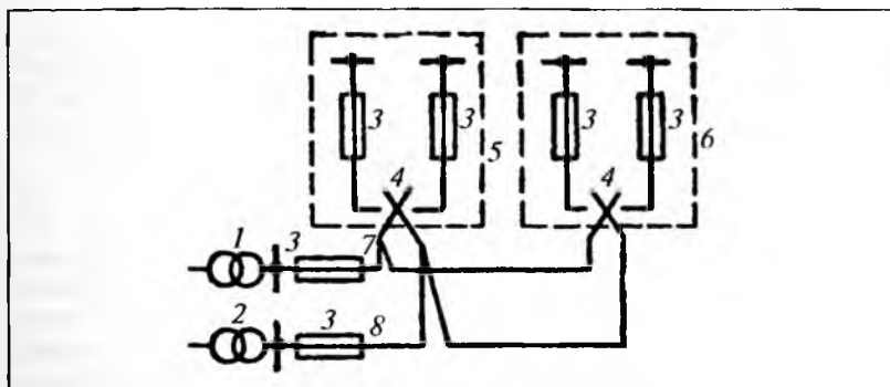
Рис. 2.5. Принципиальная схема электроснабжения жилых домов высотой 9 — 16 этажей с двумя переключателями на вводах:
