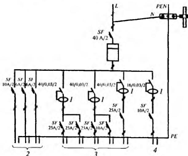
Рис. 4.14. Пример электроснабжения двухкомнатной квартиры повышенной комфортности (TN-C-S):
