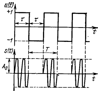
Рис. 3.2. Временные диаграммы модулирующего и манипулированного сигналов
