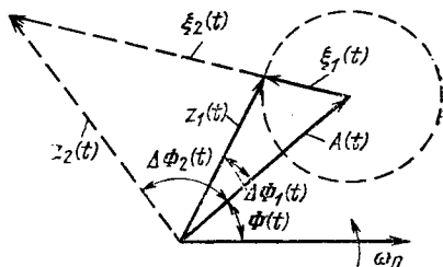
Рис. 7.3. Иллюстрация появления порогового эффекта
