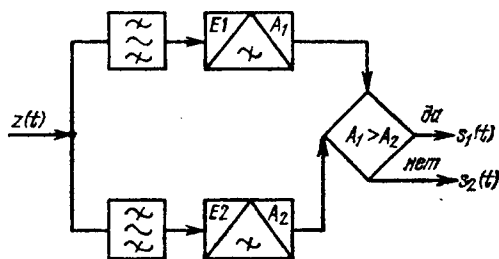
Рис. 6.8. Некогерентный приемник бинарной системы с ЧМ
