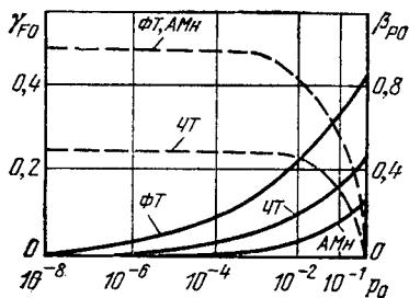
Рис. 10.1. Зависимость \beta_{\mathcal{P}0} и \gamma_{F0} от p_0
