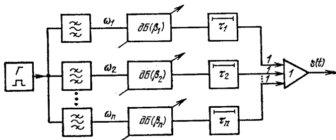
Рис. 2.10. Структурная схема генератора широкополосных сигналов
