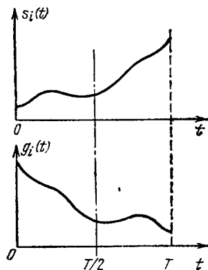
Рис. 6.4. Графики сигнала и характеристики согласованного фильтра
