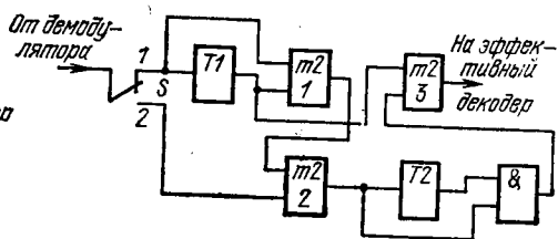
Рис. 8.6. Схема декодера непрерывного кода
