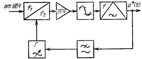
Рис. 7.5. Фрагмент схемы приемника ЧМ сигналов с обратной связью по частоте
