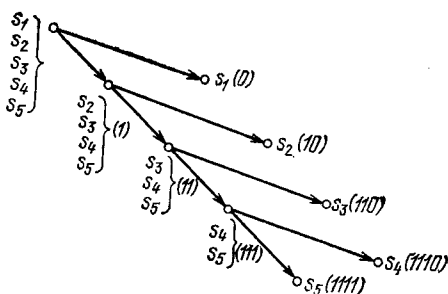
Рис. 5.2. Граф кодирования
