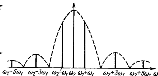
Рис. 3.3. Спектр АМн сигнала
