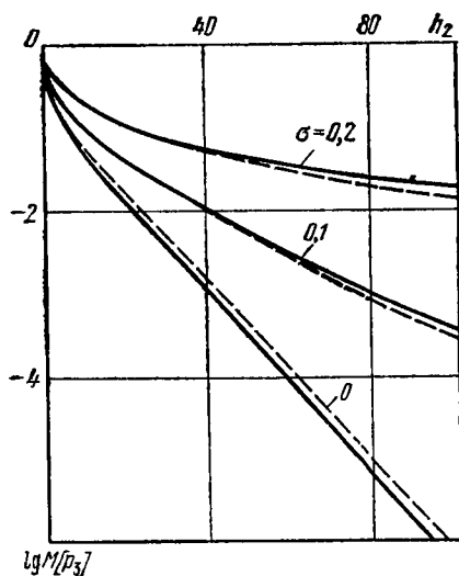
Рис. 6.11. Влияние рассинхронизации на помехоустойчивость приема АМн сигналов
