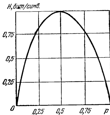
Рис. 5.1. График функции (5.13)
