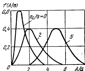
Рис. 2.7. Распределение Релея
