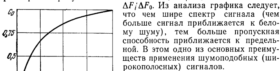
Рис. 5.3. График C_0(\Delta F / \Delta F_0)
