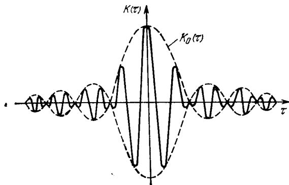
Рис. 2.6. Корреляционная функция узкополосного процесса
