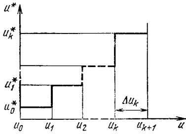
Рис. 3.8. Характеристика квантования
