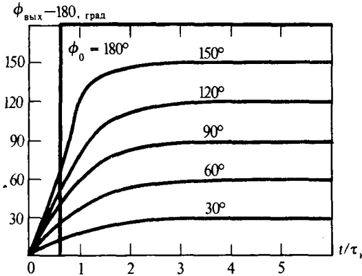
Рис. 9.10. Зависимость мгновенной фазы сигнала на выходе усилителя от безразмерного параметра t/\tau_k
