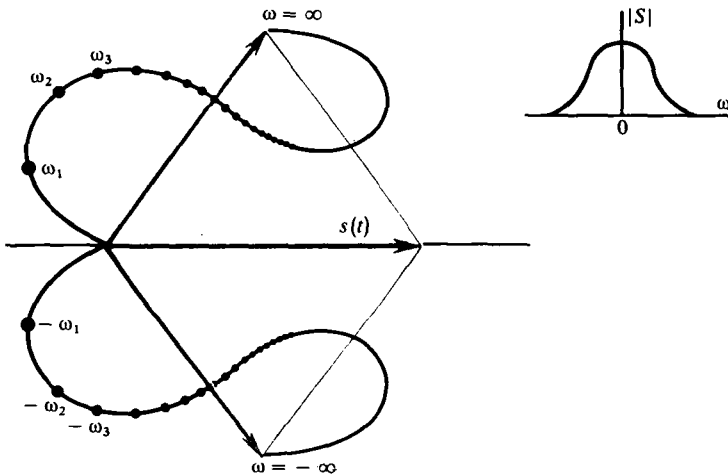
Рис. 2.5. Векторная диаграмма непериодического сигнала (справа изображена зависимость модуля спектральной плотности от частоты)
