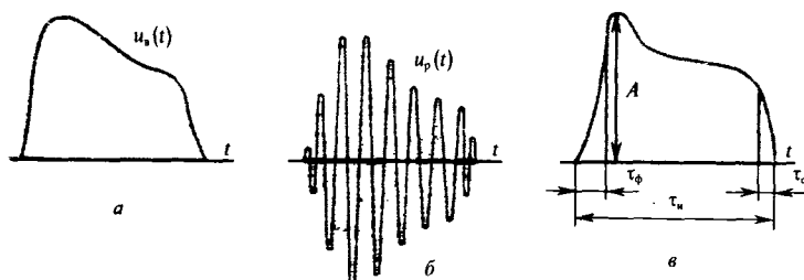
Рис. 1.1. Импульсные сигналы и их характеристики:
