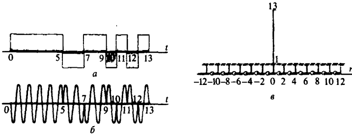
Рис. 3.7. Сигнал Баркера при M = 13 :
