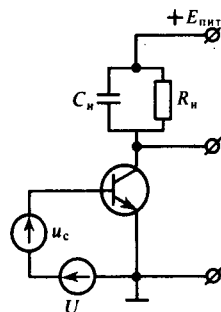
Схема коллекторного детектора
