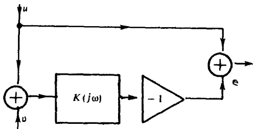
Рис. 16.9. Принцип получения сигнала ошибки
