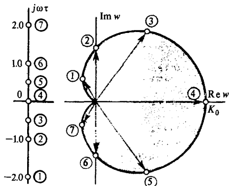
Рис. 14.6. Амплитудно-фазовая характеристика двухступенчатого усилителя с апериодическими нагрузками
