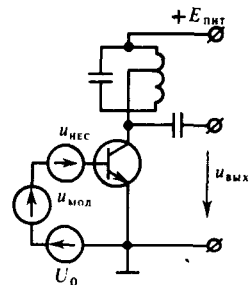
принцип работы амплитудного модулятора с кусочно-линейной характеристикой
