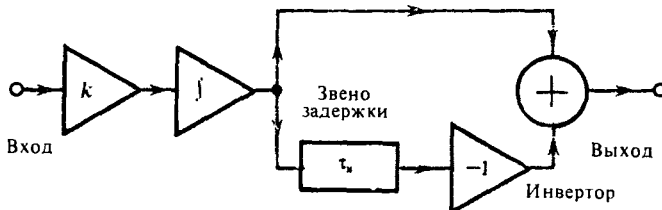
Рис. 16.3. Структурная схема согласованного фильтра для прямоугольного видеоимпульса
