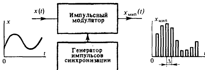
Рис. 15.1. Структурная схема импульсного модулятора
