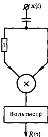
Коррелометр
