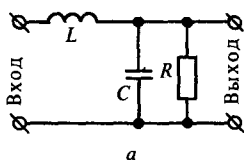
Рис. 13.5. Звено 2-го порядка:
