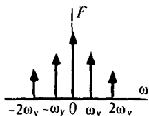
Спектральная плотность управляющего сигнала
