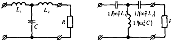
Рис. 13.6. Переход от схемы ФНЧ к схеме ФВЧ
