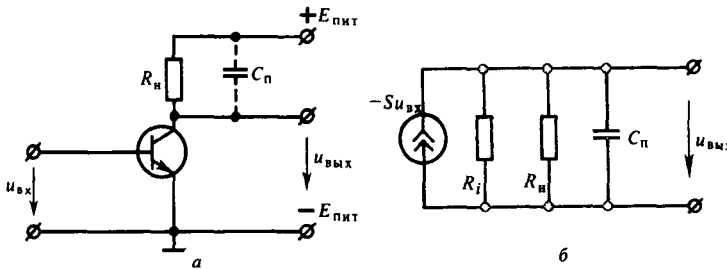
Рис. 8.1. Усилитель напряжения:
