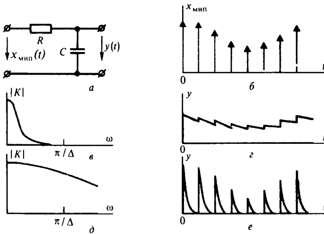
Рис. 15.3. Восстановление непрерывного сигнала по его импульсным отсчетам с помощью RC-цепи:
