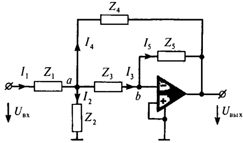
Рис. 14.9. Схема активного фильтра с двухпетлевой обратной связью
