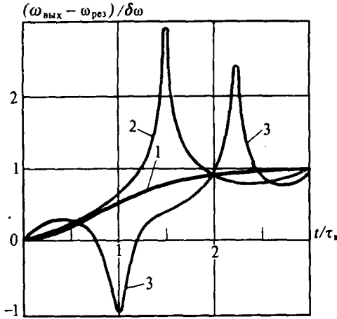
Рис. 9.12. Процесс установления мгновенной частоты на выходе резонансного усилителя:
