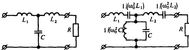
Рис. 13.7. Переход от схемы ФНЧ к схеме ПФ
