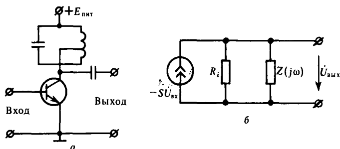
Рис. 9.2. Резонансный усилитель малых колебаний: а — принципиальная схема; б — схема замещения
