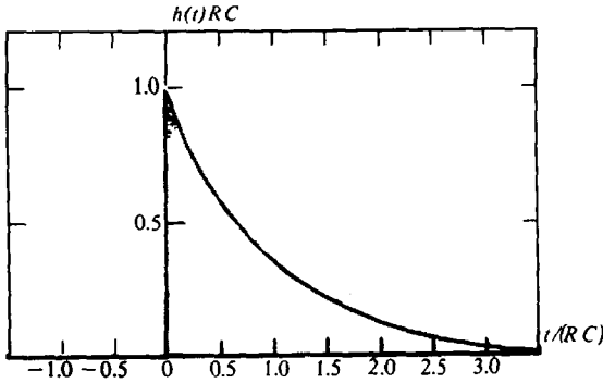
Рис. 8.2. График импульсной характеристики RC -цепи
