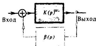
Рис. 14.1. Структурная схема линейной системы с обратной связью
