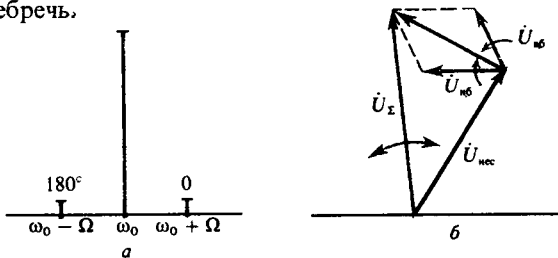
Рис. 4.6. Диаграммы сигнала с угловой модуляцией при m \ll 1 : а — спектральная; б — векторная
