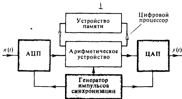
Рис. 15.6. Структурная схема цифровой обработки непрерывных сигналов
