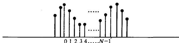
Рис. 15.4. Дискретное представление периодического сигнала
