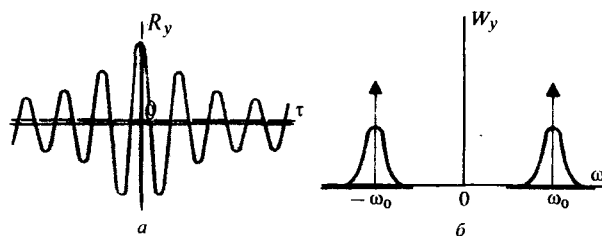
Рис. 12.7. Характеристики сигнала на выходе случайного амплитудного модулятора:
