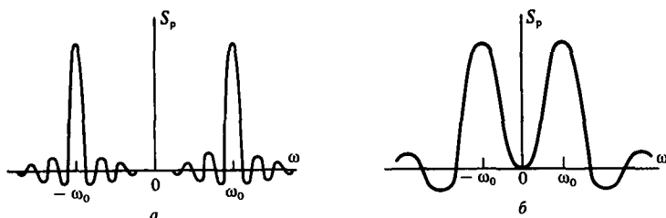
Рис. 2.9. Графики спектральных плотностей радиоимпульса с прямоугольной огибающей:
