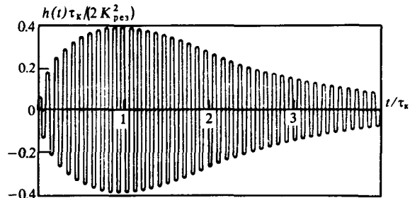
Рис. 9.5. Импульсная характеристика двухконтурного резонансного усилителя
