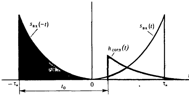
Рис. 16.1. Построение импульсной характеристики согласованного фильтра
