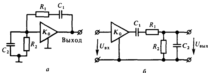
Рис. 14.13. Автогенератор с двумя RC -цепями: а — принципиальная схема; б — схема с разомкнутой цепью обратной связи
