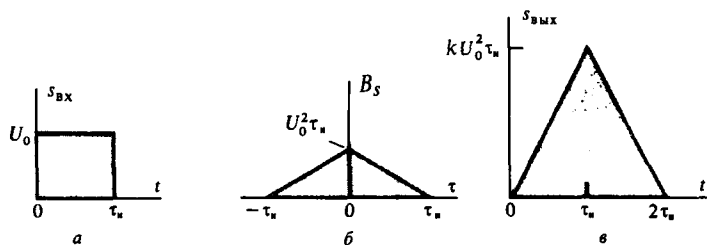
Рис. 16.2. Построение сигнала на выходе фильтра, согласованного с прямоугольным видеоимпульсом:
