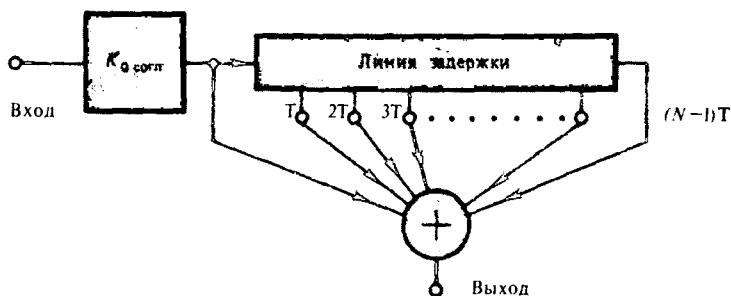
Рис. 16.4. Структурная схема согласованного фильтра для пачки видеоимпульсов
