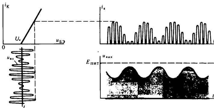
Рис. 11.11. Осциллограммы токов и напряжений в коллекторном детекторе
