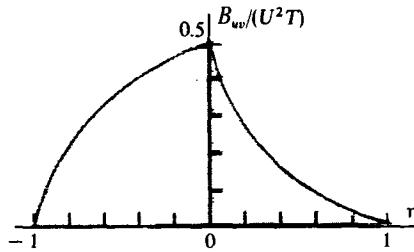
Рис. 3.8. График взаимокорреляционной функции прямогоугольного и треугольного видеоимпульсов
