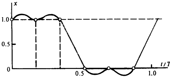
Рис. 15.5. Сигнал, восстановленный по коэффициентам ДПФ
