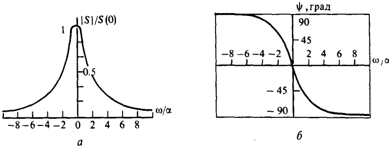
Рис. 2.7. Спектральная плотность экспоненциального видеоимпульса: a – нормированный амплитудный спектр; b – фазовый спектр
