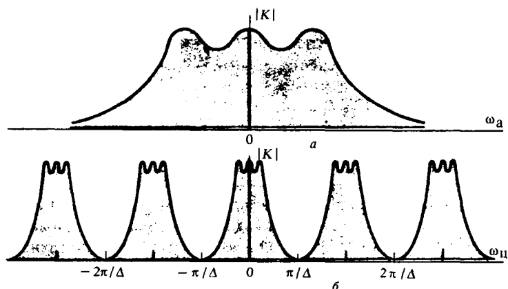
Рис. 15.12. Амплитудно-частотные характеристики фильтров:
