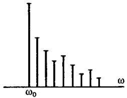
Спектр однополосного сигнала
