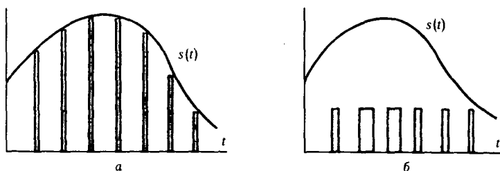
Рис. 1.2. Дискретизация аналогового сигнала:
