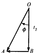
Векторные диаграммы сигнала на выходе модулятора Армстронга в два последовательных момента времени t_1 и t_2
