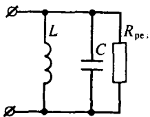
Эквивалентная схема параллель- ного колебатель- ного контура
