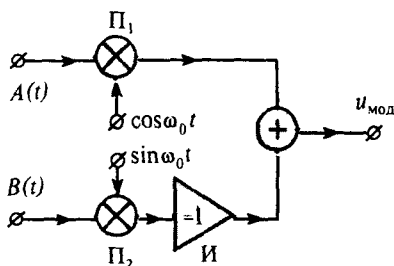
Рис. 12.3. Структурная схема параметрического модулятора
