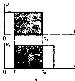
Рис. 3.4. Нахождение АКФ прямоугольного видеоимпульса
