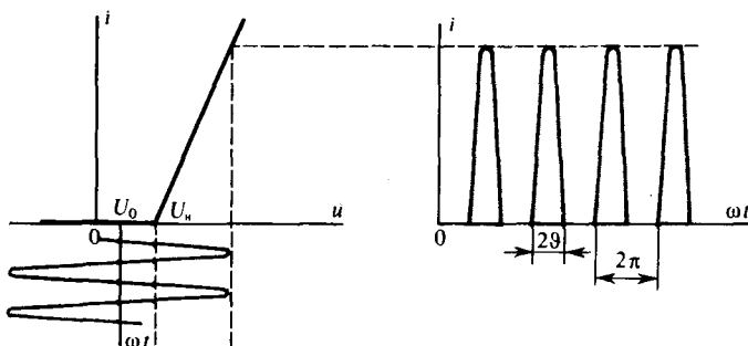
Рис. 11.5. Форма тока в цепи, содержащей нелинейный элемент с кусочно-линейной характеристикой
