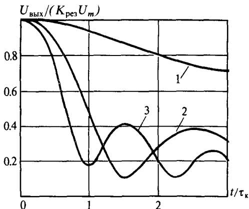
Рис. 9.11. Процесс установления физической огибающей сигнала на выходе усилителя после скачка частоты при различных параметрах b = \delta\omega\tau_k :
