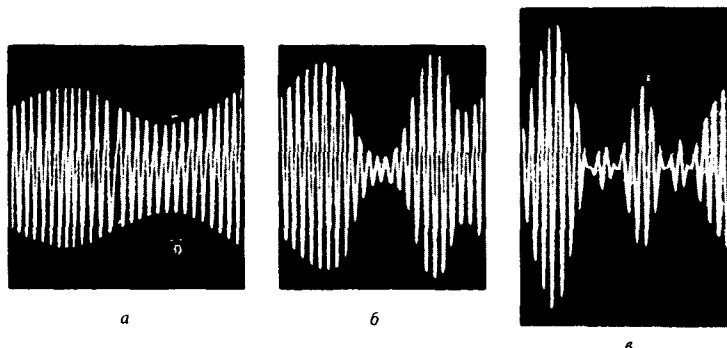
Рис. 4.1. АМ-сигналы при различных глубинах модуляции: а — неглубокая модуляция; б — глубокая модуляция; в — перемодуляция
