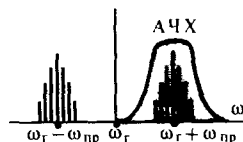
Подавление зеркального канала
