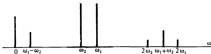
Рис. 11.7. Спектральная диаграмма тока в нелинейном двухполюснике с вольт-амперной характеристикой, описываемой квадратичным многочленом (входной сигнал — бигармоническое колебание, спектр которого на рисунке выделен)
