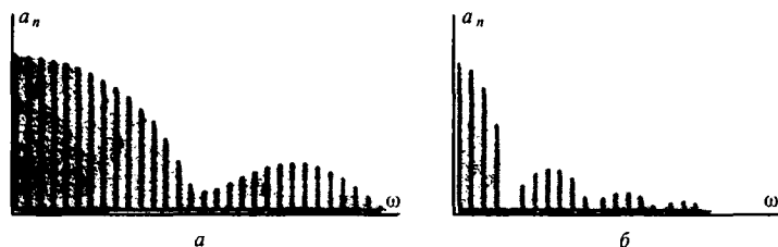
Рис. 2.2. Амплитудный спектр периодической последовательности прямоугольных видеоимпульсов:
