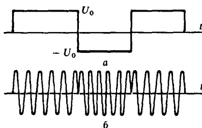
Рис. 3.6. Трехпозиционный сложный сигнал: а — амплитудное кодирование; б — фазовое кодирование
