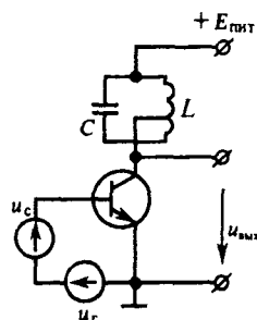
Схема преобразователя частоты
