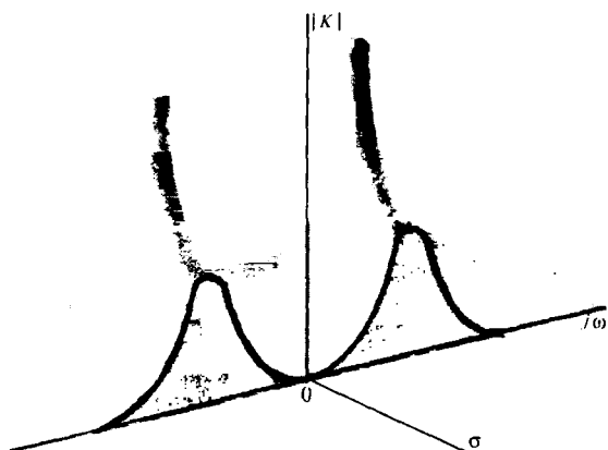
Рис. 8.4. Характер поверхности |K(p)| для передаточной функции, имеющей два комплексно-сопряженных полюса p_{1,2} = -\alpha \pm j\omega_0 и один нуль z = 0
