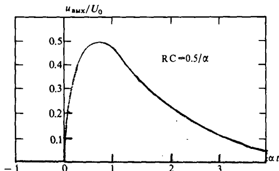
Рис. 8.3. Отклик RC -цепи на экспоненциальный видеопульс
