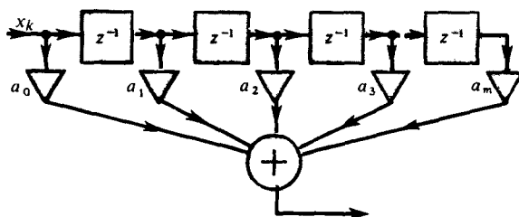
Рис. 15.7. Схема построения трансверсального ЦФ
