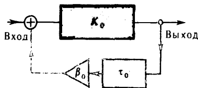
Рис. 14.4. Структурная схема системы с запаздывающей обратной связью
