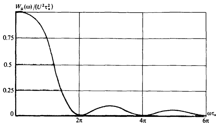
Рис. 3.2. Нормированный энергетический спектр прямоугольного видеоимпульса как функция безразмерной частотной переменной \omega\tau_n
