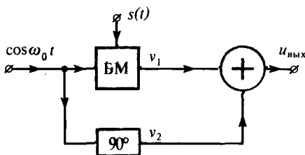
Рис. 11.10. Модулятор Армстронга
