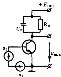
Схема синхронного детектора
