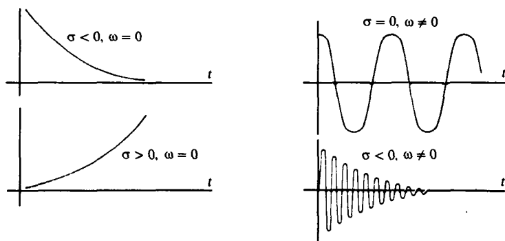
Рис. 2.10. Вещественные сигналы, отвечающие различным значениям комплексной частоты
