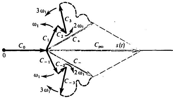
Рис. 2.4. Графическое отображение ряда Фурье в комплексной форме
