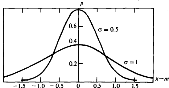
Рис. 6.1. График гауссовской плотности вероятности при различных значениях параметра \sigma
