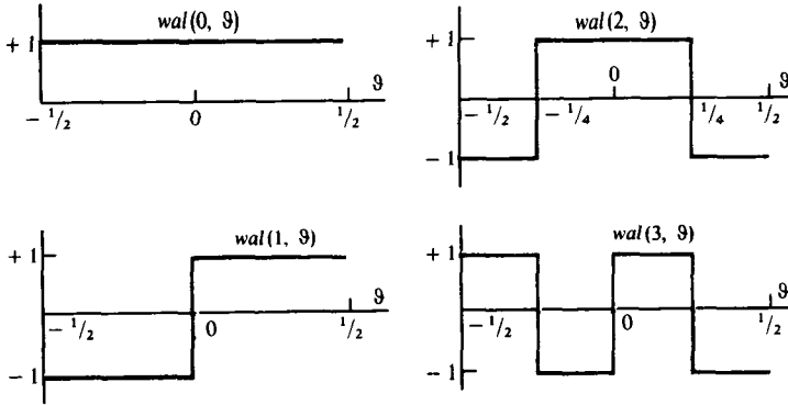
Рис. 1.4. Графики нескольких первых функций Уолша
