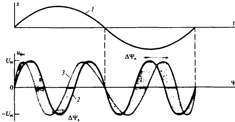
Рис. 4.5. Фазовая модуляция:
