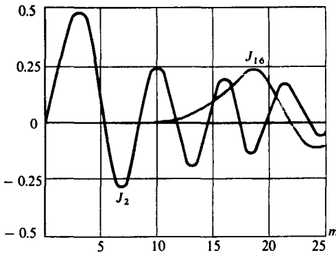
Рис. 4.7. Графики функций Бесселя J_2(m) и J_{16}(m)
