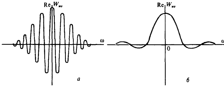
Рис. 3.1. Взаимный энергетический спектр двух экспоненциальных видеоимпульсов:
