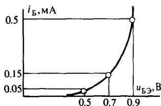
Рис. 11.3. Степенная аппроксимация входной характеристики транзистора КТ301
