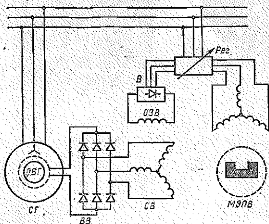
Рис. 1.3. Схема синхронного генератора с вращающимися выпрямителями:
