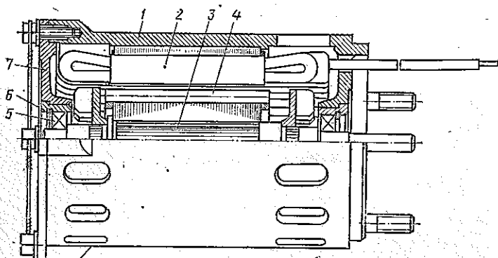
Рис. 1.7. Продольный разрез короткозамкнутого асинхронного двигателя:
