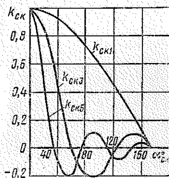
Рис. 6.25. Коэффициенты скоса для первой, третьей и пятой гармонической в зависимости от угла скоса зубцов
