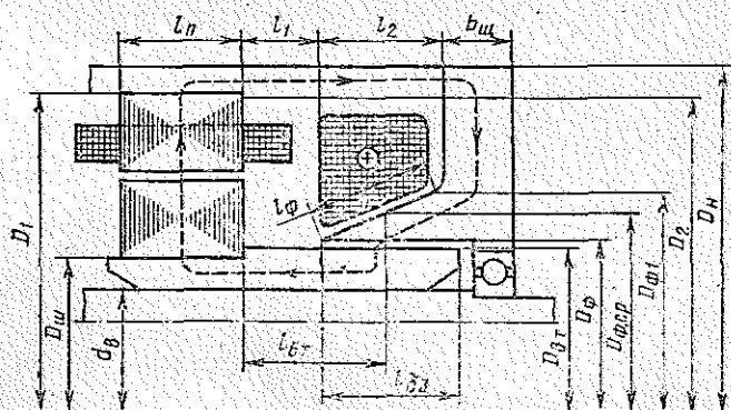
Рис. 6.38. Одноименнополюсный однопакетный генератор
