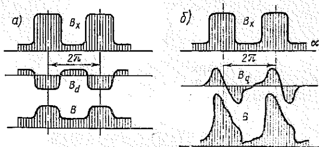
Рис. 6.10. Магнитные поля в индукторном генераторе (без скоса пазов ротора) при индуктивной (а) и активной (б) нагрузках
