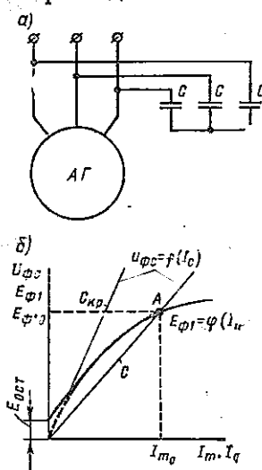
Рис. 4.1. Схема подключения конденсаторов к асинхронному генератору (а) и характеристики самовозбуждения (б)
