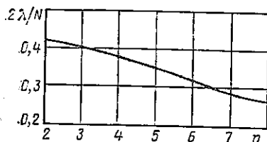
Рис. 5.9. Кривая значений конструктивного коэффициента в зависимости от числа пар полюсов (материал сталь 10 и 35ХГСЛ)
