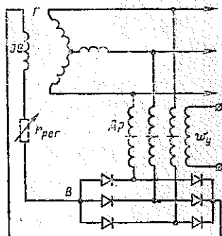
Рис. 2.43. Схема с самовозбуждением и регулированием напряжения с помощью управляемых дросселей: Г — генератор; ОВ — обмотка возбуждения; В — выпрямитель; Др — дроссель; w_y — обмотка управления; r_{пер} — регулируемое сопротивление регулятора
