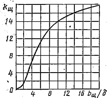
Рис. 2.49. Кривая коэффициента k_{ш} от отношения b_{ш}/\delta
