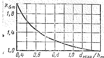
Рис. 2.36. Кривая зависимости k_{sm} от отношения d_{мин}/h_m
