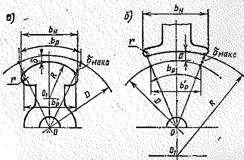
Рис. 2.11. Схема для расчета радиуса кривизны полюсного башмака для генераторов с полюсами на роторе (а) и с полюсами на статоре (б)
