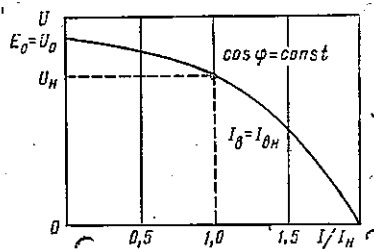
Рис. 2.46. Внешняя характеристика генератора
