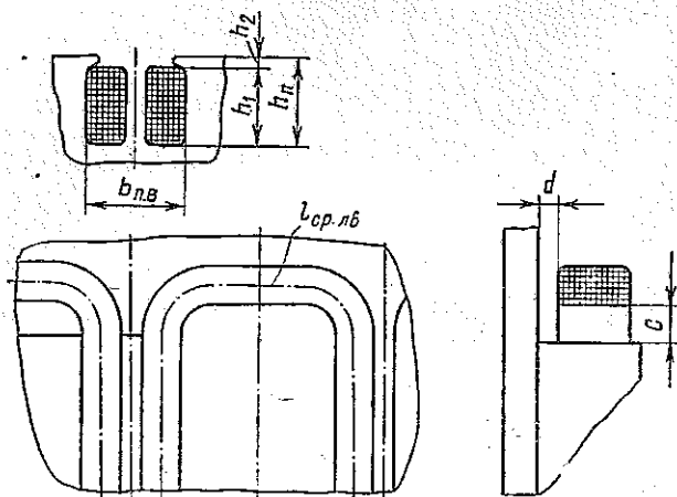
Рис. 6.42. Схема обмотки возбуждения разноремненнополюсного генератора
