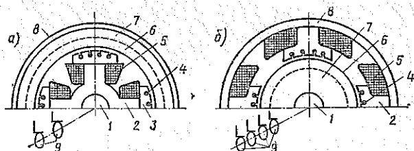
Рис. 1.1. Магнитная цепь контактных генераторов:
