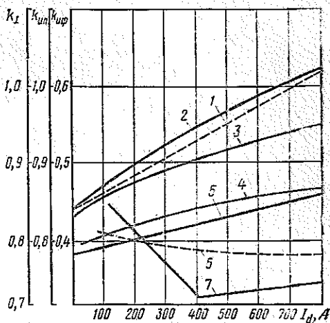
Рис. 3.14. Опытные значения коэффициентов k_{u\phi} , k_{u\pi} и k_I для генератора мощностью 24 кВт в функции тока нагрузки I_d при U_d=28,5 \text{ В}=\text{const} :
