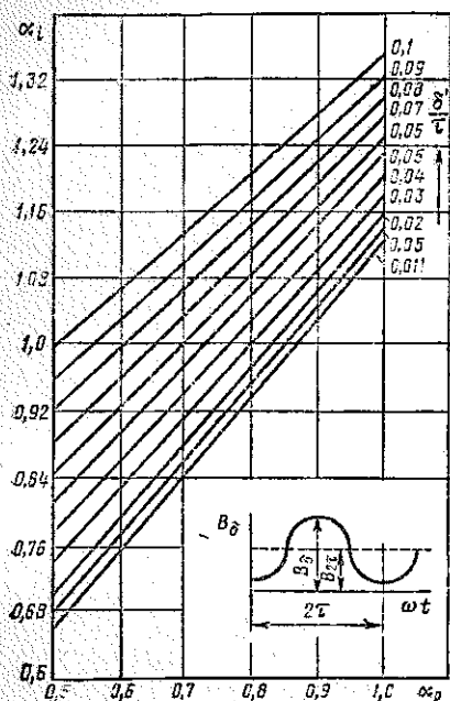
Рис. 6.29. Кривые расчетного коэффициента полюсного перекрытия \alpha_i = 2B_{2\tau} / B_\delta
