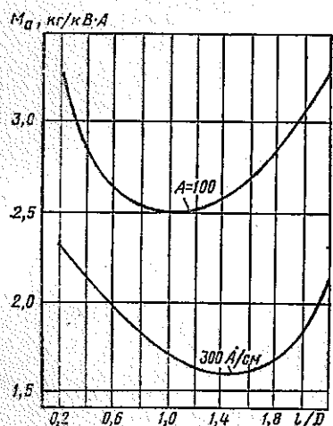
Рис. 4.6. Зависимость удельной массы асинхронного генератора от отношения \lambda/D :
