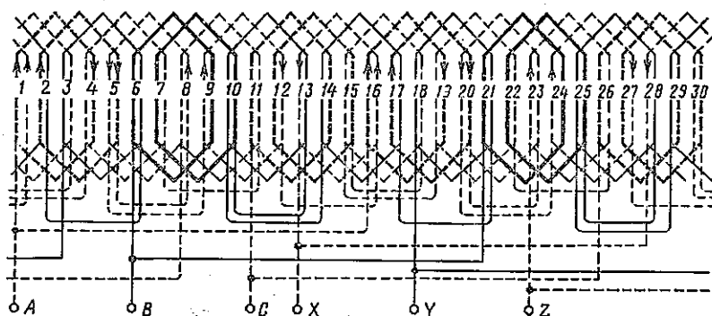
Рис. 2.14. Электрическая схема соединений обмотки якоря:
