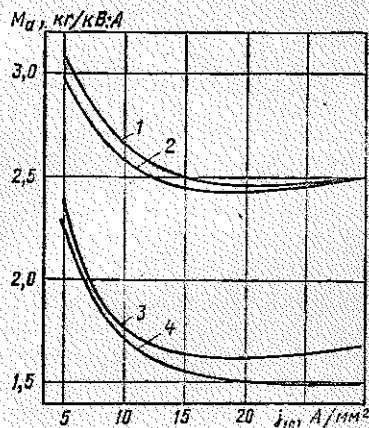
Рис. 4.8. Зависимость удельной массы асинхронного генератора с самоохлаждением от плотности тока в обмотке статора: P_n = 1000 В·А; \cos \varphi = 0.9 ; f = 400 Гц; m = 3 ; q = 3 ; p = 1 ; U_{\phi} = 115 В; B_2 = 1.4 Тл; 1 - B_{\delta} = 0.6 Тл; A = 100 А/см; 2 - B_{\delta} = 0.5 Тл; A = 100 А/см; 3 - B_{\delta} = 0.5 Тл; A = 300 А/см; 4 - B_{\delta} = 0.6 Тл; A = 300 А/см
