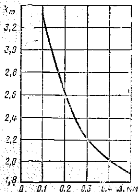
Рис. 6.46. Кривая коэффициента, учитывающего увеличение потерь в стали вследствие обработки
