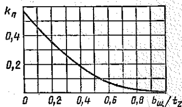
Рис. 2.50. Значение коэффициента k_n в зависимости от b_m/t_z
