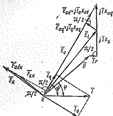
Рис. 6.45. Векторная диаграмма напряжений
