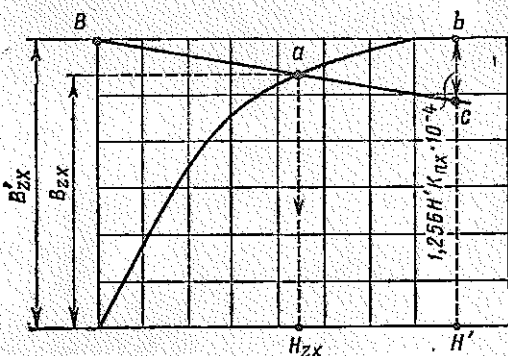
Рис. 2.31. Графическое нахождение действительной индукции в зубце B_{zx}
