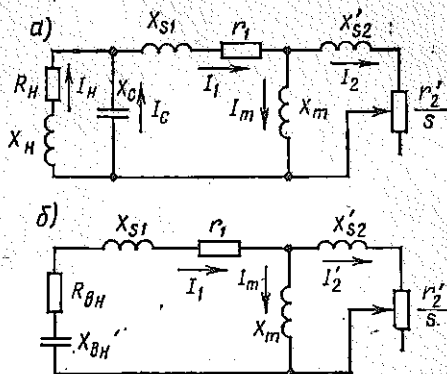
Рис. 4.2. Схема замещения асинхронного генератора с самовозбуждением: а — без приведения внешней магнитной цепи; б — с приведением внешней цепи
