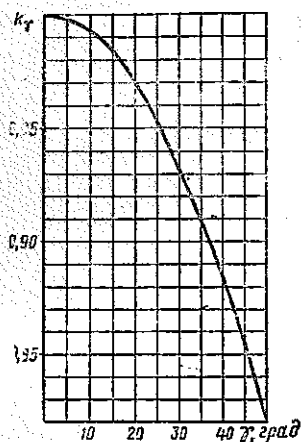
Рис. 3.11. Зависимость коэффициента k_\gamma от угла \gamma
