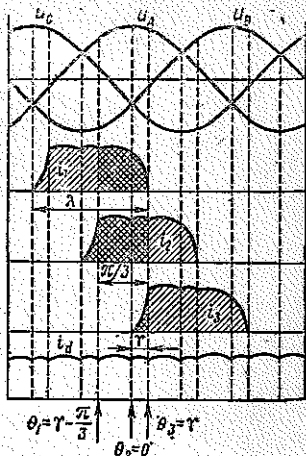
Рис. 3.12. Кривые фазных и выпрямленных токов при трехфазной мостовой схеме выпрямления
