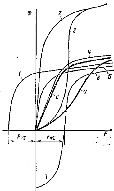
Рис. 4.18. Графическое построение характеристики магнитной цепи асинхронного генератора при действии МДС подмагничивания спинки якоря F_{\pi} :
