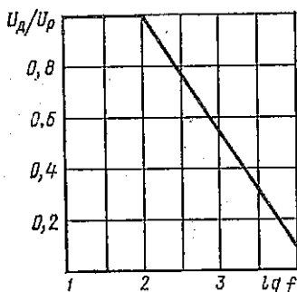
Рис. 4.10. Зависимость допустимого напряжения конденсатора от частоты
