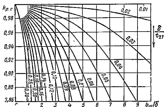
Рис. 6.44. Кривые коэффициента, учитывающего увеличение сопротивления магнитной цепи из-за раскрытия пазов якоря
