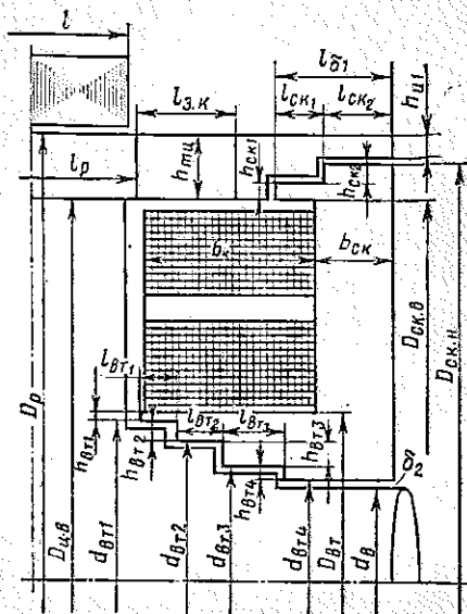
Рис. 5.11. Схема для расчета размеров скобы
