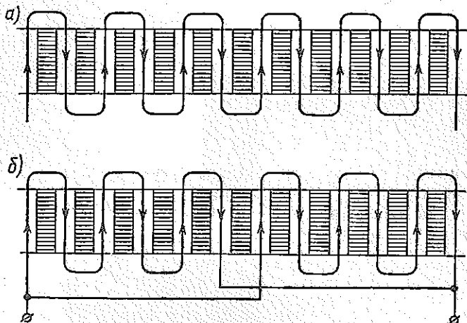
Рис. 6.34. Схема образования якорной обмотки с параллельными ветвями:
