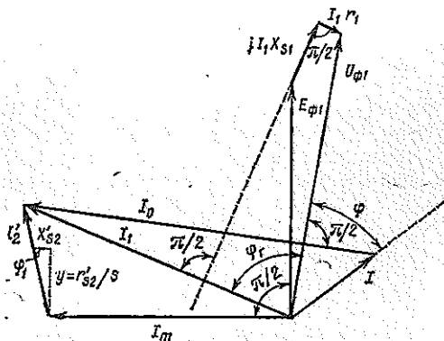
Рис. 4.3. Векторная диаграмма напряжений асинхронного генератора с самовозбуждением
