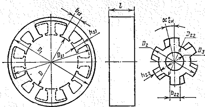
Рис. 6.41. Магнитная система разноименнополюсного генератора
