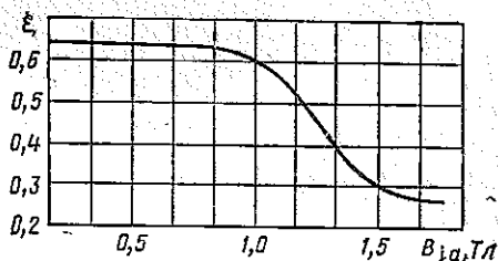
Рис. 2.33. Кривая поправочного коэффициента \xi
