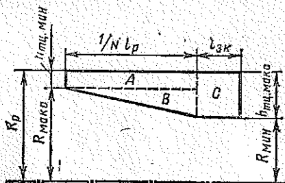
Рис. 5.13. Боковая поверхность полюса цилиндра
