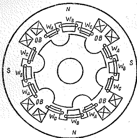
Рис. 6.35. Схема разноименнополюсного трехфазного генератора (генератор Лоренца)
