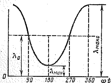
Рис. 6.7. Кривая проводимости воздушного зазора (первой гармонической)
