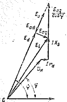
Рис. 2.40. Векторная диаграмма напряжений Blondеля
