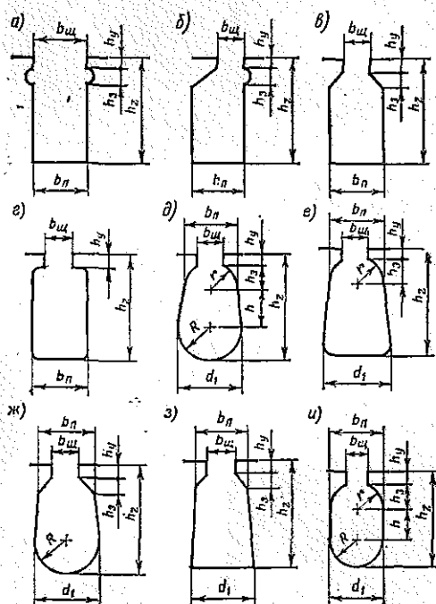
Рис. 2.20. Схемы для расчета пазовых рассеяний
