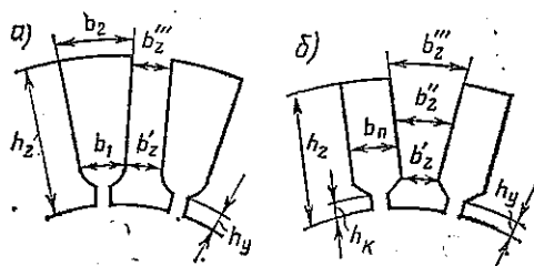
Рис. 2.32. Схема зубцов якоря на статоре: а — прямые; б — трапециевидальные
