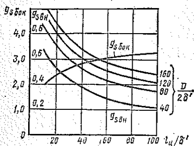
Рис. 5.17. Относительные магнитные проводимости внешнего потока:
