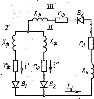
Рис. 3.9. Электрическая схема замещения коммутируемой секции двухполупериодной трехфазной системы выпрямления: r_\phi и X_\phi — активное и индуктивное сопротивления обмоток якоря; r_H и X_H — активное и индуктивное сопротивления нагрузки; I, II, III — фазы
