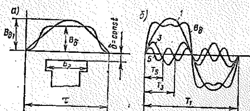
Рис. 2.8. Кривая распределения индукции в воздушном зазоре (а) и разложение ее на гармонические составляющие (б)
