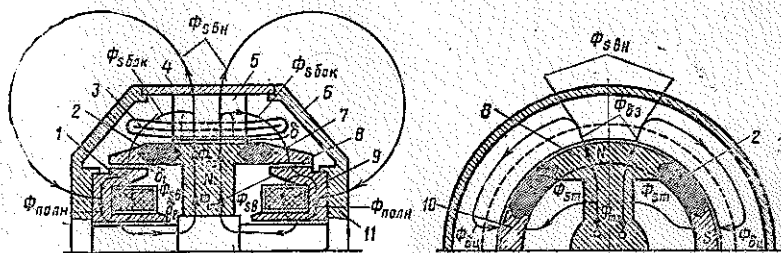
Рис. 5.1. Магнитная цепь генератора типа сексин с двусторонней системой возбуждения и пути магнитных потоков ( 2p=4 ):
