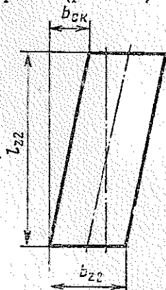
Рис. 6.24. Схема определения коэффициента скоса
