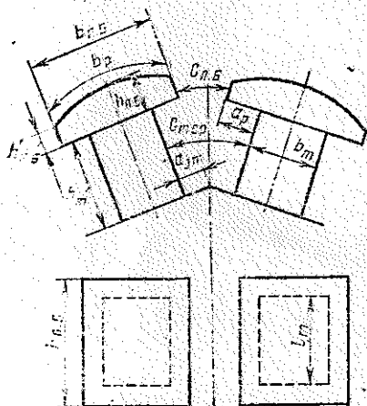
Рис. 2.34. Схема полюсов на роторе
