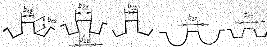
Рис. 6.23. Конструкция зубцов ротора
