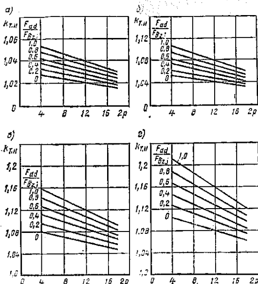
Рис. 5.16. Коэффициент магнитного потока торцевой поверхности полюса звезды:
