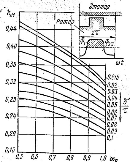
Рис. 6.30. Кривые коэффициента использования магнитного потока для режима холостого хода k_{uc} = \Phi_1 / \Phi_{2\tau}
