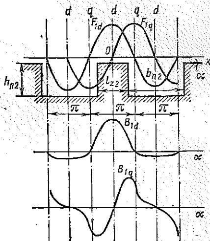
Рис. 6.9. МДС реакции якоря (первая гармоническая) по продольной и поперечной осям зубца ротора и создаваемые ими поля
