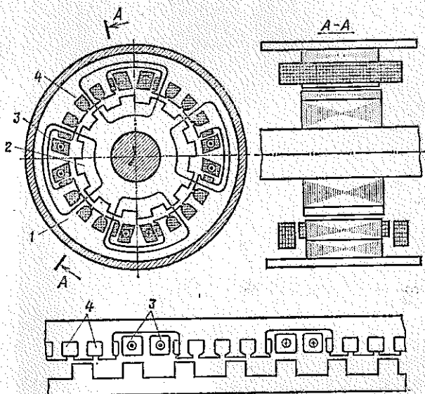
Рис. 6.3. Разноименнополюсный индукторный генератор с классической зубцовой зоной:
