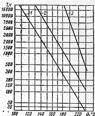
Рис. 2.16. Кривые зависимости срока службы изоляции различных классов нагревостойкости от температуры \theta :
