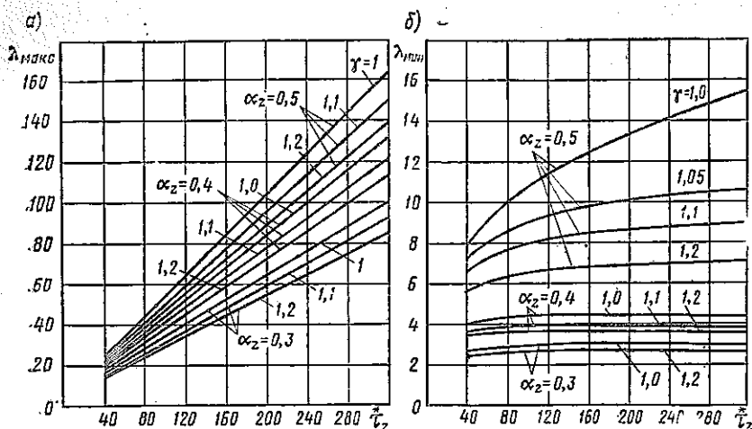
Рис. 6.26. Кривые зависимостей максимальной \lambda_{\text{макс}} (а) и минимальной \lambda_{\text{мин}} (б) удельных магнитных проводимостей в функции относительных параметров зубцовой зоны
