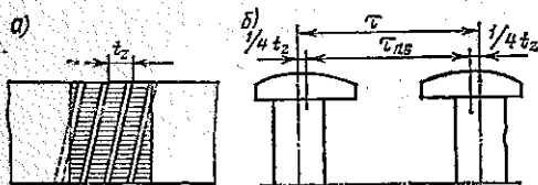
Рис. 2.12. Методы уменьшения зубцовых гармоник:
