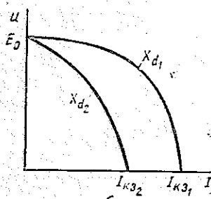
Рис. 2.3. Внешние характеристики генератора при различных значениях X_d : X_{d2} > X_{d1} ; I_{кз2} < I_{кз1}
