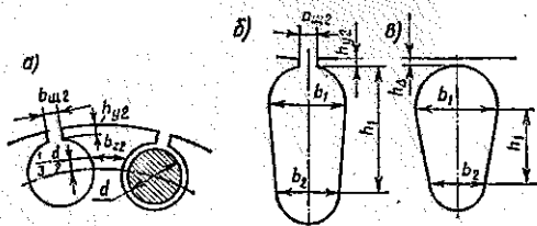
Рис. 4.9. Форма пазов ротора асинхронной машины:
