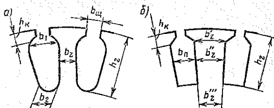
Рис. 2.30. Схема зубцов якоря на роторе: а — прямые; б — трапециевидные
