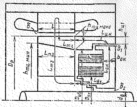
Рис. 5.15. Схема для расчета магнитной цепи генератора
