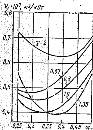
Рис. 6.22. Зависимость удельного объема генератора от геометрии зубцовой зоны:
