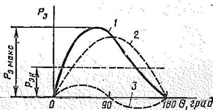
Рис. 2.7. Кривые электромагнитной мощности и ее составляющих в зависимости от угла \theta :
