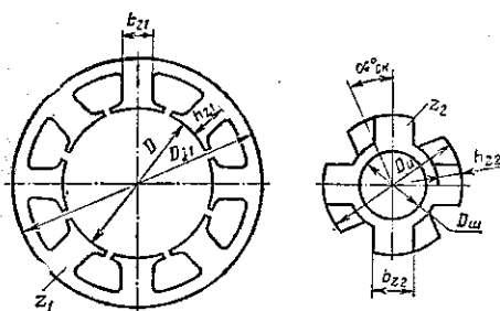
Рис. 6.39. Магнитная система пакета одноименнополюсного генератора
