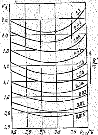
Рис. 6.11. Коэффициент приведения МДС якоря по продольной оси
