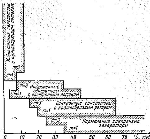
Рис. 6.15. Области применения различных типов генераторов
