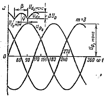
Рис. 3.5. Кривые фазных напряжений трехфазного генератора и пульсаций выпрямленного напряжения в режиме холостого хода
