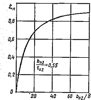
Рис. 6.18. Зависимость \xi_{II}=f(b_{\pi 2}/\delta)
