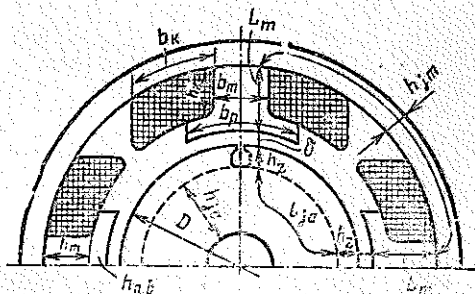
Рис. 2.24. Эскиз магнитной цепи генератора с вращающимся якорем
