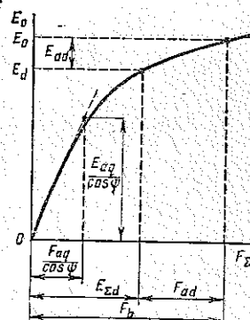
Рис. 2.39. Характеристика холостого хода генератора E_0 = f(F_z)
