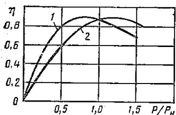
Рис. 2.5. Влияние соотношения A и B_\delta на характер кривой КПД:
