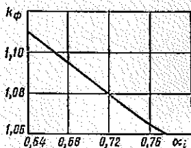
Рис. 4.13. Зависимость коэффициента k_\phi от коэффициента \alpha_i
