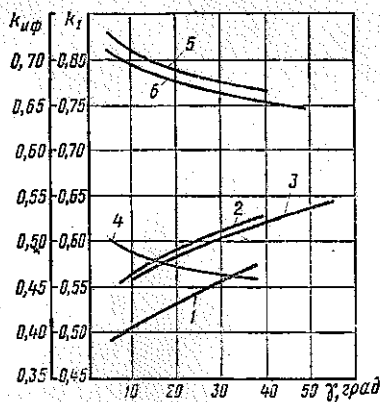
Рис. 3.13. Экспериментальные коэффициенты преобразования напряжения k_{u\phi} и тока k_I в функции угла коммутации \gamma :
