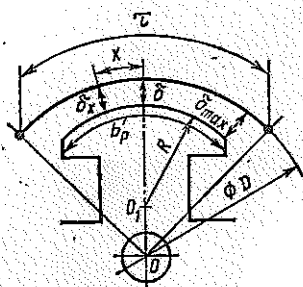
Рис. 2.10. Полюс индуктора при неравномерном воздушном зазоре
