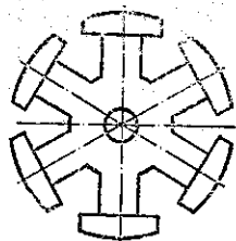
Рис. 2.26. Целноштампованный лист индуктора ротора
