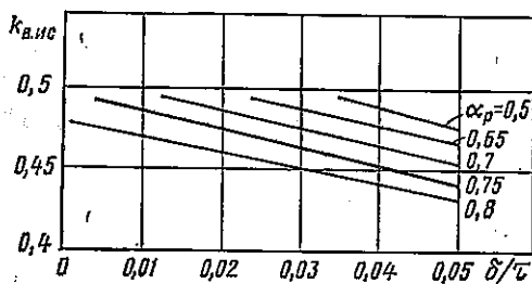
Рис. 5.10. Зависимость k_{в.лс} = f(\alpha_p, \delta'/\tau)
