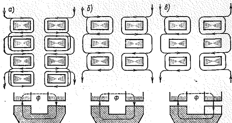
Рис. 6.33. Схема образования обмоток якоря:
