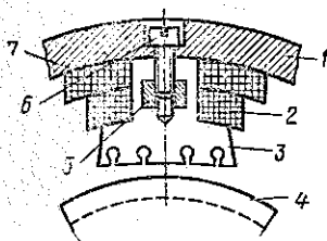
Рис. 2.25. Крепление полюса на корпусе:
