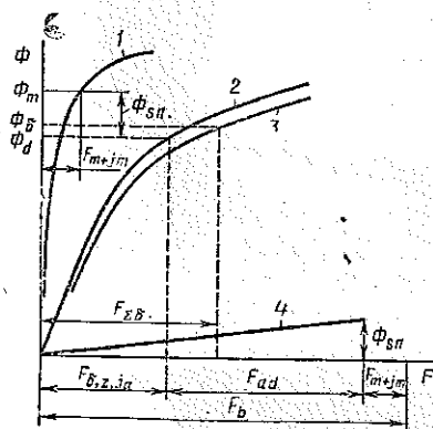
Рис. 2.38. Характеристики намагничивания генератора:
