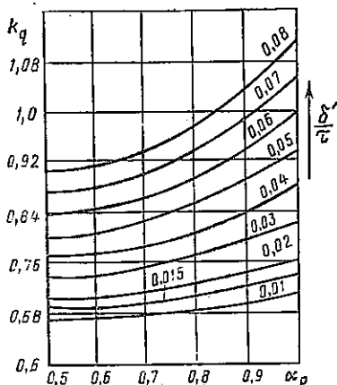
Рис. 6.14. Коэффициент приведения МДС реакции якоря по поперечной оси для открытых пазов ( m=1, q=1 )
