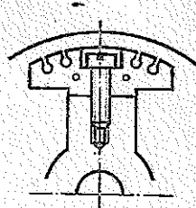
Рис. 2.28. Крепление полюсных башмаков на полюсе с помощью винтов
