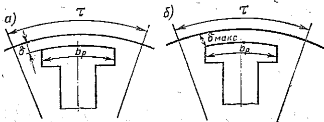
Рис. 2.1. Полусный башмак при равномерном (а) и неравномерном (б) воздушном зазоре
