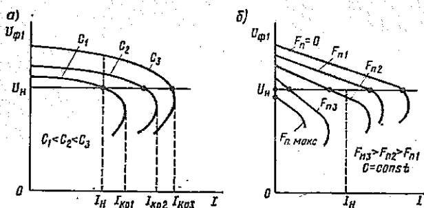
Рис. 4.4. Внешние характеристики асинхронного генератора
