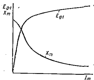
Рис. 4.14. Характеристики намагничивающего контура E_{\phi 1} = f(I_m) и B_{\delta} = \varphi(I_m)
