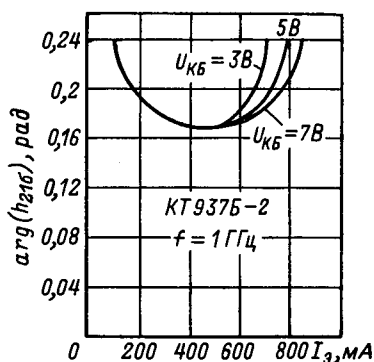
Зависимость фазы коэффициента передачи тока от тока эмиттера.
