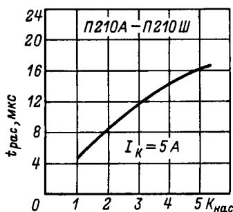
Зависимость времени рассасывания от коэффициента насыщения.
