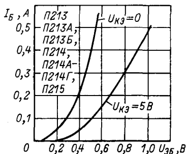
Входные характеристики.
