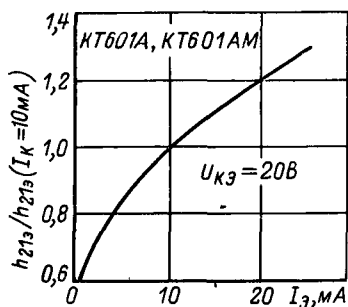
Зависимость относительного коэффициента передачи тока от тока эмиттера.
