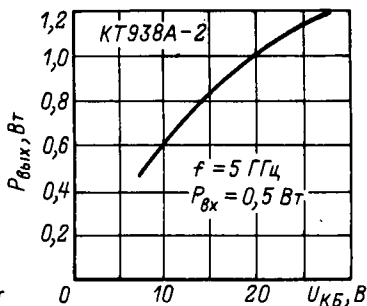
Зависимость выходной мощности от напряжения коллектор-база.
