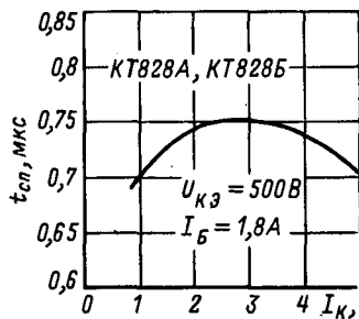
Зависимость времени спада от тока коллектора.
