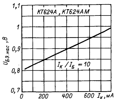
Зависимость напряжения насыщения база-эмиттер от тока коллектора.
