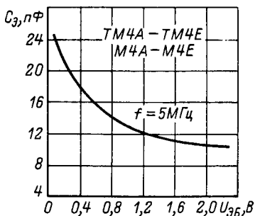
Зависимость емкости эмиттер- ного перехода от напряжения эмиттер-база.
