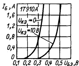
Входные характеристики.
