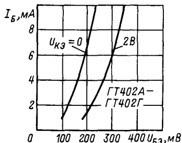
Входные характеристики.
