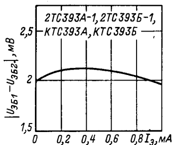
Зависимость модуля разности прямых падений напряжений база-эмиттер от тока эмиттера.
