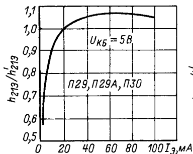
Зависимость относительного статического коэффициента передачи тока в схеме с общим эмиттером от тока эмиттера.
