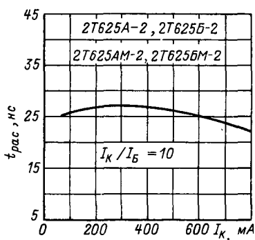
Зависимость времени рассасывания от тока коллектора.
