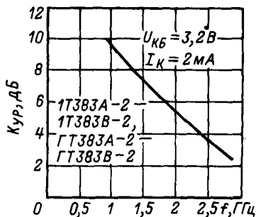
Зависимость коэффициента усиления по мощности от частоты.
