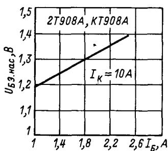
Зависимость напряжения насыщения база-эмиттер от тока базы.
