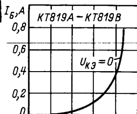
Входная характеристика.
