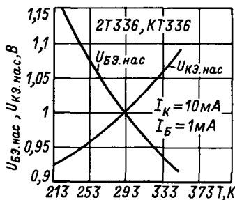
Зависимости напряжений насыщения коллектор-эмиттер и база-эмиттер от температуры.
