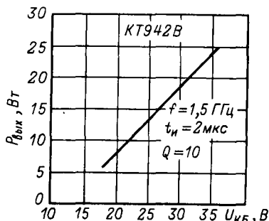
Зависимость выходной мощности в схеме импульсного автогенератора от напряжения коллектор-база.
