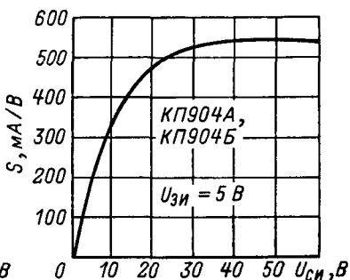
Зависимость крутизны характеристики от напряжения сток-исток.
