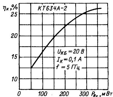
Зависимость коэффициента полезного действия от входной мощности.
