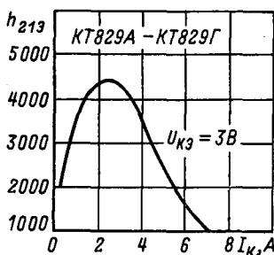
Входные характеристики.
