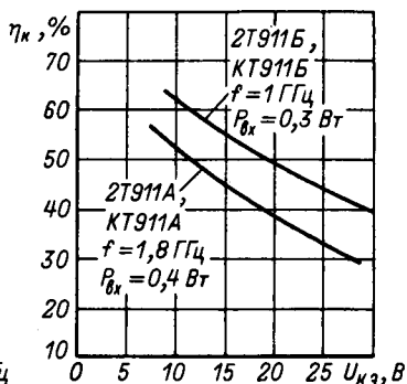
Зависимость коэффициента полезного действия от напряжения коллектор-эмиттер.
