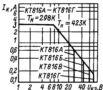
Область максимальных режимов.
