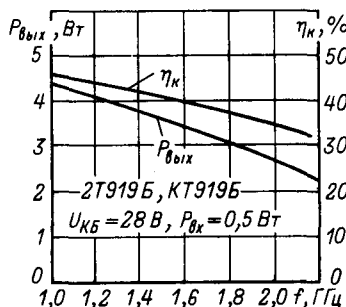
Зависимость выходной мощности и коэффициента полезного действия от частоты.
