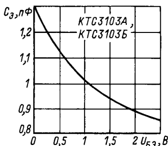
Зависимость емкости эмиттерного перехода от напряжения база-эмиттер.
