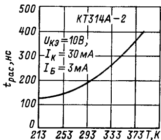
Зависимость времени рассасывания от температуры.
