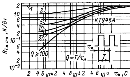
Зависимость импульсного теплового сопротивления переход-корпус от длительности импульса.
