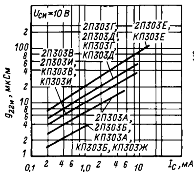
Зависимость активной составляющей выходной проводимости от тока стока.
