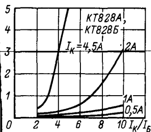
Зависимость напряжения насыщения коллектор-эмиттер от I_K/I_E .
