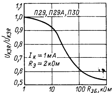
Зависимость относительного постоянного напряжения коллектор-эмиттер от сопротивления в цепи эмиттер-база.
