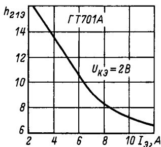
Зависимость статического коэф. ффициента передачи тока от ток эмиттера.
