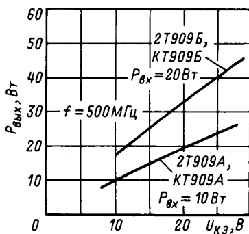
Зависимость выходной мощности от напряжения коллектор-эмиттер.
