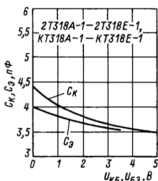
Зависимости емкостей коллекторного и эмиттерного переходов от напряжения коллектор-база и база-эмиттер.
