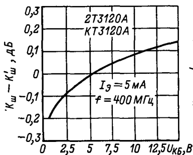
Приведенная зависимость коэффициента шума от напряжения коллектор-база.
