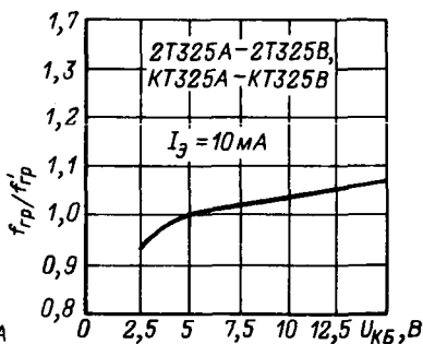
Зависимость относительной граничной частоты от напряжения коллектор-база.
