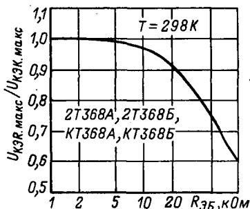
Зависимость относительного максимально допустимого постоянного напряжения коллектор-эмиттер от сопротивления в цепи база-эмиттер.
