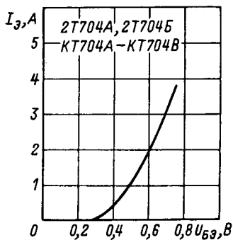
Зависимость тока эмиттера от напряжения база-эмиттер.
