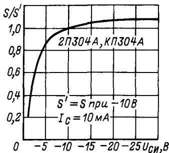
Зависимость относительной крутизны характеристики от напряжения сток-исток.
