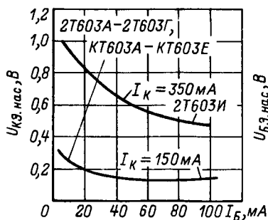
Зависимость напряжения насыщения коллектор-эмиттер от тока базы.
