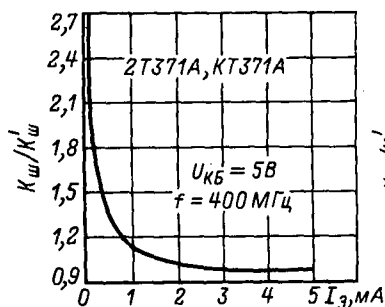
Зависимость относительного коэффициента шума от тока эмиттера.
