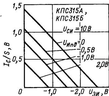
Зависимость отношения тока стока к крутизне характеристики от напряжения затвор-исток.
