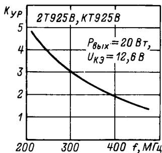
Зависимость коэффициента усиления по мощности от частоты.
