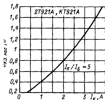
Зависимость напряжения насыщения коллектор-эмиттер от тока коллектора.
