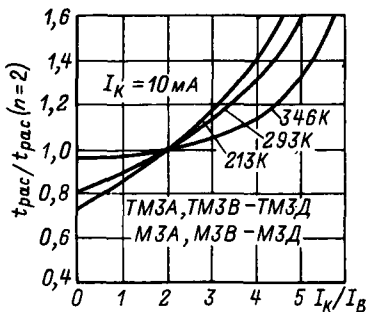
Зависимость относительного времени рассасывания от I_K/I_B .
