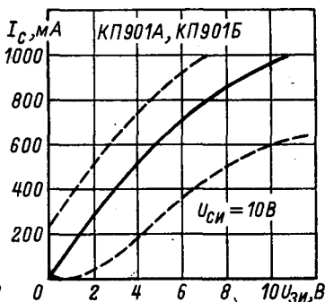
Зона возможных положений зависимости тока стока от напряжения затвор-исток.
