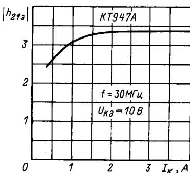
Зависимость модуля коэффици- ента передачи от тока коллек- тора.
