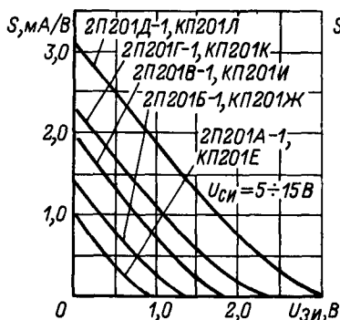
Зависимости крутизны характеристики от напряжения затвористок.
