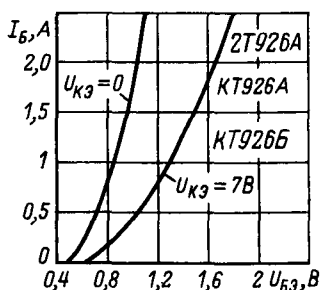
Входные характеристики.
