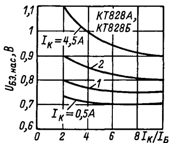
Зависимость напряжения насыщения база-эмиттер от I_K/I_E .
