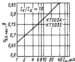
Зависимость напряжения насыщения база-эмиттер от тока коллектора.
