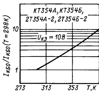
Зависимость относительного обратного тока коллектора от температуры.
