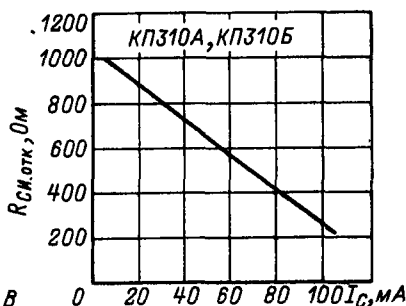
Зависимость сопротивления сток-исток в открытом состоянии от тока стока.
