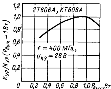
Зависимость относительного коэффициента усиления от выходной мощности.
