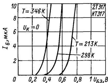
Входные характеристики.
