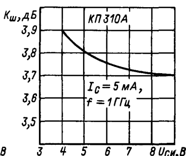
Зависимость коэффициента шума от напряжения сток-исток.
