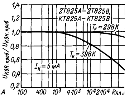
Зависимость относительно пробивного напряжения коллектор-эмиттер от сопротивления база-эмиттер.
