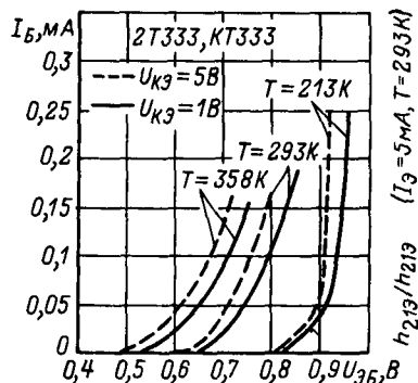
Входные характеристики.
