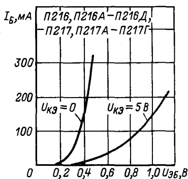
Входные характеристики.
