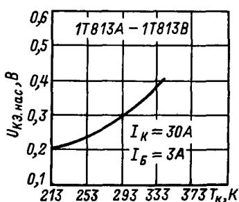
Зависимость напряжения насыщения коллектор-эмиттер от температуры корпуса.
