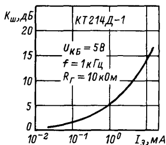
Зависимость коэффициента шума от тока эмиттера.
