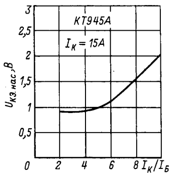
Зависимость напряжения насыщения коллектор-эмиттер от I_K/I_B .
