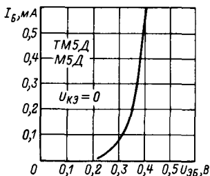
Входная характеристика.
