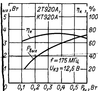
Зависимость выходной мощности и КПД от входной мощности.
