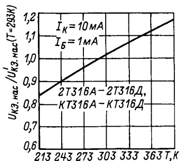
Зависимость относительного напряжения насыщения коллектор-эмиттер от температуры.
