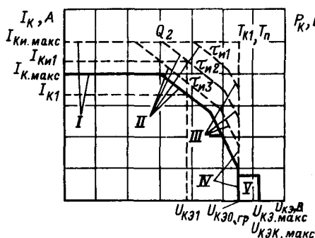
Рис. 2.3. Область максимальных режимов мощного биполярного транзистора.
