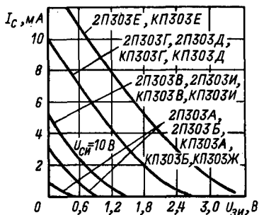
Зависимость тока стока от напряжения затвор-исток.
