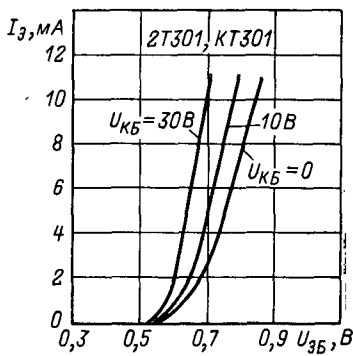
Зависимость тока эмиттера от напряжения эмиттер-база.
