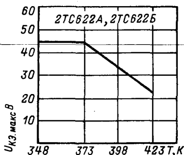
Зависимость максимально допустимого напряжения коллектор-эмиттер от температуры.
