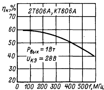
Зависимость коэффициента полезного действия от частоты.
