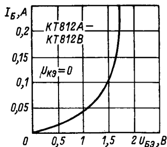
Входная характеристика.
