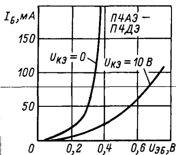
Входные характеристики.
