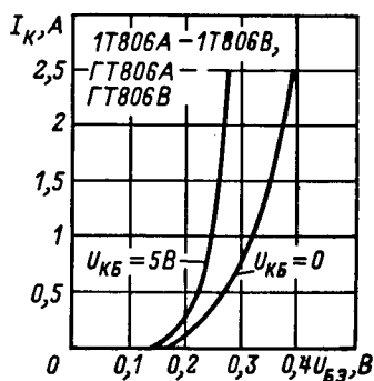
Зависимость тока коллектора от напряжения база-эмиттер.
