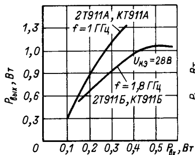
Зависимость выходной мощности от входной.
