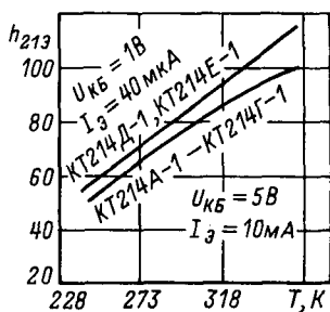
Зависимость статического коэффициента передачи тока от температуры.
