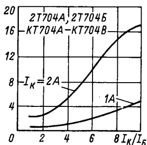
Зависимость напряжения насыщения коллектор-эмиттер, В, от отношения I_K/I_B .
