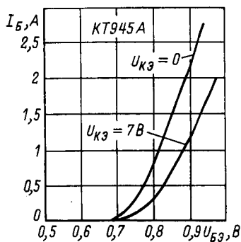
Входные характеристики.
