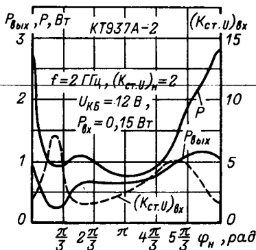
Зависимости выходной мощности, рассеиваемой мощности и коэффициента стоячей волны на входе от фазы коэффициента отражения нагрузки при расфазировании с K_{ст.у} = 2 при сопротивлении автоматического смещения, равном нулю, в режиме оптимальной нагрузки: (K_{ст.у})_{вх} = 1 , P_{вых} = 1.3 Вт, P = 1.6 Вт.
