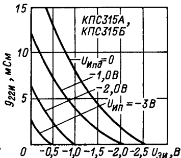
Зависимость выходной проводимости от напряжения затвор-исток.
