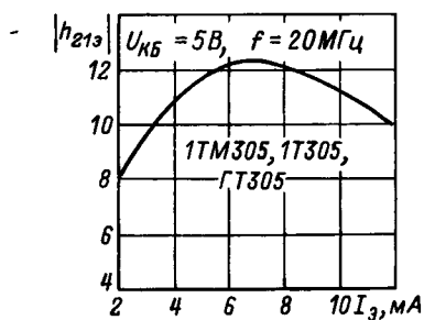
Зависимость модуля коэффициента передачи тока от тока эмиттера.
