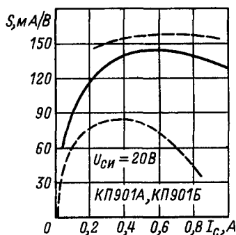
Зона возможных положений зависимости крутизны характеристики от тока стока.
