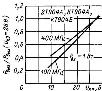
Зависимость относительной выходной мощности от напряжения коллектор-эмиттер.
