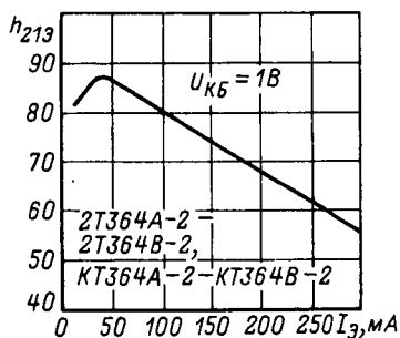
Зависимость статического коэффициента передачи тока эмиттера.
