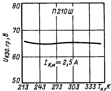
Зависимость граничного напряжения от температуры корпуса.
