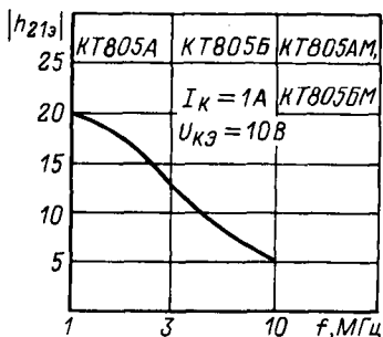
Зависимость модуля коэффици- ента передачи тока от частоты.
