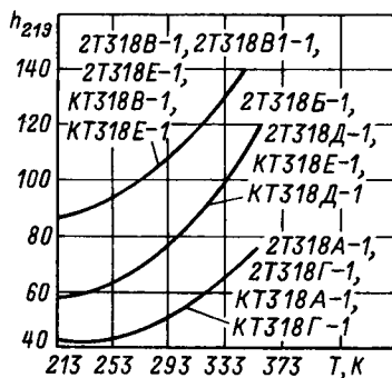
Зависимость статического коэффициента передачи тока от температуры.
