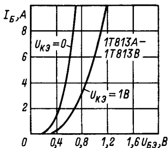
Входные характеристики.
