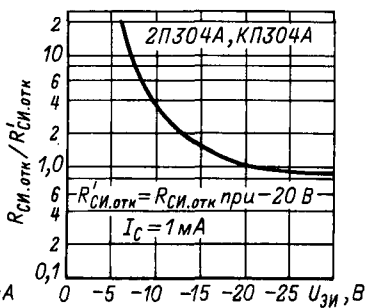
Зависимость относительного сопротивления сток-исток в открытом состоянии от напряжения затвор-исток.
