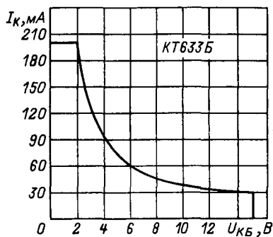
Зависимость тока коллектора от напряжения коллектор-база.
