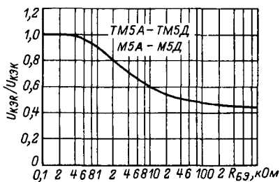
Зависимость относительного напряжения коллектор-эмиттер от сопротивления база-эмиттер.
