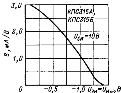
Зависимость крутизны характеристики от напряжения затвор-исток.
