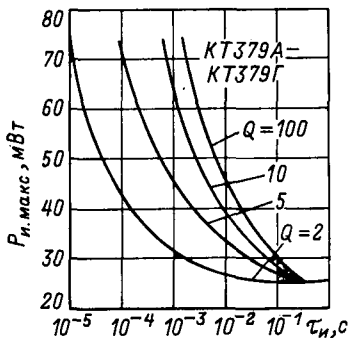
Зависимость максимально допустимой импульсной мощности от длительности импульса.
