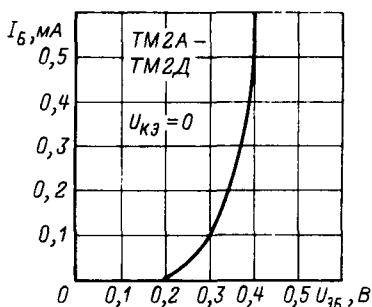
Входная характеристика.
