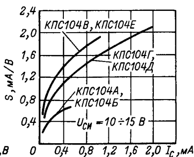
Зависимости крутизны характеристики от тока стока.
