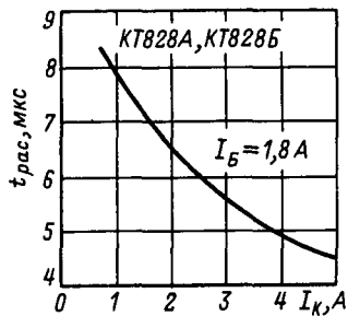
Зависимость времени рассасывания от тока коллектора.
