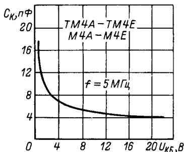
Зависимость емкости коллек- торного перехода от напряже- ния коллектор-база.
