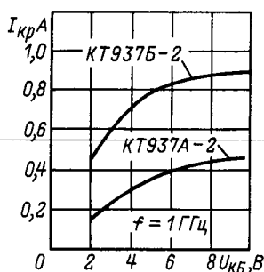
Зависимость критического тока от напряжения коллектор-база.
