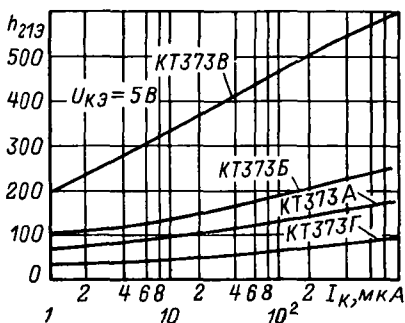
Зависимость статического коэффициента передачи тока от тока коллектора.
