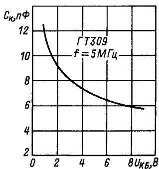
Зависимость емкости коллекторного перехода от напряжения коллектор-база.
