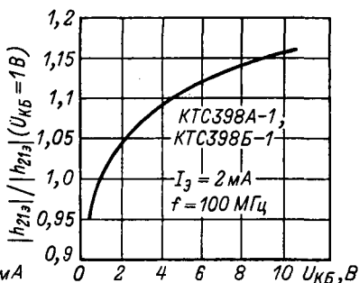
Зависимость относительного модуля коэффициента передачи тока от напряжения коллектор-база.
