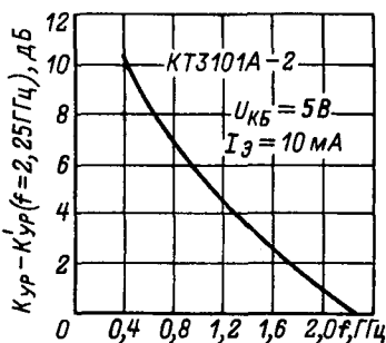
Приведенная зависимость коэффициента усиления по мощности от частоты.
