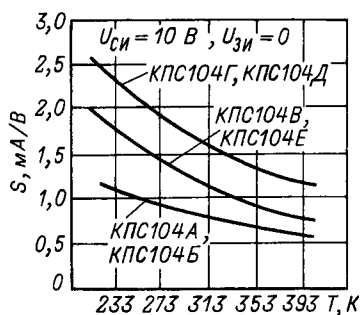
Зависимости крутизны характеристики от температуры.
