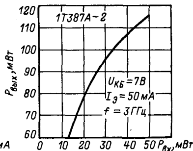
Зависимость выходной мощности от входной в классе С в схеме с общей базой.
