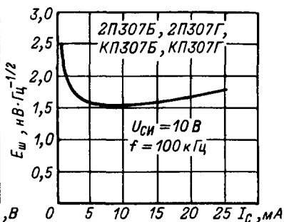
Зависимость ЭДС шума от тока стока.
