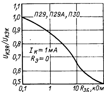
Зависимость относительного постоянного напряжения коллектор-эмиттер от сопротивления в цепи эмиттер-база.
