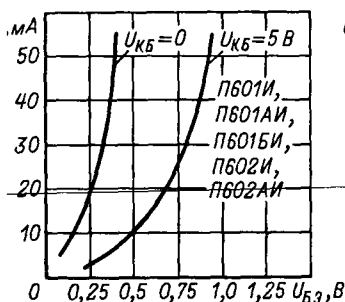
Входные характеристики.
