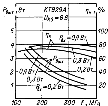
Зависимость выходной мощности и КПД от частоты.
