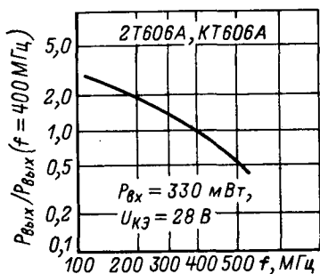
Зависимость относительной выходной мощности от частоты.
