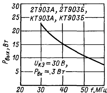
Зависимость выходной мощности от частоты.
