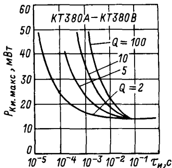
Зависимость максимально допустимой импульсной мощности рассеивания коллектора от длительности импульса.
