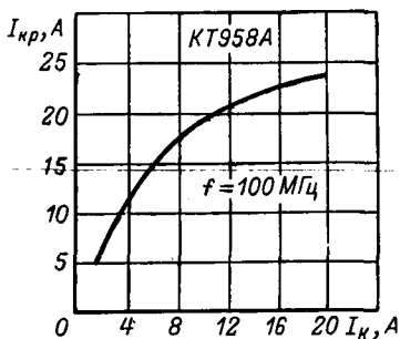
Зависимость критического тока от тока коллектора.
