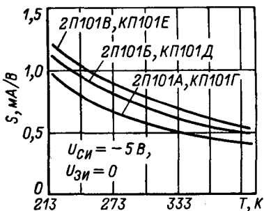
Зависимость крутизны характеристики от температуры.
