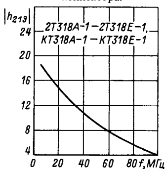
Зависимость модуля коэффициента передачи тока от частоты.
