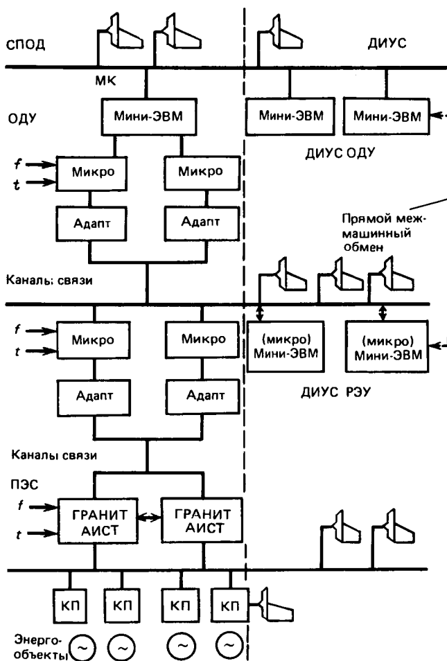
Рис. 3.6. Централизованная информационно-управляющая система:
