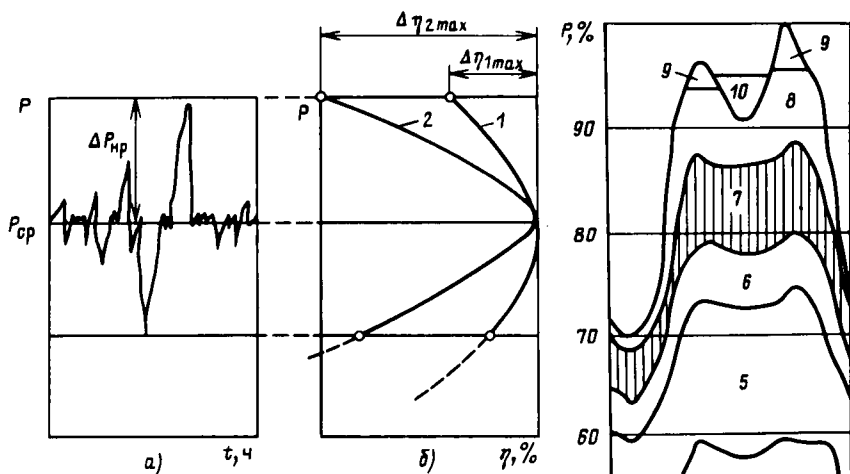
Рис. 1.4. Снижение КПД при регулировании частоты:
