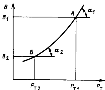
Рис. 6.2. Режим тепловых станций при работе ГЭС с различным расходом воды
