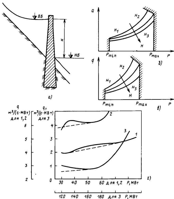
Рис. 7.9. Характеристики гидроагрегата:
