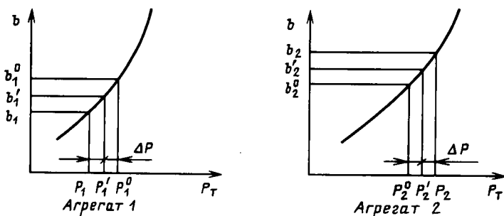
Рис. 6.1. Иллюстрация оптимальности режима при равенстве относительных приростов
