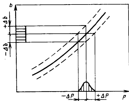
Рис. 11.2. Моделирование случайной характеристики относительных приростов
