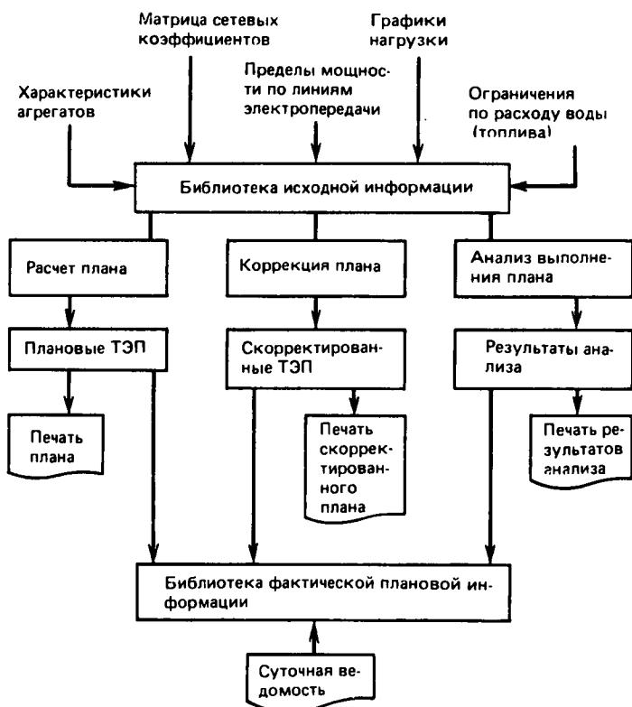
Рис. 10.7. Схема автоматизированных плановых расчетов в энергосистеме
