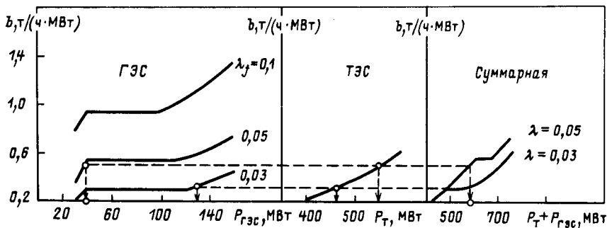
Рис. 6.5. Пример распределения нагрузки между ТЭС и ГЭС
