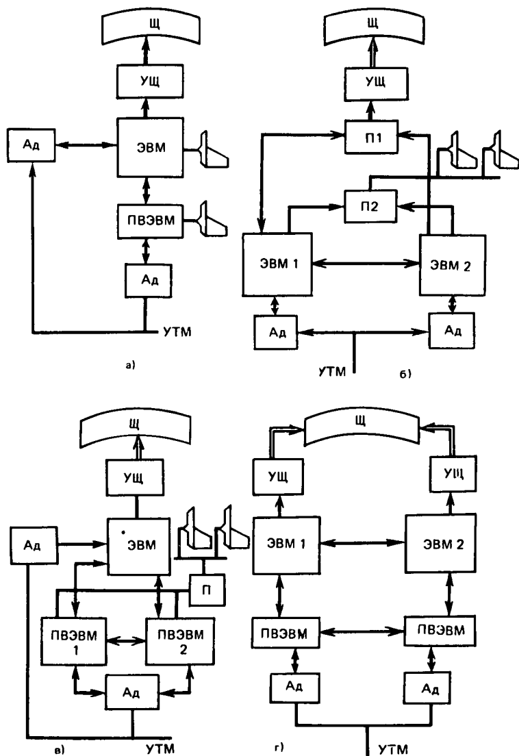
Рис. 4.3. Основные типы ОИК:
