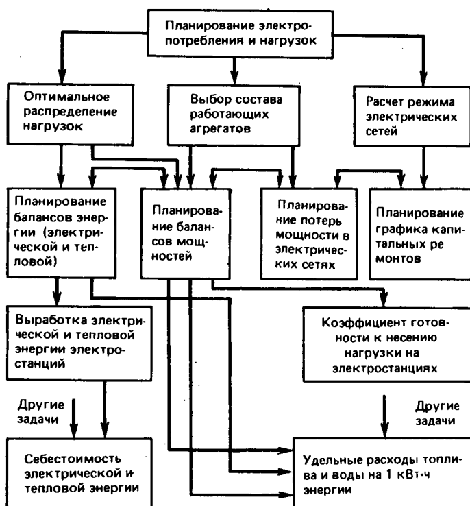
Рис. 10.1. Схема плановых расчетов режимов и технико-экономических показателей системы
