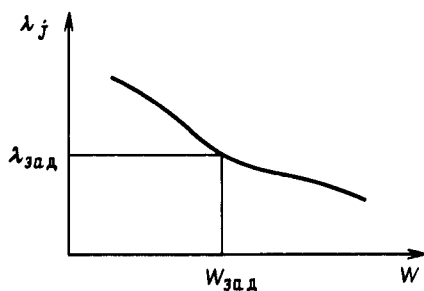
Рис. 6.3. Зависимость \lambda_j от стока воды ГЭС
