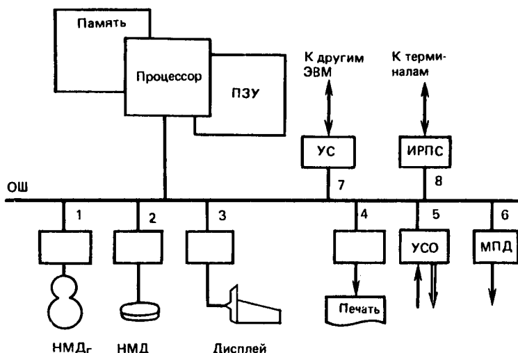
Рис. 2.11. Структурная схема микроЭВМ:
