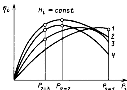
Рис. 8.5. К методике определения оптимального состава агрегатов при равномерном распределении нагрузки
