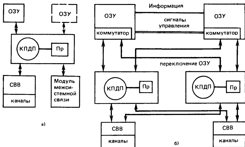
Рис. 2.9. Структурная схема ЭВМ СМ-2м упрощенная:
