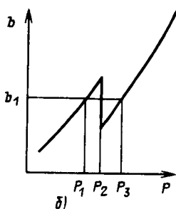
Рис. 7.13. Два вида разрыва непрерывности на характеристиках относительных приростов
