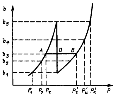
Рис. 7.15. Устранение разрыва непрерывности на характеристике относительных приростов
