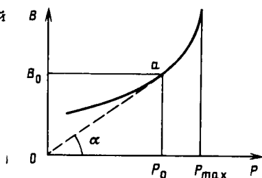
Рис. 8.2. К определению экономической мощности агрегата
