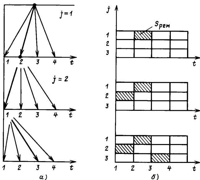
Рис. 9.6. Схема вариантных расчетов при построении графика ремонтов оборудования:
