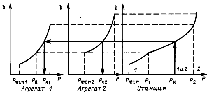
Рис. 7.12. Эквивалентная характеристика двух агрегатов
