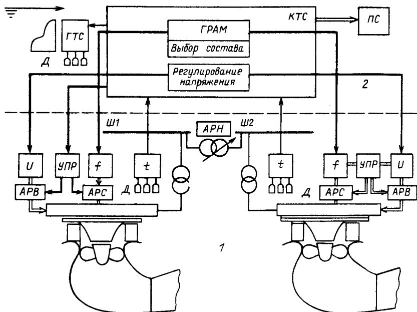
Рис. 4.16. Технические средства АСУ ГЭС:
