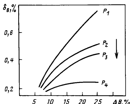
Рис. 11.3. Влияние погрешностей расходных характеристик агрегатов на эффективность оптимизации режимов:
