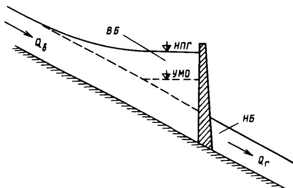
Рис. 9.1. Иллюстрация терминов, применяемых для ГЭС:
