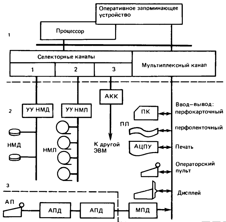
Рис. 2.6. Принципиальная схема машины ЕС ЭВМ:
