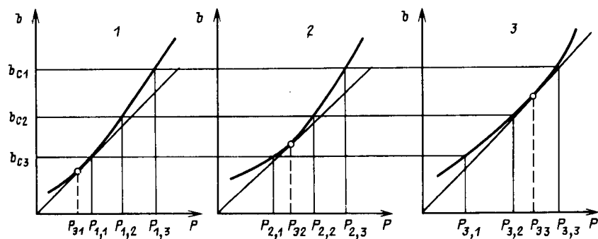
Рис. 8.3. Определение состава агрегатов с использованием критерия выгоды отключения:
