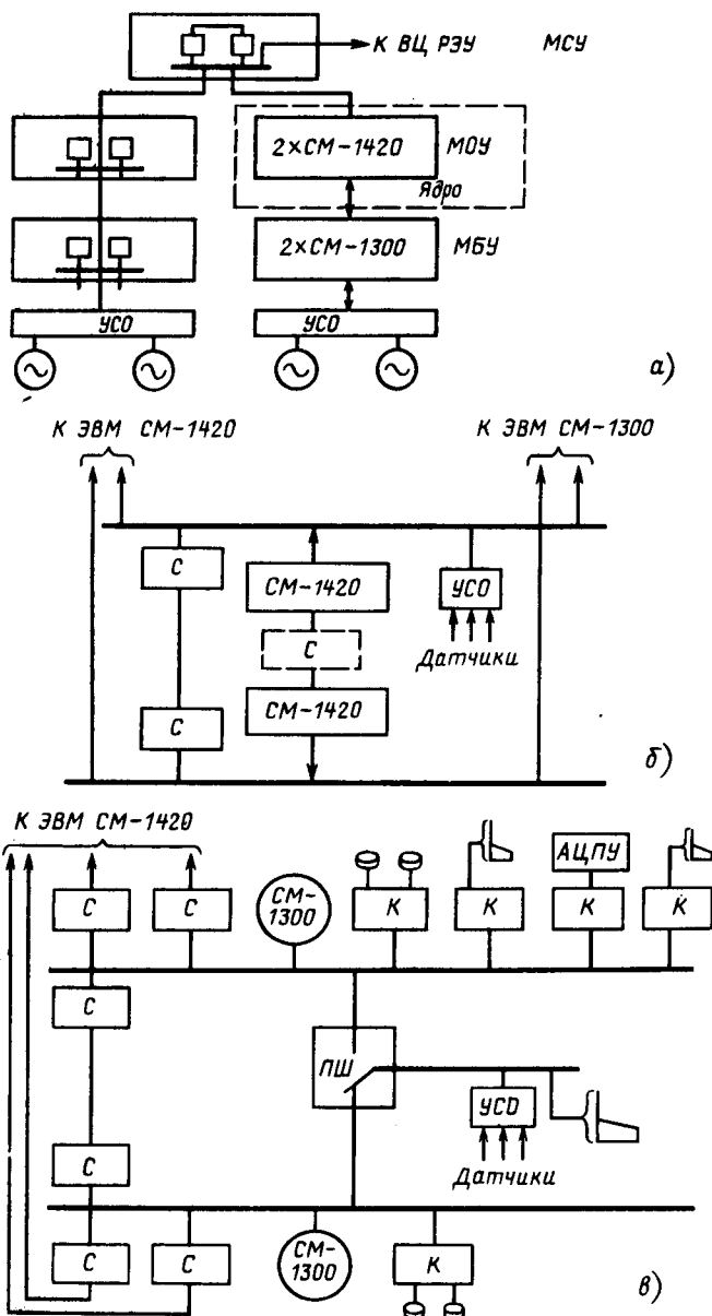
Рис. 4.9. Комплекс технических средств АСУ ТП крупной ТЭС, использующий CM-1420:
