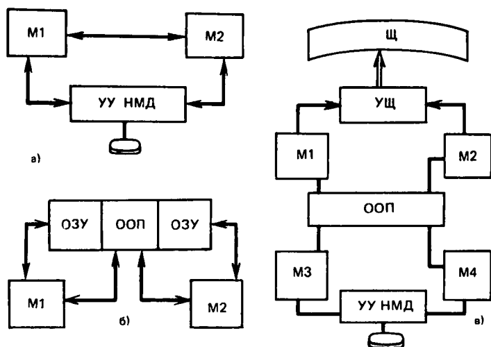
Рис. 4.4. Работа ЭВМ на общее поле памяти:
