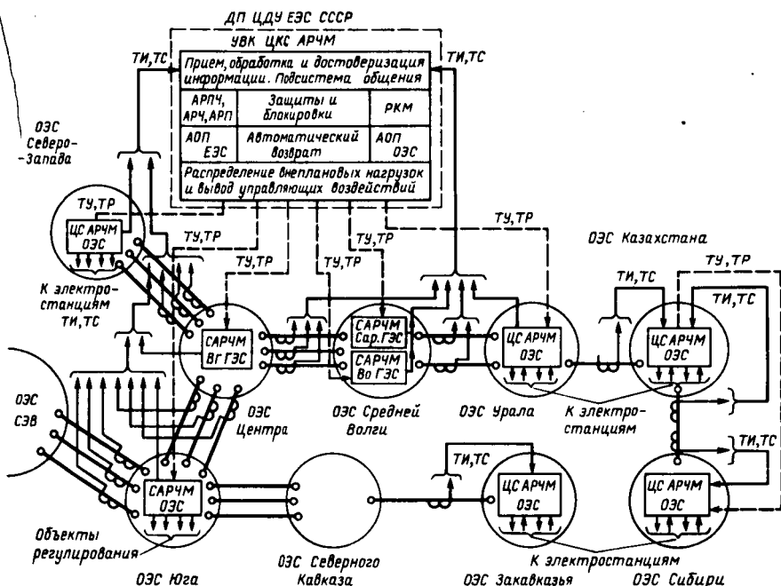
Рис. 6.11. Схема системы регулирования частоты и активной мощности в ЕЭС СССР
