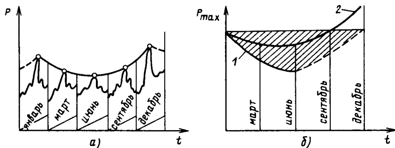
Рис. 1.2. Ход годовых максимумов нагрузки:
