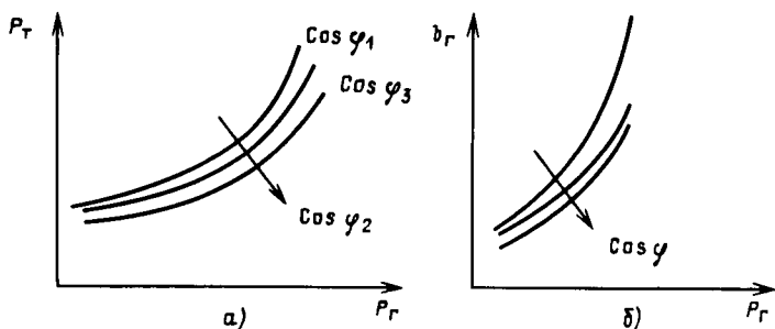
Рис. 7.7. Характеристики генератора: а — абсолютных показателей; б — дифференциальная
