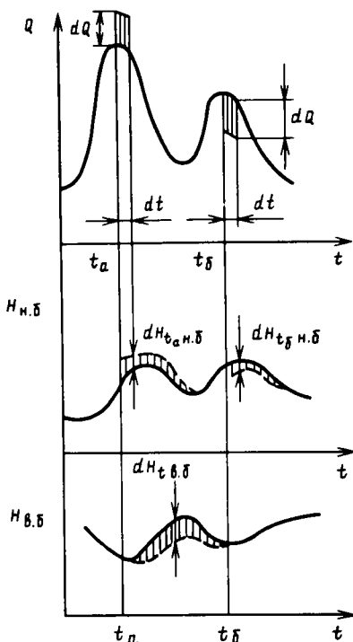
Рис. 6.6. Влияние режима расходов ГЭС на напор
