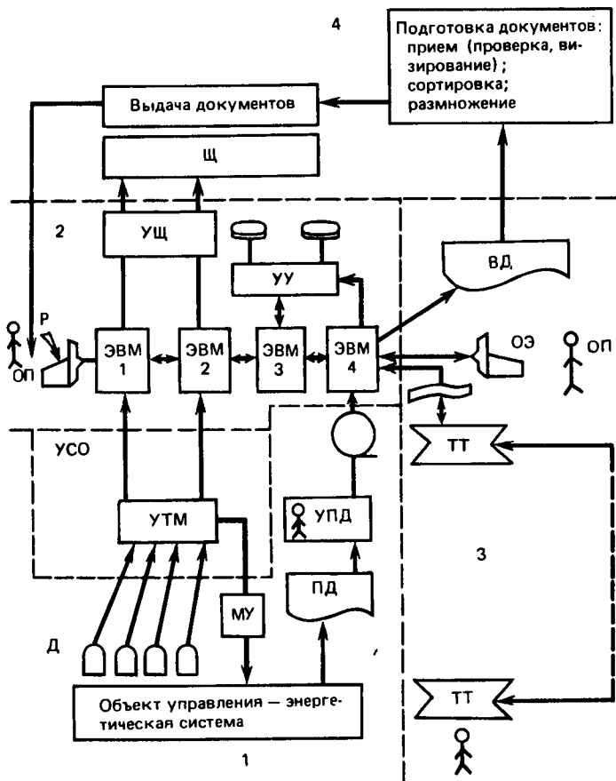
Рис. 4.2. Комплекс технических средств АСУ ЭЭС:
