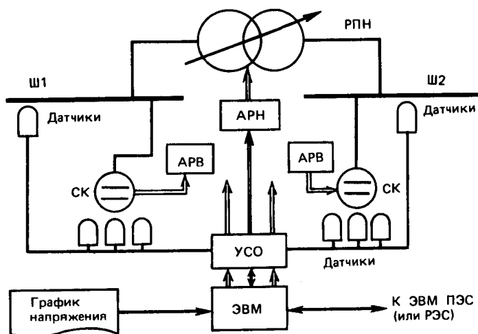
Рис. 4.22. Управление реактивной мощностью на подстанции:
