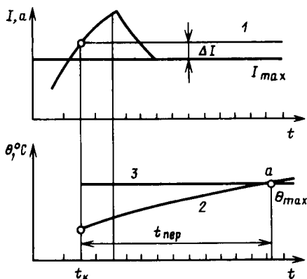
Рис. 4.21. Контроль перегрузки трансформаторов в АСУ ТП
