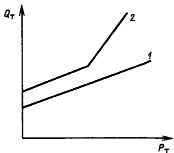
Рис. 7.5. Расходные характеристики турбин ТЭС:
