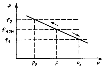
Рис. 6.9. Характеристики регуляторов оборотов РО
