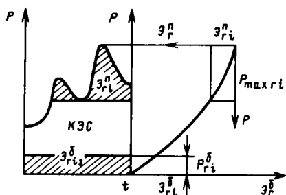
Рис. 9.4. Определение режима ГЭС по интегральной кривой нагрузки
