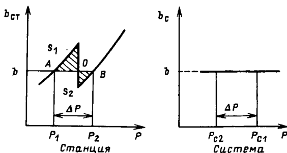
Рис. 7.14. К методике устранения разрыва непрерывности характеристики относительных приростов
