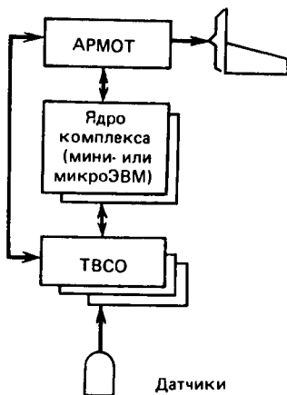
Рис. 4.8. Комплекс технических средств АСУ ТП ТЭС с децентрализованной системой сбора информации
