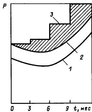
Рис. 1.3. Баланс мощности энергосистемы:
