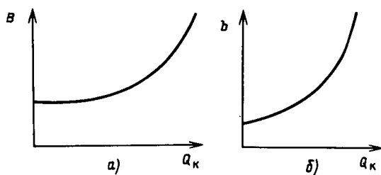
Рис. 7.4. Характеристики котла ТЭС:
