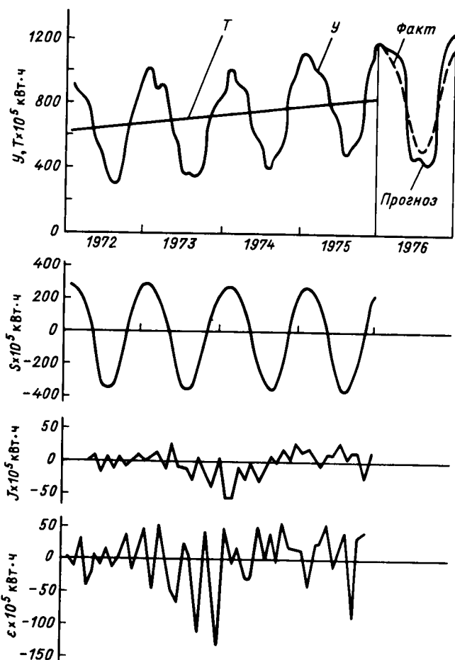
Рис. 10.4. Временной ряд потребления электроэнергии на собственные нужды ГЭС:
