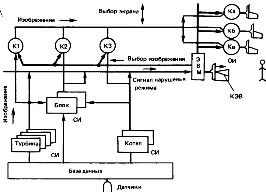
Рис. 4.10. Автоматизация выдачи и отображения технологической информации в АСУ ТП ТЭС:
