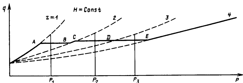
Рис. 7.16. Дифференциальные характеристики ГЭС: z – число агрегатов
