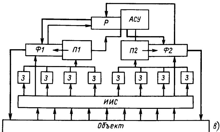
Рис. 2.1. К понятию структуры АСУ:
