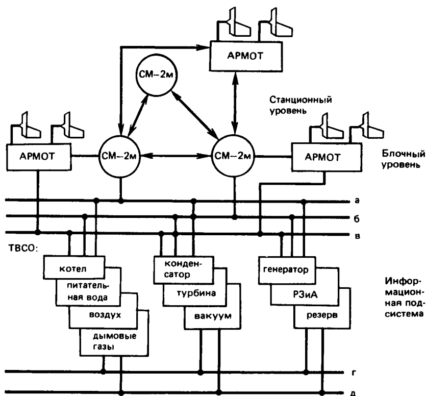
Рис. 4.14. Пример КТС энергоблока 800 МВт
