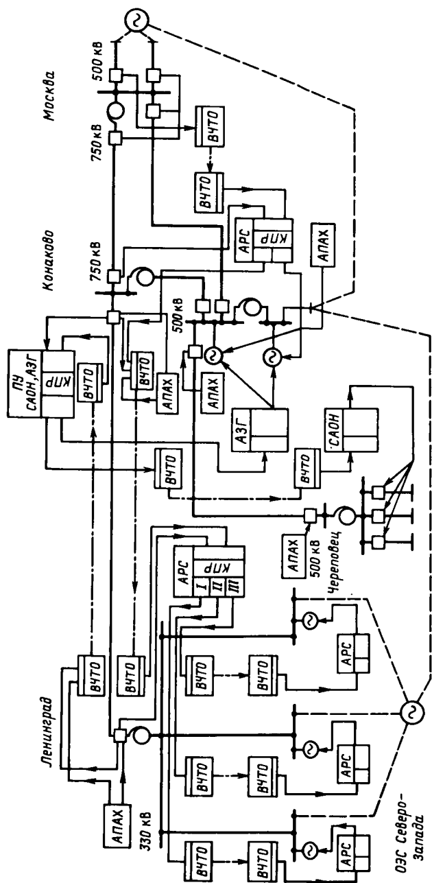
Рис. 6.12. Схема противоаварийной автоматики межсистемных связей ОЭС Северо-Запада и Центра:
