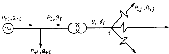
Рис. 6.7. Узел электрической системы
