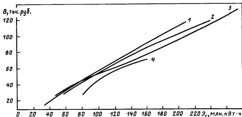
Рис. 7.19. Статистические характеристики зависимости расхода топлива ТЭС от выработки электрической энергии:
