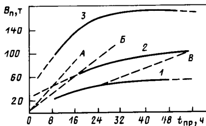
Рис. 8.1. Зависимость пускового расхода условного топлива от времени простоя:
