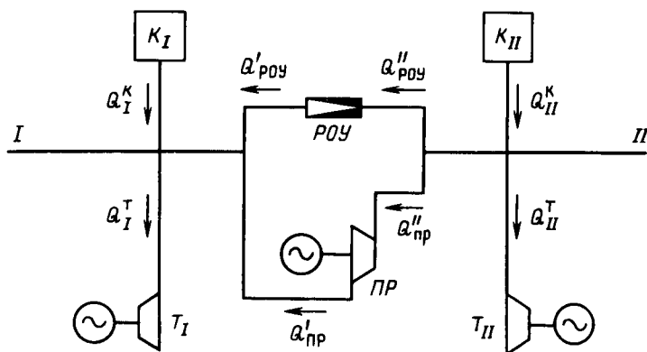
Рис. 7.17. Схема тепловой станции
