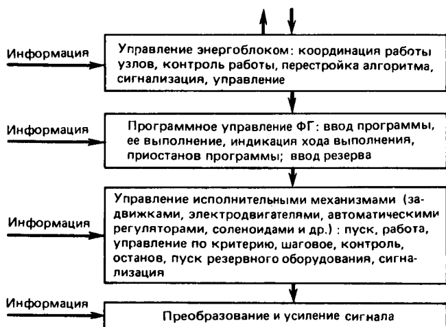
Рис. 4.11. Трехуровневая система функционально-группового управления блоком
