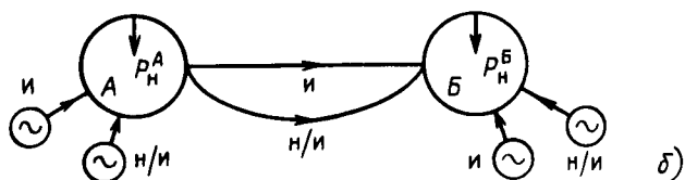
Рис. 4.7. Организация оперативного контроля баланса мощности:
