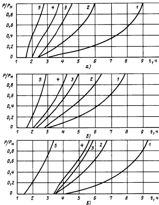
Рис. 7.10. Характеристики нормативной положительности пусков некоторых моблоков с пылеугольными котлами:
