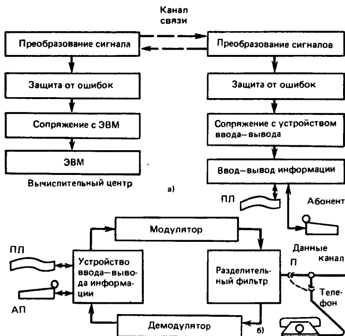
Рис. 3.8. Схема организации связи абонентского пункта с ЭВМ: а — схема соединения абонента с ВЦ; б — схема стационарного модема
