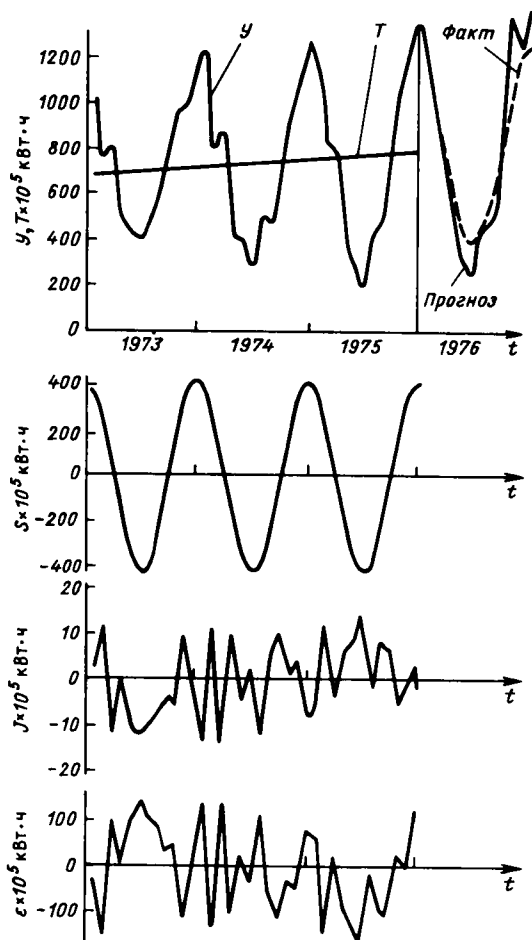
Рис. 10.3. Временной ряд электропотребления районной системы :
