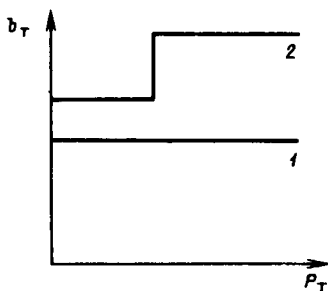
Рис. 7.6. Дифференциальные характеристики турбин ТЭС:
