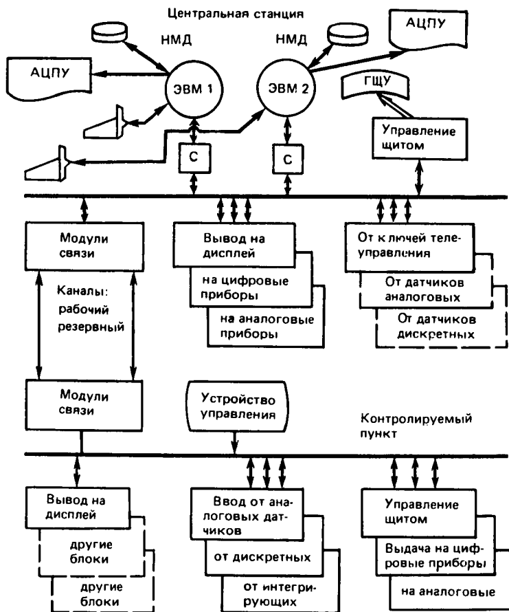
Рис. 3.5. Телеинформационная система ГРАНИТ
