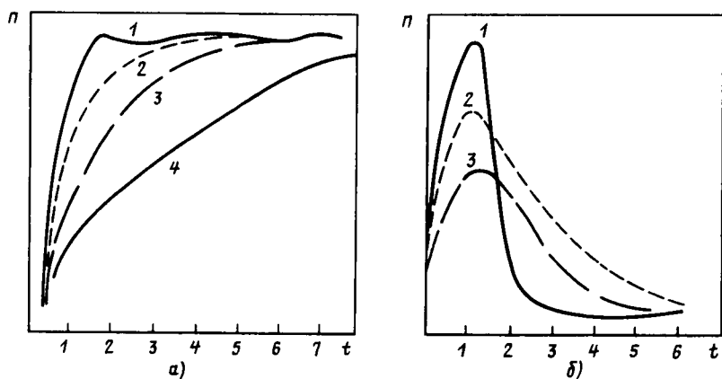
Рис. 3.3. Работа сглаживающего фильтра:
