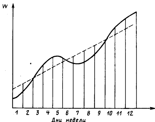
Рис. 10.5. Недельные временные ряды суточного потребления электроэнергии в системе
