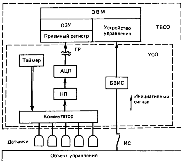
Рис. 3.2. Организация сбора информации с датчиков:
