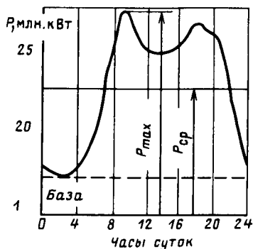
Рис. 1.1. Пример суточного графика нагрузки
