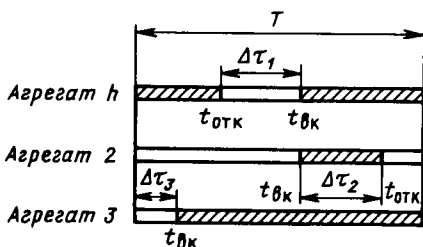
Рис. 8.7. Диаграмма работы агрегатов для расчета пусковых расходов
