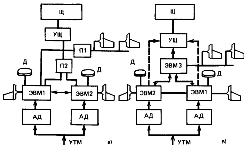
Рис. 4.17. Комплекс технических средств ПЭС АСУ:
