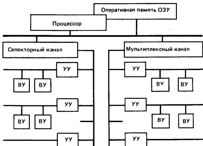
Рис. 2.5. Структура машины Единой системы: ВУ — внешнее устройство; УУ — устройство управления
