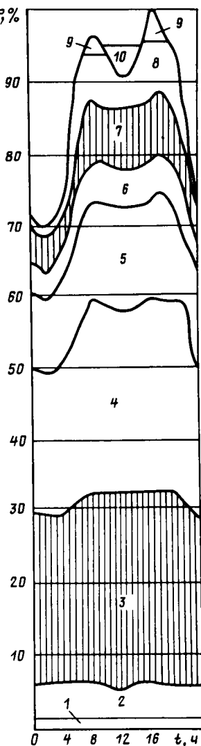
Рис. 1.4. Снижение КПД при регулировании частоты:
