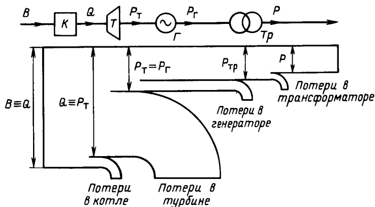
Рис. 7.3. Ленточная диаграмма режимных потерь блока ТЭС
