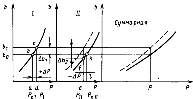
Рис. 11.1. Влияние погрешностей характеристик на распределение нагрузки
