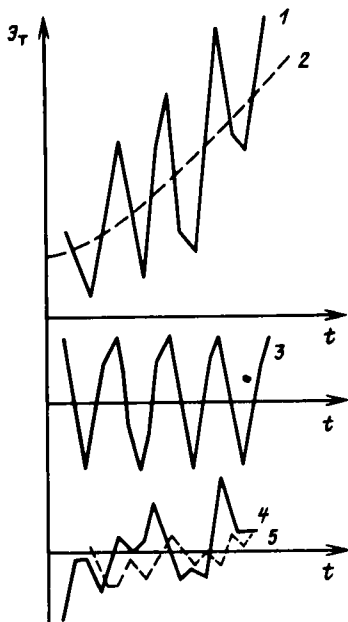
Рис. 10.2. Временной ряд и его составляющие: 1 — исходный ряд ( Y ); 2 — основной тренд ( T ); 3 — сезонная составляющая ( S ); 4 — авторегрессия ( J ); 5 — остатки ( \varepsilon )
