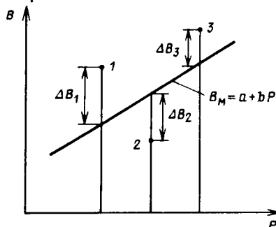
Рис. 7.18. Иллюстрация к методу наименьших квадратов
