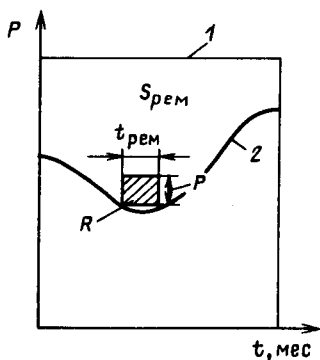
Рис. 9.5. К определению ремонтной площади в годовом графике:
