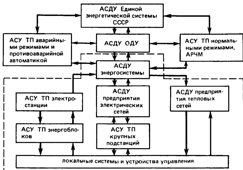
Рис. 4.6. Уровни управления и подсистемы АСДУ
