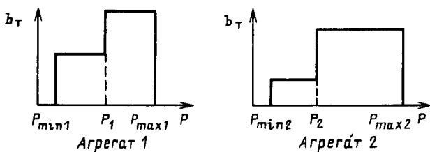
Рис. 6.8. К распределению нагрузки при ступенчатых характеристиках агрегатов
