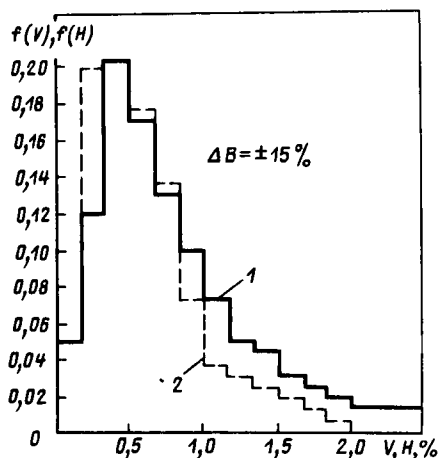
Рис. 11.4. Гистограмма перерасхода топлива в зависимости от погрешностей расходных характеристик агрегатов:
