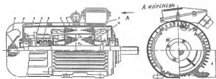
32.4-rasm. 4PO seriyali o'zgaras tok motorining bo'ylama va ko'ndalang qirqimlari:
