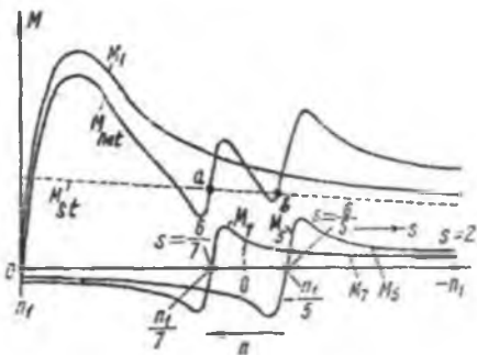
12.6-rasm. Maydonning yuqori (5 va 7) garmonikalari va 1-garmonikasi (asosiy maydon) hosil qilgan asinxron momentlar ( M_{st} , M_5 va M_7 ) hamda natijaviy asinxron moment ( M_{nat} ); M_{st} — statik moment.
