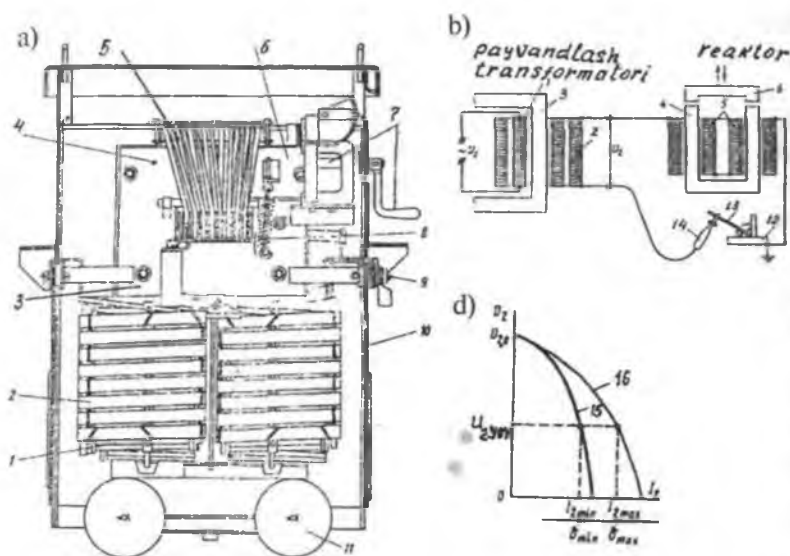
9.2-rasm. STN-500-1 tipli payvandlash transformatorining tuzilishi (a) va ishingining prinsipial sxemasi (sxemada reaktor ajratib ko'rsatilgan) (b): [1, 2 – tegishli YK va PK chulg'amlar; 3 – magnit o'tkazgich; 4, 6 – reaktor magnit sistemasining qo'zg'almas (4) va qo'zg'aluvchi (6) qismlari; 5 – reaktor chulg'ami; 7 – qo'zg'aluvchi qismni harakatga keltirish uchun dastakli yurituvchi vint; 8 – qo'zg'aluvchi qismning titrashini kamaytirish uchun prujina; 9 – ikkilamchi chulg'am va reaktor chulg'ami qisqichi; 10 – kojux; 11 – g'ildirak; 12 – payvandlanadigan detal; 13 – elektrod; 14 – tokli simning izolatsion tutqichi]; payvandlash transformatorining tashqi xarakteristikalar (d): [minimal (1) va maksimal (2) zazorlar uchun; U_{2, \text{yoy}} – elektr yoyining turg'un yonishi uchun zaruriy kuchlanish].
