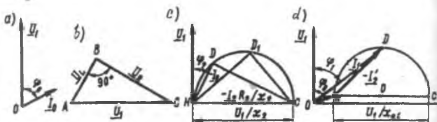
13.1-rasm. Asinxron motorning doiraviy diagrammasini asoslashga doir chizmalar.
