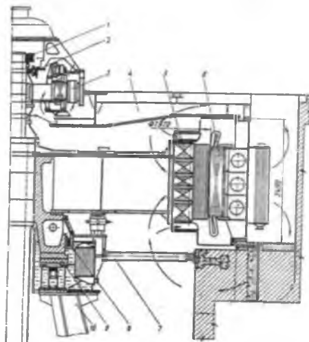
34.10-rasm. VGS 850/135-56 tipli soyabonsimon bajarilgan bir yo'naltiruvchi podshipnikli takomil-lashtirilgan konstruksiyali (hunda: 1 – kontakti halqalar; 2 – rostlash generatori; 3 – qo'zg'atgich; 4 – yuqorgi krestovina, ya'ni bir-biriga ko'ndalang chalishtirilgan detal"; 5 – rotor; 6 – stator; 7 – tirgo-vich; 8 – yo'naltiruvchi podshipnik; 9 – tayanchostligi; 10 – konussimon tayanch) gidrogeneratorning radial sistemali ventilatsiya sxemasi.
