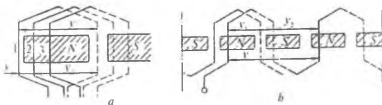
10.7-rasm. Sirtmoqsimon ( a ) va to'liqinsimon ( b ) chulg'amlarning seksiyalari.
