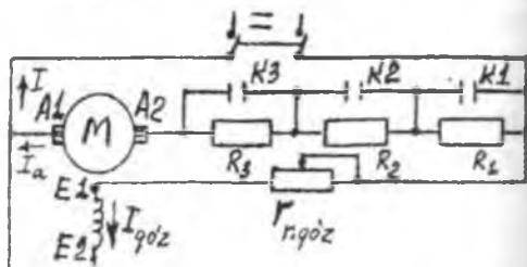
31.3-rasm. Avtomatlashtirilgan elektr yuritmasida parallel qo'zg'atishli O'TM ni ishga tushirishning prinsipial sxemasi.
