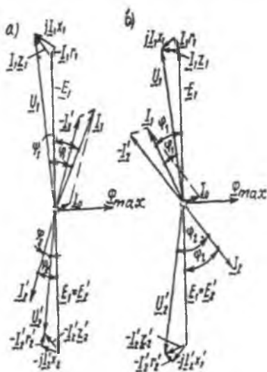
4.1-rasm. Transformatorning aktiv-induktiv (a) va aktiv-sig'imiyy (b) yuklamalar uchun vektor diagrammalari.
