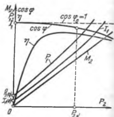
24.4-rasm. Sinxron motorning xarakteristikalari.
