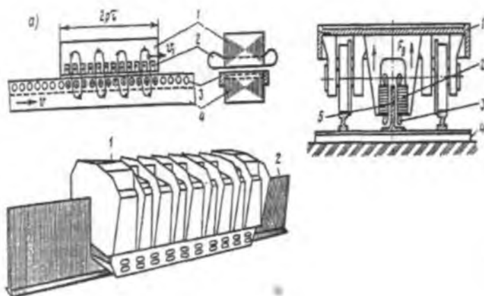
17.5-rasm. Chiziqli asinxron motorning: a —elektromagnit sxemas (bunda: 1 — stator, 2 — uch fazali chulg'am; 3— qisqa tutashgan chulg'am, 4 — o'zak); b — temiryo'l transportining harakatlanuvchi qismi (1)da o'rnatish sxemasi (bunda: 2 — stator, 3 — chulg'am, 4 — uzun po'lat tilimi 5 ni relslar orasida mahkamlash uchun moslama); d — umumiy ko'rinishi (bunda: 1 — stator, 2 — uzun po'lat tilimi, ya'ni shinasi); F_k — chegaraviy effekt tufayli hosil bo'ladigan ko'ndalang kuch.
