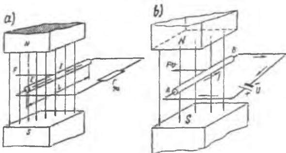
K.2-rasm. Elektr mashinalarida mexanik energiyaning elektr energiyaga (a) va elektr energiyaning mexanik energiyaga (b) aylantirilishiga oid chizmalar.
