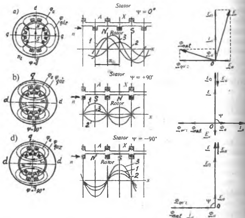
19.1-rasm. Noayon qutbli sinxron mashinada turli (a – aktiv, b – induktiv va c – sig'imiyy) xarakterli yuklamadagi magnit oqimlar ( \Phi_{\psi z} – qo'zg'atish oqimi va \Phi_a – yakor reaksiyasi oqimi), magnit induksiyalari (1 – qo'zg'atish chulg'ami induksiyasi B_{\psi z} , 2 – yakor chulg'ami induksiyasi B_a va 3 – natijaviy induksiya B_{nat} ) ning taqsimlanish egri chiziqlari hamda vagnit oqimlar va EYklarning vektor diagrammalari; \Phi_{nat} – natijaviy oqim.
