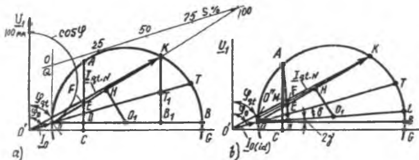
13.3-rasm. Asinxron motorining soddalashgan (a) va aniqlashtirilgan (b) doiraviy diagrammalarini salt ishlash va qisqa tutashuv tajribalari ma'lumotlari bo'yicha qurish; I_{0(id)} — ideal salt ishlash toki
