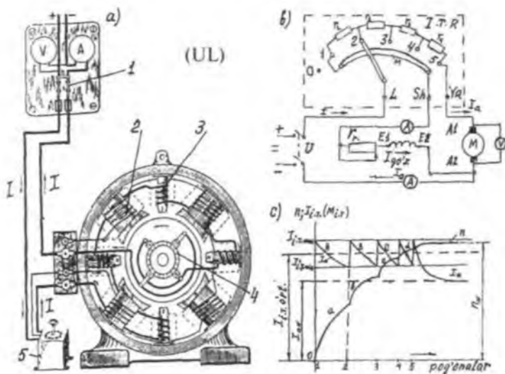
31.2-rasm. Parallel qo'zg'atishli o'zgarmas tok motorda: a - tajri o'tkazish qurilmasi (bunda: 1 – ulab uzgich (UL); 2 – qo'zg'atish chulg'an; 3 – qo'shimcha qutb chulg'ami; 4 – kollektor; 5 – ishga tushirish reostat b – motorni ishga tushirish sxemasi (ITR – ishga tushirish reostati, M – mis yoyi); d – «reostatli» ishga tushirish jarayonidagi tok, moment va aylan chastotalarining o'zgarish xarakteri.
