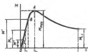
12.2-rasm. Asinxron mashinaning motor, generator va elektomagnet tormoz rejimlari uchun mexanik xarakteristikalari (a, b) — M = f(s) .
