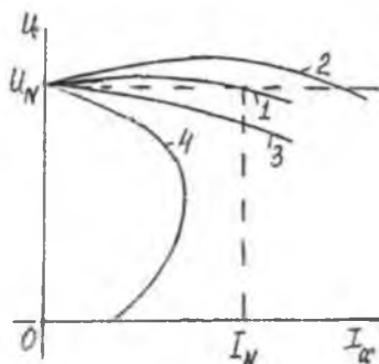
30.6-rasm. Aralash qo'zg'atishli generatorning tashqi xarakteristikallari (1; 2; 4); 3 — parallel qo'zg'atishli uchun (taqqoslash uchun keltirilgan).
