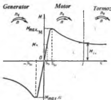
12.2-rasm. Asinxron mashinaning motor, generator va elektomagnet tormoz rejimlari uchun mexanik xarakteristikalari (a, b) — M = f(s) .
