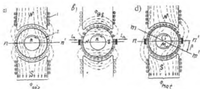
28.1-rasm. O'zgarmas tok mashinasining magnit maydoni: a) qo'zg'atish chulg'aming maydoni F_{02} , 1 – qo'zg'atish chulg'ami, 2 – yakor; b) yakor chulg'aming maydoni F_{01} ; d) mashinaning natijaviy magnit maydoni F_{01} .
