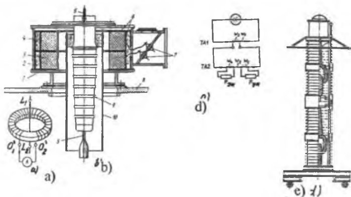
9.7-rasm. Kuchlanishi 110 kV bo'lgan kuch transformatori bakining ichiga o'rnatilgan tok transformatorining ulanish sxemasi (a): L_1 va L_2 — birlamchi chulg'am uchlari; O_1 va O_2 — ikkilamchi chulg'am uchlari; b) tok transformatorining konstruksiyasi: 1 — kiritgichning o'tish flanetsi (birlashtiruvchi qismi); 2 — qora qayindan yasalgan plastina; 3, 4 — tok transformatorlari; 5 — birinchi chulg'am vazifasini bajaruvchi o'tkazgich; 6 — elektrokarton izolatsiya; 7 — ikkilamchi chulg'am o'tish izolatori qisqichi; 8 — bak qopqog'i; 9 — moy to'ldirilgan kiritgich; 10 — qog'oz-bakelitli silindr; d) kaskadli tok transformatorining sxemasi; e — kaskadli tok transformatori.
