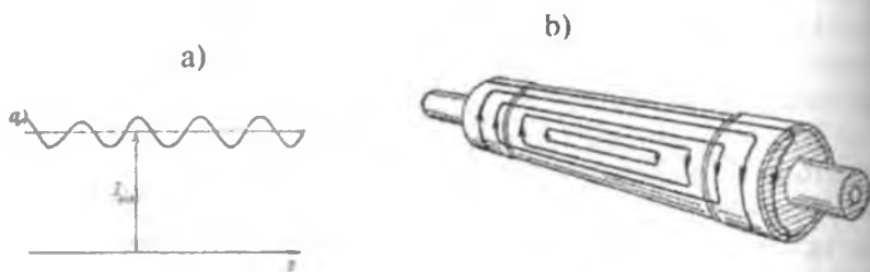
21.2-rasm. Sinxron generatorning nosimmetrik yuklamasida qo'zg'atish chulg'ami tokining o'zgarish shakli (a) va turbogenerator rotorida teskari ketma-ketlik maydoni hosil qilgan toklar o'tadigan yo'llar sxemasi (b).
