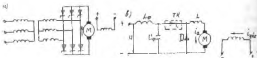
31.13-rasm. Boshqariladigan to'g'rilagichdan ta'minlanadigan mustaqil qo'zg'atishli motorning aylanish chastotasini rostlash sxemasi (a) va o'zgaras tok motorini impulsli rostlash (b): \alpha S_f — kirish filtri (tozalagichi); TK — tiristorli kalit; D — teskari diod; L_f — induktivlik.
