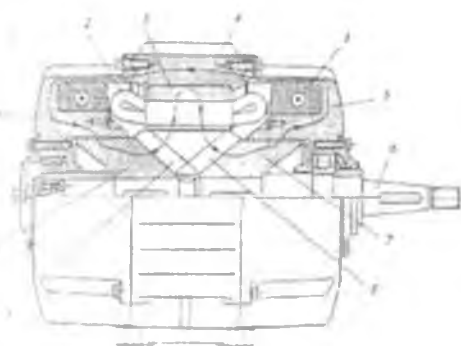
26.3-rasm. Rotori changalsimon qutblardan iborat bo'lgan kontaksiz sinxron generator, bunda: 1 – halqasimon qo'zg'atish g'altaklari; 2 – yakor chulg'ami; 3 – yakorning magnit o'tkazgichi; 4 – stanina (tana gardishi); 5, 11 – podshipnik qalqonlari; 6 – val; 7, 10 – janubiy va shimoliy qutblarning yarmosi; 8, 9 – janubiy va shimoliy qutblar.
