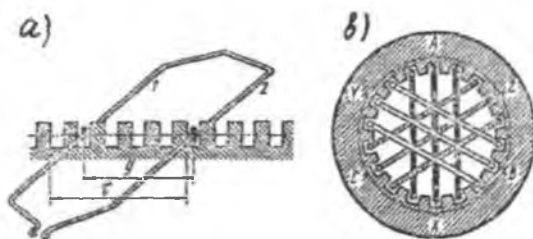
10.4-rasm. Ikkita o'tkazgichdan hosil bo'lgan o'ram (a) va uch fazali chulg'am g'altaklarining statorda joylashishi (b)
