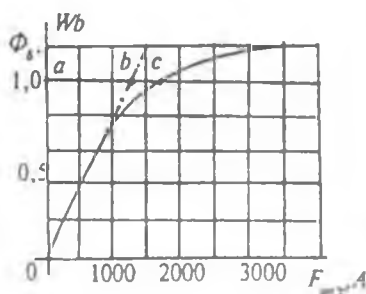
33.3-rasm. O'zgarmas tok mashinasining magnit xarakteristikasi.
