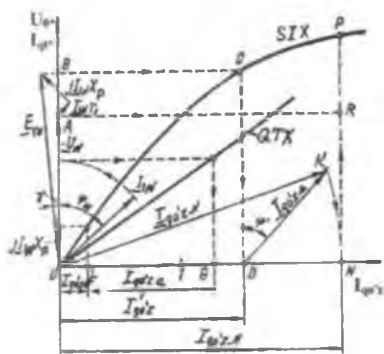
20.3-rasm. Sinxri generator EYK larining amc (Pote) diagrammasi.
