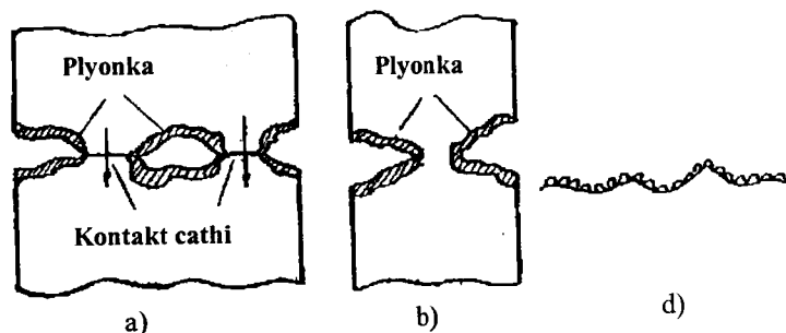
3.2-rasm. Tutashish vaqtidagi fizik hodisalar.
