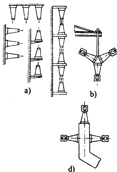
8.13-rasm. Yuqori kuchlanish o'tkazgichlariga misollar: a — tekis joylashgan shinalar; b — osma shina; d — uchburchak shaklidagi tayanch shinalar.
