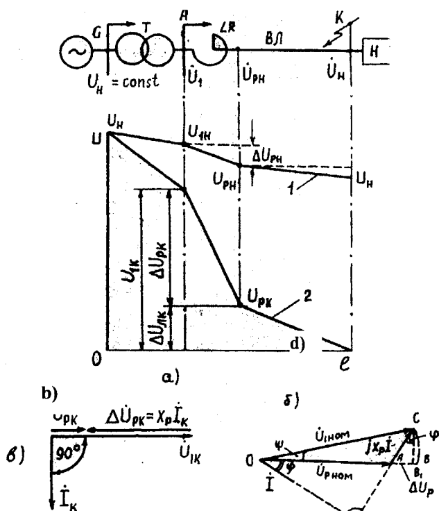
2.18-rasm. Elektra taʼminoti va QT va yuklanish davridagi kuchlanishlar taqsimoti sxemalari (a); normal rejimdagi reaktor kuchlanishlari vektor diagrammalari (b); b — holatning QT davridagi vektor diagrammalari (d).
