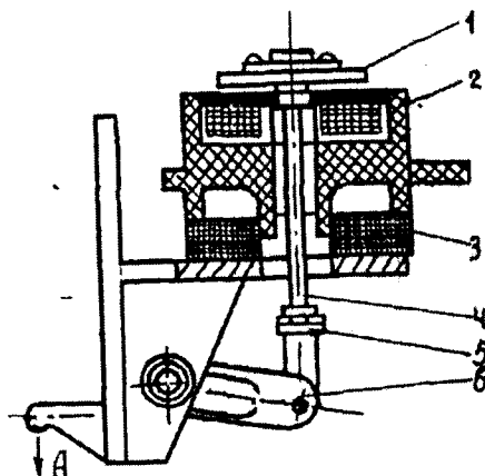
6.10-rasm. VAT—42 turdagi uzgichning induksiya — dynamik yuritmasi: 1—disk; 2—g'altak; 3—qatlam; 4—tortgich; 5—gaykalar; 6—richag.
