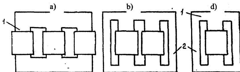
9.2-rasm. Transformatorning magnit tizimi: a — uch fazali sterjenli; b — bir fazali bronozakli; v — bir fazali bronli; 1 — o'zaklar; 2 — yarmo.
