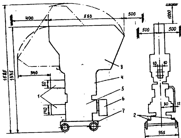
6.12-rasm. VAB — 43—4000/10—K turidagi katodli tezkor avtomatik uzgich: 1—chiquvchi shinalar; 2—yerlatish bolti; 3—yoy soʻndirgich kamera; 4—asosiy kontaktlar bloki; 5—elektromagnitli mexanizm; 6—blokirlochi kontaktlar; 7—aravacha.
