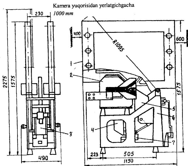
6.2-rasm. VAB— 28 turidagi tezkor uzgichning umumiy ko'rinishi: 1 — yoy so'ndirgich kamera; 2 — qo'zg'almas kontakt; 3 — magnit o'tkazgich; 4 — yakor; 5 — qo'zg'aluvchi kontakt; 6 — korpus; 7 — ushlab turuvchi kontakt.
