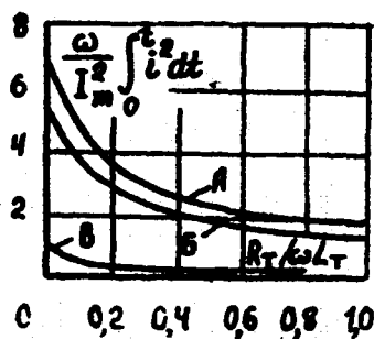
9.36-rasm. Avariya toki birinchi yarim to'liqini ekvivalent issiqlik ta'sirining teskari kuchlanishi maksimal qiymatidagi diagrammalari:
