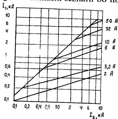
8.3-rasm. PKT turidagi saqlagichning tok cheklash tavsifi: I_1 — saqlagichdan o'tadigan eng katta tok qiymati; I — nominal toki 2 — 50 A bo'lgan eruvchi elementning hisobiy qisqa tutashish toki.
