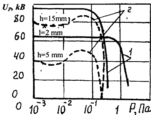
5.18-rasm. Vakuum oralig'i elektr puxtaligining qoldiq gazlar bosimiga bog'liqligi: 1 – bir jisimli maydondagi razryad (elektrodlar kislorodsiz misdan bo'lib, oralig'i 1 ga teng); 2 – pleksiglas silindr yuzalaridagi razryad (silindr diametri 25 mm va balandligi h ga teng, ular bir jinsli maydonda nikellangan elektrodlar orasiga joylashgan).
