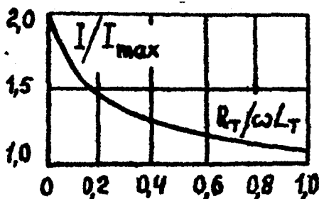
9.28-rasm. Tashqi qisqa tutashgan to'g'rilagich avariya tokning R_T/\omega L_T ga bog'liqlik diagrammasi.
