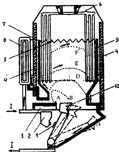
5.6-rasm. Yoy so'ndirgich kameraning konstruktiv sxemasi: 1 — qo'zg'aluvchi kontakt; 2 — qo'zg'almas kontakt; 3, 10 — yoy so'ndirgich kontaktlar; 4 — kamera; 5 — P simon magnit o'tkazgich; 6 — yoy so'ndirgich g'altak; 7, 9 — yoy so'ndirgich shoxchalar; 11, 12 — plastinalar; 13 — qatlam.
