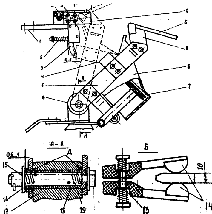
5.10-rasm. Elektromagnitli uzgichning konstruktiv sxemasi: 1— kontakt korpusi; 2,13 — prujina; 3 — asosiy qo'zg'almas kontakt; 4 — asosiy qo'zg'aluvchi kontakt; 5 — shina; 6 — sharnirli kontakt; 7 — porshen; 8 — havo puflagich silindri; 9 — yoy so'ndirgich qo'zg'almas kontakt; 11— plastina; 12 — vint; 14 — yoyso'ndirgich qo'zg'aluvchi kontakt; 15 — gayka; 16 — shayba; 17— kontakt; 18 — vtulka; 19 — prujina; a — «ulangan» holat; b — «uzilgan» holat.
