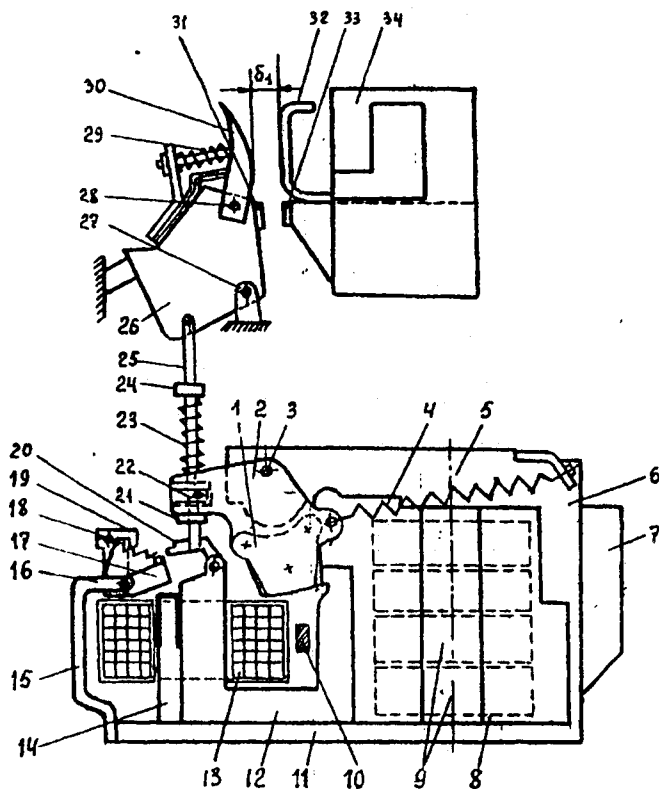
6.13-rasm. VAB-43 turidagi uzgichning elektr magnitli mexanizmi va asosiy kontaktlar bloki: 1—qo'zg'aluvchi yakor; 2—yonboshlar; 3, 16, 22, 27, 28—o'qlar; 4—uzuvchi prujina; 5—yuqori to'sin; 6—asos; 7—rostlanuvchi planka; 8—o'zak; 9—ushlovchi g'altak; 10—shina; 11—pastki to'siq; 12—magnit o'tkazgich; 13—boshqarish g'altagi; 14—erkin ajralish mexanizmi o'zagi; 15—qisqich; 17—yakor; 18, 29—prujina; 19—zashchelka; 20—richag; 21, 24—tirgak; 23—qisish prujinasi; 25—tortish; 26—qo'zg'aluvchi kontakt; 29, 30, 32—yoy so'ndirgich kontaktlari; 31, 33—kontaktning kumushlangan uchlari; 34—qo'zg'aluvchi kontakt.
