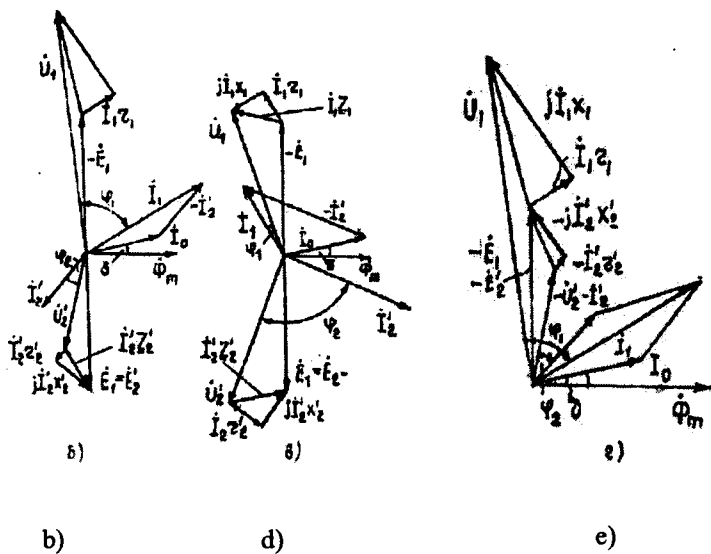
9.6-rasm. Transformatorning ekvivalent sxemasi (a), potentsial (e) va vektor diagrammalari: b — aktiv induktiv yuklama uchun; d — aktiv sig'im yuklama uchun.
