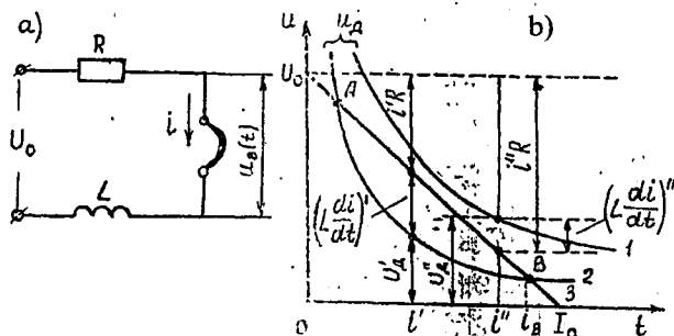
4.2-rasm. O'zgaras tok yoyining so'ndirilishi.
