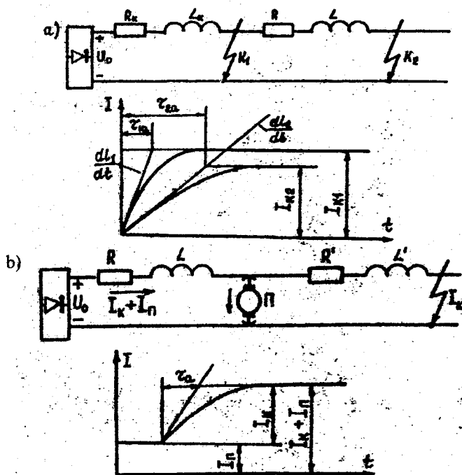
2.7-rasm. Tortish tarmog'i yuklamasiz ishlaganda (a) va yuklama bilan (b) ishlagandagi QT toklarining grafiklari.
