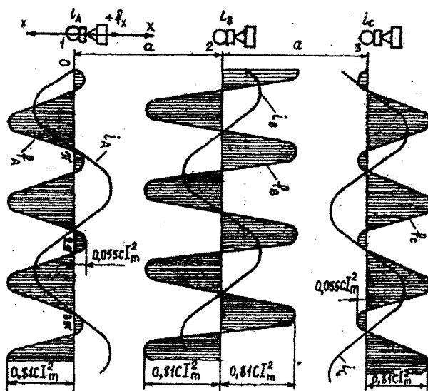
2.10-rasm. Uch fazali tizimdagi elektrodinamik kuchlar.
