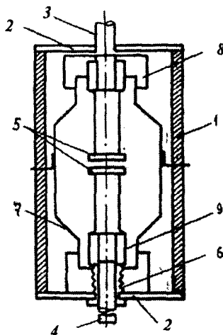
5.17-rasm. Vakuum kamerasing tuzilishi: 1 — dielektrik qoplam; 2 — yon boshmoqlar; 3 — qo'zg'almas kontakt; 4 — qo'zg'aluvchi kontakt; 5 — kontaktlar (elektrodlar); 6 — po'lat qovurg'ali sifon; 7 — parni kondensatsiyalash ekrani; 8 — yon ekran; 9 — o'zak ekрани.
