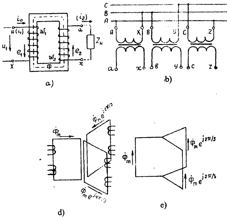
9.1-rasm. Transformatorning ishlash tamoyili:
