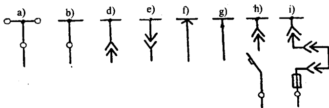
8.14-rasm. Past kuchlanish tarmoqlanuvchi shinalar sxemasi:
