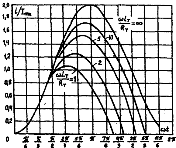
9.27-rasm. Tashqi qisqa tutashgan to'g'rilagich toklarining qiymatlari diagrammalari.
