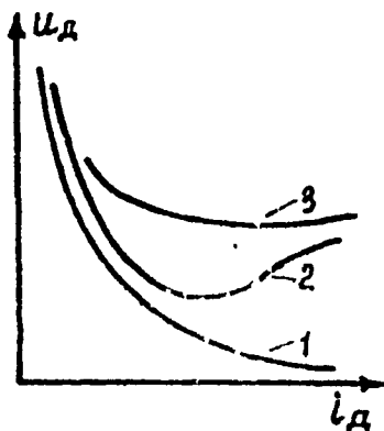
4.8-rasm. Ochiq yoy (1), teshik kamerali yoy (2) va yoy soʻndirgich turli usullarga taalluqli volt-amper tavsiflar.
