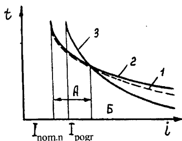
8.1-rasm. Himoyalagich va himoyalanuvchi obyekt tavsiflarining muvofiqlashuvi.
