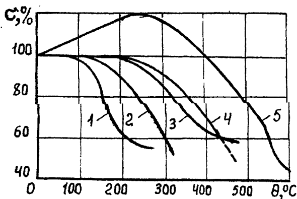
1.8-rasm. Material pishqlik chegarasining haroratga bog'liqligi: 1 – elektrolitik mis (uzluksiz rejim); 2 – aluminiiy; 3 – elektrotexnik mis (qisqa rejim); 4 – bronza; 5 – po'lat.
