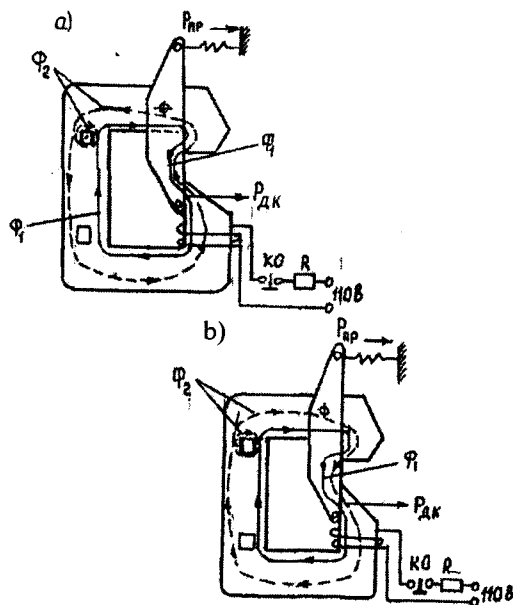
6.5-rasm. VAB—28—K turidagi uzgich elektr magnetida magnet oqimlarining yo‘nalishi: a — tok teskari yo‘nalishda oqqanda; b — tok turi yo‘nalishda oqqanda; F_1 — ushlovchi g‘altak tokidan hosil bo‘lgan magnet oqimi; F_2 — uzuvchi o‘ram tokidan hosil bo‘lgan magnet oqimi.
