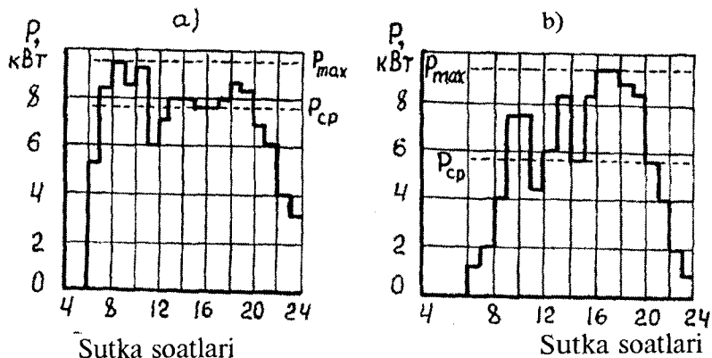
1.3-rasm. Haftaning ishchi kunlariga taalluqli nimstansiyasining sutka soatlari bo'yicha namunaviy yuklama grafigi: a — uch agregatli nimstansiya ( R_{sr}=0,6 \cdot R_{max} ); b — bir agregatli nimstansiya ( R_{sr}=0,5 \cdot R_{max} ).
