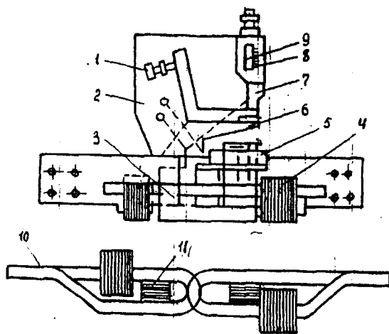
6.9-rasm. Relesi: 1—uzuvchi kontakt; 2—panel; 3,11—magnit oʻtkazgich; 4—plastinkalar; 5—gʻaltak; 6—yakor; 7—prujina; 8—shkala; 9—mil; 10—tok oʻtkazuvchi shina.
