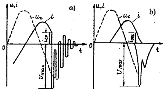
5.4-rasm. Moyli uzgich (a) va elektromagnitli uzgich (b) yordamida kichik qiymatli induktiv yuklama uzilganda tok va kuchlanishlarning o'zgarishi: i_{sr} — qir qilish toki; U_{max} — o'takuchlanish amplitudasi.
