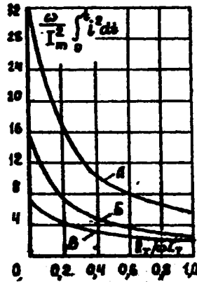
9.33-rasm. Boshqarilmaydigan to'g'rilagich ichki shikastlanganda avariya toklari ekvivalent issiqlik ta'sirining R_T/\omega L_T ga bog'liqlik diagrammalari; A — shikastlangan ventill zanjirida; B va V — shikastlanmagan ventillar zanjirida.
